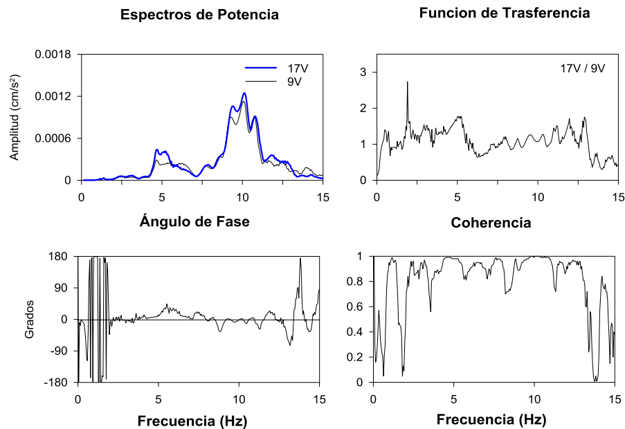
Fig. 4.26 Espectros de la prueba 5c puntos 17 y 9 dirección vertical
