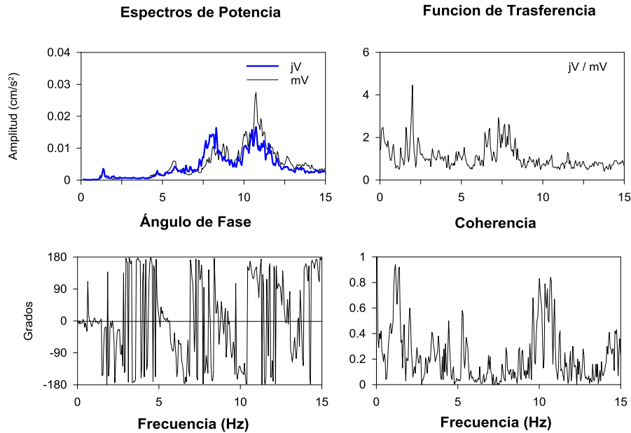
Fig. 4.18 Espectros de los puntos j y m en dirección vertical de la prueba 7
