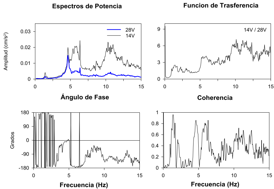
Fig. 4.6 Espectros de la prueba 3 puntos 14 y 28 en dirección vertical
