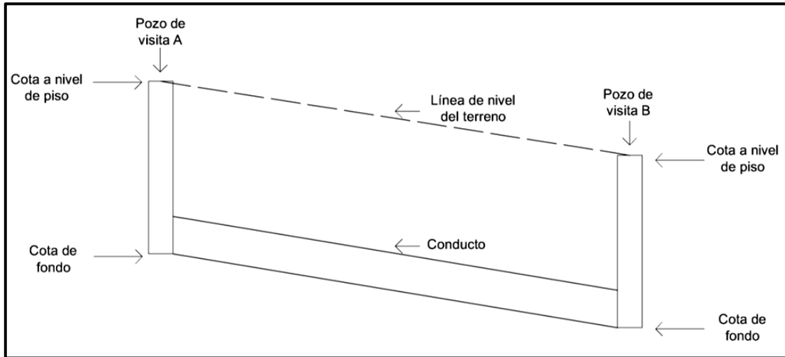
Figura 5.2 Cotras de nivel en un pozo de visita
