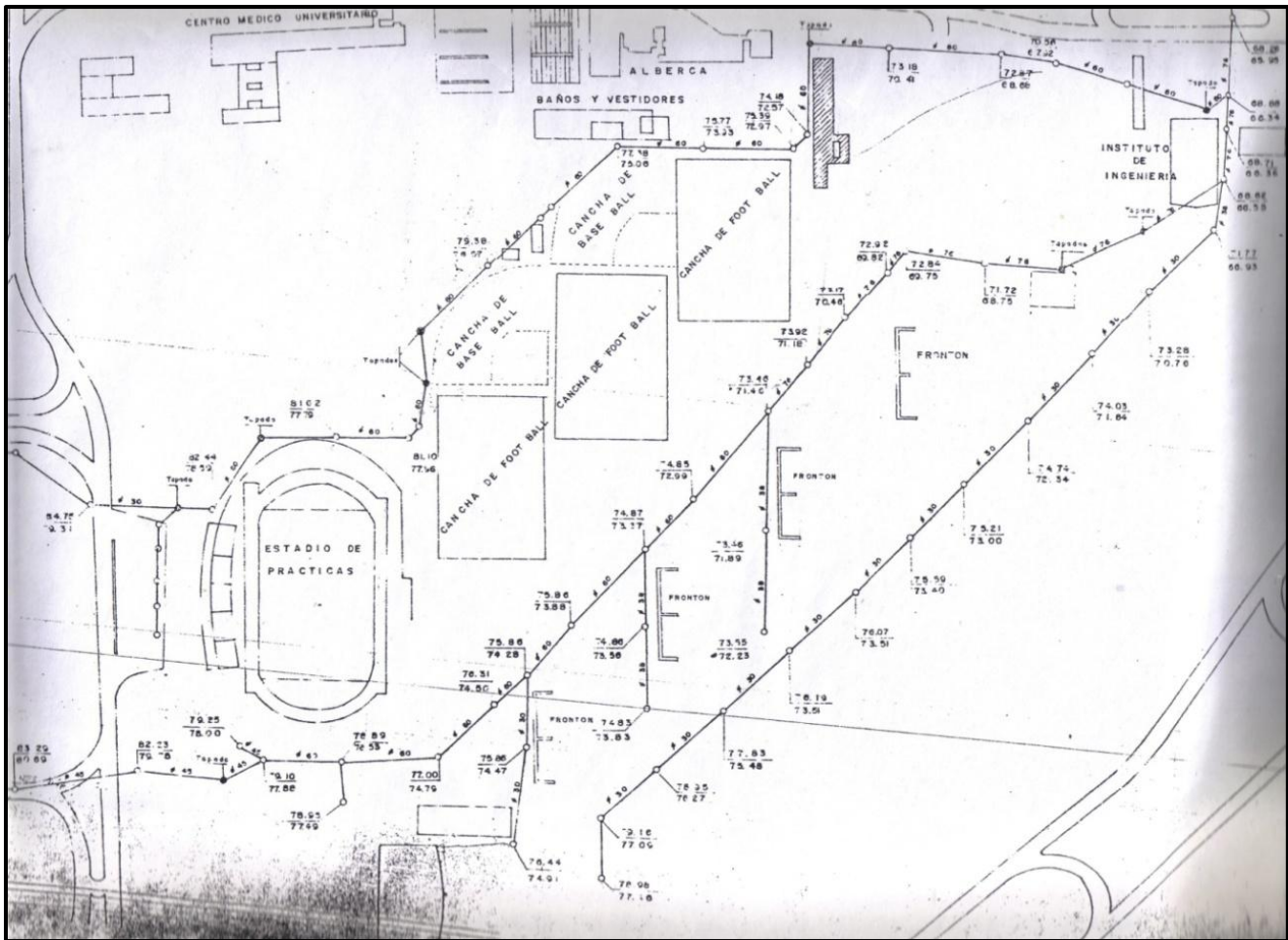
Figura 3.2 Sección del plano brindado por la DGOyC
