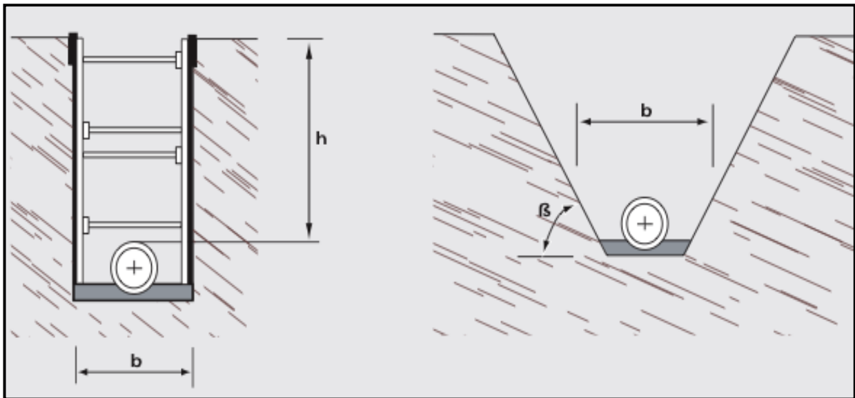
Figura 1.11 Esquema de zanjas para la instalación de conductos
