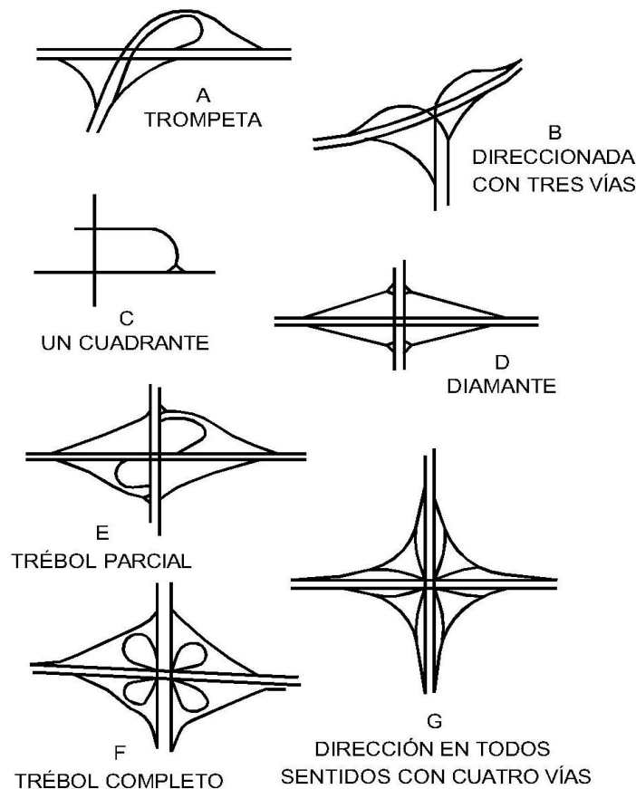
Figura 4.1 Intersecciones a desnivel
