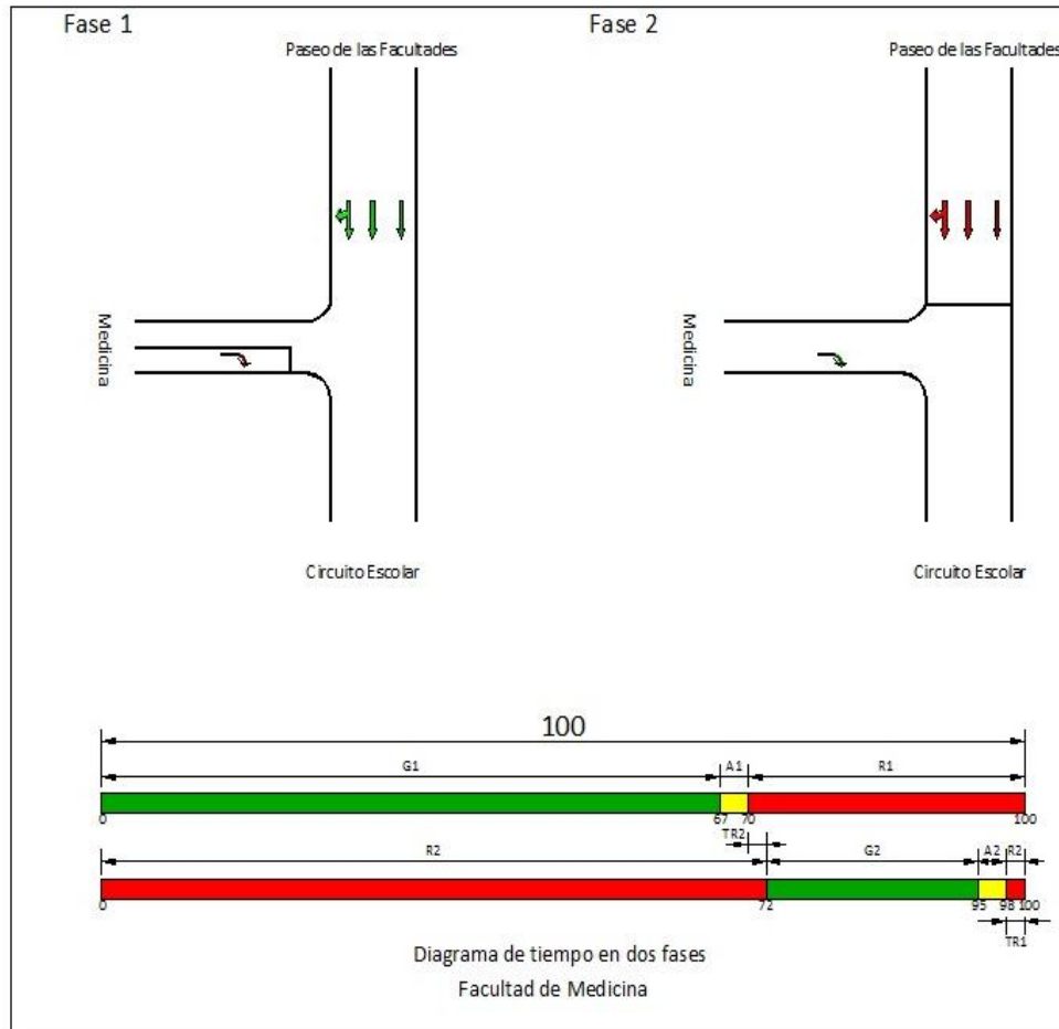
Figura 7.14 Intersección aislada C: fases y diagrama de fases
