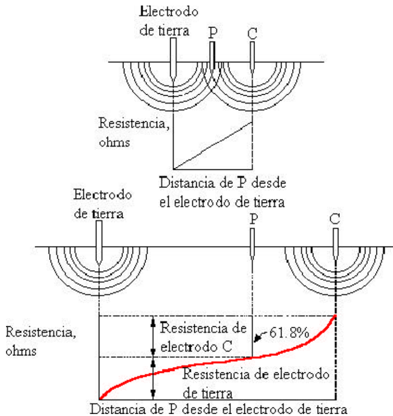
Fig. 29 EFECTO DE LOS CAMPOS ELECTRICOS EN LOS ELECTRODOS DE CORRIENTE
