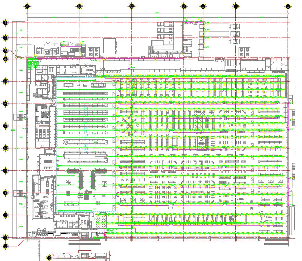
Fig. 3 Plano donde se muestra la distribución de las luminarias en piso de ventas.
