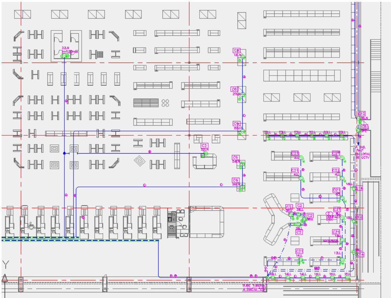
Figura 15. Ubicación de contactos en piso de ventas
