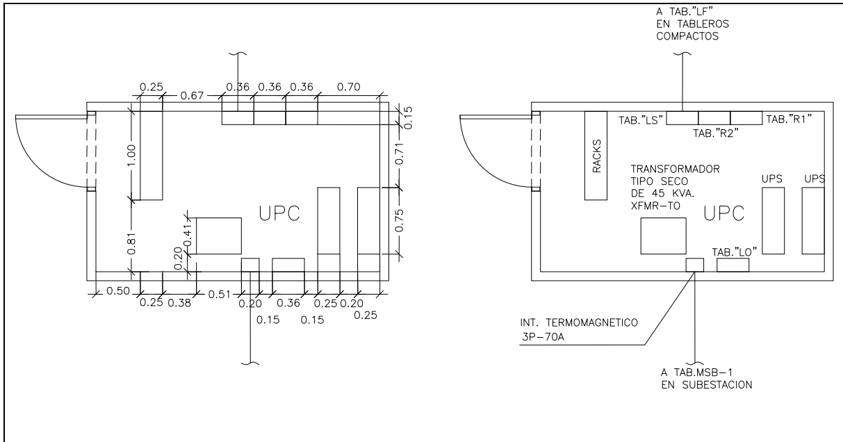
Figura 17. CUARTO DE SISTEMAS IDF
