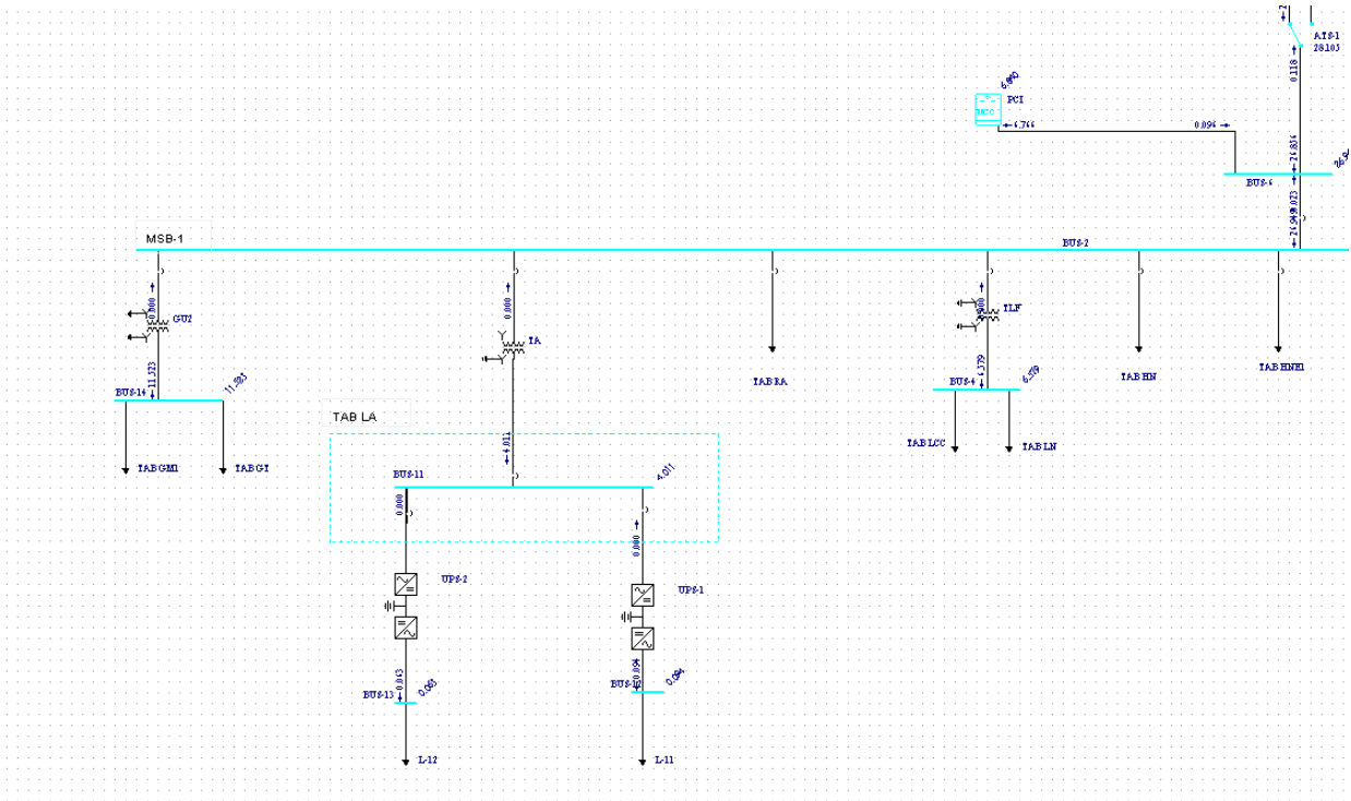
Fig. 35 Estudio de corto circuito en buses del sistema
