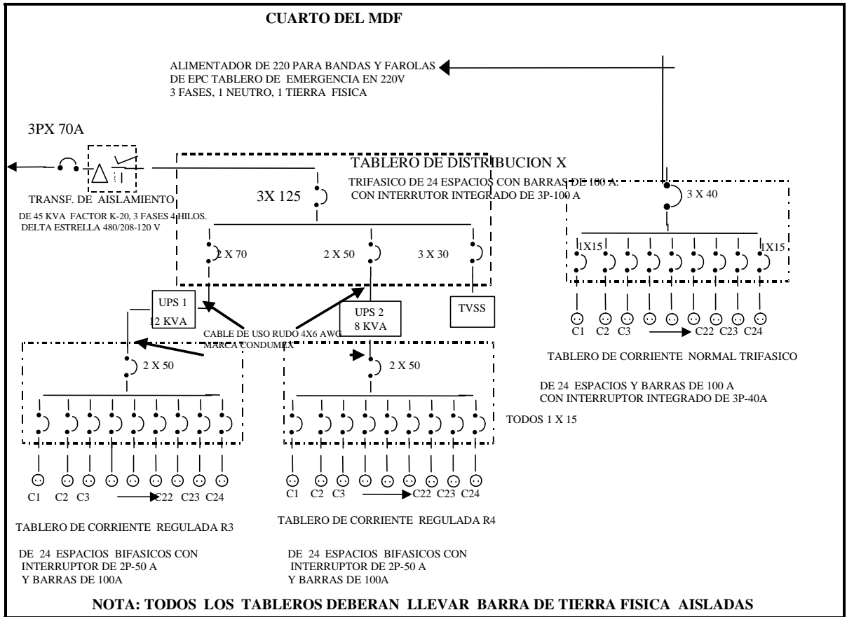
Fig 19. Diagrama Unifilar del sistema de Datos MDF
