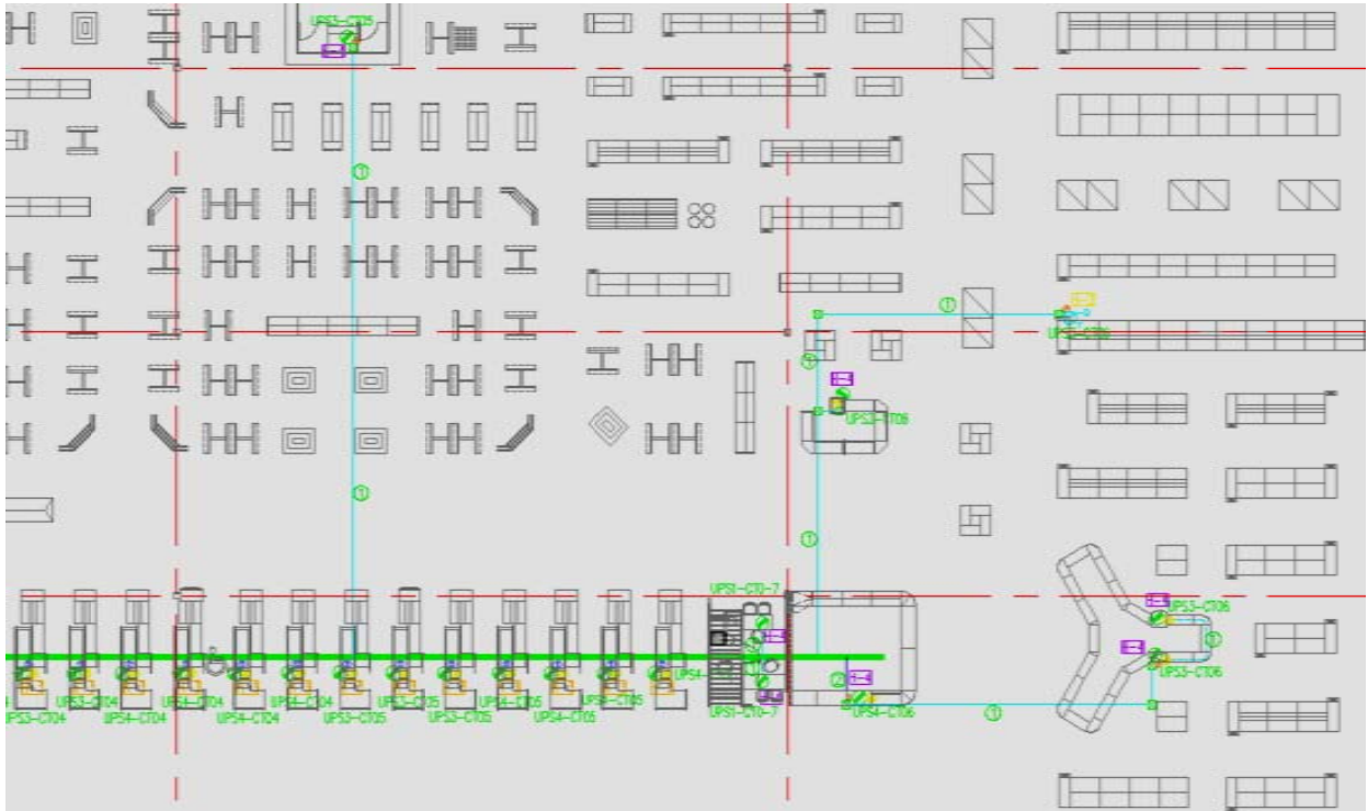
Figura 22. Ubicación de contactos regulados en piso de ventas
