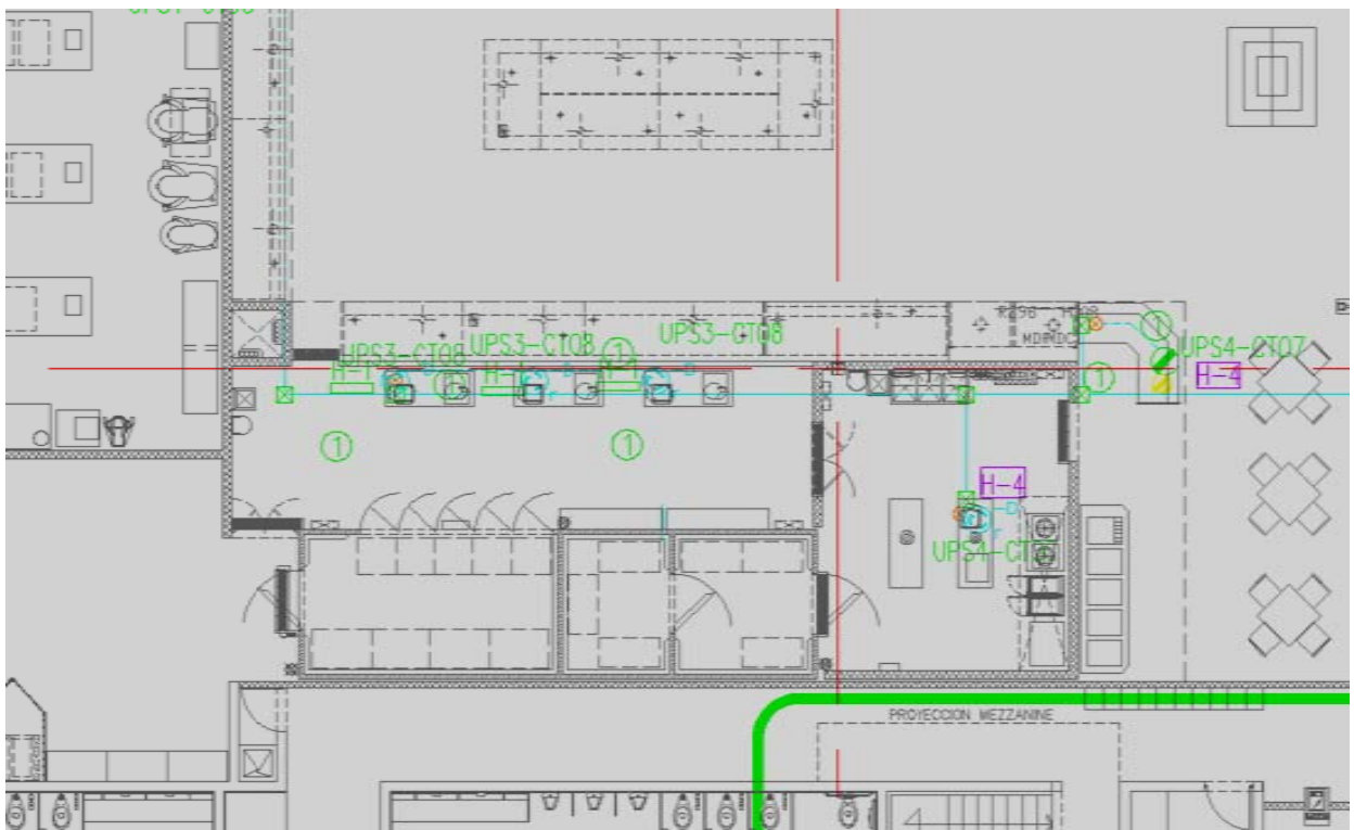
Figura 23. Ubicación de contactos regulados en punto de ventas
