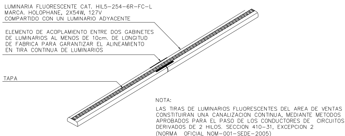
Fig. 2 Arreglo de luminaria en piso de ventas
