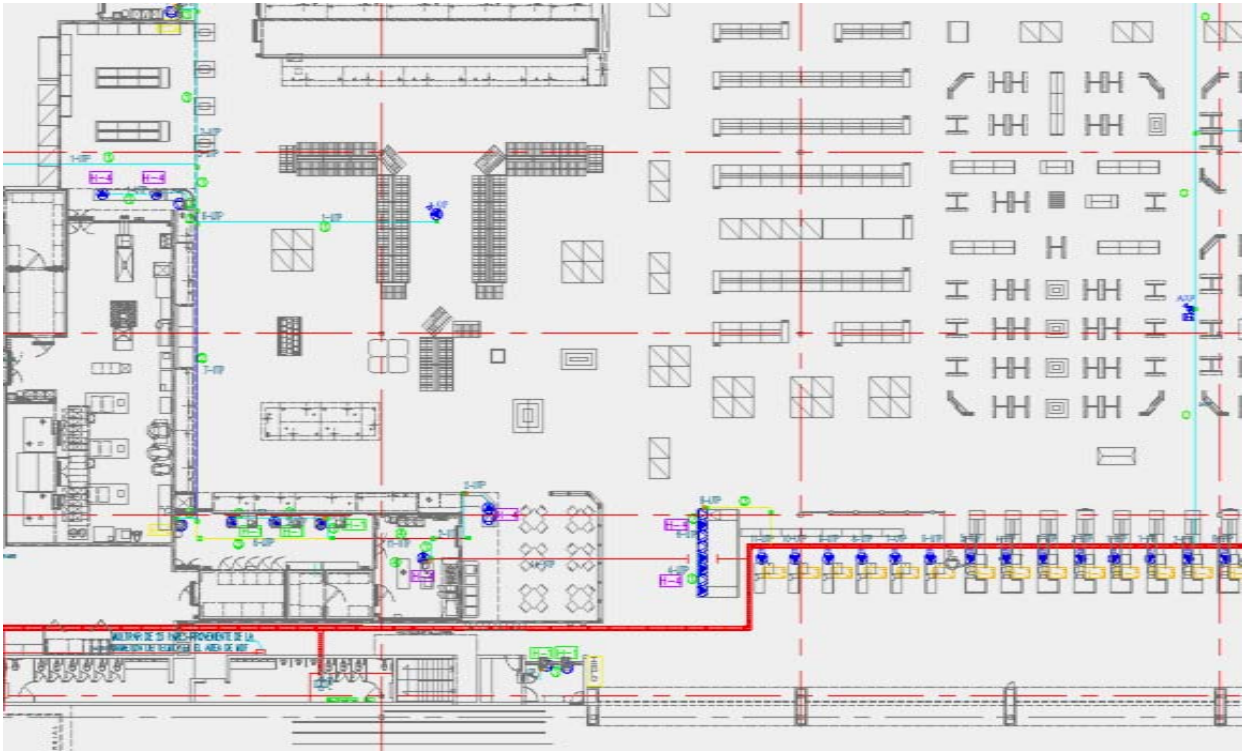
Figura 26. Ubicación de salida de datos en piso de ventas.
