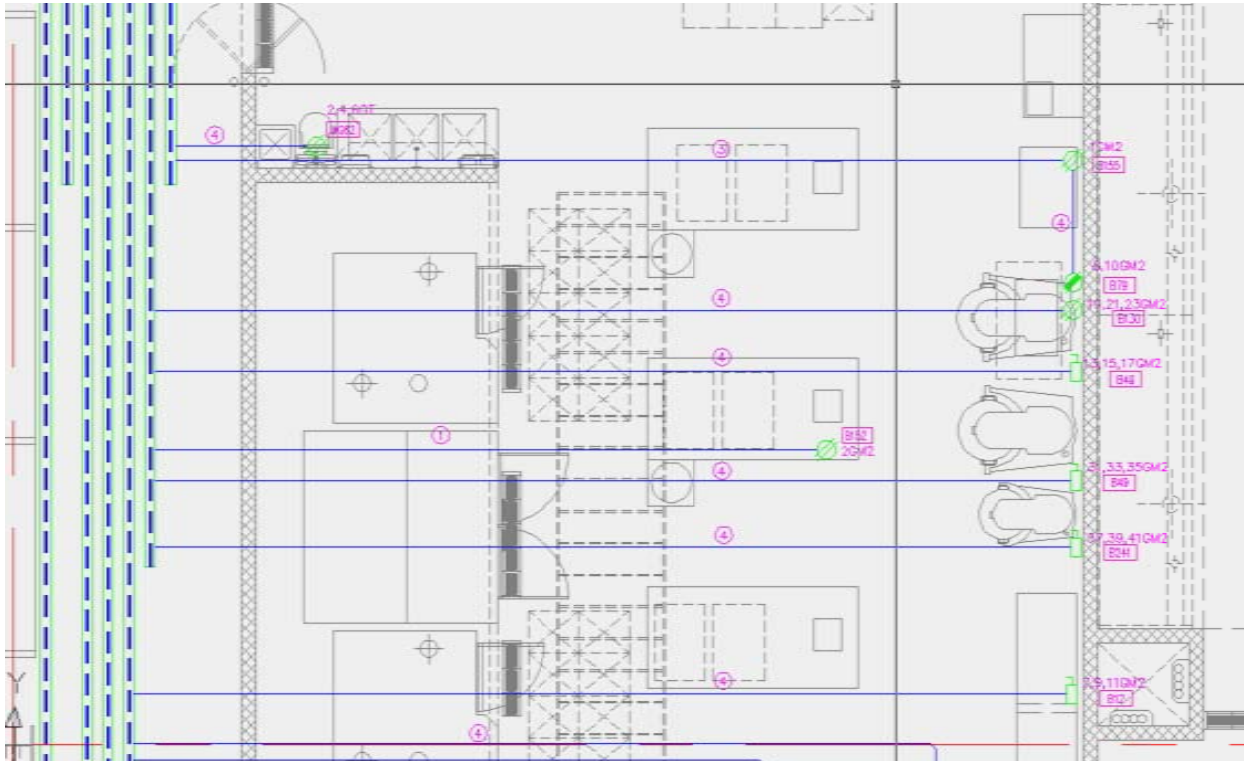
Figura 14. Ubicación de contactos y desconectores en amasijo
