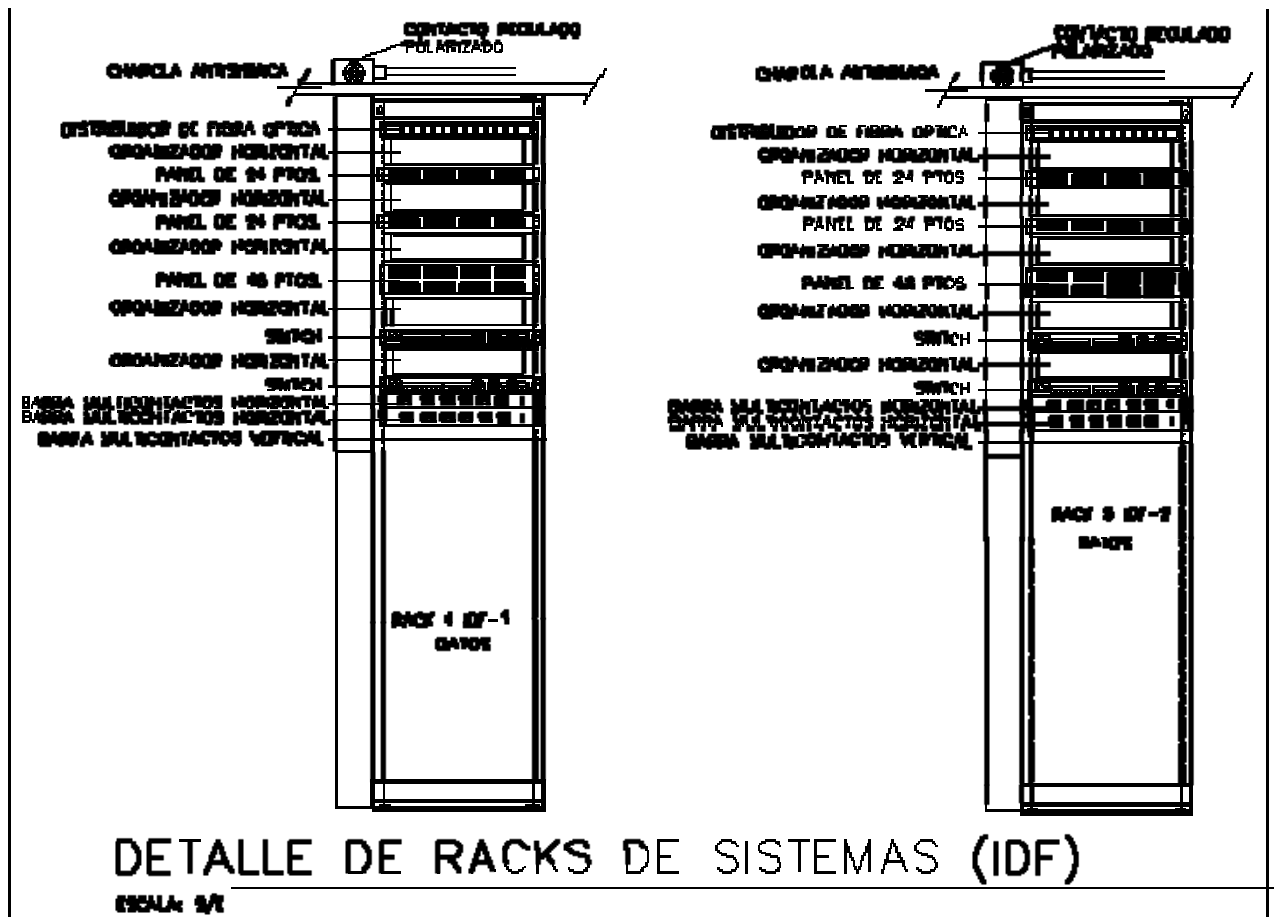
Figura 25 Detalle de Racks de Sistemas
