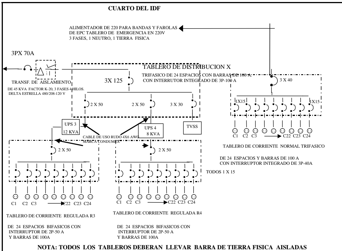
Fig.20 Diagrama Unifilar del Sistema de Datos IDF
