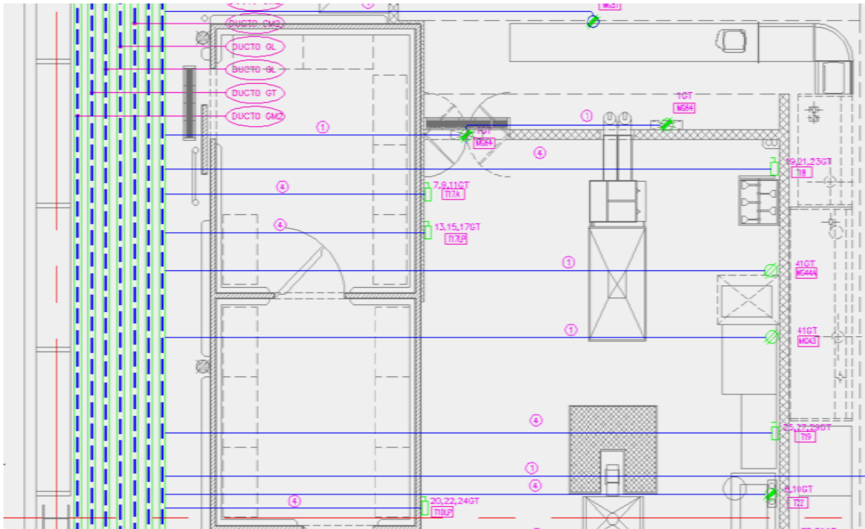
Figura 13. Ubicación de contactos y desconectores en tortillería
