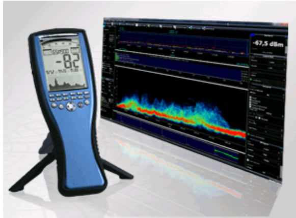
Imagen 84. Medidor Spectran 60100 V4. Fuente: http://www.aaronia.es/ (Consulta: 26 de Noviembre 2011)
