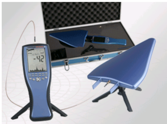
Imagen 82. Medidor Spectran HF-4060 V3. Fuente: http://www.aaronia.es/ (Consulta: 26 de Noviembre 2011)
