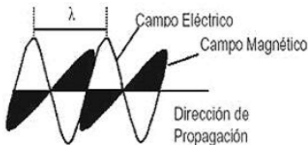
Imagen 1. Onda Electromagnética. Fuente: Normatividad de la Telefonía Móvil en México Relacionada con las Radiaciones Electromagnéticas y sus Riesgos para la Salud, Leonel Alejandro Ordaz Hernández, pág.17.
