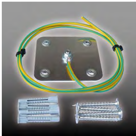
Imagen 62. Toma a tierra para paredes interiores ES. Fuente: electrocontaminación.net (Consulta: 26 de Noviembre 2011)
