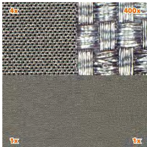
Imagen 52. Filtro HNG80 con diversos acercamientos. Fuente: electrocontaminación.net (Consulta: 26 de Noviembre 2011)
