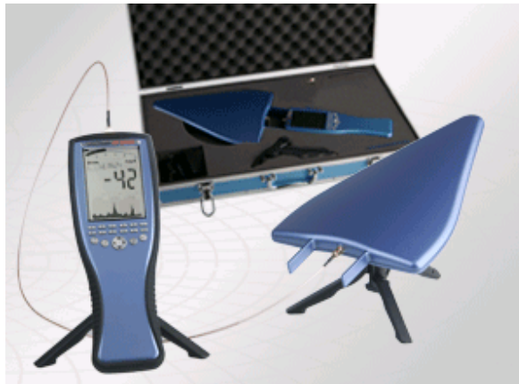
Imagen 81. Medidor Spectran HF-2025E V3. Fuente: http://www.aaronia.es/ (Consulta: 26 de Noviembre 2011)
