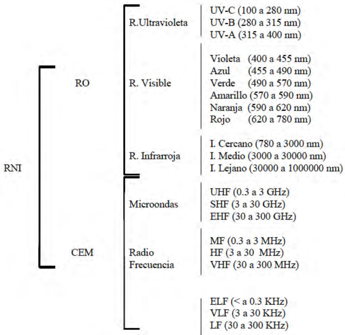
Imagen 3. Clasificación de las radiaciones no ionizantes. Fuente: http://www.bioingenieria.edu.ar/academica/catedras/radiaciones/Descargas/Unidad1.pdf (Consulta: 26 de Noviembre 2011)
