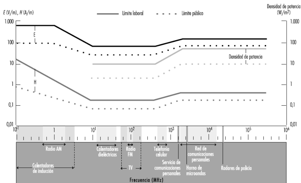
Imagen 16. Límites de exposición según la IRPA (1988) para la intensidad de campo eléctrico E , la intensidad de campo magnético H y la densidad de potencia. Fuente: http://www.irpa.net
