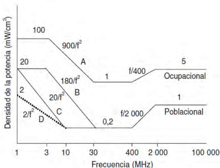
Imagen 15. Valores límite para la densidad de potencia según la frecuencia en Argentina.
