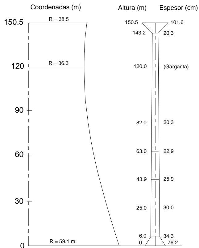
Fig 4.1 Corte en elevación y espesores de la torre de enfriamiento
