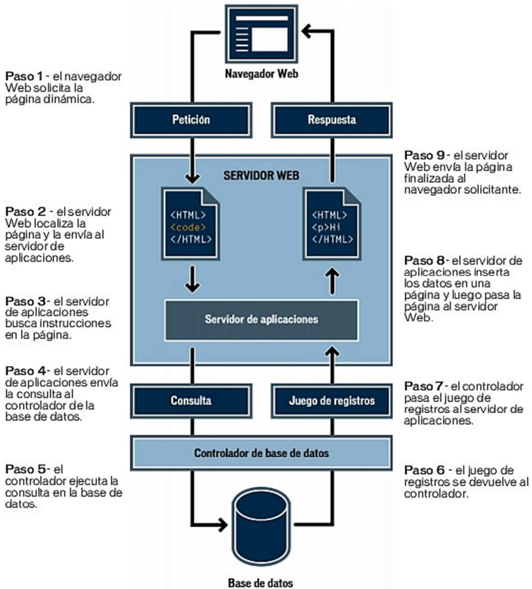
Figura 2.3.3 Proceso del Accesos a una Base de Datos
