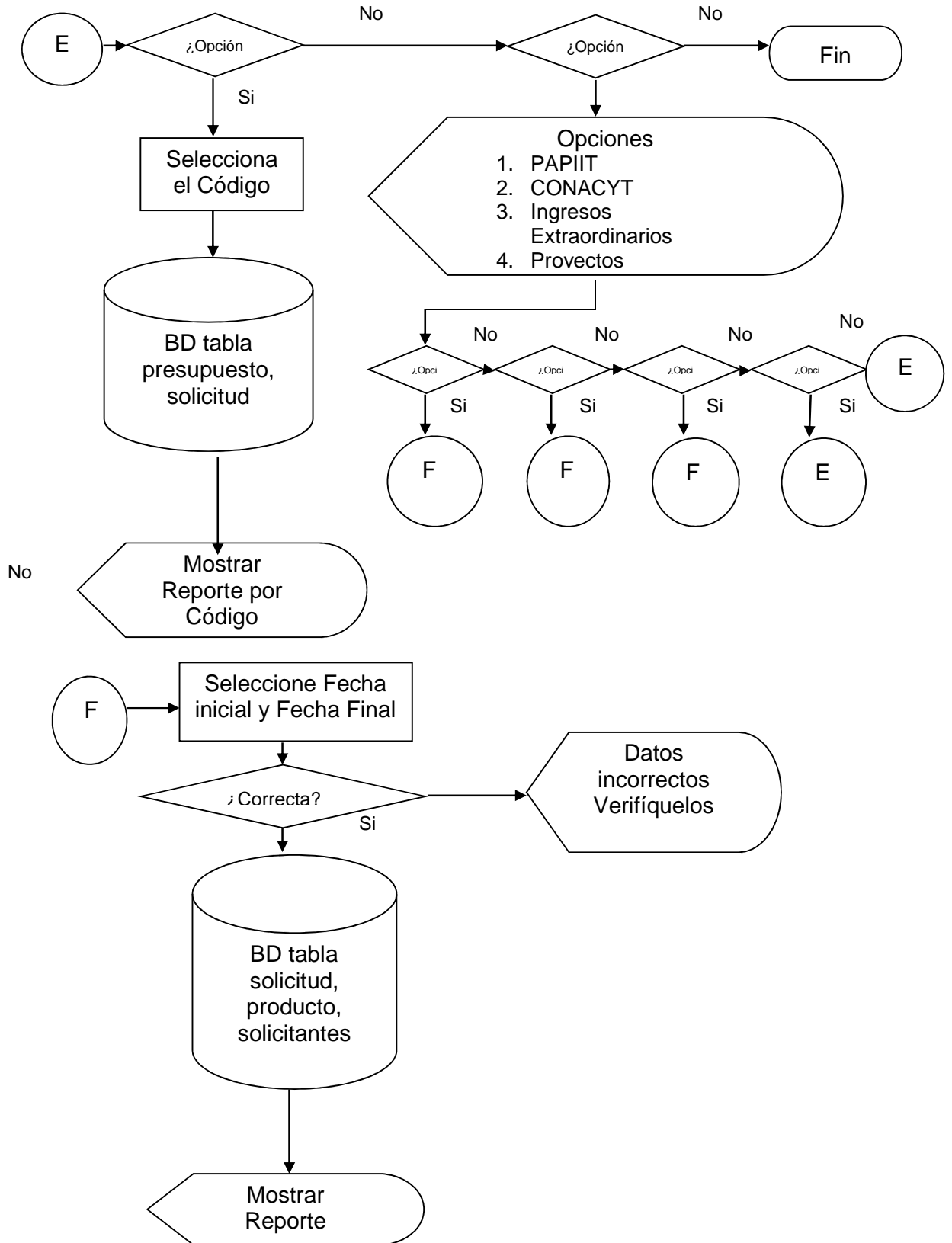
Figura 4.2.1.9. Diagrama de flujo para Reportes de Compra.
