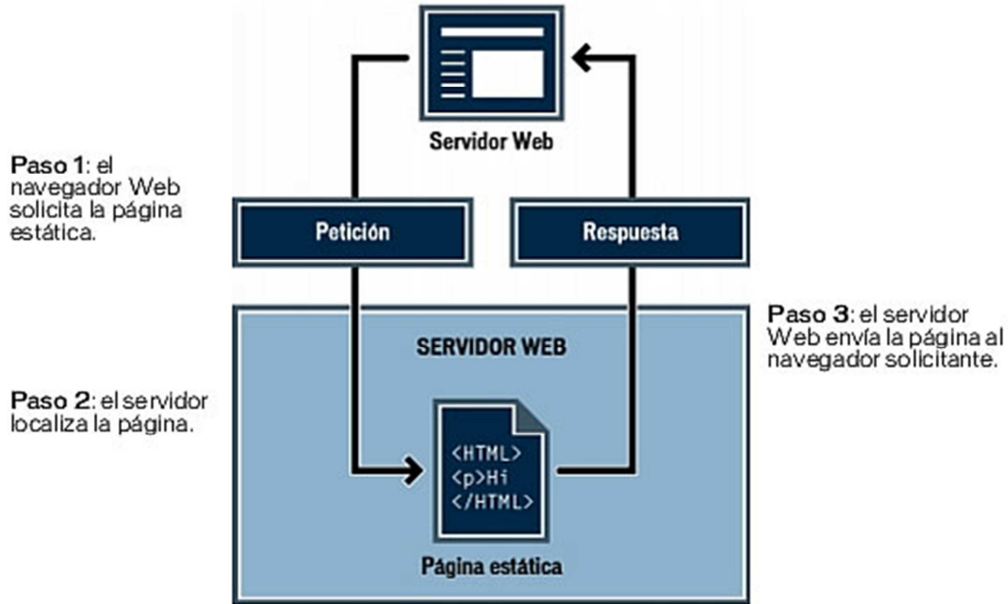
Figura 2.3.1 Procesamiento de una página WEB estática.
