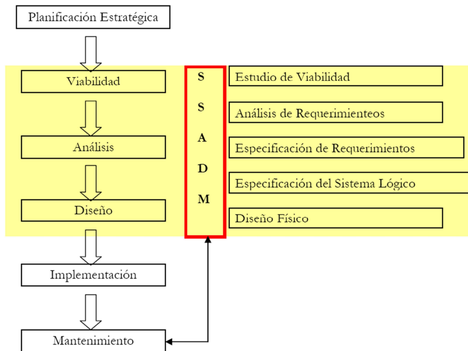
Fig. 4.1.1 Alcance de SSADM
