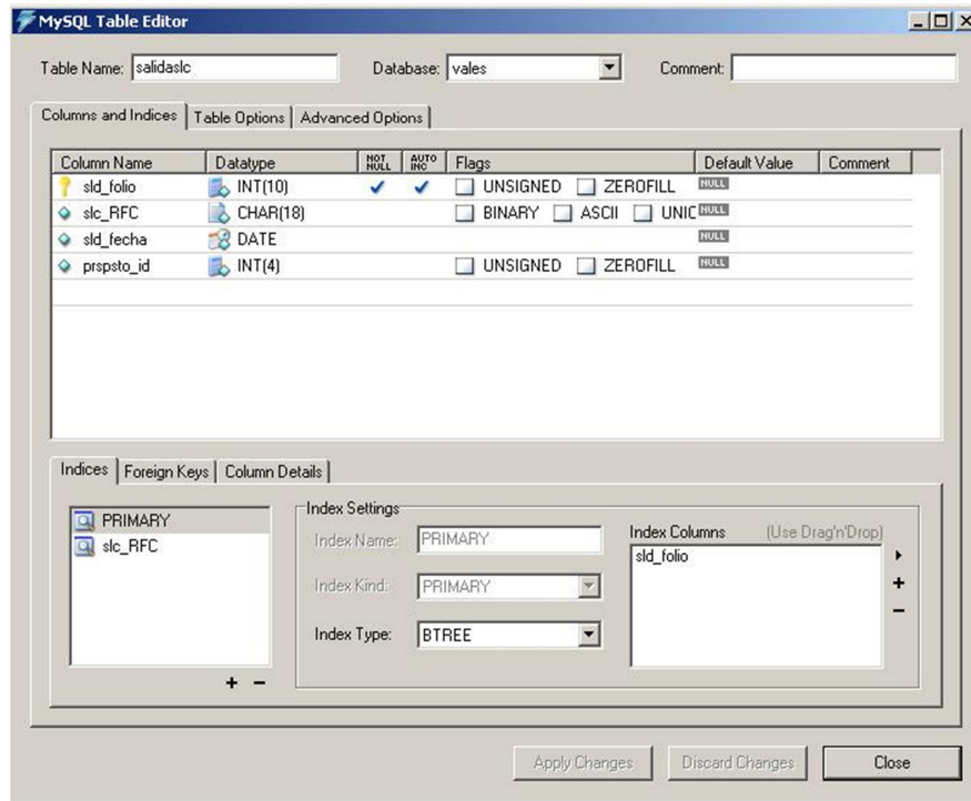
Figura. 4.3.3 Creación de tablas con MySQL Query Browser
