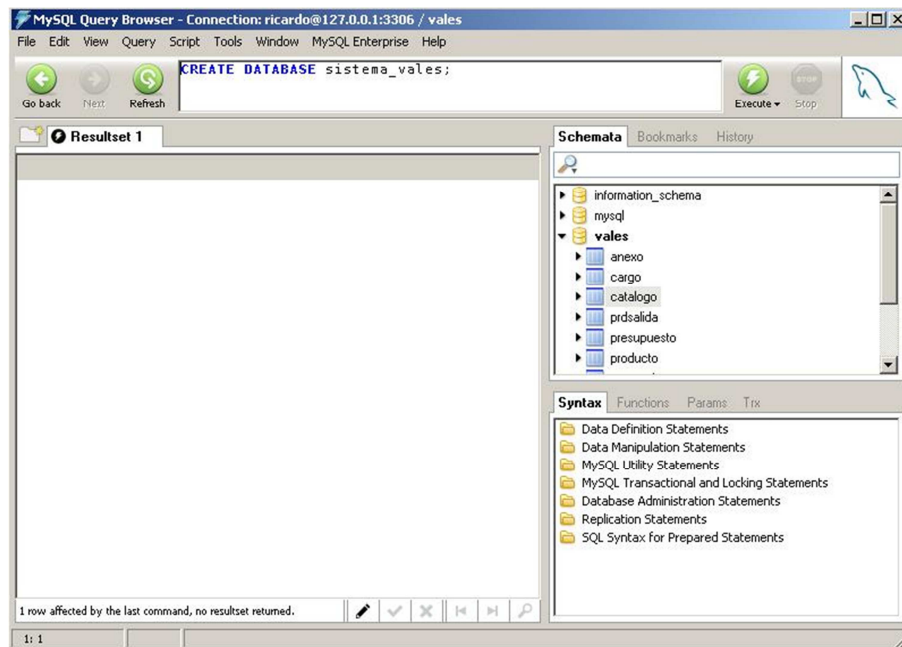
Figura. 4.3.1 Creación de la base de datos
