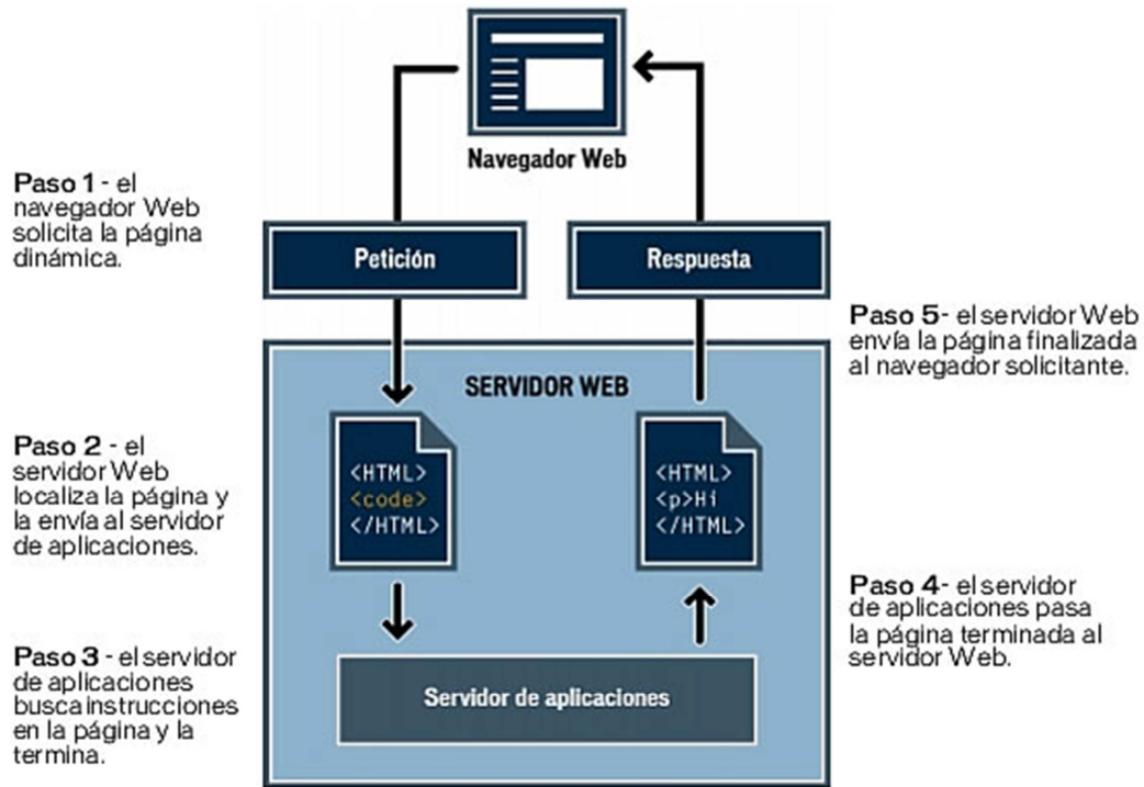
Figura 2.3.2 Procesamiento de una página WEB dinámica.
