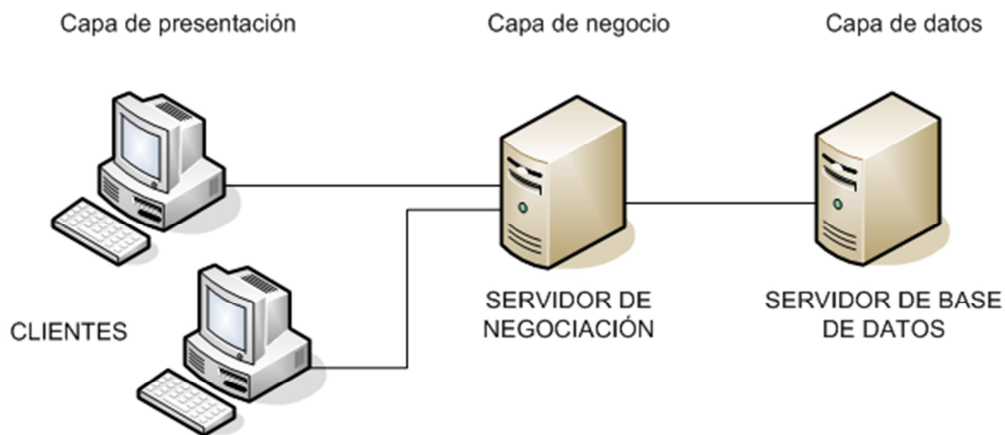
Fig. 2.8.3 Aplicación Cliente/Servidor de tres capas
