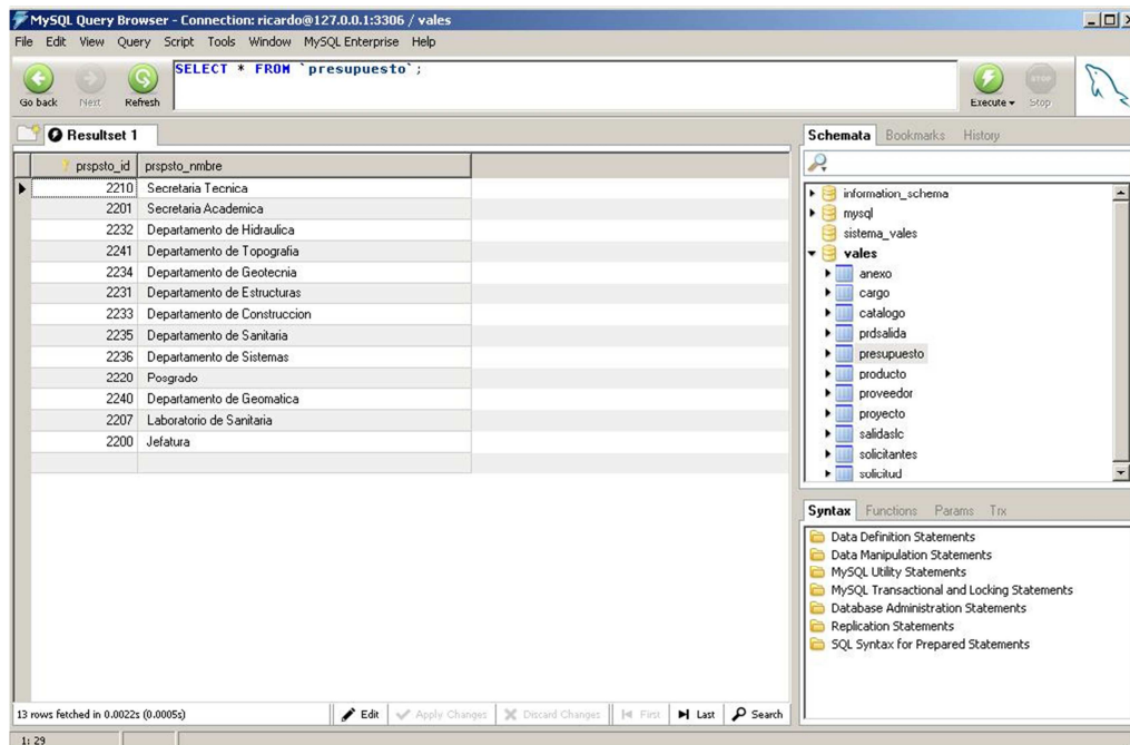
Figura. 4.3.7 Sentencia SELECT
