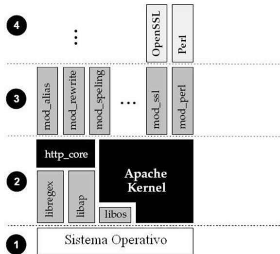
Fig. 2.5.3 Arquitectura de Apache
