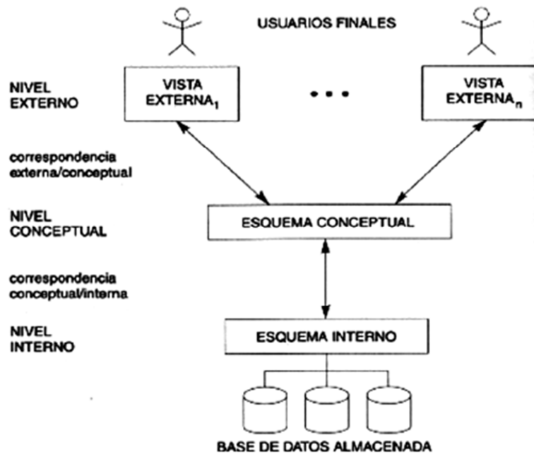
Figura 2.1.1 Niveles de abstracción de un DBMS.
