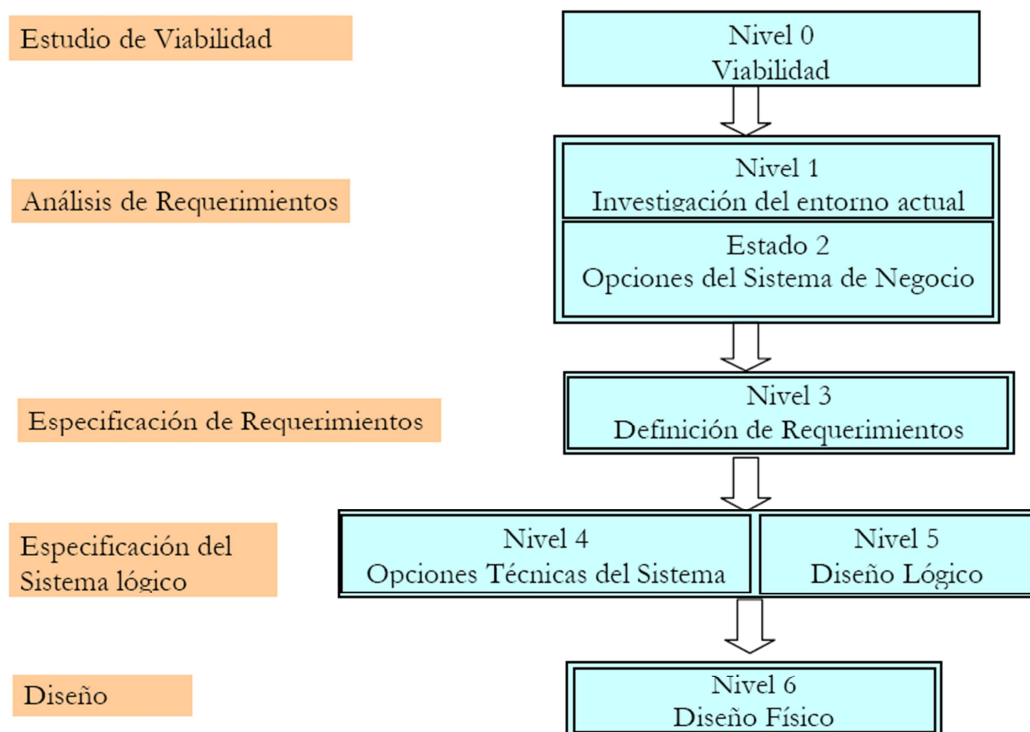
Figura. 4.1.2 Estructura de SSADM.
