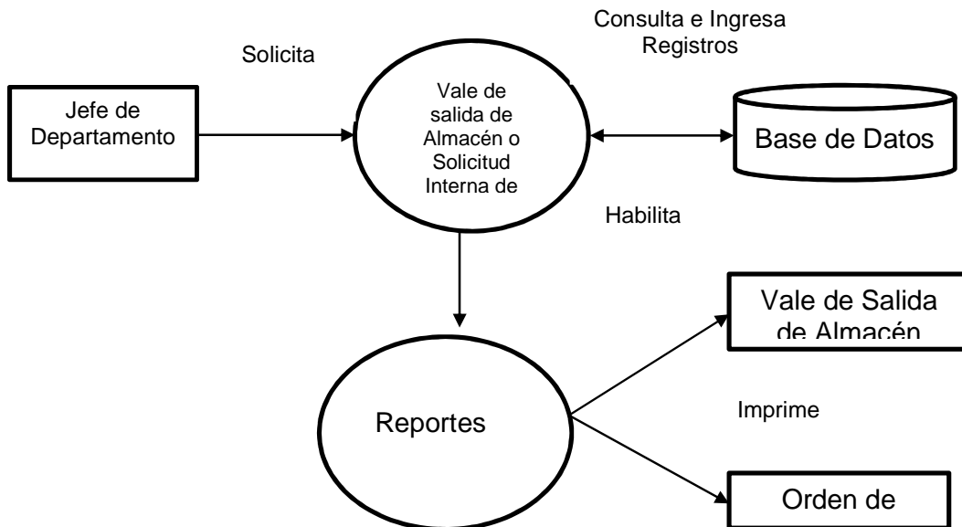
Figura 4.2.1.4 Proceso de solicitud de vale de compra o salida de almacén.
