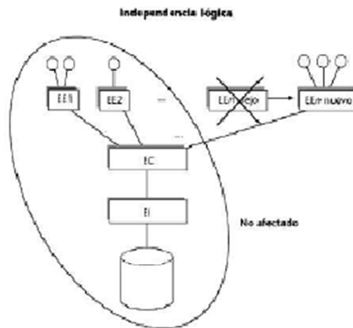
Figura 2.1.3 Hay independencia lógica cuando los usuarios (programas de aplicación o usuarios directos) no se ven afectados por los cambios en el nivel lógico.
