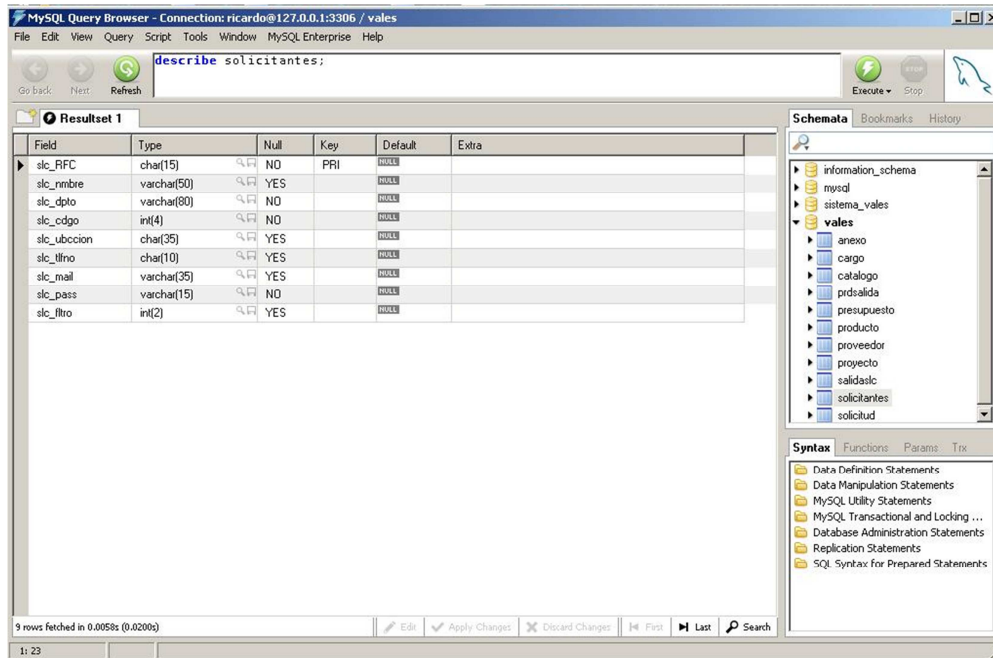
Figura. 4.3.4 Descripción de tabla solicitantes
