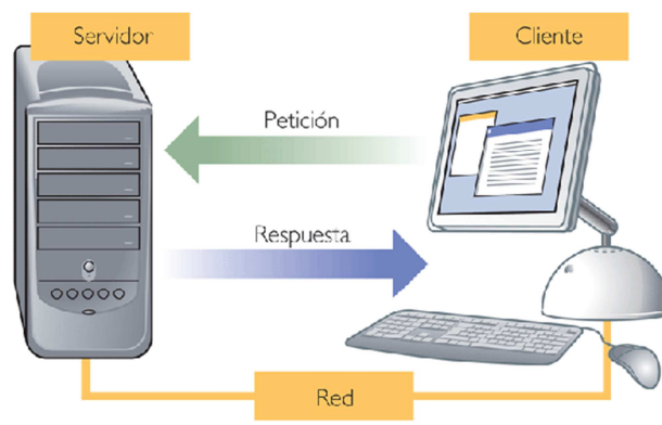
Fig. 2.8.1 Modelo Cliente/Servidor
