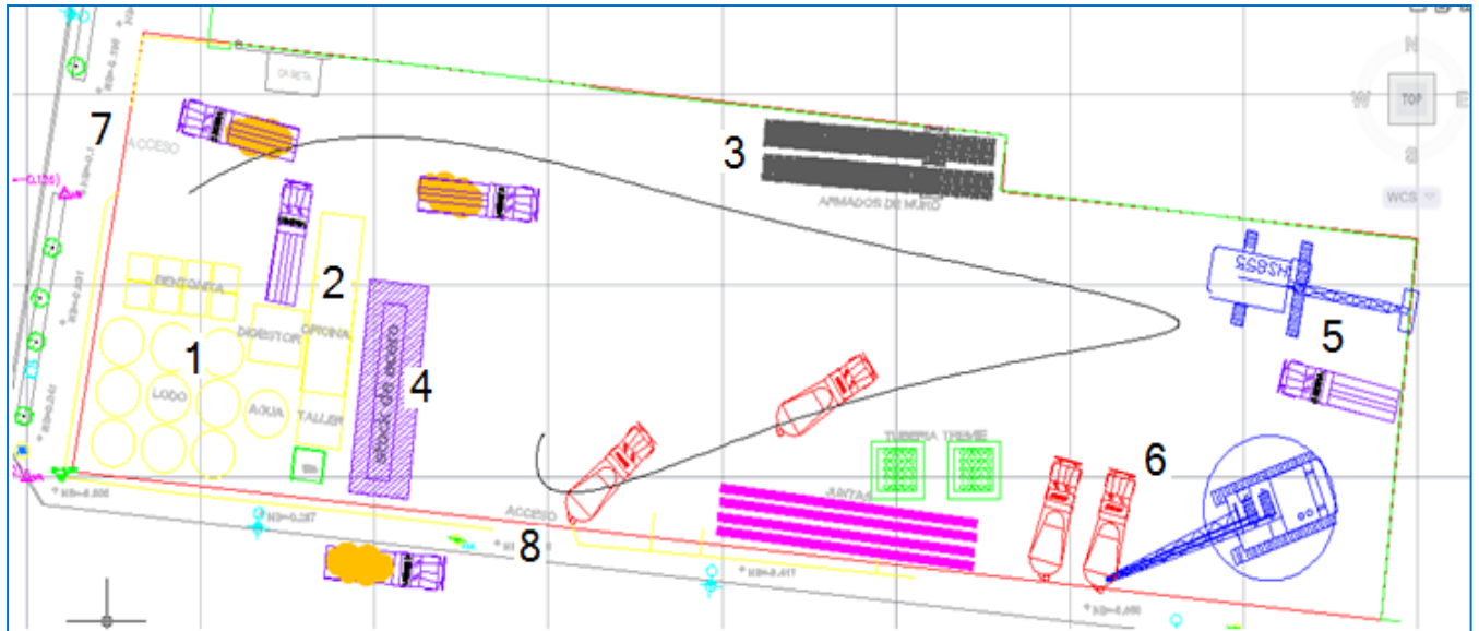
FIGURA NO. 1 Plano de logística de la obra
