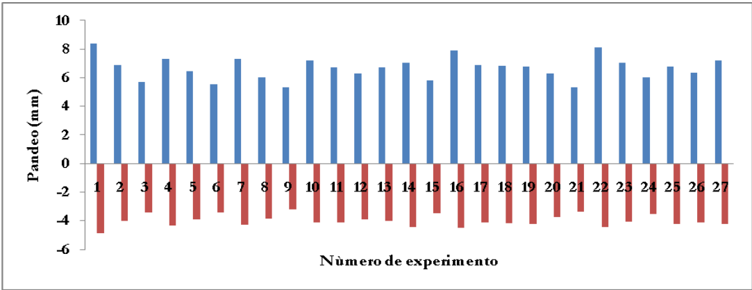
Figura 5.2. Resultados de Pandeo.
