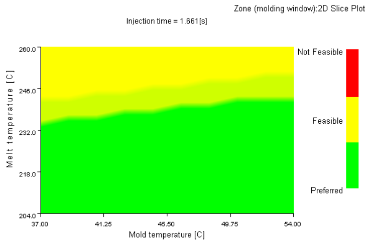
Figura 4.4. Ventana de procesamiento ( Moldflow ).
