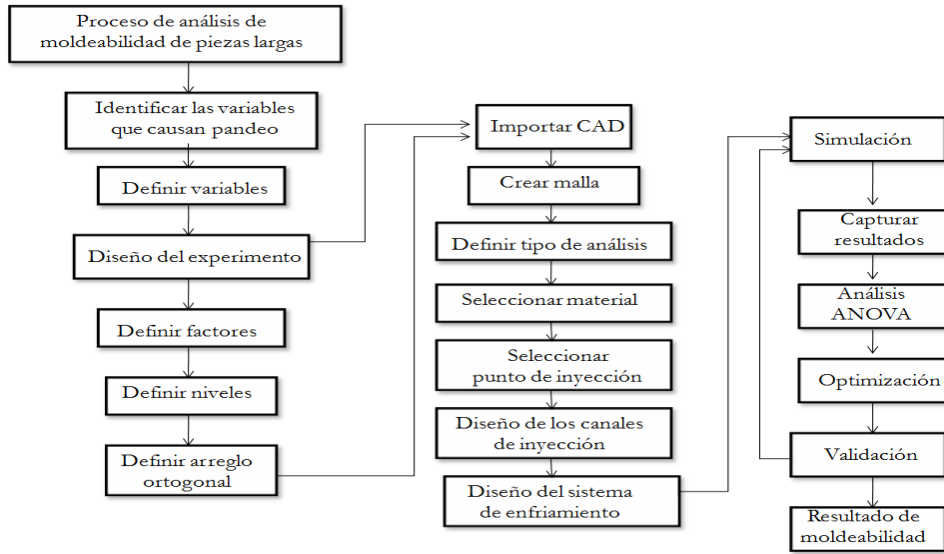
Figura 4.1. Proceso de análisis de moldeabilidad de piezas largas.
