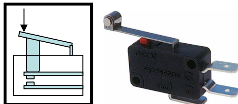
Figura 2.2 Microinterruptor de palanca con rodillo.
