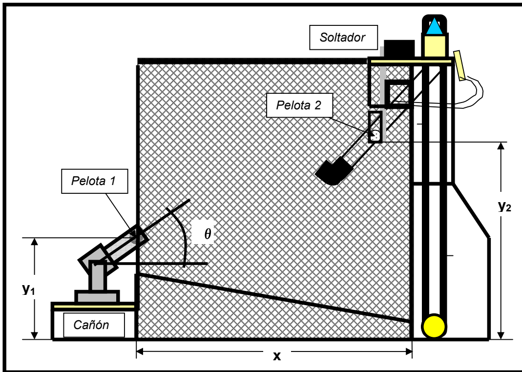
Figura 1.1 Ilustración del sistema.
