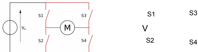
Figura 2.17 Estructura del puente H.
