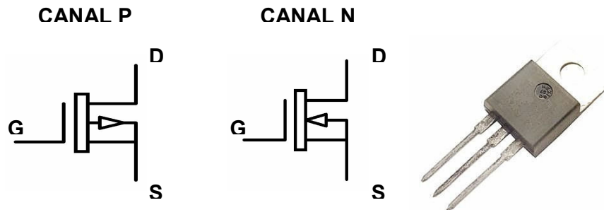
Figura 2.15 Tipos de MOSFET (izq.) y encapsulado (der.).
