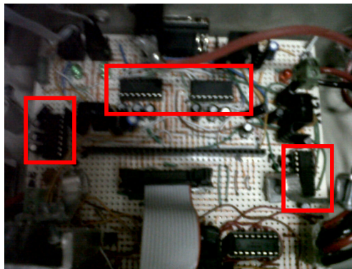
Figura 5.15 Tratamiento de entradas para el circuito de control.
