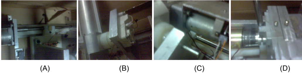
Figura 1.3 Actuadores del subsistema de tiro. (A. tornillo sinfín, B. motor angular, C. motor de tensión, D. trinquete)
