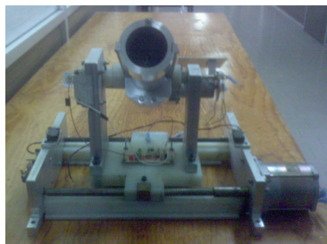
Figura 1.2 El subsistema de tiro.
