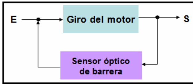
Figura 5.3 Esquema de control para el conteo de vueltas.
