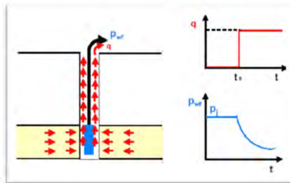
Figura 3.12. Prueba de decremento de presión.
