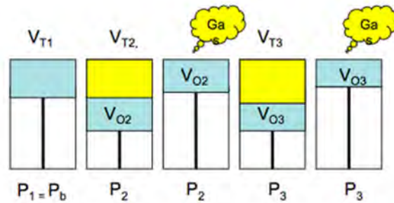
Figura 3.5. Separación diferencial.
