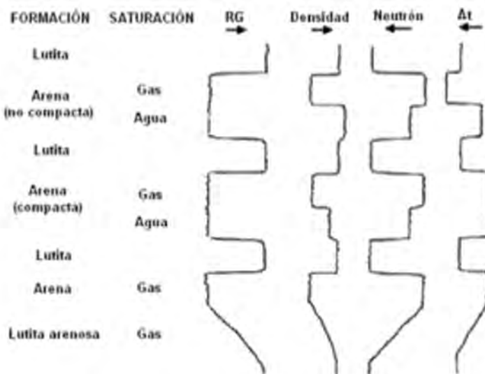
Figura.3.9. Influencia del gas en registros de porosidad.
