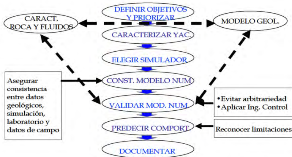
Figura 4.13. Esquema de la simulación numérica de yacimientos.
