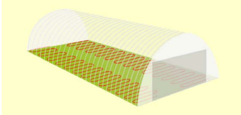
Fig.12.- Calefacción en un invernadero mediante parrillas.
