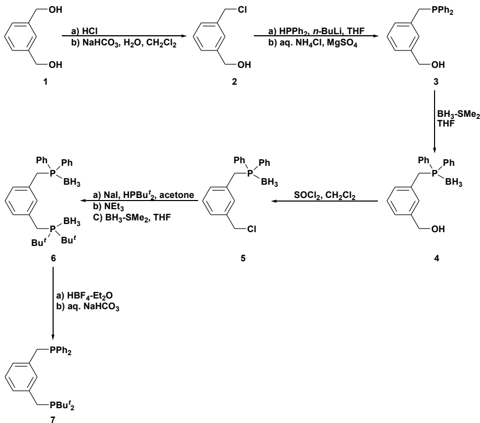
Esquema 8. Síntesis del ligante no simétrico {C 6 H 4 -1-(CH 2 Bu t ) 2 }-3-(CH 2 PPh 2 )}.
