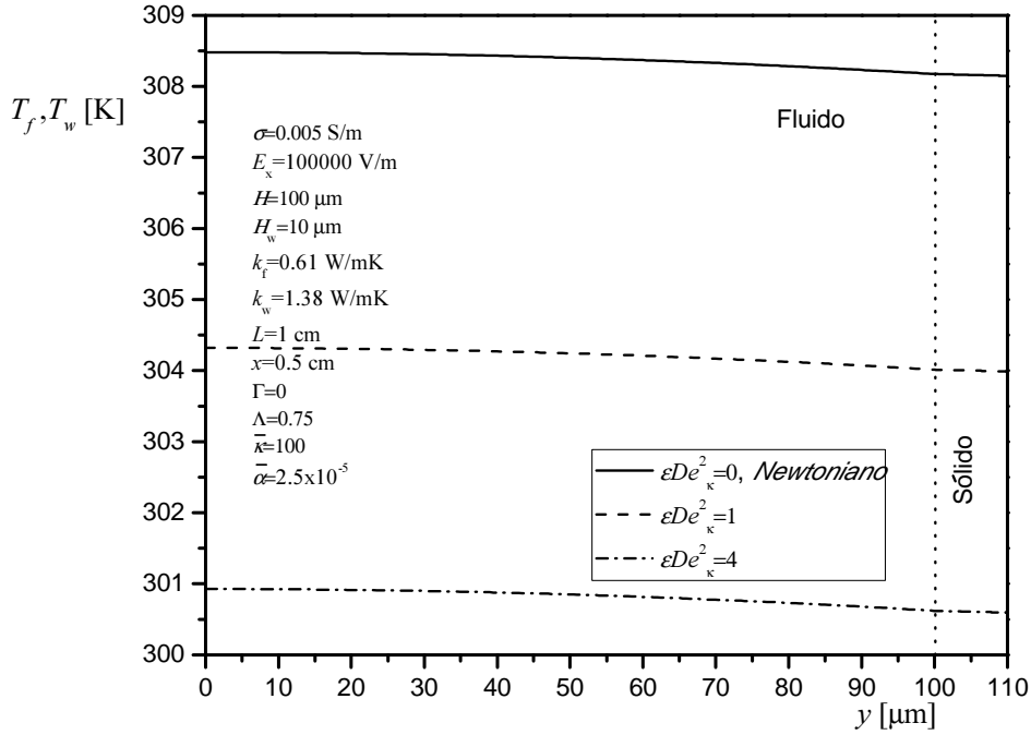
Figura 5.11. Perfil de temperatura como función de la coordenada transversal del microcanal en las regiones del fluido y sólido, en x = 0.5 \text{ cm} , para diferentes valores de \varepsilon De_x^2 y \sigma = 0.005 \text{ S/m} .
