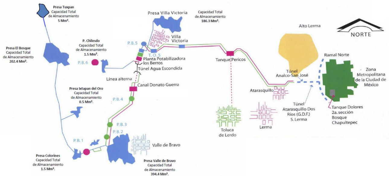
Figura 2. 3 Componentes del Sistema Cutzamala
