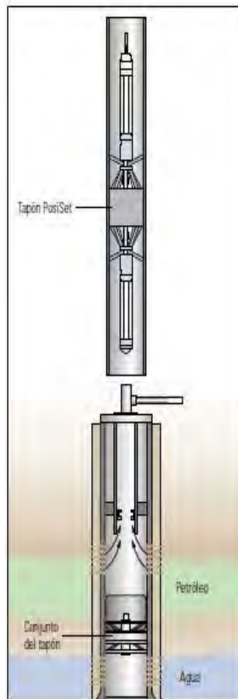
Fig. 2.5.1 Herramienta PosiSet
