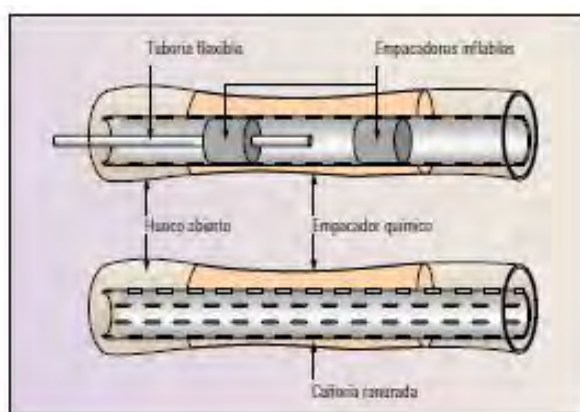
Fig. 2.5.5 Empacador Químico Anular (ACP)
