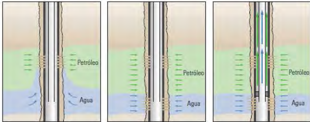
Fig. 2.5.10 Drenaje Doble
