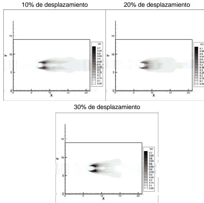
Figura 42. Contornos de las fluctuaciones u'u' para la frecuencia natural con desplazamiento de 10% (arriba izquierda), desplazamiento de 20% (arriba derecha), desplazamiento de 30% (abajo).
