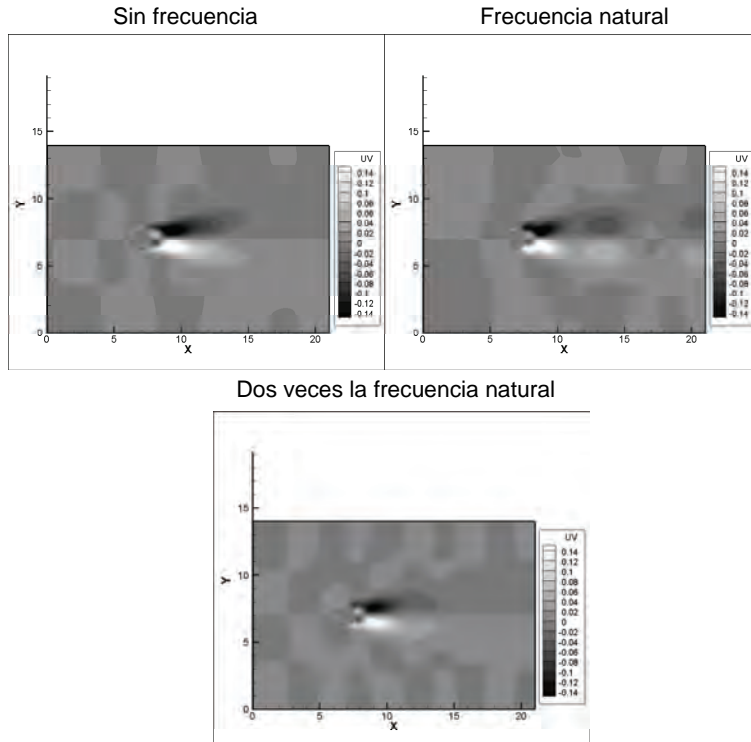
Figura 47. Contornos de las fluctuaciones u' y v' para las frecuencias cero (arriba izquierda), frecuencia natural (arriba derecha), doble de la frecuencia natural (abajo).
