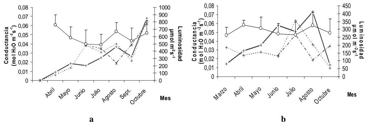
Figura 32. Promedios de luminosidad \circ en la nave sin sombra (a) y con sombra 70% (b) del invernadero en comparación con la conductancia estomática de L. graveolens (—), G. glutinosum (.....) y C. tortuosa (- - -)
