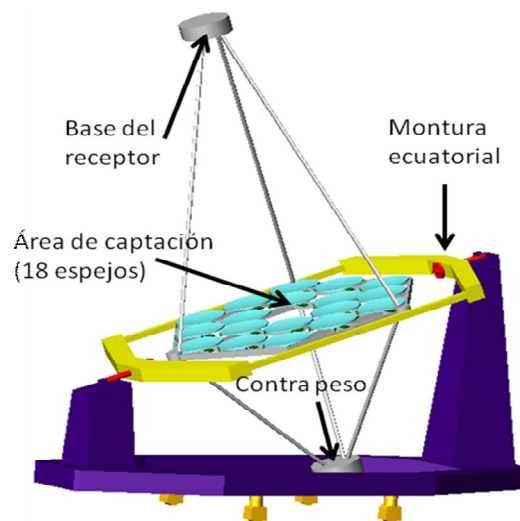
Figura 1.9. Diagrama del Dispositivo Experimental de Flujo Radiativo Altamente Concentrado (DEFAC).
