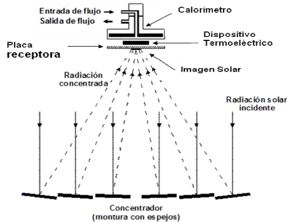
Figura 1.12. Sistema de generación de potencia eléctrica, integrado al sistema de concentración solar (DEFAC).
