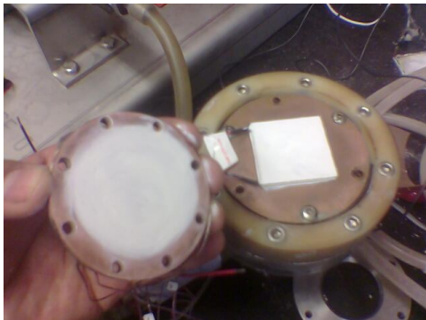
a) Se aplicó un silicón conductor térmico y se colocó la placa receptora.
