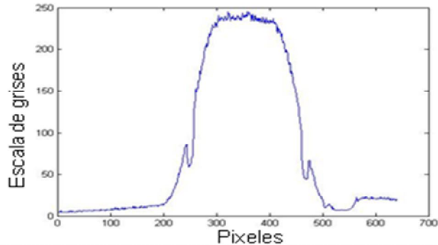
Figura 4.12. Imagen de la distribución de la radiación solar concentrada sobre la placa receptora en la parte central del spot procesada en MatLab en escala de grises y píxeles.
