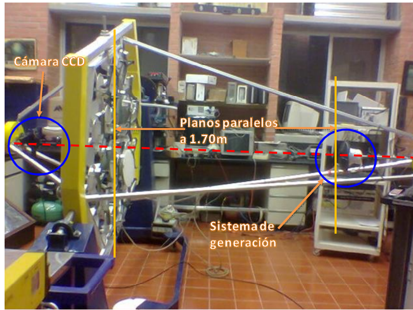
Figura 3.7. Esquema de la alineación del sistema de generación eléctrica, el conjunto de espejos concentradores y una cámara CCD.
