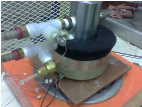
a) Integración del sistema de generación y la resistencia eléctrica.
