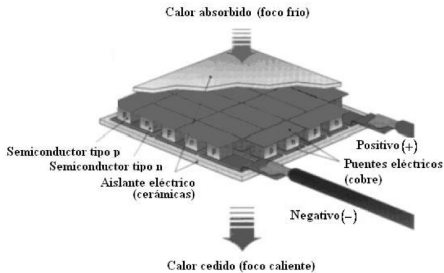
Figura 1.13. Esquema de una celda termoelectrica.
