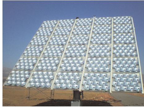
Figura 1.5. Fotografía de un sistema fotovoltaico con concentración.
