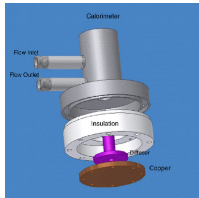
Figura 3.2. Esquema del ICPP.
