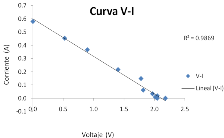
Figura 4.2. Gráfica de la curva voltaje-corriente (V-I), obtenida de la campaña experimental en el medio controlado.
