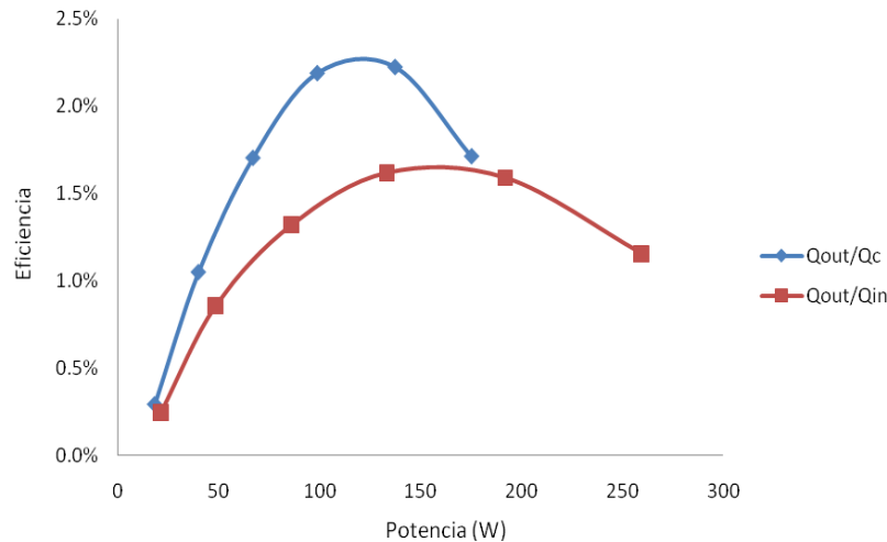
Figura 4.4. Grafica de las curvas de eficiencia, una del dispositivo termoelectrico ( Q_{out}/Q_c ) y la otra del sistema de generación ( Q_{out}/Q_{in} ).
