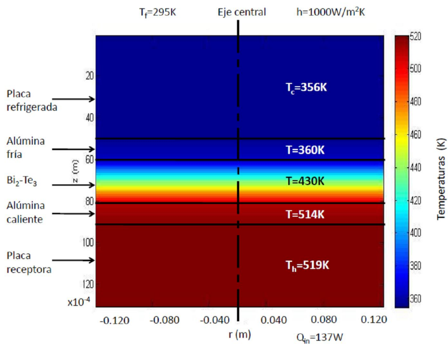
Figura 2.15. Imagen de la distribución de temperaturas en las placas de cobre y el dispositivo termoeléctrico, obtenidos del modelo en MatLab.
