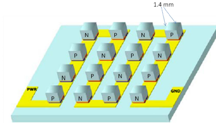
Figura 2.8. Se muestran los cubos de \text{Bi}_2\text{Te}_3 que forman el generador termoeléctrico.
