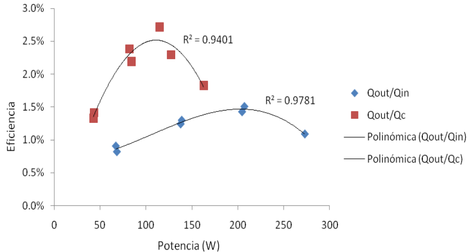
Figura 4.9. Gráfica de las curvas de eficiencia, una del dispositivo termoeléctrico ( Q_{out}/Q_c ) y la otra del sistema de generación ( Q_{out}/Q_{in} ) de los experimentos en el DEFRACT.
