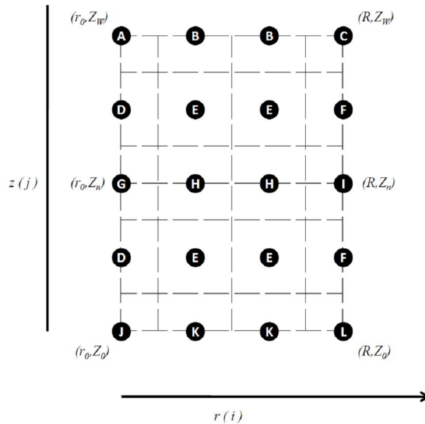
Figura 2.11. Esquema de los nodos del sistema.
