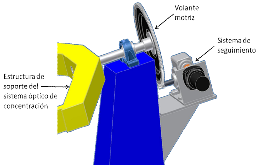
Figura A1.2. Esquema del sistema de seguimiento montado y acoplado en el DEFRAC.
