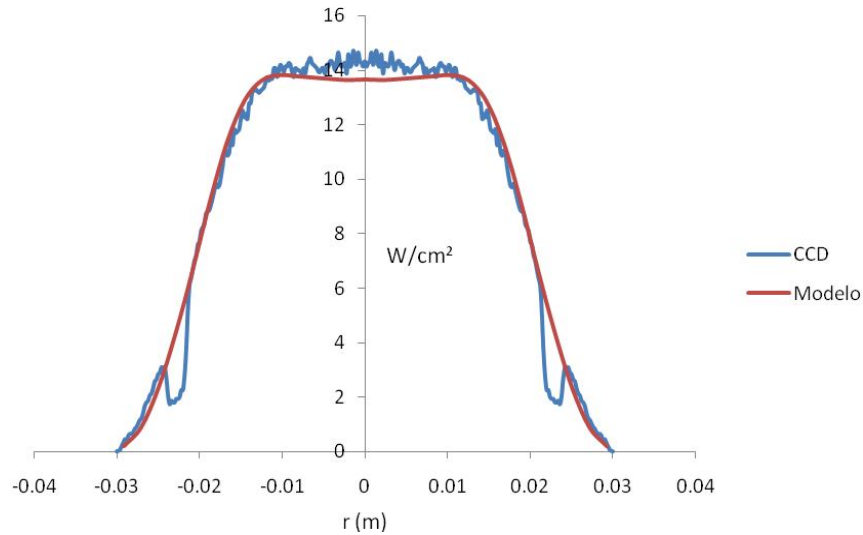
Figura 4.15. Comparativa de la distribución de radiación solar concentrada sobre la placa receptora entre la modelación en código CIRCE2 y la imagen de la cámara CCD
