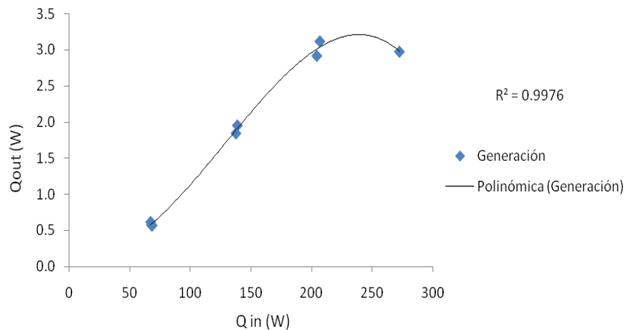
Figura 4.8. Gráfica de la curva de generación de potencia eléctrica Q_{out} en función de la potencia de entrada Q_{in} del DEFAC.
