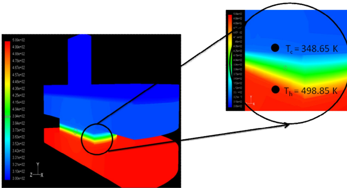
Figura 2.16. Imagen de la distribución de temperaturas simulado en FLUENT
