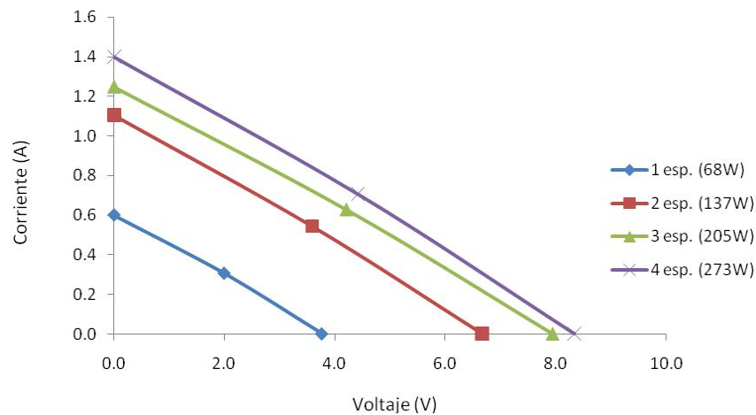
Figura 4.7. Gráfica de la curva voltaje-corriente obtenida en la campaña experimental para diferente número de espejos del DEFAC.
