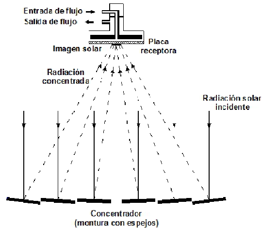
Figura 1.11. Esquema del calorímetro de placa plana en operación.
