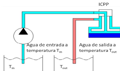
Figura 3.3. Esquema del sistema de refrigeración usado en los experimentos.
