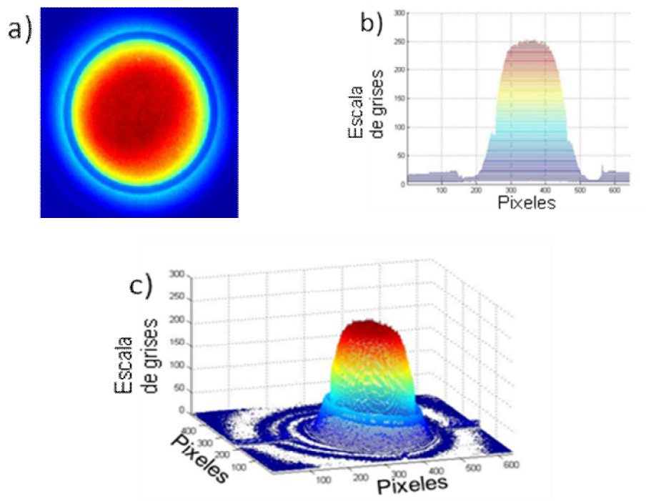
Figura 4.11. Imagen del spot de radiación solar concentrada sobre la placa receptora procesada en MatLab.
