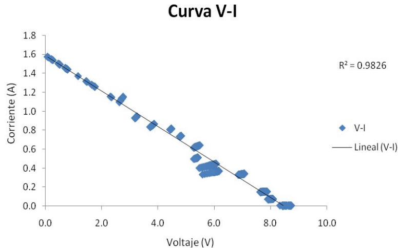
Figura 4.6. Gráfica de la curva voltaje-corriente obtenida en la campaña experimental con el DEFAC.
