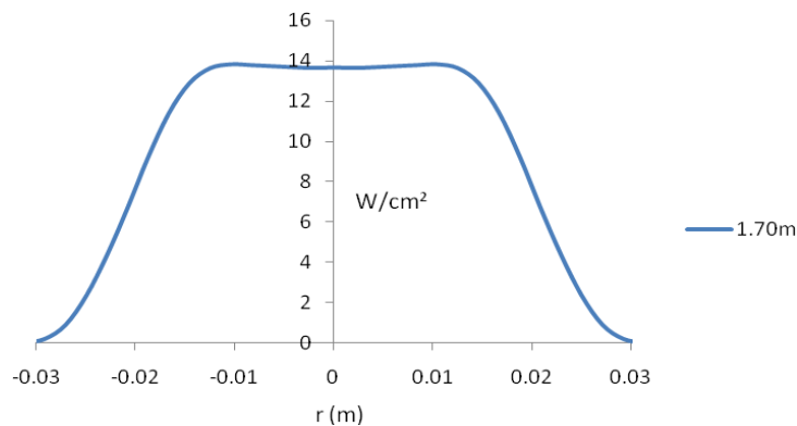
Figura 2.5. Distribución del flujo de radiación concentrada, ubicando el receptor fuera de foco (a 1.70 \text{ m} ) del sistema de concentración, usando solo 3 espejos y orientándolos a esa distancia focal.
