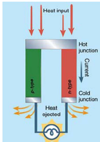
Figura 1.14. Esquema de un generador termoeléctrico y su funcionamiento.
