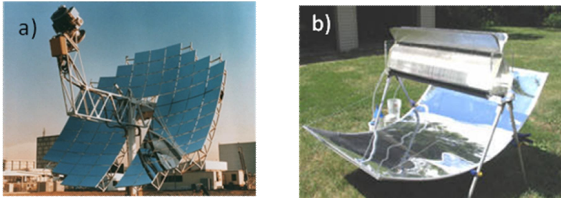
Figura 1.2. Sistemas de concentración solar a través de sistemas de reflexión. a) Plato parabólico, b) Canal parabólico.
