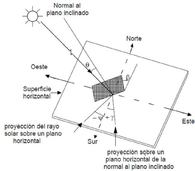
Figura 3.11. Esquema de la radiación solar con respecto a una superficie receptora.
