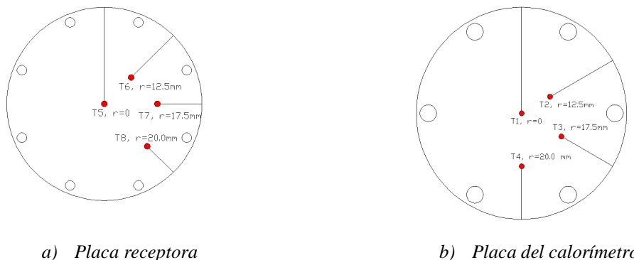
Figura 3.9. Ubicación de los termopares en las placas de cobre.
