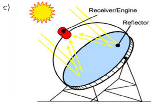
Figura 1.3. Sistemas de concentración solar. La figura a) corresponde a un concentrador solar tipo canal parabólico de enfoque lineal, la b) corresponde a un concentrador tipo torre central y la c) corresponde a un concentrador tipo plato parabólico de foco puntual.
