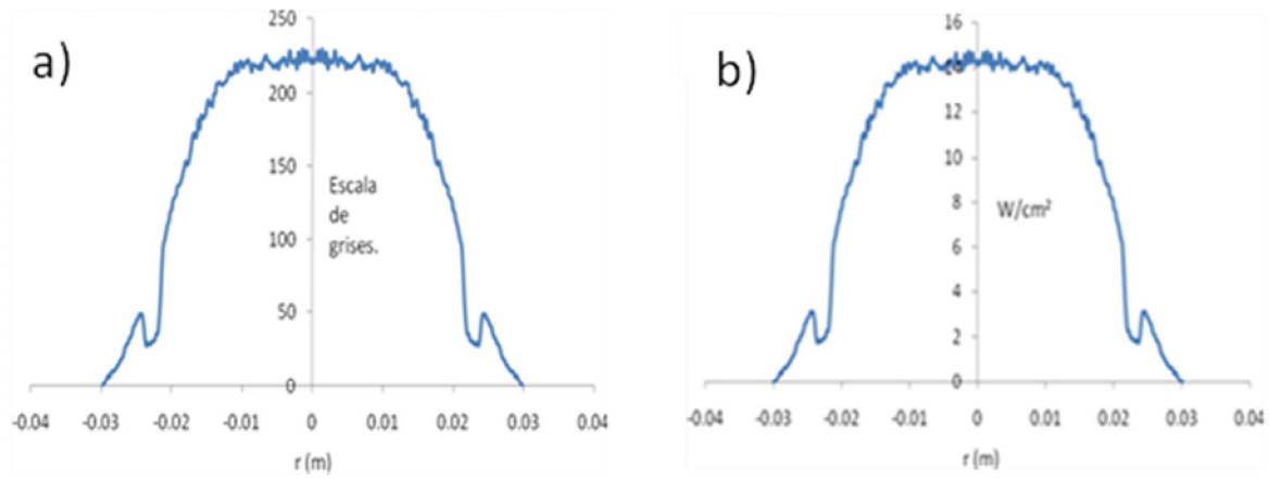
Figura 4.14. Se muestra la comparativa de la transformación de la distribución de niveles de grises a la de la intensidad de flujo radiativo. a) Distribución de la intensidad de niveles de grises de la imagen tomada con la cámara CCD. b) Distribución de la intensidad de flujo radiativo concentrado obtenida de la transformación de la imagen tomada con la cámara CCD.
