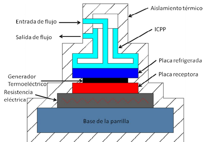
Figura 2.1. Diagrama esquemático de la fuente de calor controlada.
