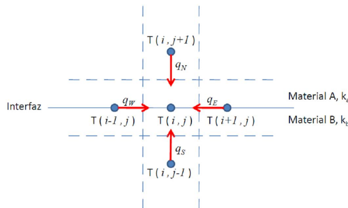
Figura 2.10. Esquema del volumen de control ubicado en las interfaces.
