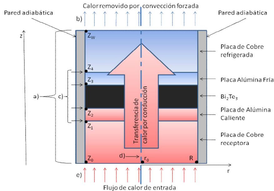
Figura 2.9. Esquema del sistema de generación, en el que se muestra la forma y ubicación de cada elemento, así como las condiciones de frontera.
