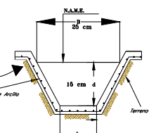
Canal perimetral de aguas pluviales
