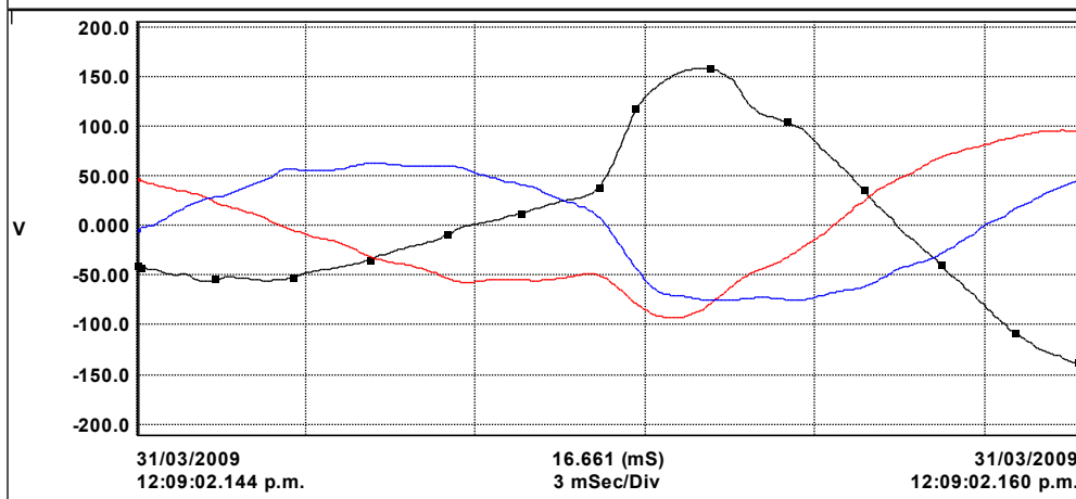
Figura 12. Tensión en los ciclos donde ocurre la falla
