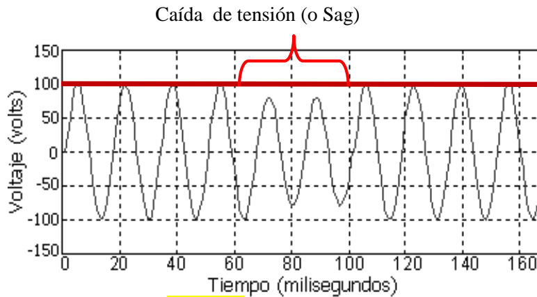
Figura 3. Señal de voltaje con sag
