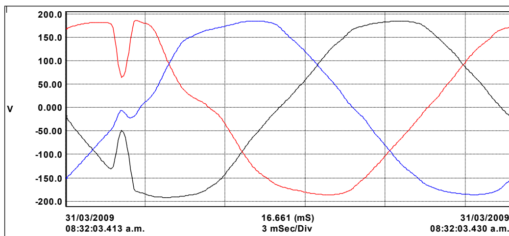
Figura 8. Tensión en el ciclo donde ocurre la falla
