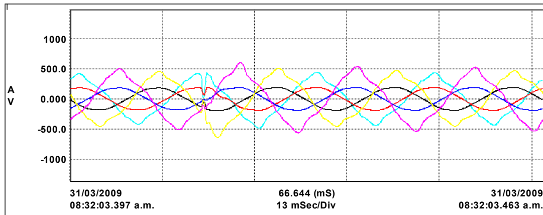
Fig. 20. Tensión y corriente durante cuatro ciclos
