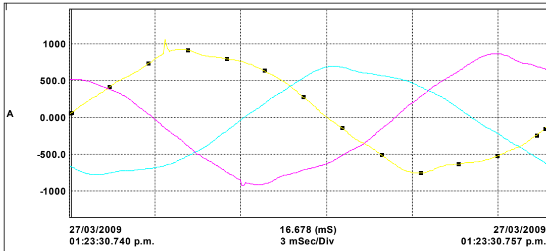
Figura 23. Corriente en los ciclos donde ocurre la falla
