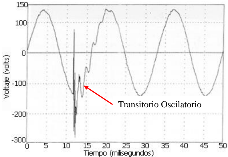
Fig.6. Transitorio oscilatorio en una señal de tensión.
