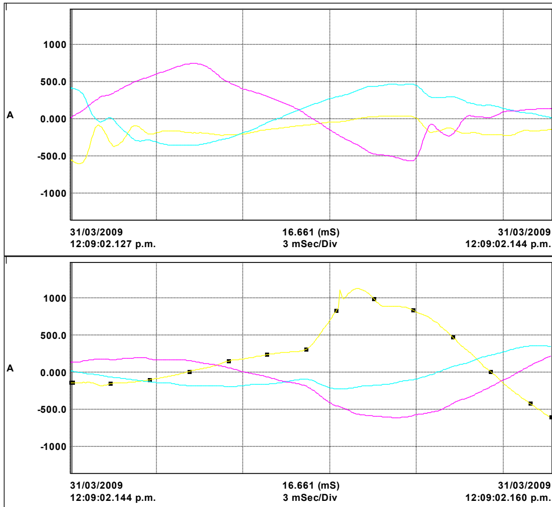
Figura 16. Corriente en los ciclos donde ocurre la falla
