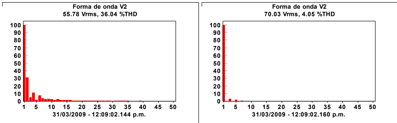
Figura 14. Contenido armónico en la tensión durante la falla en la fase B
