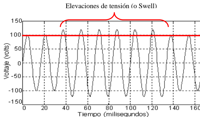
Fig. 4. Señal de voltaje con swell
