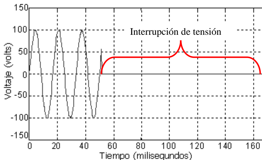
Fig. 2. Señal de voltaje con interrupción de energía
