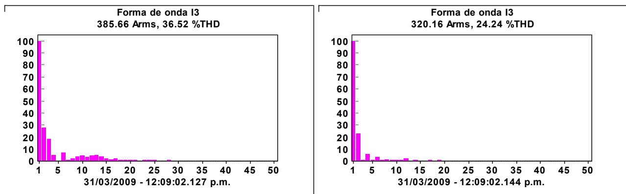
Figura 19. Contenido armónico en la corriente durante la falla en la fase C
