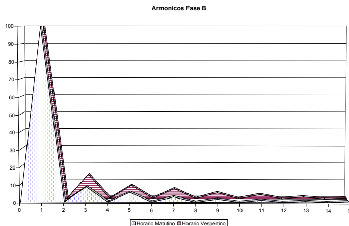
Figura 25. Porcentaje de armónicos en la fase B
