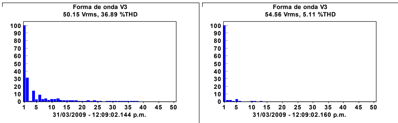
Figura 15. Contenido armónico en la tensión durante la falla en la fase C
