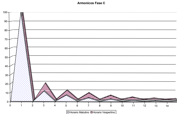
Figura 26. Porcentaje de armónicos en la fase C
