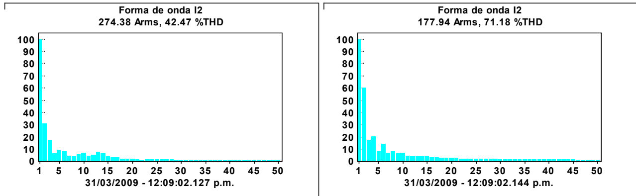
Figura 18. Contenido armónico en la corriente durante la falla en la fase B
