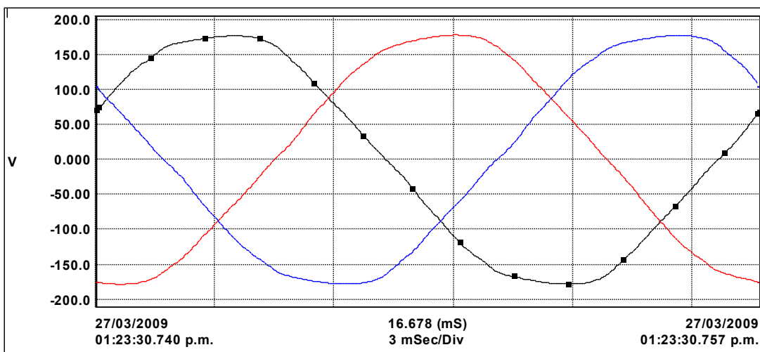
Figura 22. Tensión en los ciclos donde ocurre la falla
