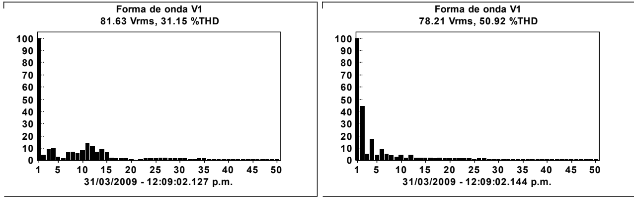
Figura 13. Contenido armónico en la tensión durante la falla en la fase A
