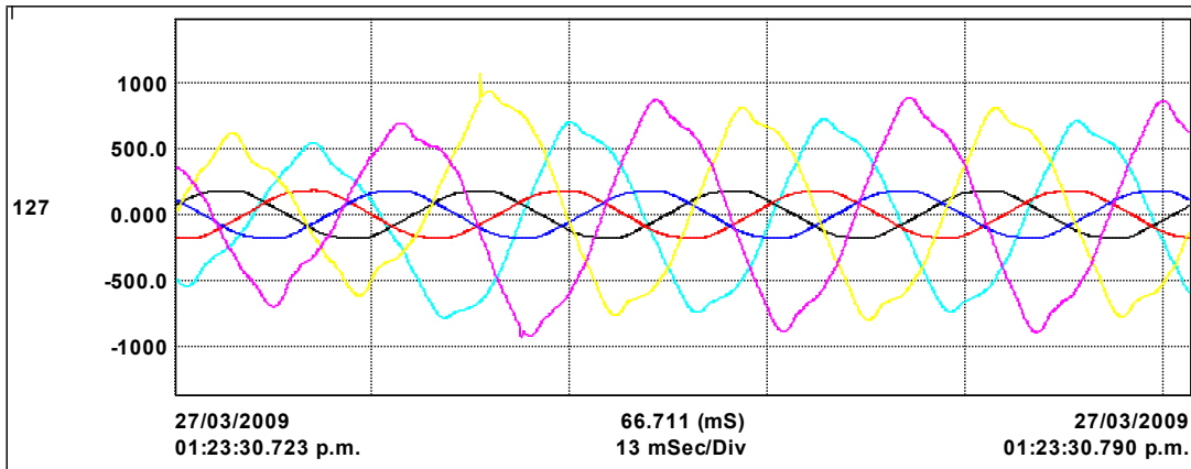
Figura 20. Tensión y corriente durante cuatro ciclos.
