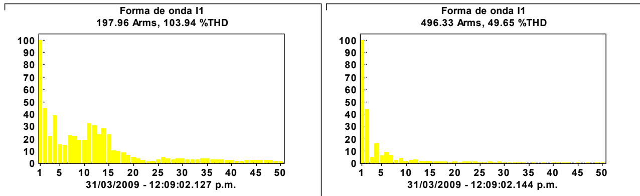
Figura 17. Contenido armónico en la corriente durante la falla en la fase A
