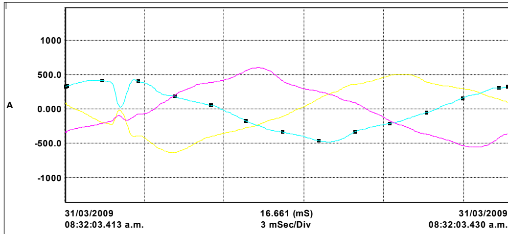
Figura 9. Corriente en el ciclo donde ocurre la falla
