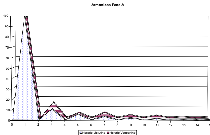
Figura 24. Porcentaje de armónicos en la fase A4
