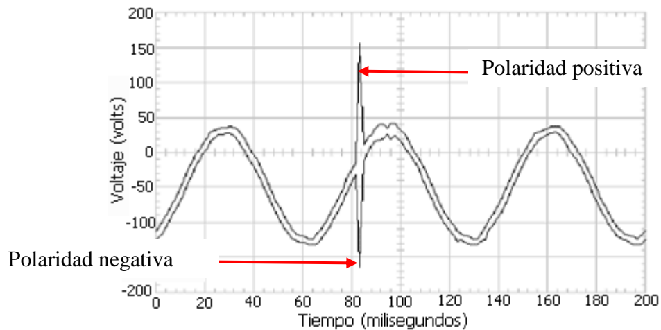
Fig. 5. Impulso transitorio en dos señales de tensión. Las dos señales de tensión tienen respectivamente polaridad positiva y negativa.
