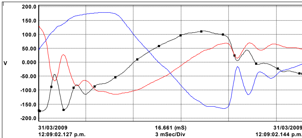
Figura 11. Tensión y corriente durante cuatro ciclos
