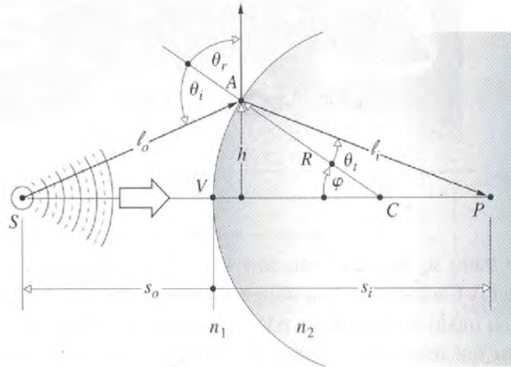
Figura 1.3: Interface entre dos medios con índice de refracción diferente
