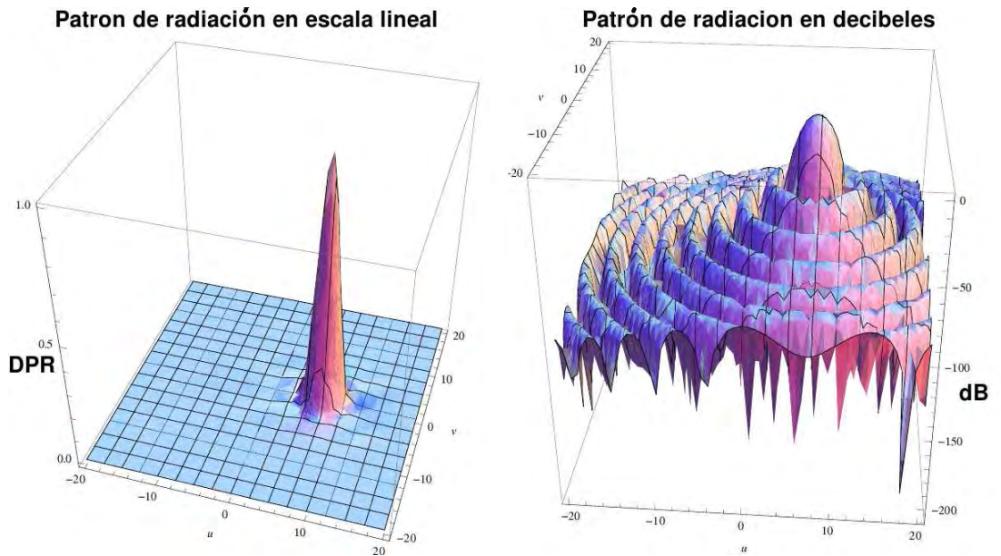
Figura 3.34: Patrón de radiación del reflector parabólico equivalente cuando el detector se desplaza 7.5 longitudes de onda
