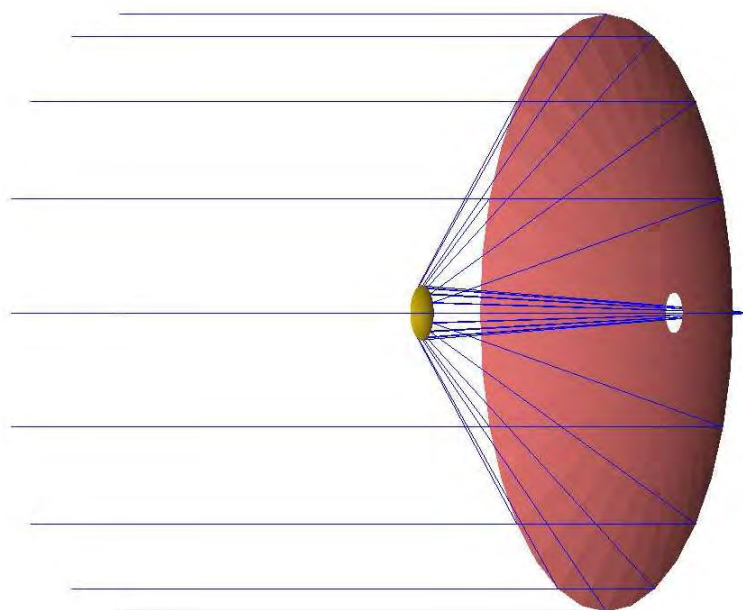
Figura 1.7: Resultado obtenido en Zemax
