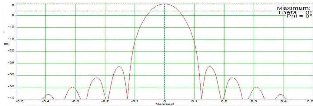
Figura 3.1: Diagrama de radiación de un reflector parabólico de 5 metros calculado por el programa SABOR
