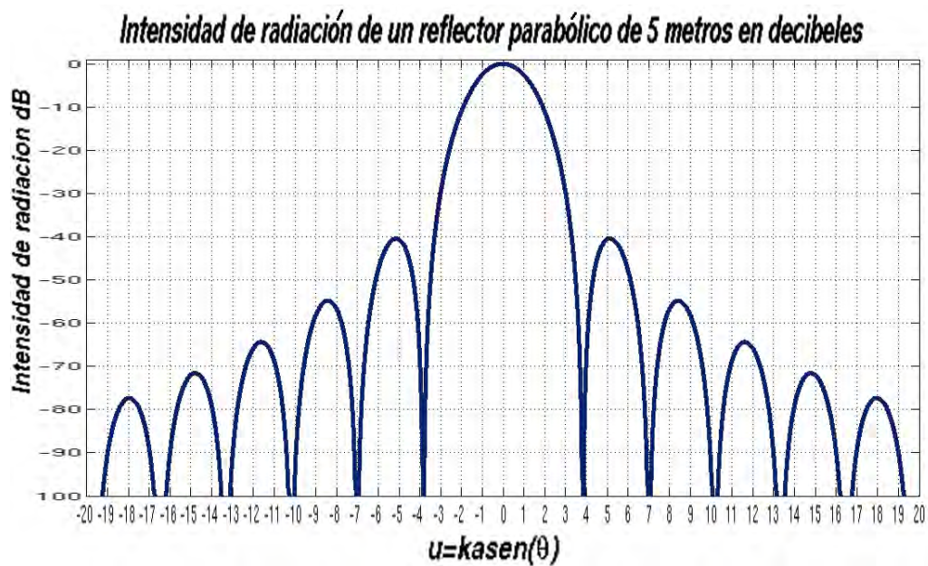
Figura 2.12: Patrón de radiación en decibeles
