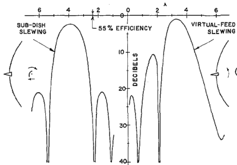
Figura 3.13: Efectos sobre el patrón de radiación al rotar el espejo secundario respecto al foco del espejo primario [13]
