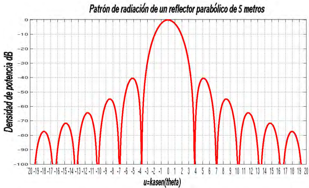
Figura 2.15: Diagrama de radiación en decibeles
