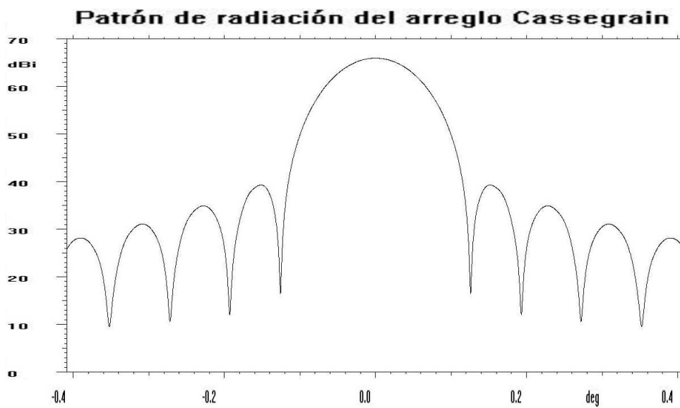
Figura 3.8: Patrón de radiación de un arreglo Cassegrain interpolado linealmente calculado por el programa GRASP9
