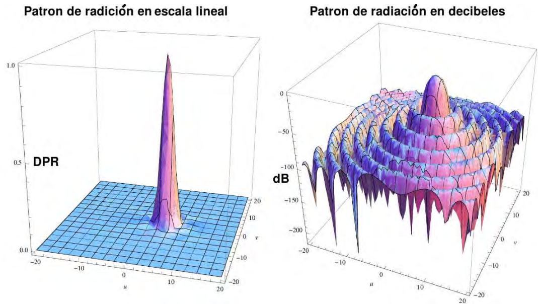
Figura 3.26: Patrón de radiación del reflector parabólico equivalente cuando el detector se desplaza 4 longitudes de onda
