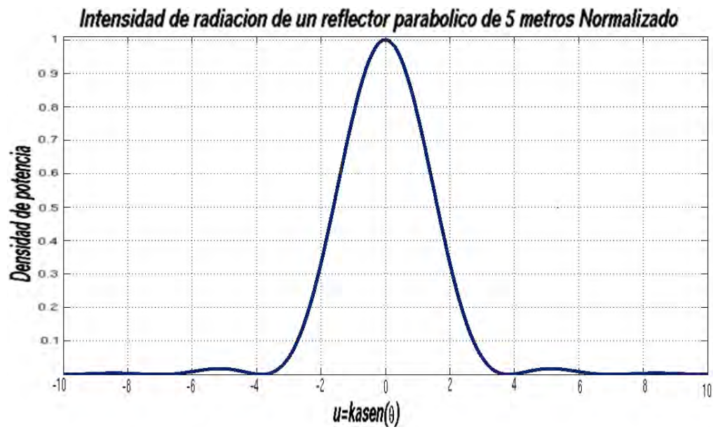
Figura 2.11: Intensidad de radiación normalizada
