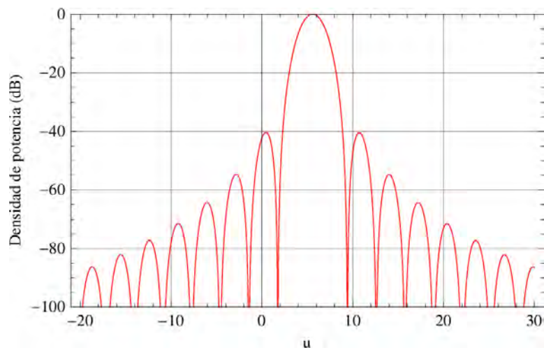
Figura 3.31: Corte del patrón de radiación del reflector parabólico equivalente cuando el detector se desplaza 6 longitudes de onda
