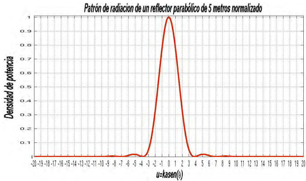
Figura 2.14: Diagrama de radiación normalizado
