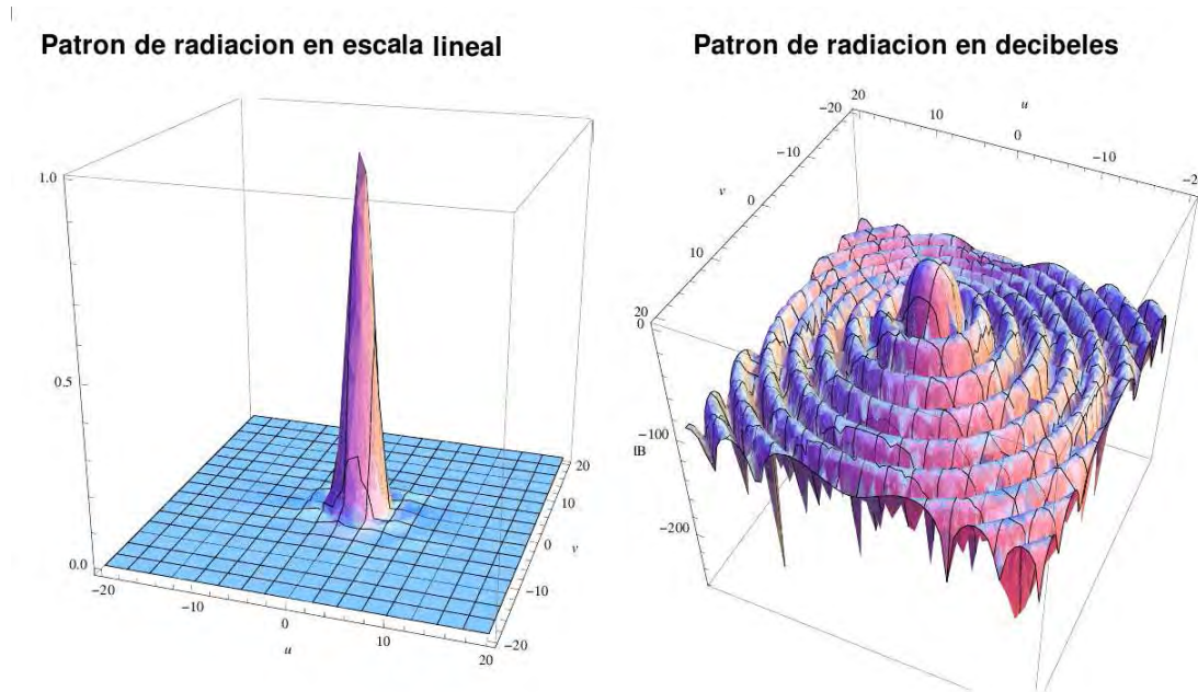
Figura 3.20: Patron de radiación del arreglo Cassegrain cuando el haz principal se desplaza una longitud de onda
