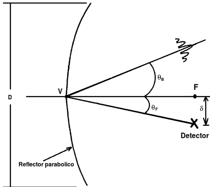
Figura 3.15: Desplazamiento lateral del detector
