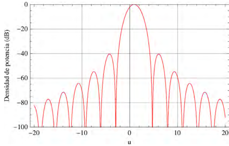
Figura 3.21: Corte del patrón de radiación cuando el detector del arreglo equivalente se desplaza una longitud de onda
