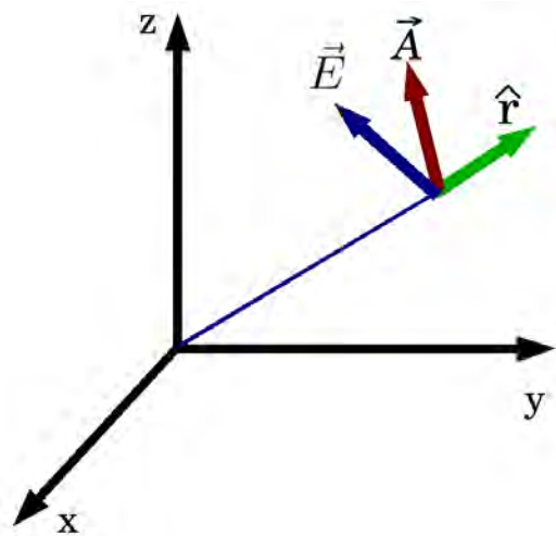
Figura 2.6: Representación geométrica de \hat{r} \times (\hat{r} \times \vec{A})
