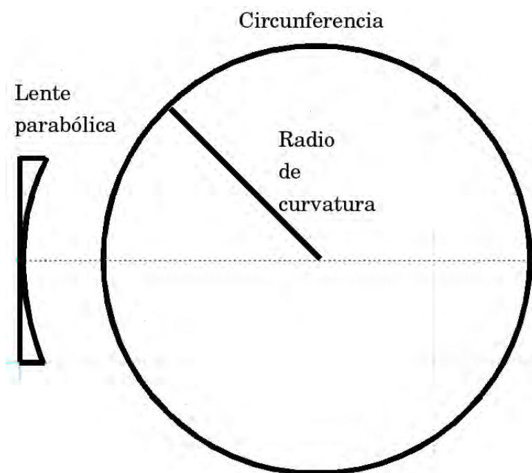
Figura 1.2: Aproximación del radio de curvatura de una lente esférica con el radio de curvatura de una circunferencia
