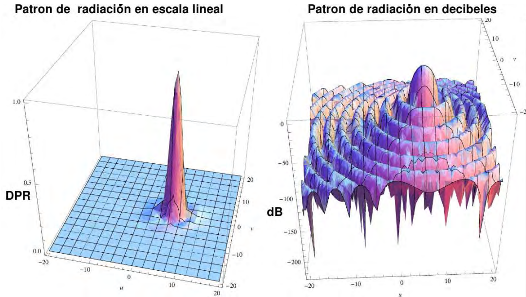
Figura 3.30: Patrón de radiación del reflector parabólico equivalente cuando el detector se desplaza 6 longitudes de onda
