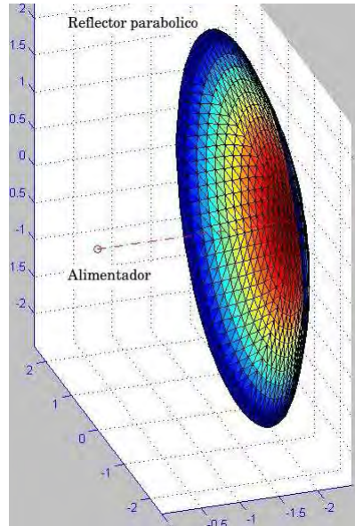
Figura 3.9: Geometría de un reflector parabólico de 5 metros generado por ICARA
