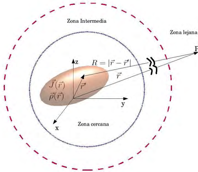
Figura 2.3: Zonas de radiación de una antena
