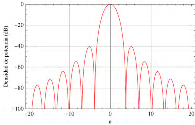
Figura 3.19: Corte del patrón de radiación cuando el espejo secundario no sufre ninguna rotación
