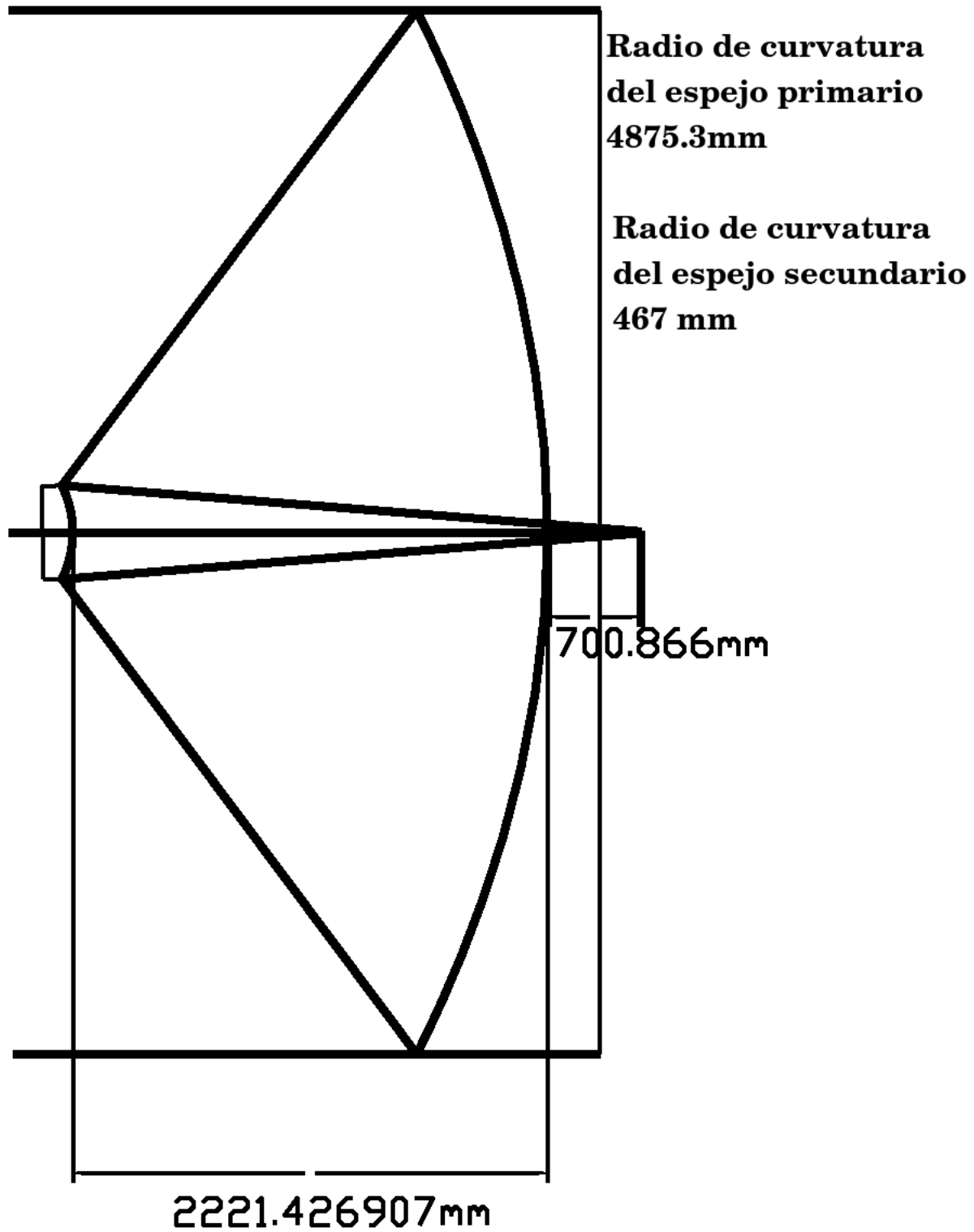
Figura 1.6: Distancia focal posterior del sistema
