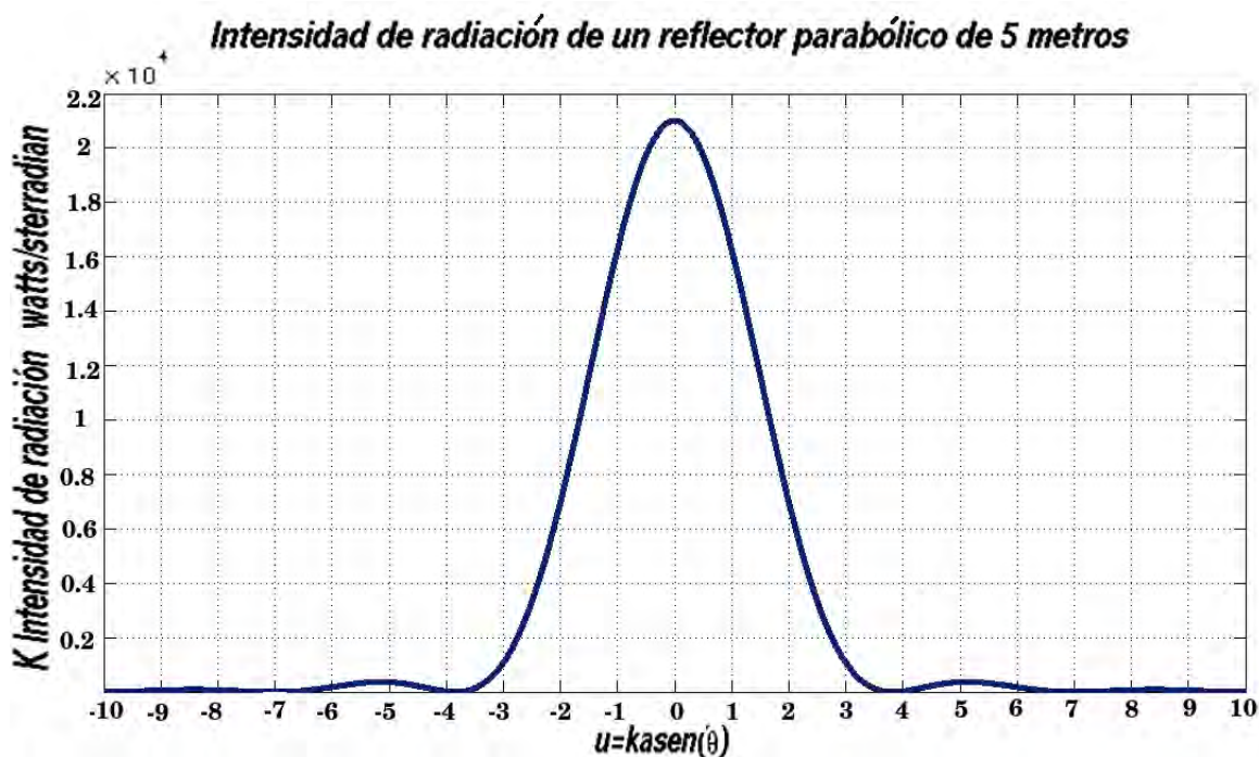
Figura 2.10: Intensidad de radiación en escala lineal
