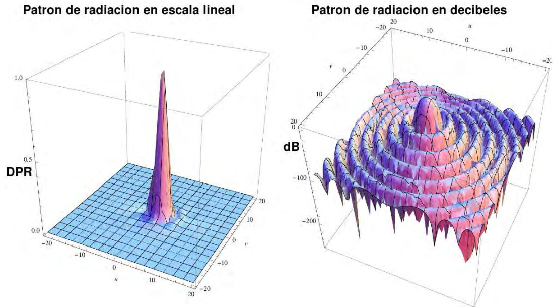
Figura 3.22: Patrón de radiación del reflector parabólico equivalente cuando el detector se desplaza 2 longitudes de onda
