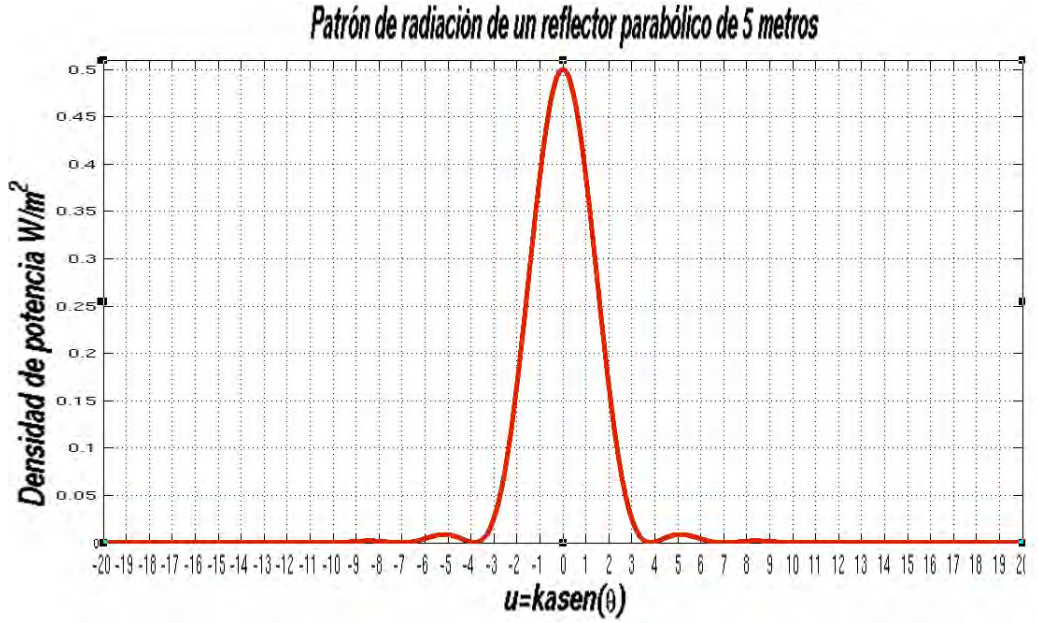
Figura 2.13: Diagrama de radiación en escala lineal
