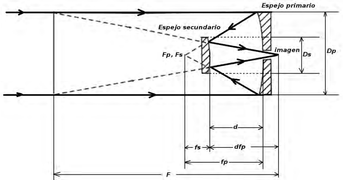
Figura 1.1: Telescopio Cassegrain
