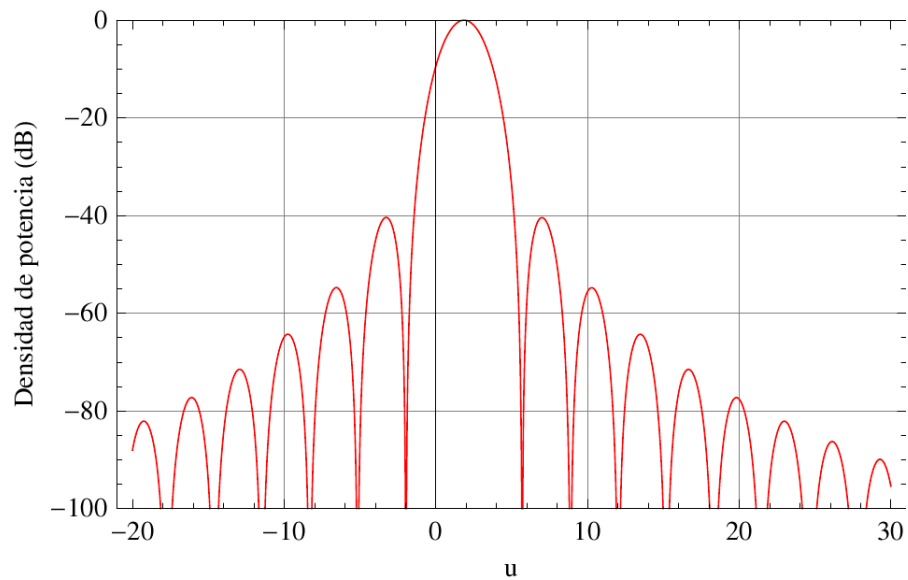
Figura 3.23: Corte del patrón de radiación del reflector parabólico equivalente cuando el detector se desplaza 2 longitudes de onda
