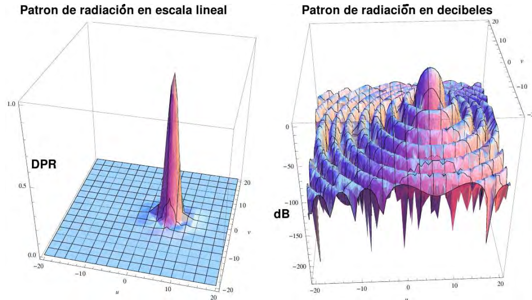
Figura 3.28: Patrón de radiación del reflector parabólico equivalente cuando el detector se desplaza 5 longitudes de onda
