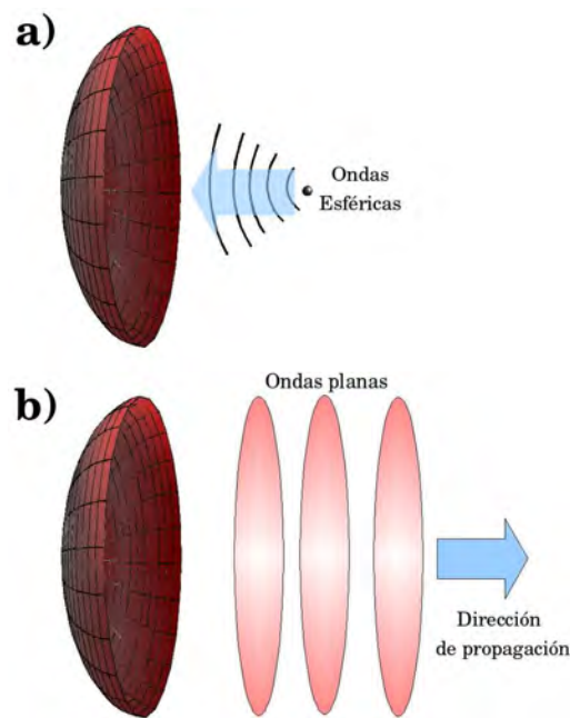
Figura 2.8: a) Ondas esféricas emergiendo del foco b) Ondas planas reflejadas
