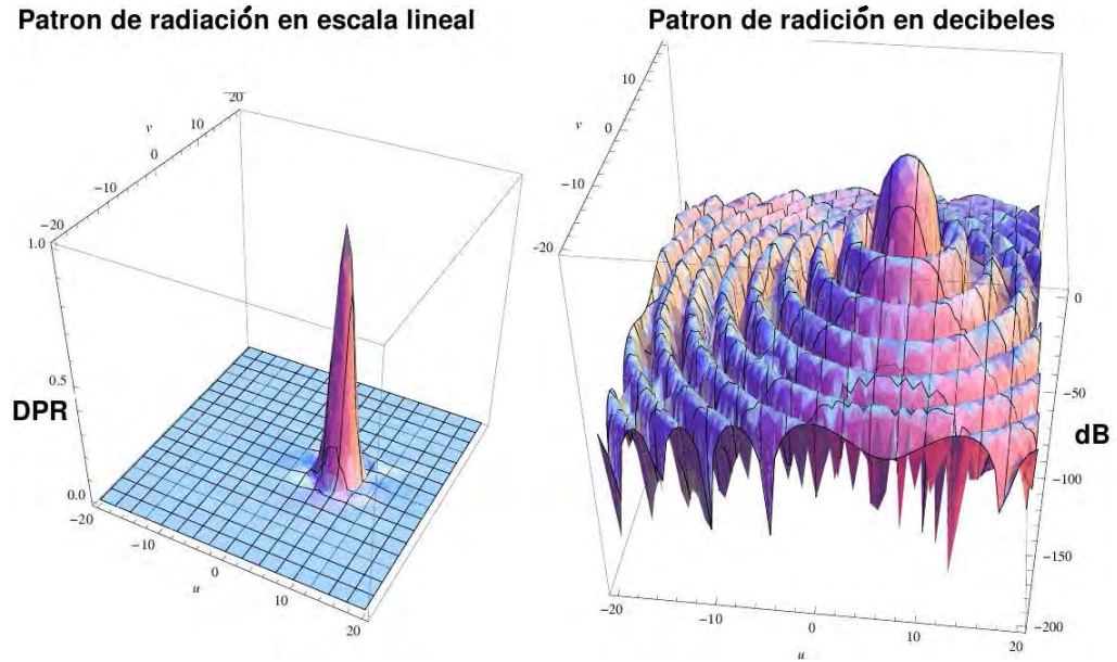
Figura 3.32: Patrón de radiación del reflector parabólico equivalente cuando el detector se desplaza 7 longitudes de onda
