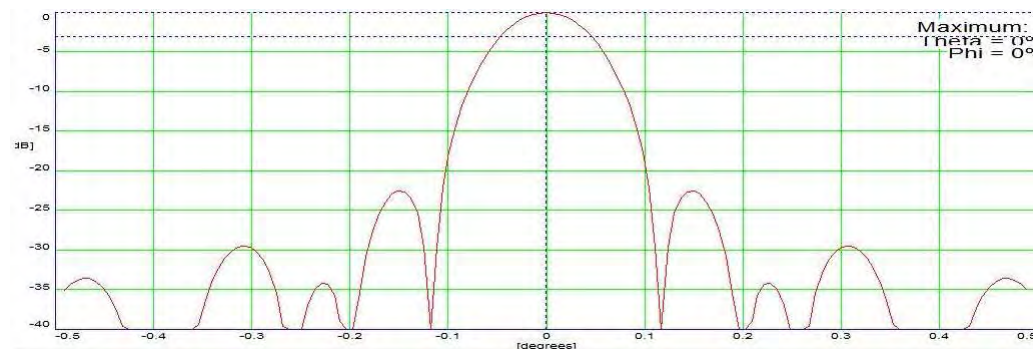
Figura 3.2: Diagrama de radiación de un arreglo Cassegrain de 5 metros calculado con el programa SABOR
