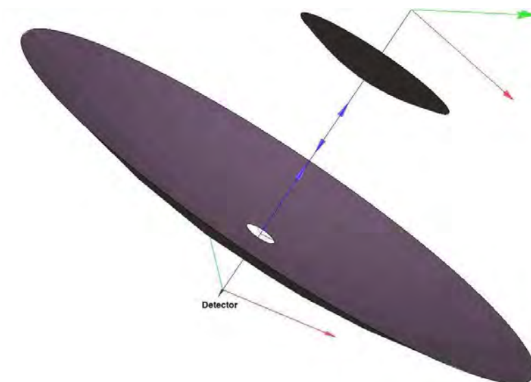
Figura 3.6: Geometría de un arreglo Cassegrain generado por el programa GRASP9
