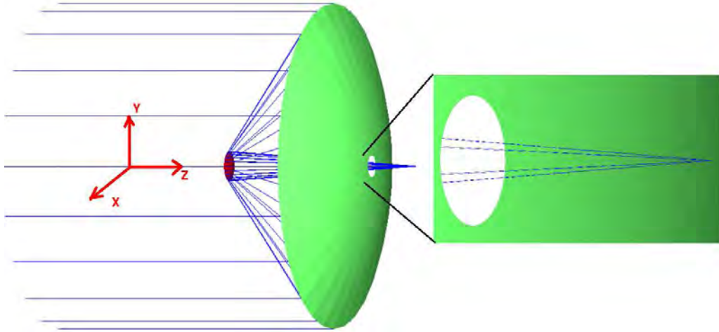
Figura 1.11: Espejo secundario sin rotar
