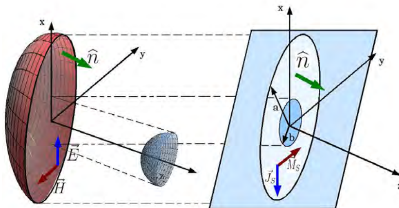
Figura 2.16: Bloqueo que produce el reflector secundario
