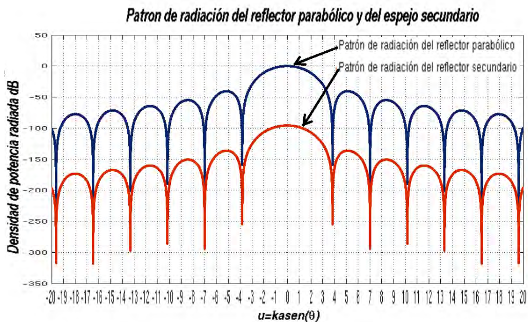
Figura 2.17: Densidad de potencia de un reflector parabólico y del bloqueo del secundario
