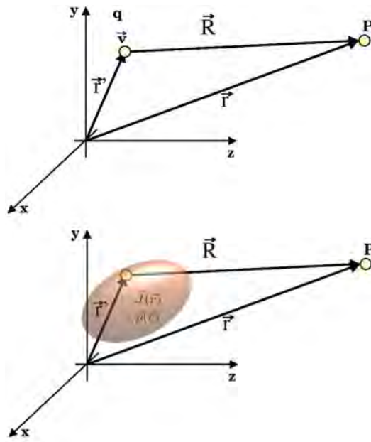
Figura 2.2: a) Carga puntual moviéndose. b) Densidad de carga
