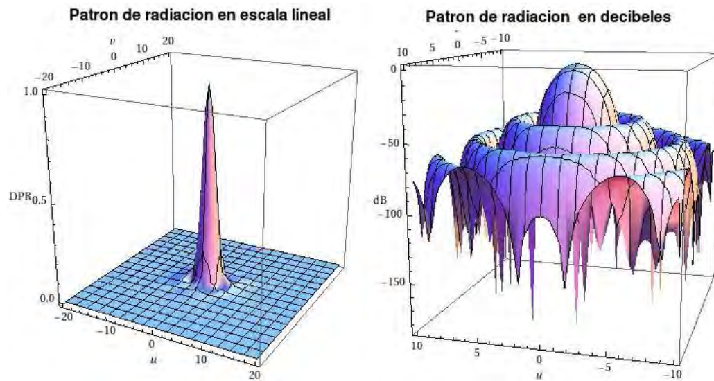
Figura 3.18: Patrón de radiación del arreglo Cassegrain cuando el espejo secundario no sufre ninguna rotación
