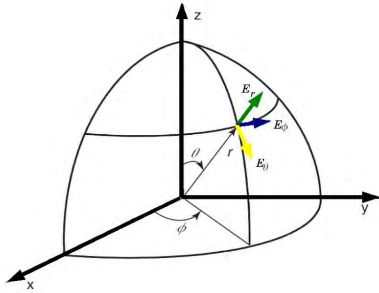
Figura 2.7: Sistema de coordenadas esféricas
