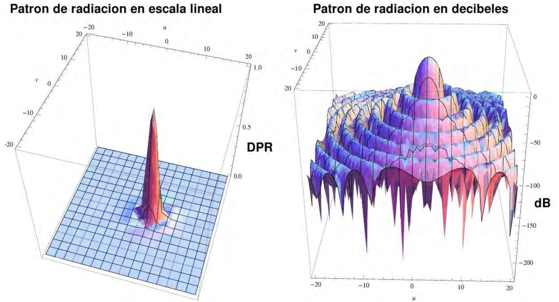
Figura 3.24: Patrón de radiación del reflector parabólico equivalente cuando el detector se desplaza 3 longitudes de onda
