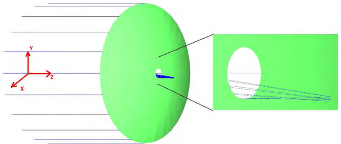
Figura 1.12: Espejo secundario rotado -1.95 grados
