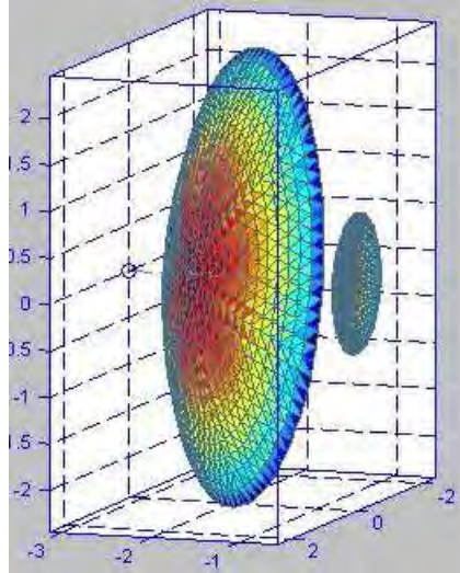
Figura 3.11: Geometría de un arreglo Cassegrain generado por el programa ICARA
