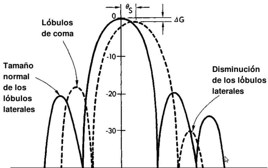
Figura 3.16: Patrón de radiación desplazado
