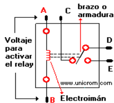
Figura 1.4 Relés electromecánicos.
