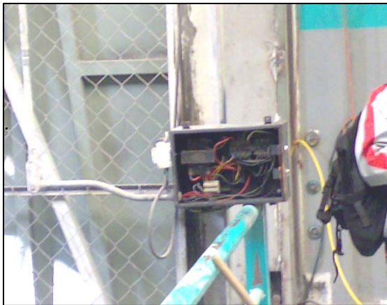
Figura 2.7A. Tablero abierto.
