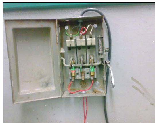
Figura 2.8B. Centro de carga abierto.
