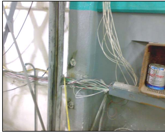
Figura 2.6. Cables expuestos y cerca de materiales inflamables.
