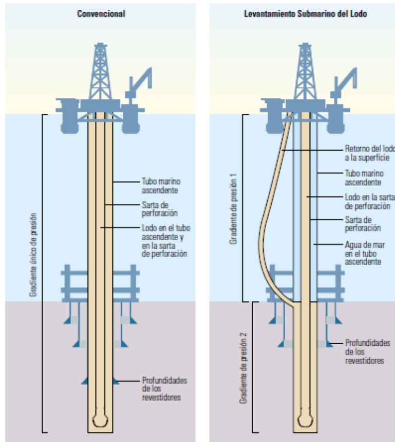
Figura 4.2. Esquema y comparación entre el sistema de perforación convencional y el sistema de perforación Doble Gradiente 4
