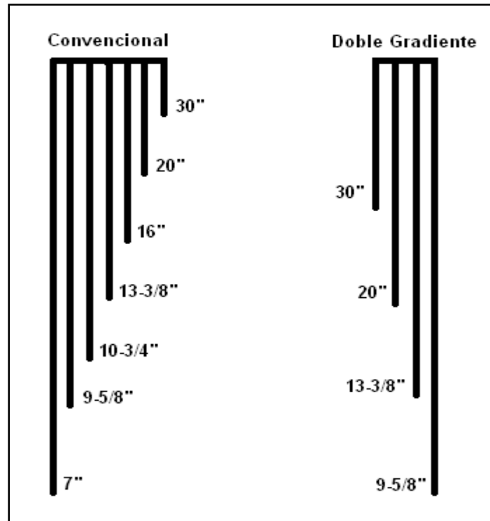
Figura 5.6. Comparación del número de tuberías de revestimiento requeridas según el tipo de perforación empleado
