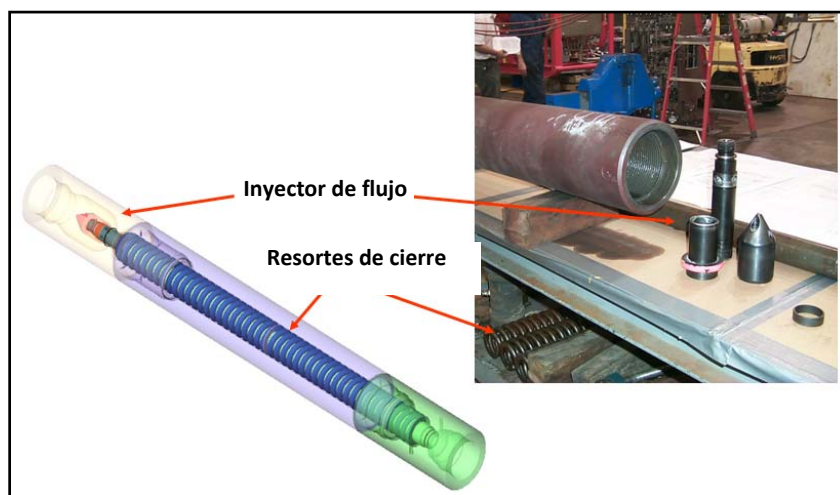
Figura 4.7. Válvula de secuencia de perforación o válvula de lodo 7
