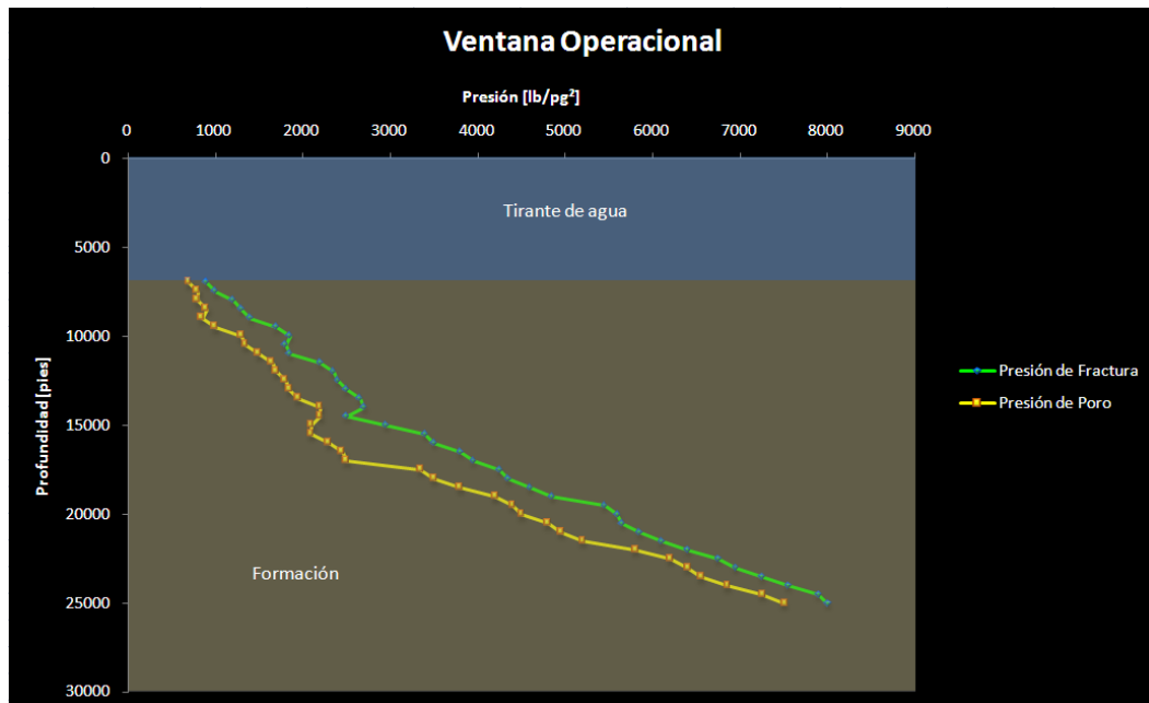
Figura 5.1. Ventana operacional de un pozo en aguas profundas. Se observan la presión de poro y la presión de fractura esperados
