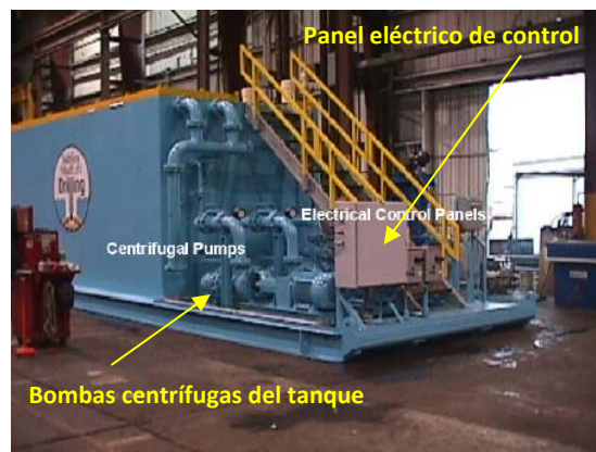
Figura 4.9. Tanque de filtrado 7
