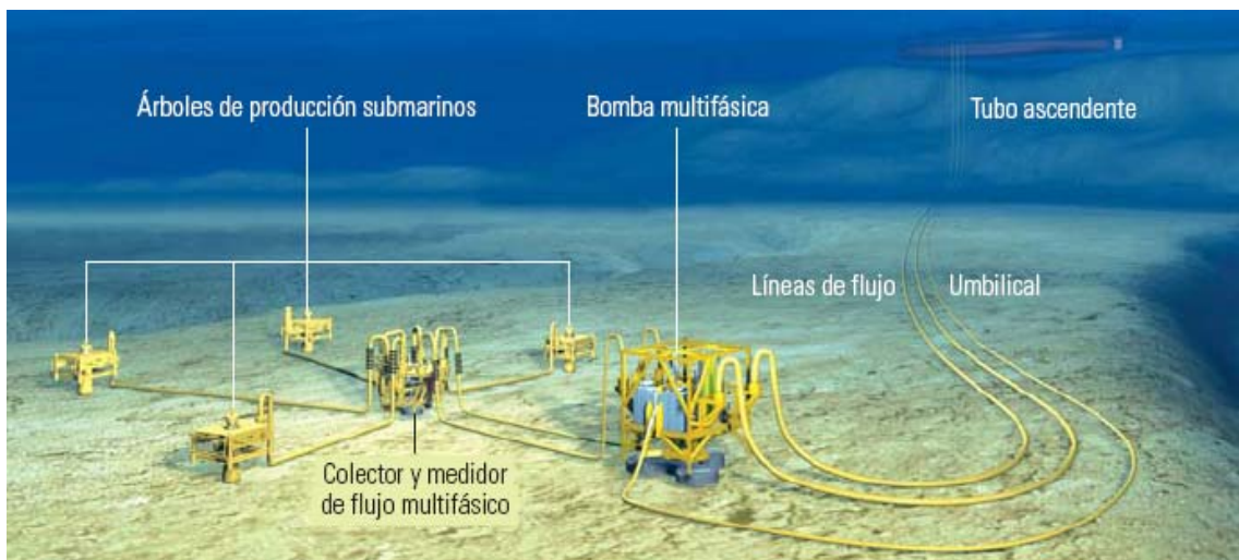
Figura 3.1. Sistema submarino a tierra (subsea-to-shore) que incluye bomba multifásica, colector, árboles de producción submarinos y líneas de flujo 2
