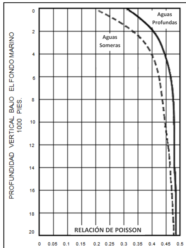
Gráfica 5.1. Relación de Poisson para aguas someras y aguas profundas
