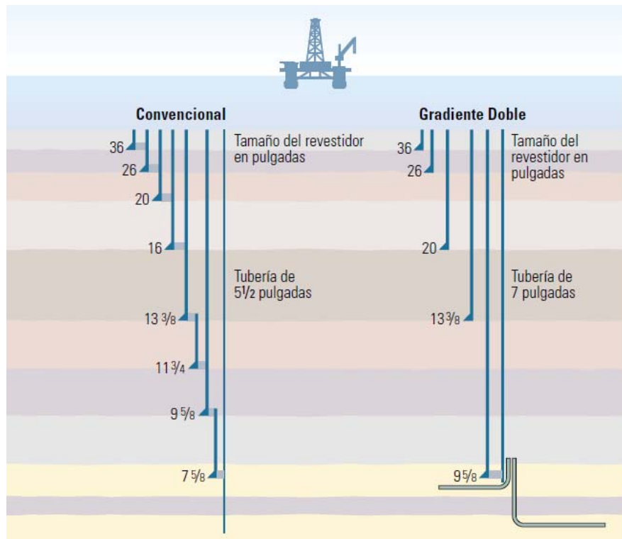
Figura 4.1. Beneficio del uso del sistema de perforación Doble Gradiente reflejado en un menor requerimiento de tuberías de revestimiento comparado con la cantidad necesaria que requiere el sistema de perforación convencional 4
