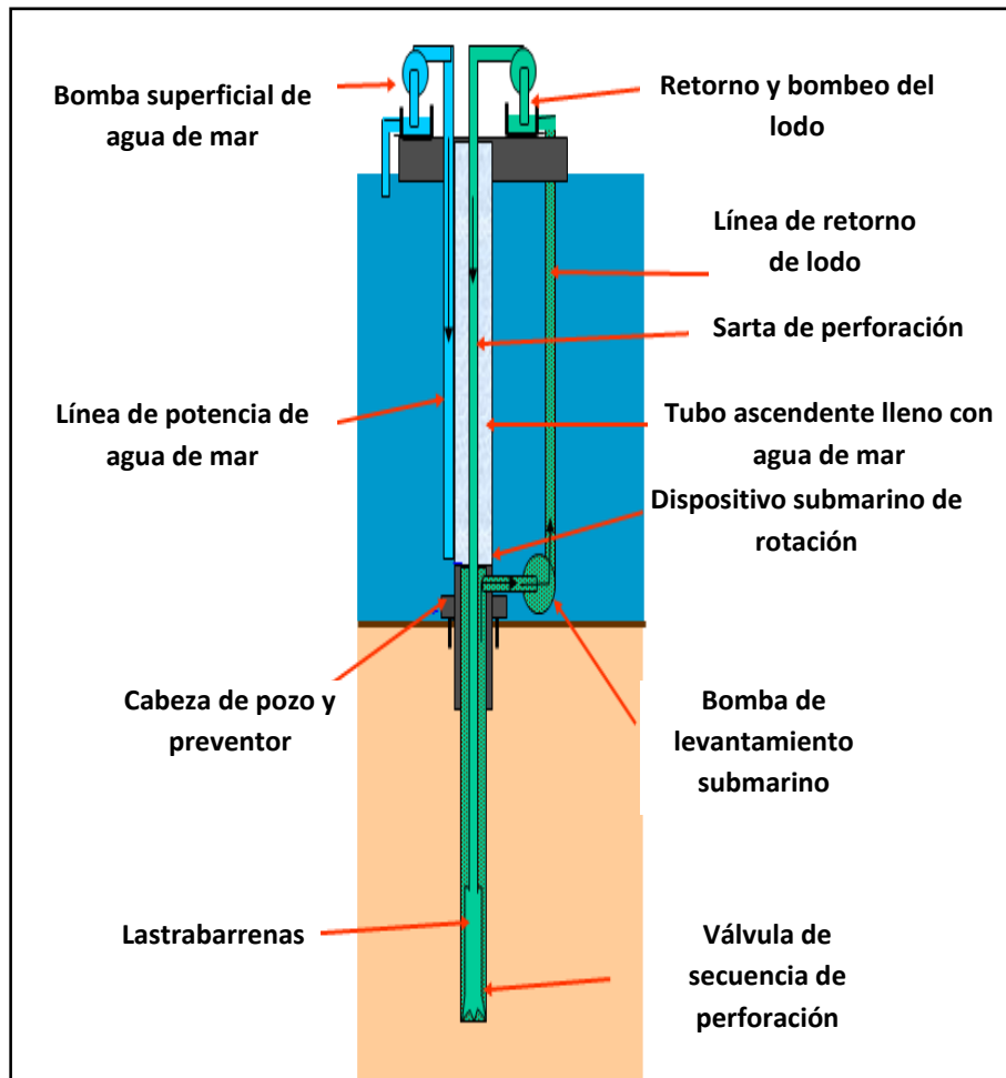
Figura 4.4. Configuración final del sistema de perforación Doble Gradiente en el que se incluye una línea de potencia de agua de mar 12
