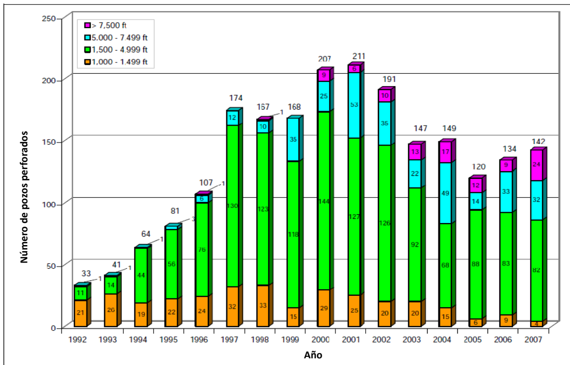
Figura 3.6. Todos los pozos perforados en aguas profundas en la región norteamericana del Golfo de México ordenados por tirante de agua 20
