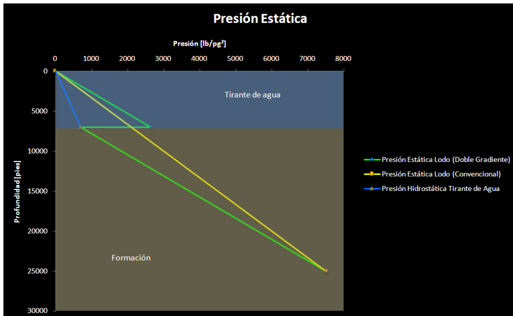
Figura 5.7. Presión estática dentro del agujero y espacio anular para ambos sistemas de perforación, convencional y Doble Gradiente
