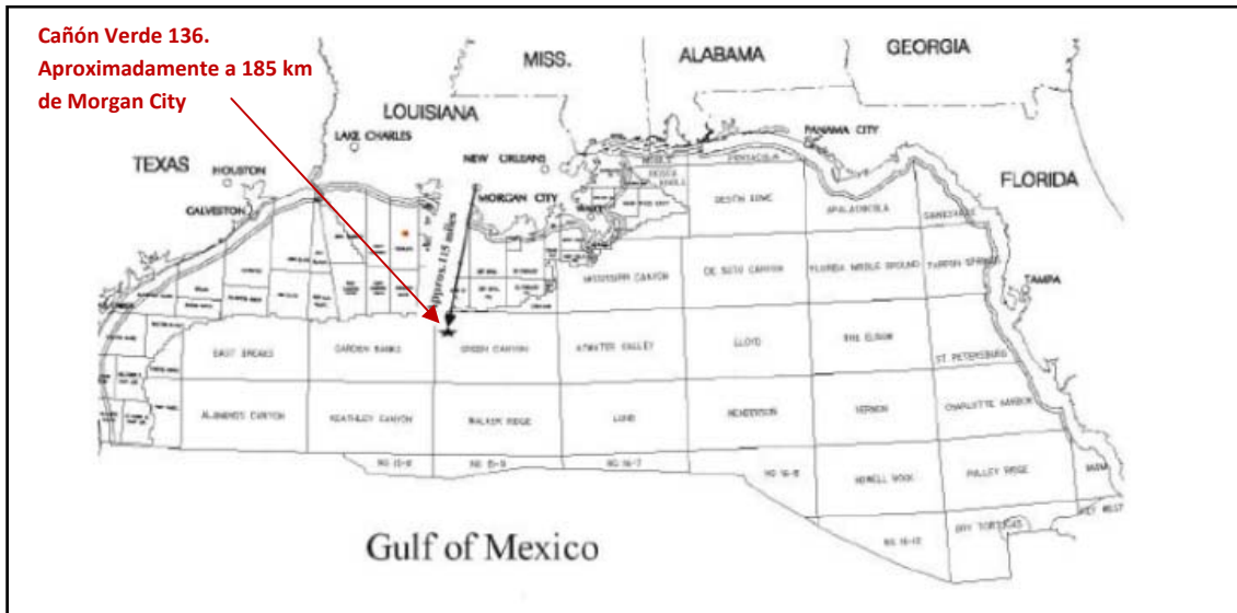
Figura 5.11. Ubicación del pozo piloto para la prueba del sistema de perforación Doble Gradiente 8
