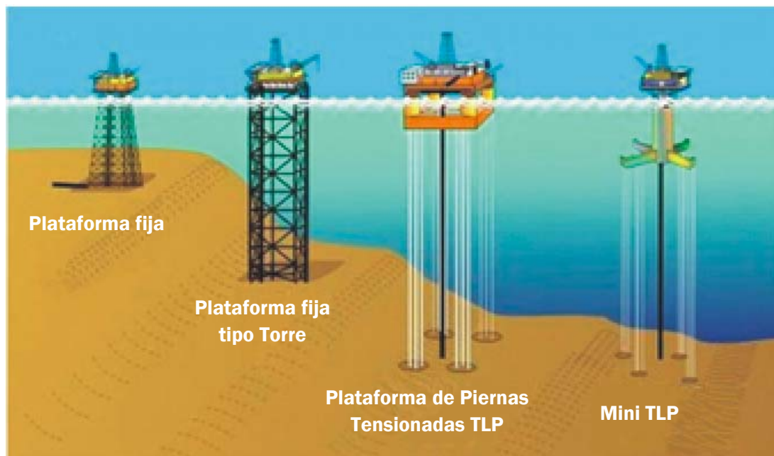
Figura 2.8. Estructuras ancladas al lecho marino. De izquierda a derecha observamos la Plataforma Fija, la Plataforma Fija tipo Torre, la Plataforma de Piernas Tensionadas y una Plataforma de piernas tensionadas de menor envergadura 20
