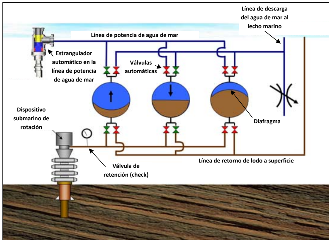
Figura 4.5. Esquema del funcionamiento de la bomba de levantamiento submarino de lodo MLP 12
