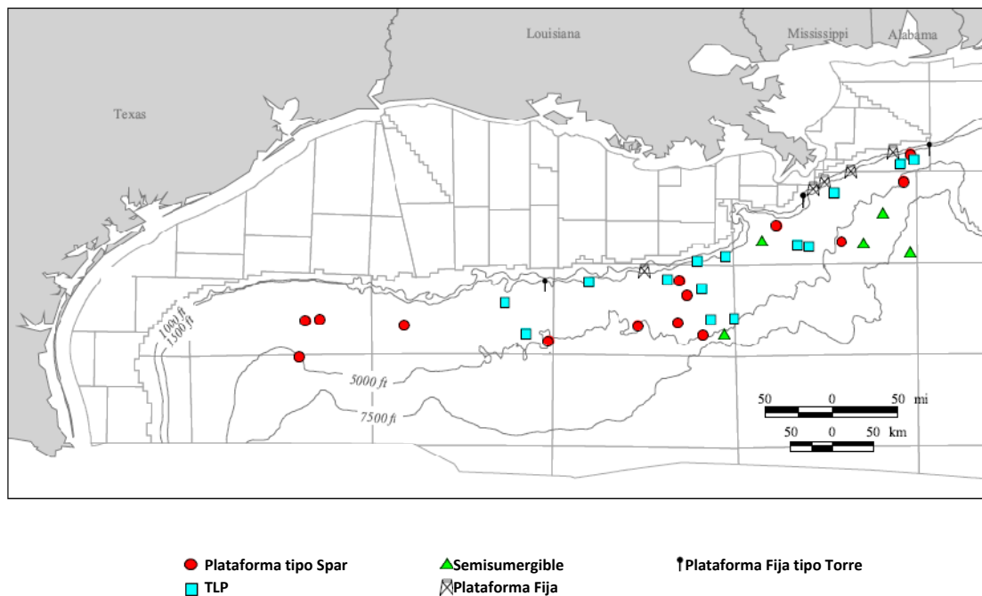
Figura 2.6. Mapa de las estructuras operando en aguas profundas de la región norteamericana del Golfo de México según su tipo 20
