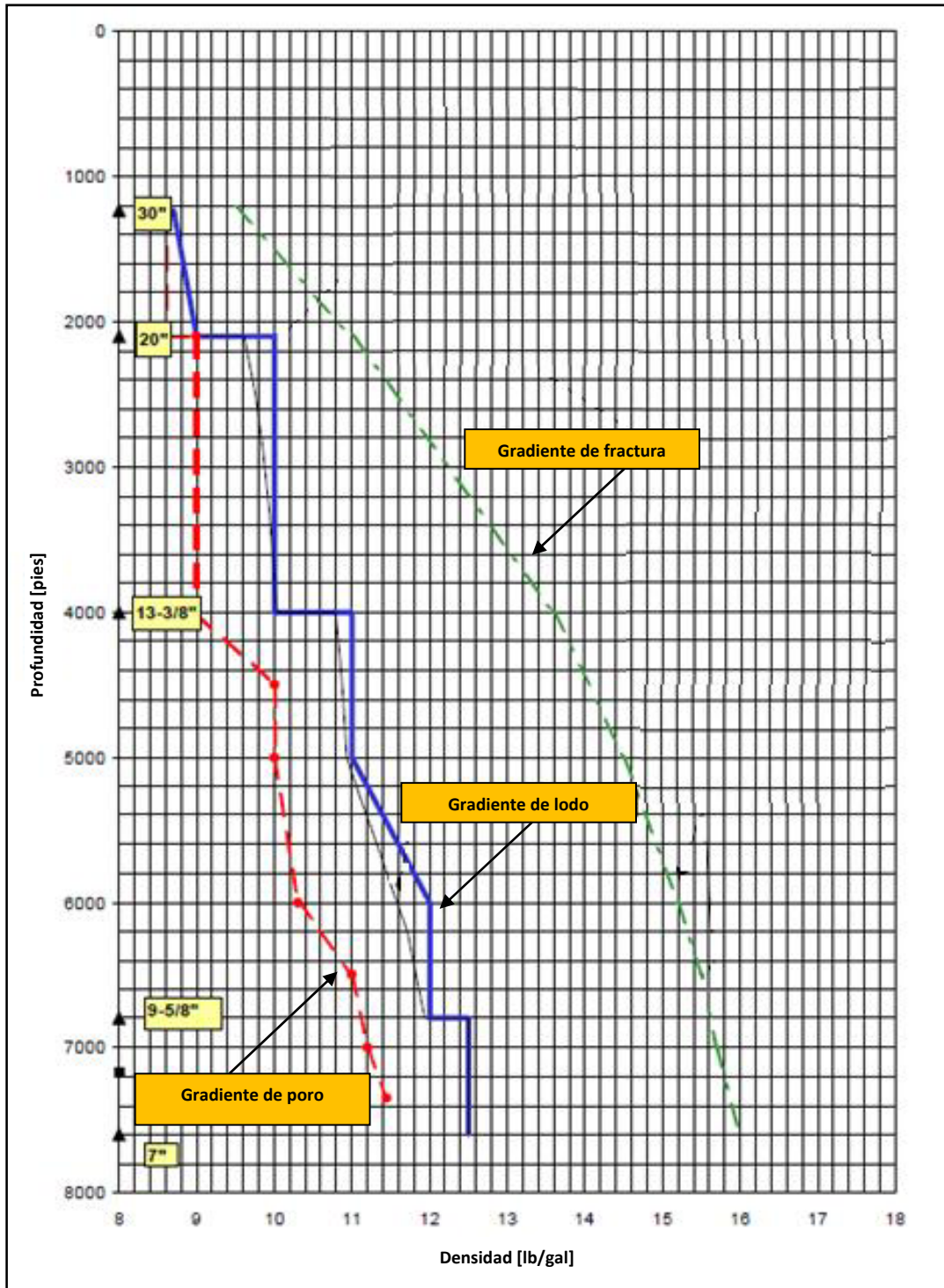
Figura 5.12. Diseño de asentamiento de TR para pozo piloto considerando de perforación convencional. Las presiones están dadas en su equivalente en densidad [lb/gal] 8
