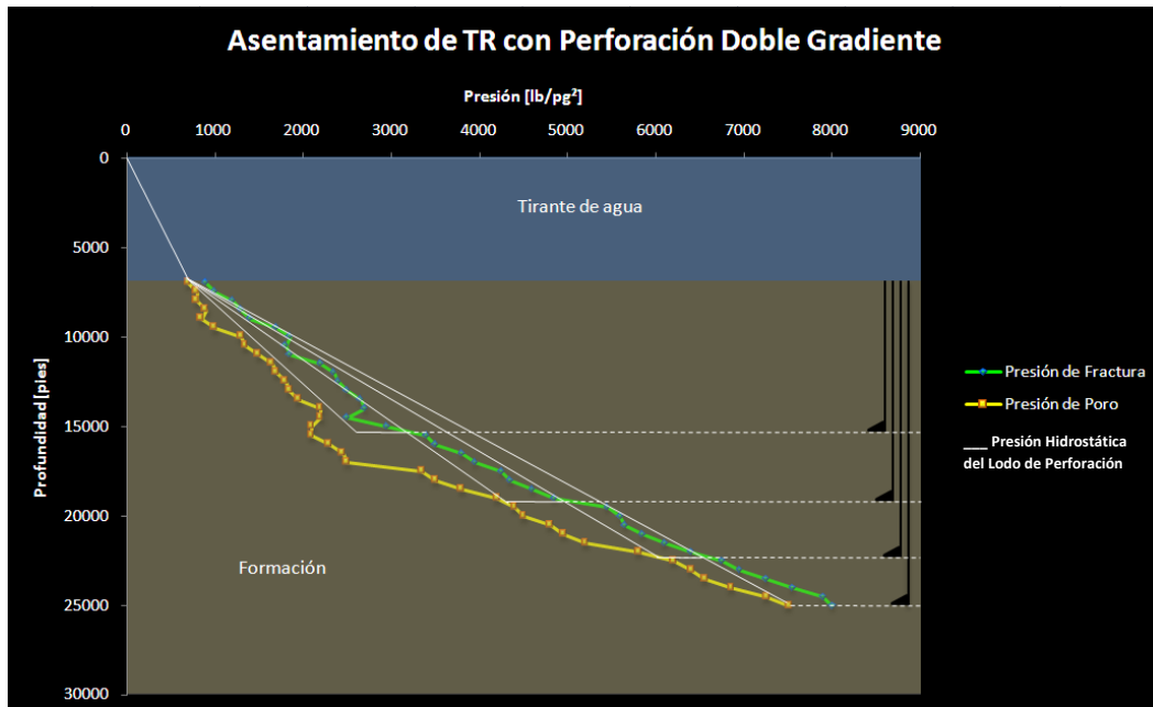
Figura 5.3. Asentamiento de TR empleando un sistema de perforación Doble Gradiente. Son requeridas solamente cuatro tuberías de revestimiento
