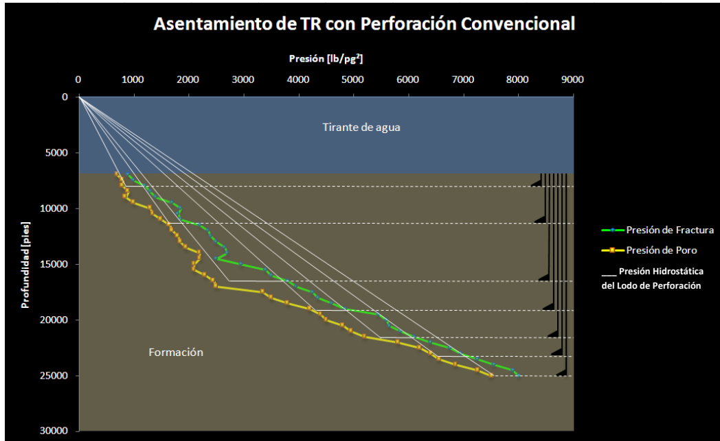
Figura 5.2. Asentamiento de TR empleando una perforación convencional. Son requeridas siete tuberías de revestimiento
