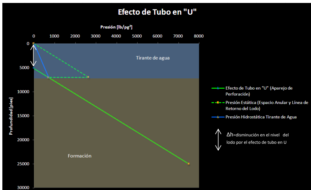
Figura 5.9. Efecto de Tubo en "U" dentro de la sarta de perforación. La prolongación de la línea verde desde el lecho marino hasta el eje de la profundidad, indica el nivel que alcanza el lodo para equilibrar las presiones cuando la bomba superficial se detiene
