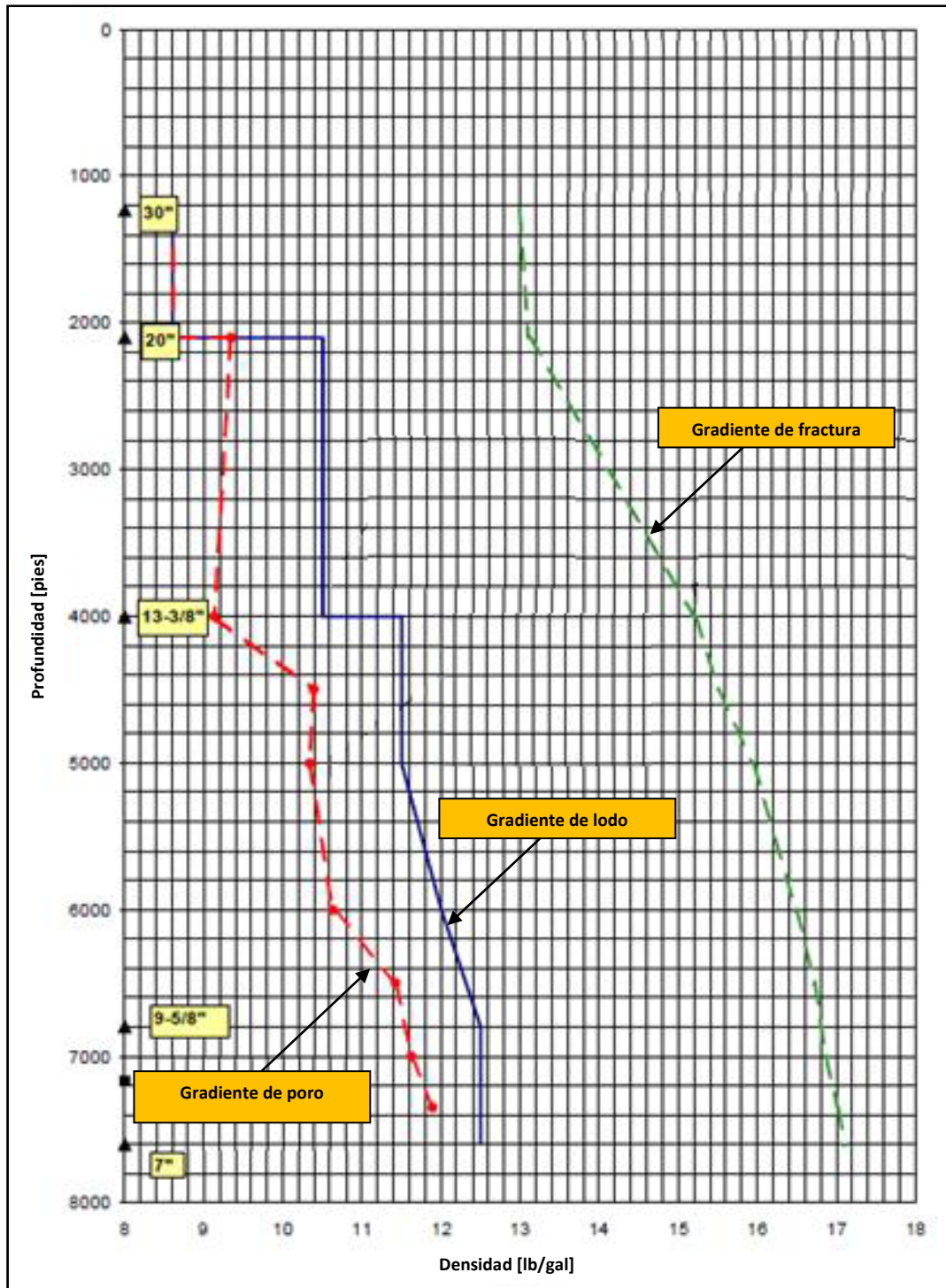
Figura 5.13. Diseño de asentamiento de TR para pozo piloto considerando de perforación Doble Gradiente. Las presiones están dadas en su equivalente en densidad [lb/gal]. En esta figura observamos una ventana operacional más amplia, lo que permite trabajar con un mayor margen de seguridad 8
