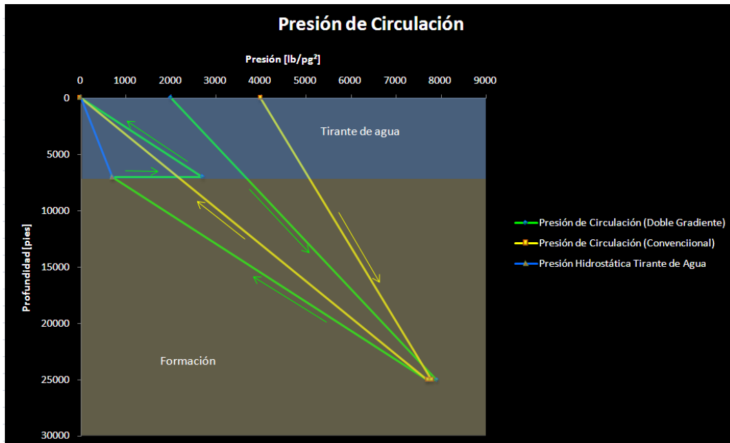
Figura 5.8. Variación de la presión de circulación del lodo en toda su trayectoria para ambos sistemas de perforación, convencional y Doble Gradiente
