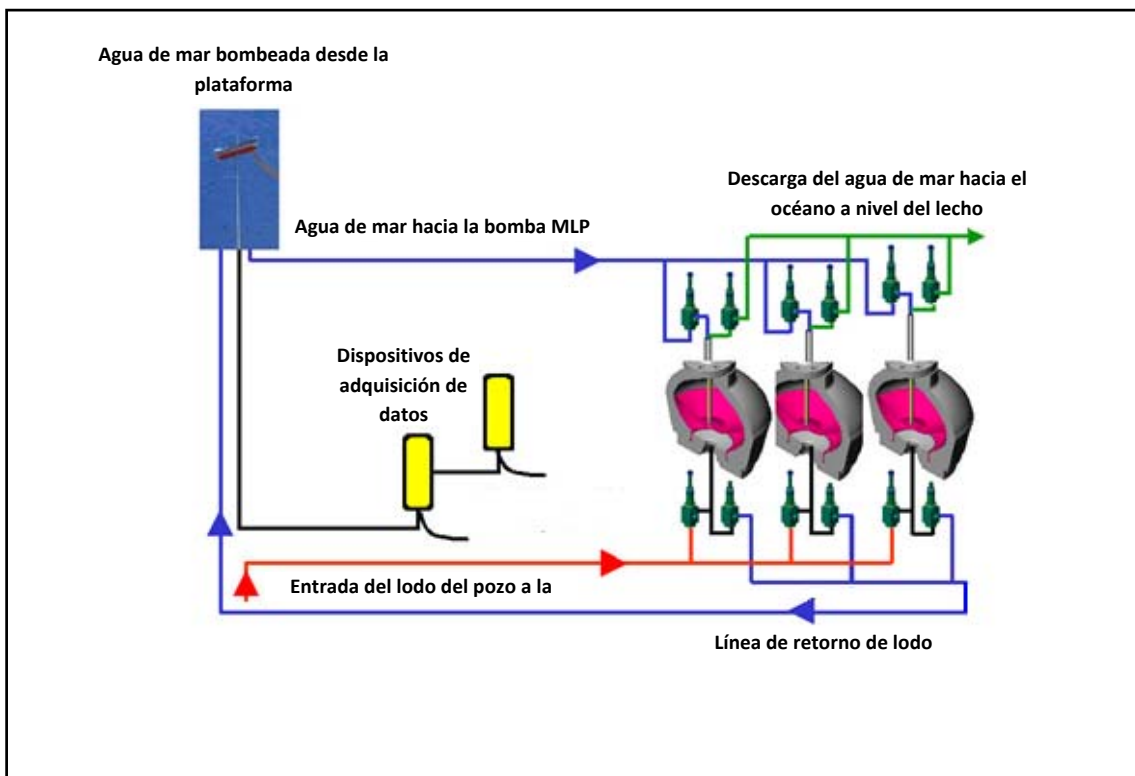
Figura 4.3. Esquema en el que se observa el agua de mar como fluido de potencia que es bombeado desde la superficie para accionar la bomba submarina de levantamiento de lodo 12
