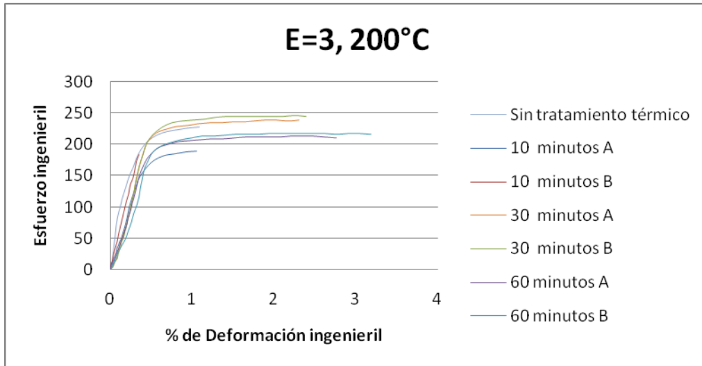
Gráfica 4.2. Esfuerzo-deformación \epsilon=3 . Recocido a 200°C.
