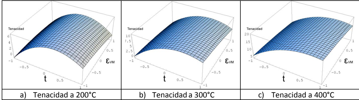
Imagen 4.16. Superficie de respuesta para tenacidad.
