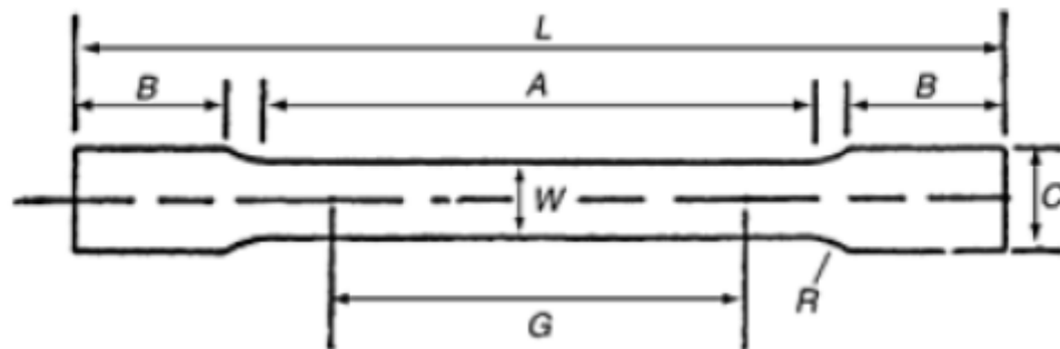
Imagen 3.1. Esquema de una probeta de tracción [22].
