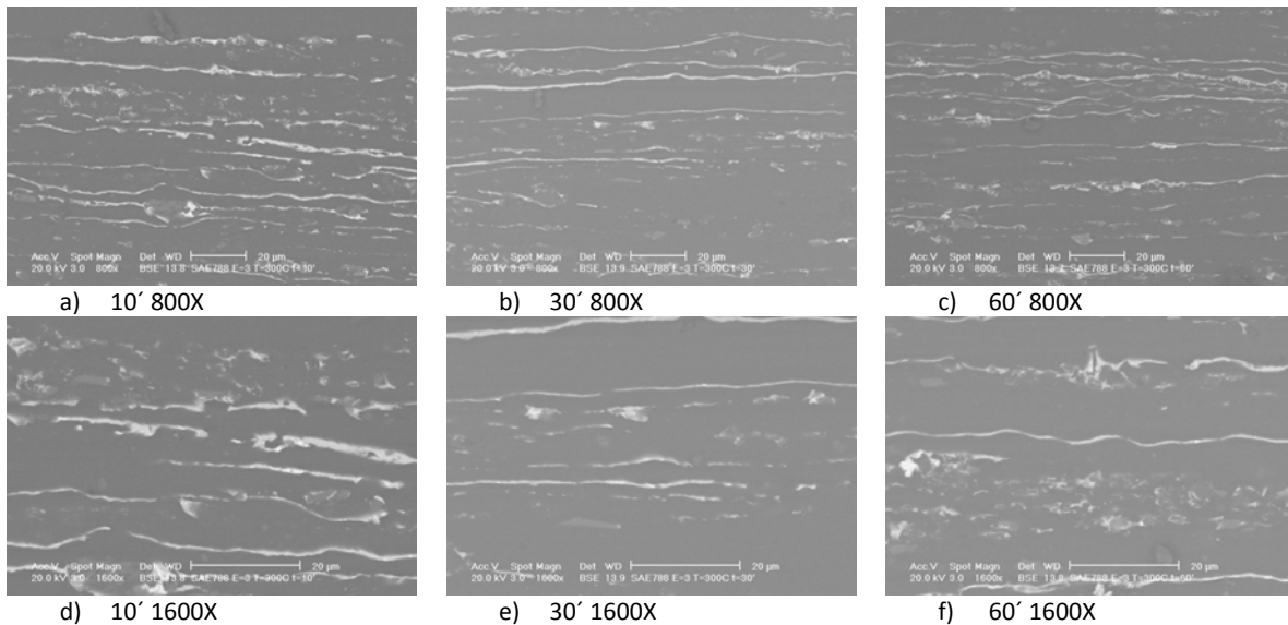
Imagen 4.3. Microestructuras de las probetas con \epsilon=3 recocidas a 300°C.
