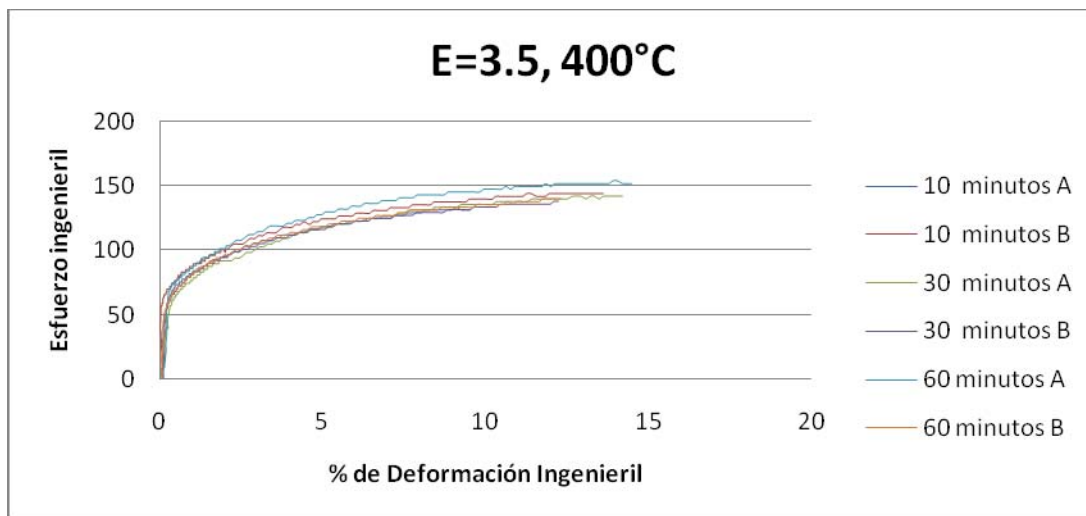
Gráfica 4.8. Esfuerzo-deformación \epsilon=3.5 . Recocido a 400°C.
