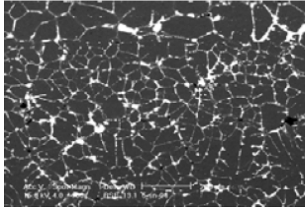
Imagen 2.1. Aleación SAE – 788 sin refinador [16].
