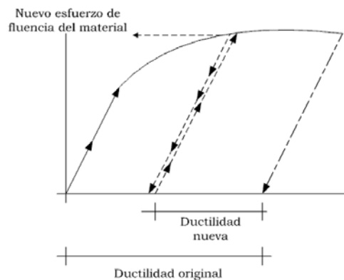
Imagen 2.5. Curva en la que se observa que al deformar plásticamente se disminuye la ductilidad del material.
