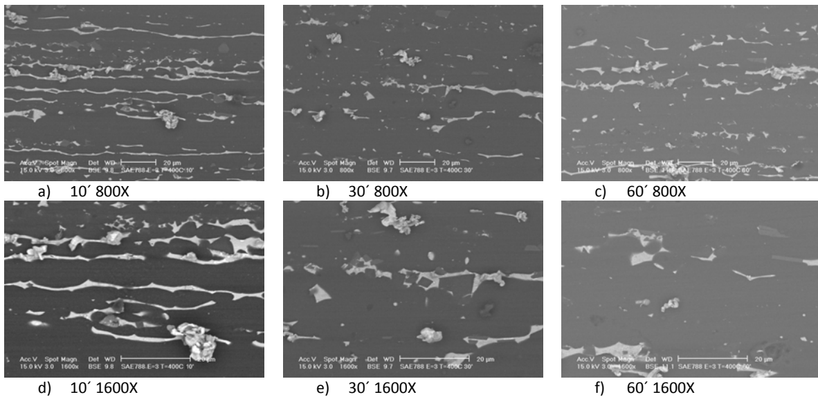
Imagen 4.4. Microestructuras de las probetas con \epsilon=3 recocidas a 400°C.
