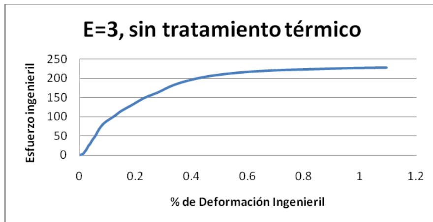
Gráfica 4.1. Esfuerzo–Deformación \epsilon=3 . STT.
