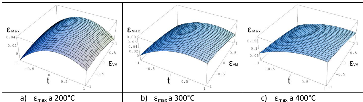
Imagen 4.14. Superficie de respuesta para deformación máxima.
