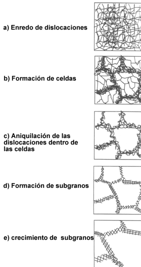
Imagen 2.7. Etapas en la deformación en frío y de la recuperación de un material [19].
