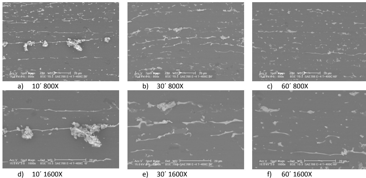
Imagen 4.12. Microestructuras de las probetas con \epsilon=4 recocidas a 400°C.
