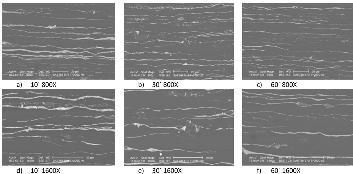
Imagen 4.2. Microestructuras de las probetas con \epsilon=3 recocidas a 200°C.
