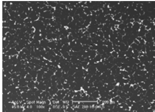
Imagen 2.2. Aleación SAE- 788 con 0.1% de refinador [16].
