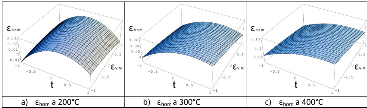
Imagen 4.13. Superficie de respuesta para deformación homogénea.
