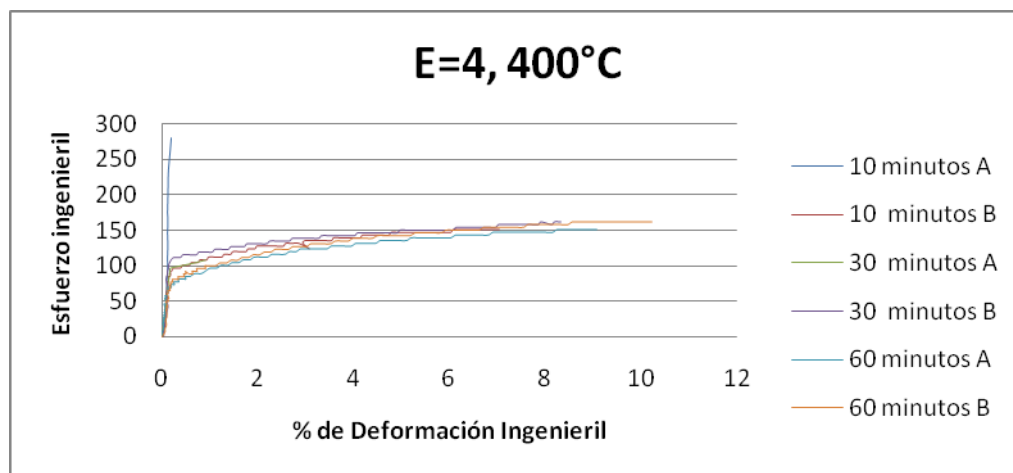
Gráfica 4.12. Esfuerzo-deformación para \epsilon=4 . Recocido a 400°C.
