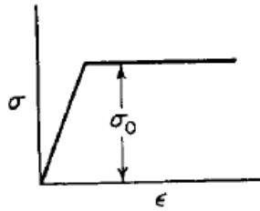
Imagen 2.4. Comportamiento idealmente plástico [13].
