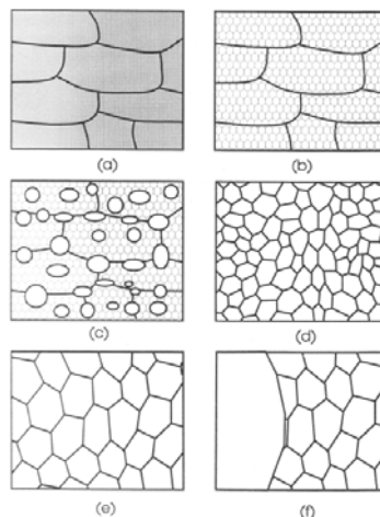
Imagen 2.8. Diagrama esquemático de las etapas en el proceso de recocido. a) Estado deformado, b) Recuperación, c) Recristalización parcial, d) Recristalización total, e) Crecimiento de grano, f) Crecimiento anormal de grano [19].
