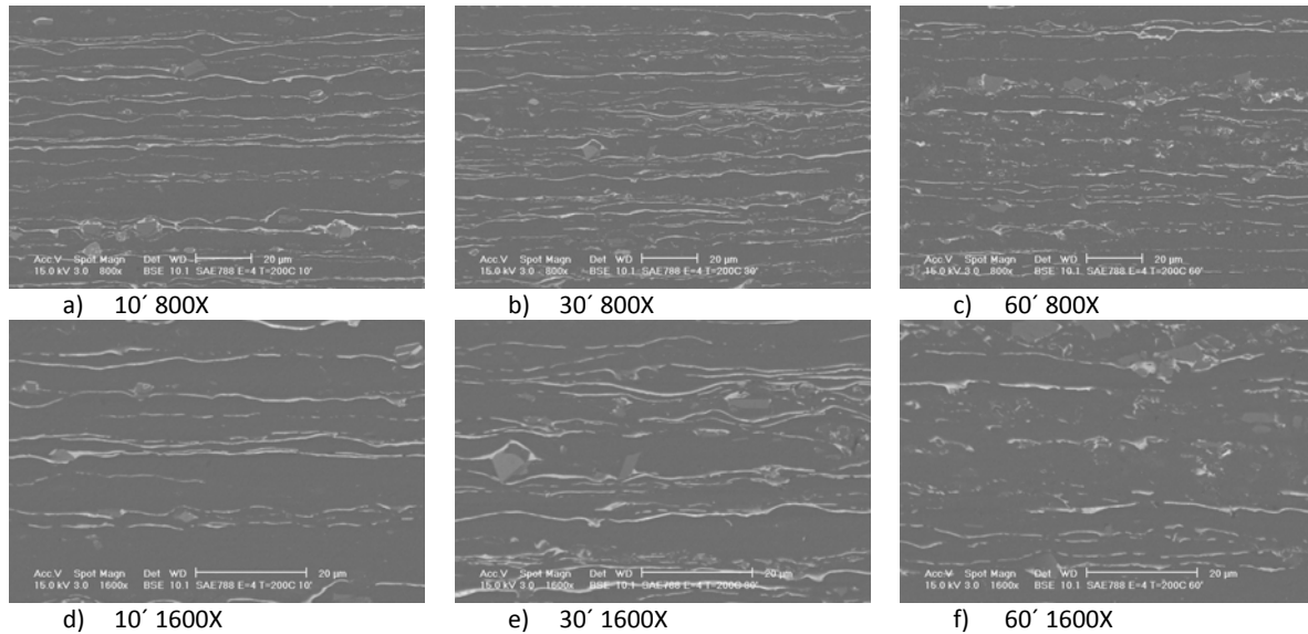
Imagen 4.10. Microestructuras de las probetas con \epsilon=4 recocidas a 200°C.
