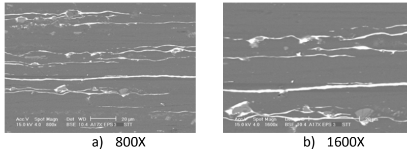
Imagen 4.1. Microestructuras de las probetas con \epsilon=3 sin tratamiento térmico.
