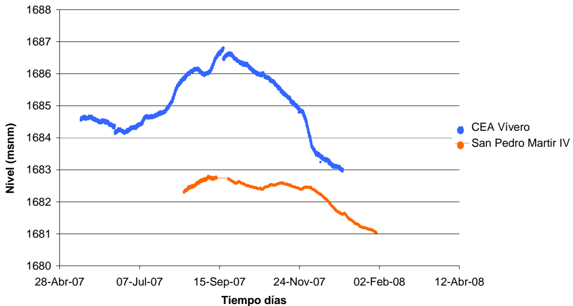
Figura 30. Evolución Piezométrica de los pozos CEA Vívero, San Pedro Martir IV y Reforma Agraria
