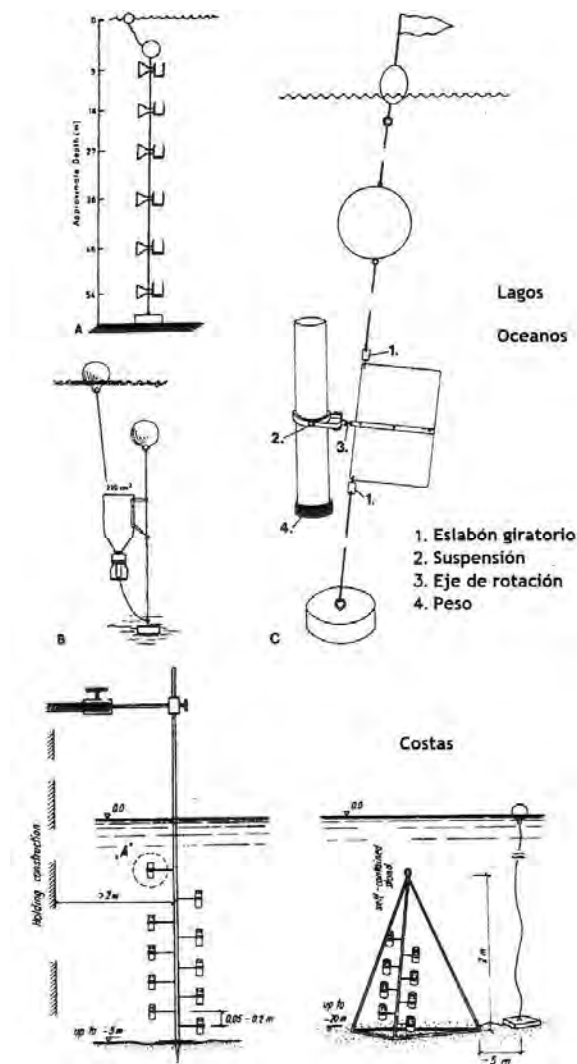
Figura 3. 13 Trampa integradora de tiempo
