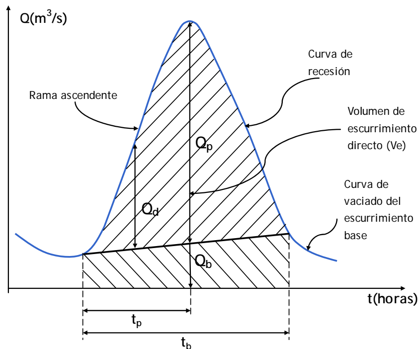
Figura 1. 3 Hidrograma típico
