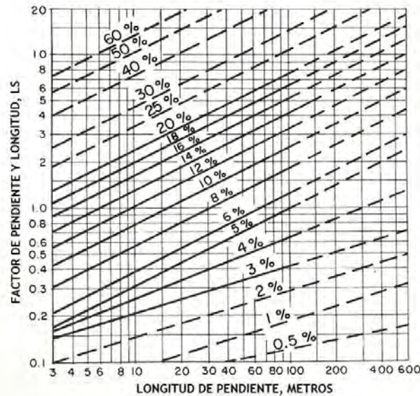
Figura 1. 9 Factor de Longitud de pendiente y pendiente, LS, para su uso con la Ecuación Universal de Pérdida de Suelo
