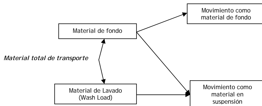
Figura 1. 1 Tipos de transporte de sedimentos
