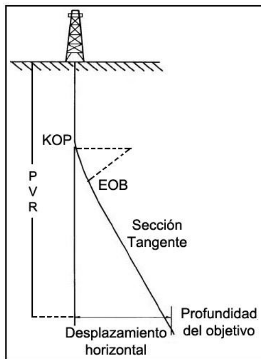
Fig. 1.2. Perfil básico de un pozo tipo I
