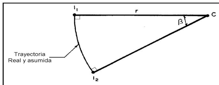
Fig. 5.12. Diferencia entre la trayectoria real vs la calculada por el método de radio de curvatura
