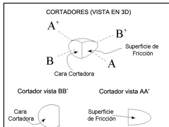
Fig. 2.6. Vista en diferentes planos de un cortador
