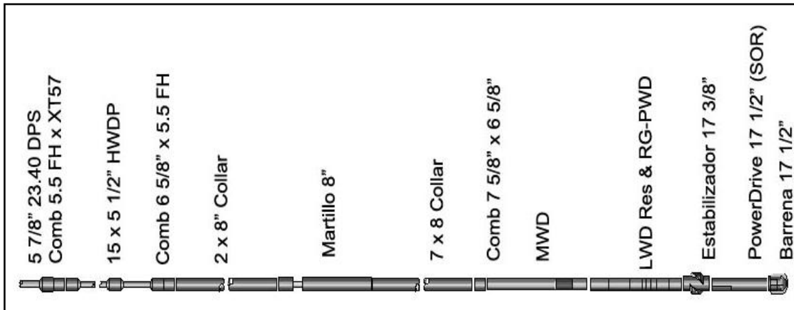
Fig. 6.15. Arreglo del ensamble de fondo para la sección de construcción
