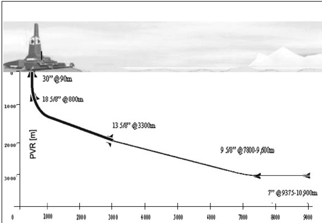
Fig. 6.12. Arreglo típico de los pozos de alcance extendido en el campo Chayvo
