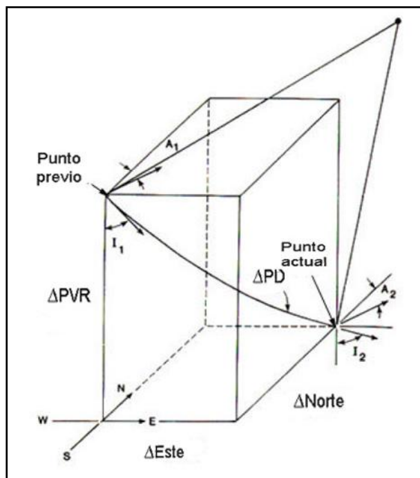
Fig. 5.9. Representación gráfica de 2 puntos por el método de Radio de curvatura
