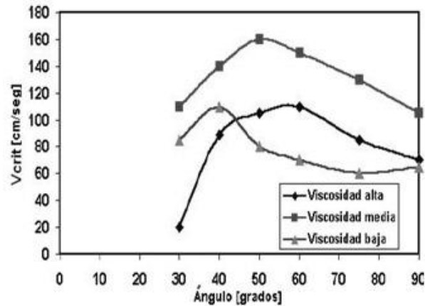
Fig. 3.14. Efecto de la reología del fluido sobre el rodamiento de recortes a diferentes ángulos de inclinación
