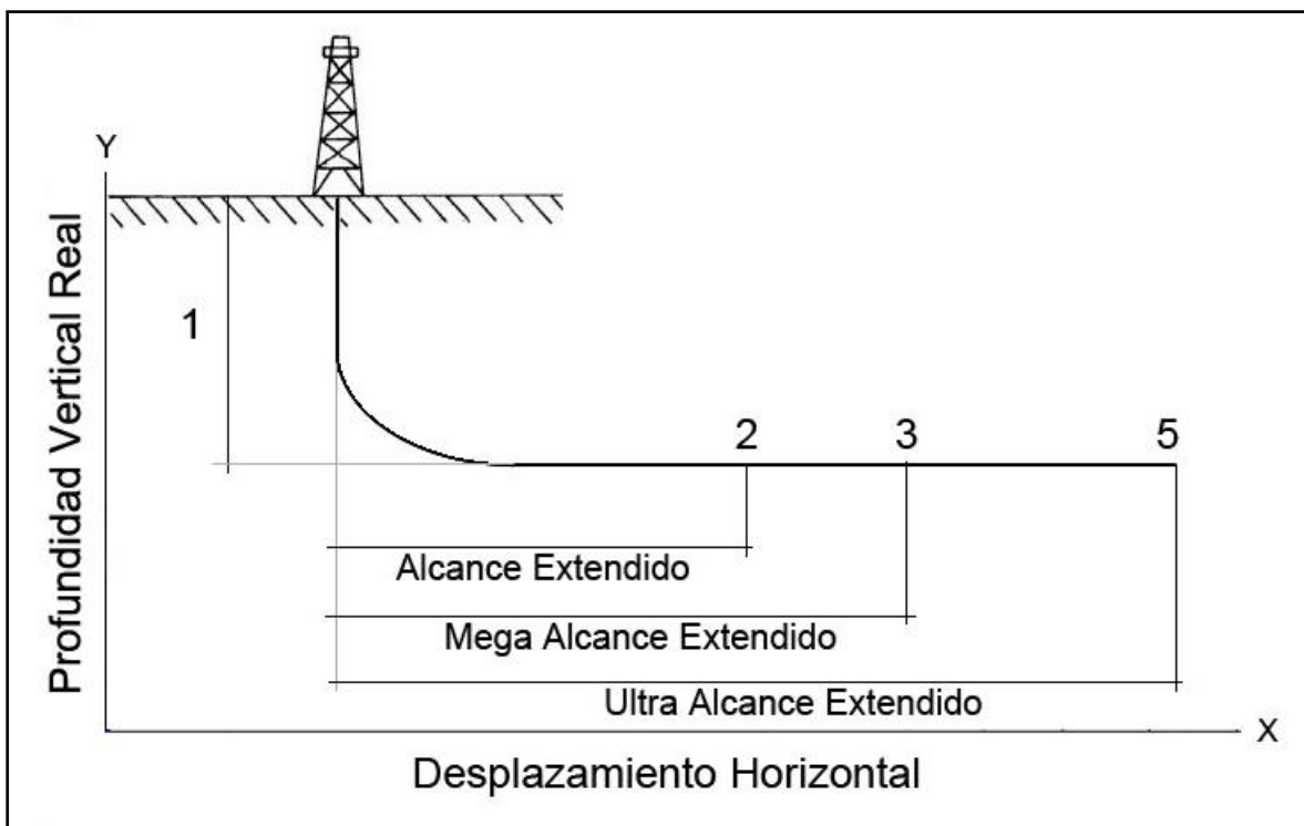
Fig. 1.8. Clasificación de acuerdo a su relación DH/PVR
