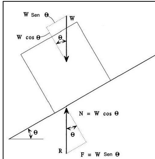
Fig. 4.6. Diagrama de cuerpo libre de un cuerpo en un plano inclinado
