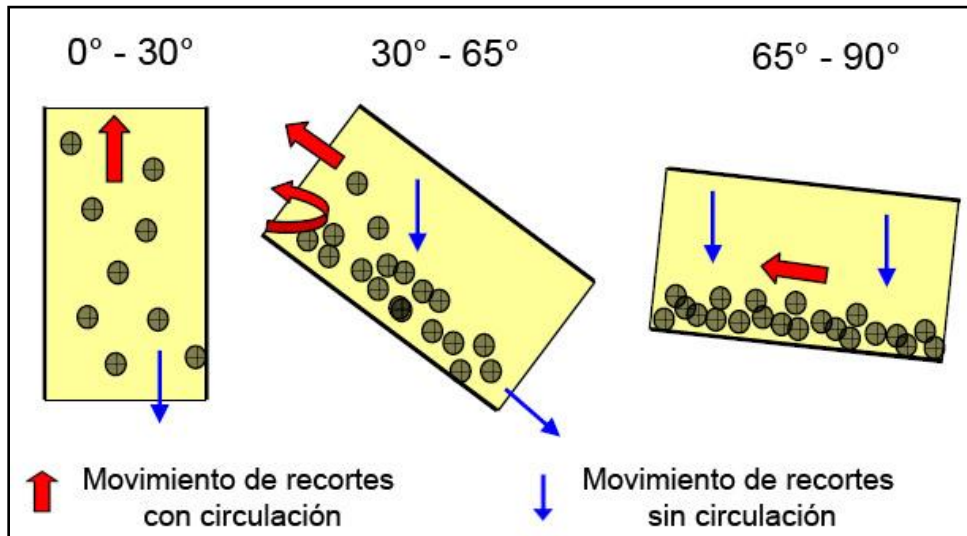
Fig. 3.3. Formación de recortes en un pozo de alcance extendido
