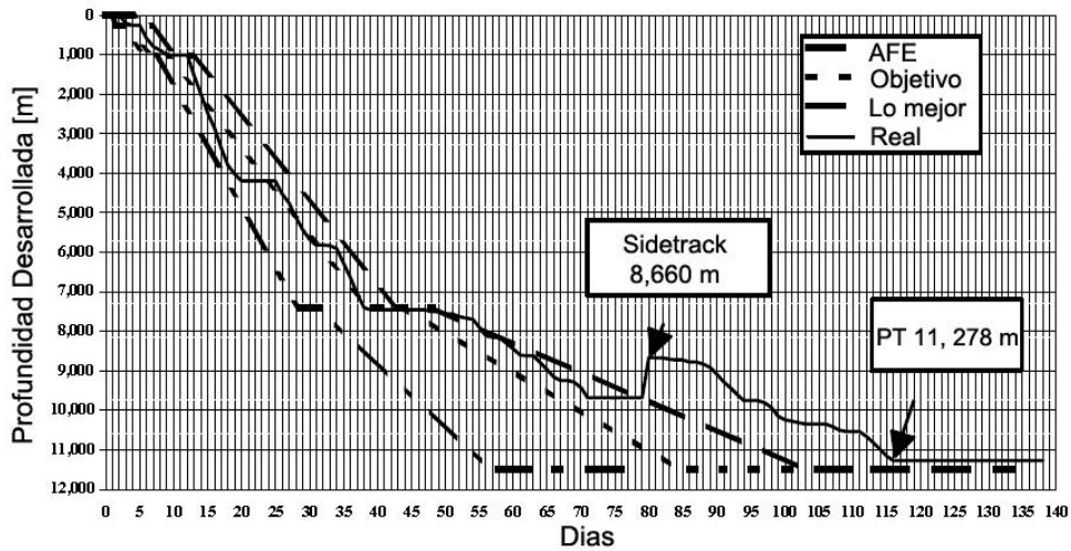
Fig. 6.7. Tiempo de perforación del pozo M-16Z
