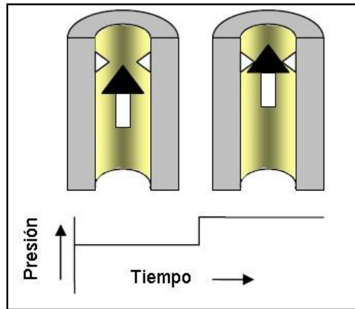
Fig. 2.10. Diagrama de pulso positivo
