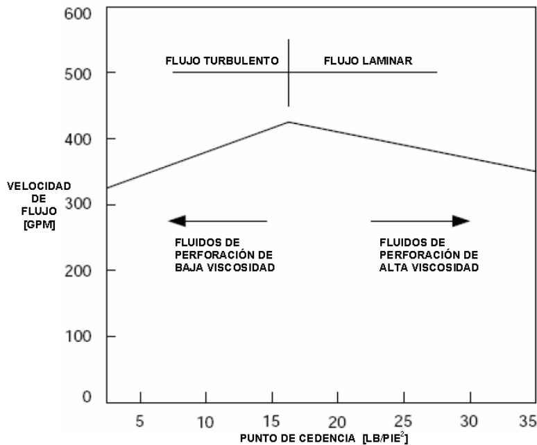
Fig. 3.11. Efecto del punto de cedencia en el régimen de flujo
