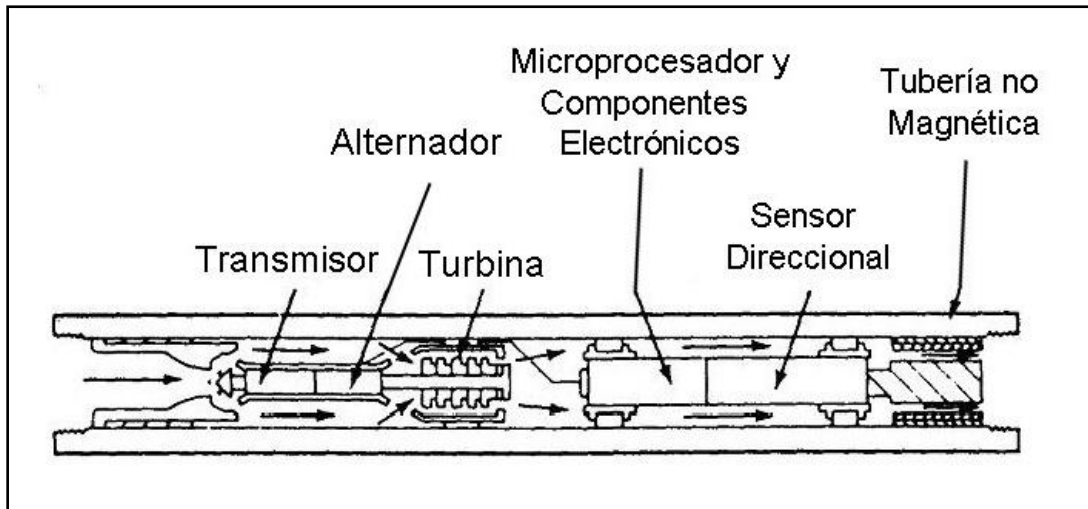
Fig. 2.8. Principales componentes de la tecnología MWD
