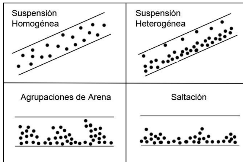
Fig. 3.6. Mecanismos de transporte por suspensión
