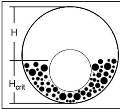
Fig. 3.5. Altura crítica de la cama de recortes
