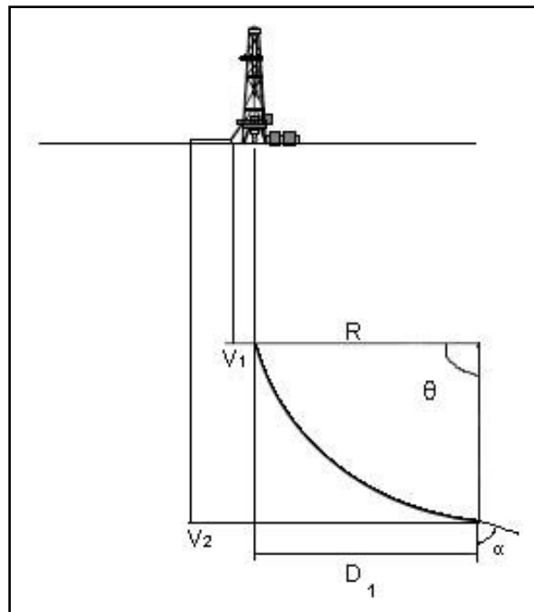
Fig. 5.4. Geometría de un pozo de incremento continuo
