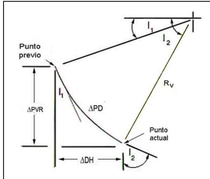
Fig. 5.10. Esquema Rv
