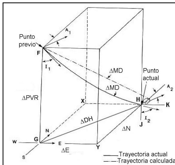
Fig. 5.6. Representación gráfica de 2 puntos por el método tangencial
