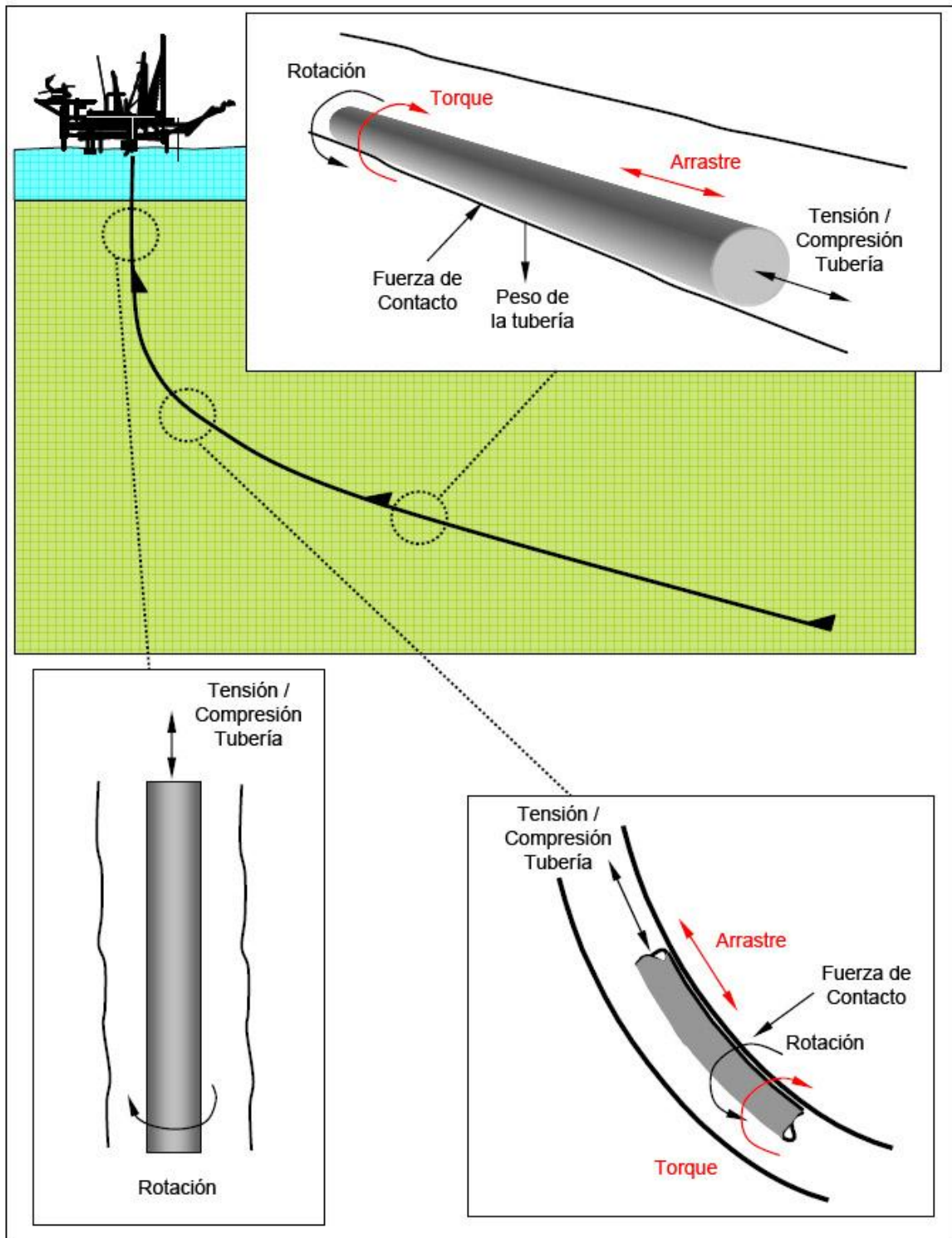
Fig. 4.1. Fuerzas que actúan en la tubería de perforación a diferentes ángulos
