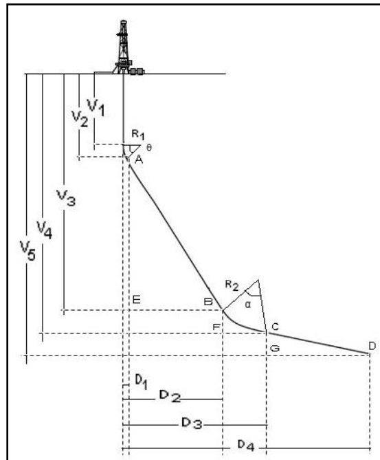
Fig. 5.5. Geometría de un pozo de doble construcción
