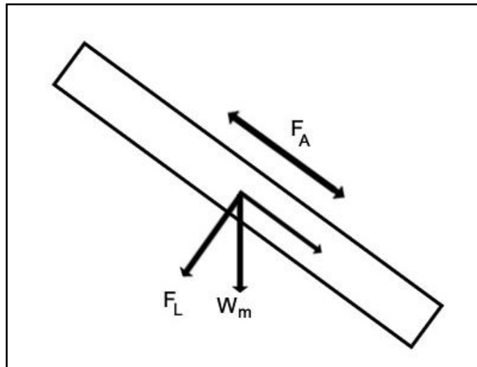
Fig. 4.7. Fuerza axial y lateral de contacto en una sección tangente
