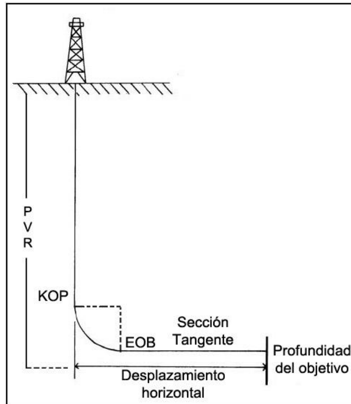
Fig. 1.5. Perfil básico de un pozo tipo IV
