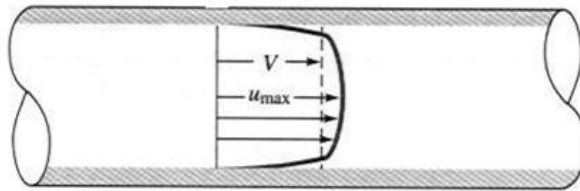
Fig. 3.10. Perfil de velocidad en flujo turbulento
