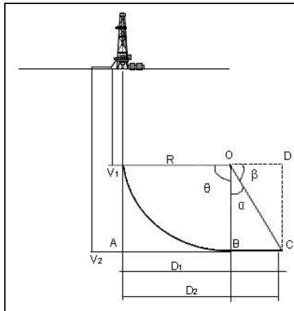
Fig. 5.3. Geometría de un pozo con radio de curvatura largo y una sección tangente de 90°
