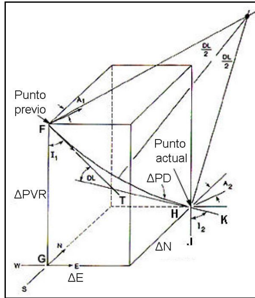
Fig. 5.13. Representación gráfica de 2 puntos por el método de Mínima curvatura
