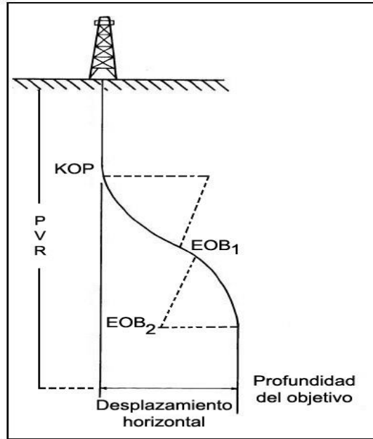
Fig. 1.3. Perfil básico de un pozo tipo II
