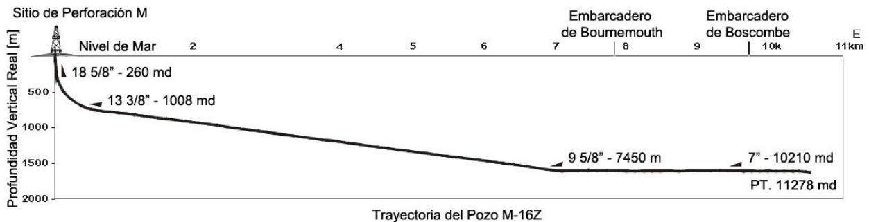
Fig. 6.5. Perfil del pozo M-16Z
