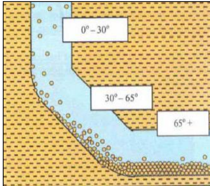
Fig. 1.9. Acumulación de recortes a diferentes ángulos
