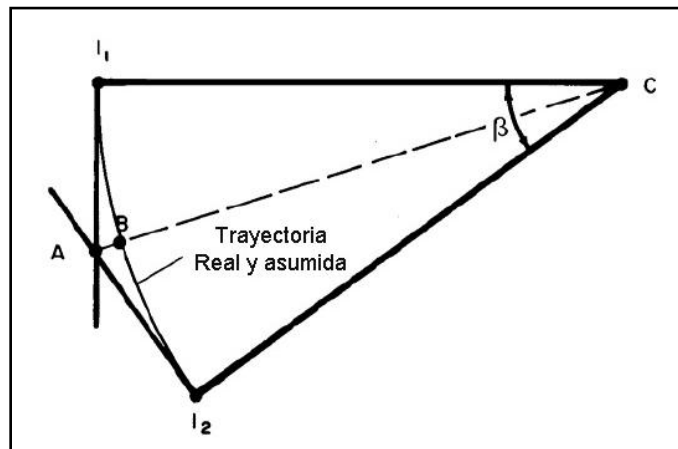
Fig. 5.14. Diferencia entre la trayectoria real vs la calculada por el método de Mínima curvatura
