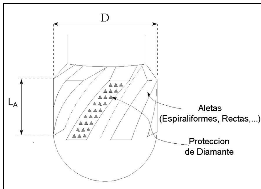
Fig. 2.7. Descripción de las aletas
