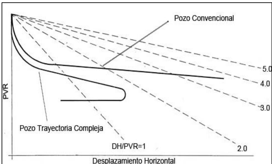
Fig. 1.7. Definición DH/PVR vs PD/PVR
