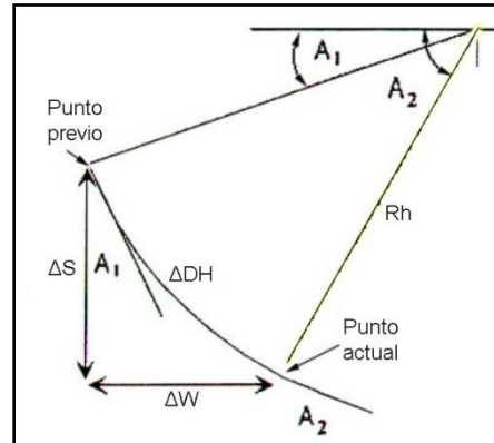
Fig. 5.11. Esquema Rh
