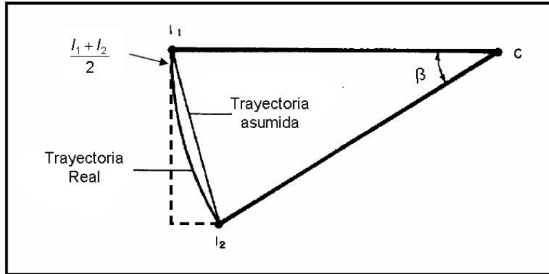
Fig. 5.8. Diferencia entre la trayectoria real vs la calculada por el método de ángulo promedio
