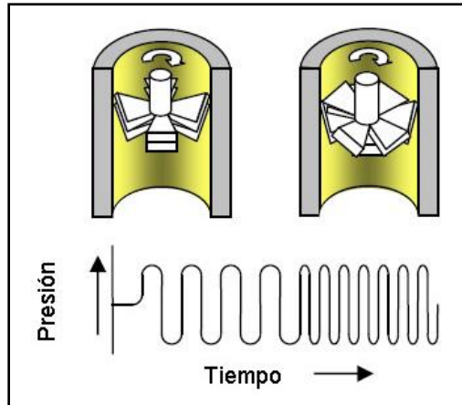
Fig. 2.12. Diagrama de ondas continuas
