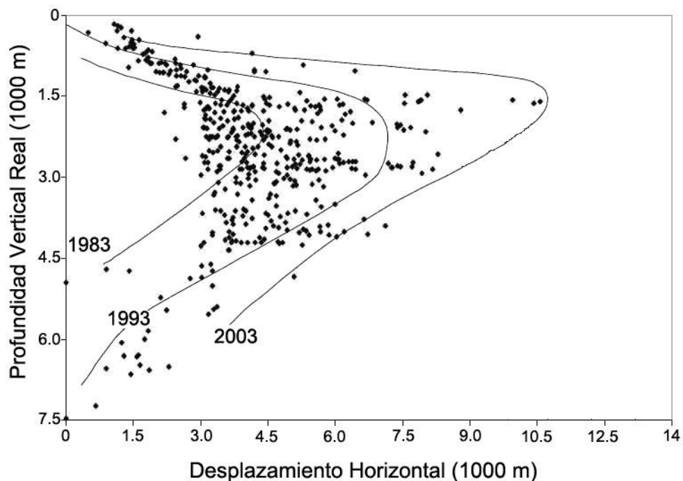
Fig. 1.1. Evolución del alcance de la perforación de alcance extendido a nivel mundial
