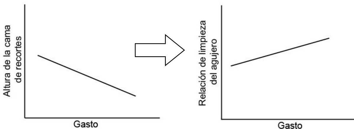
Fig. 3.12. Efecto del gasto sobre la altura de la cama de recortes
