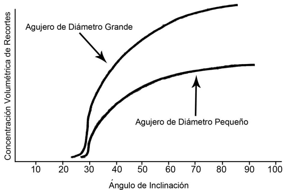
Fig. 3.2. Concentración de recortes a diferentes ángulos
