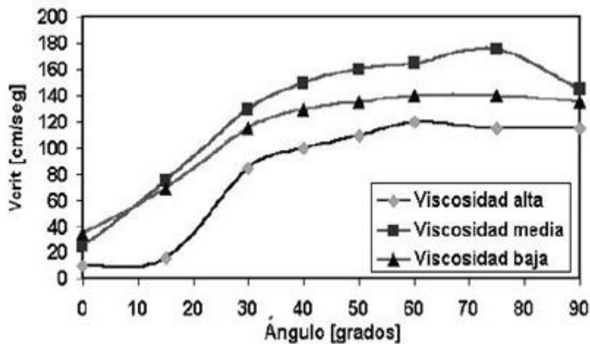
Fig. 3.13. Efecto de la reología del fluido sobre la suspensión de recortes a diferentes ángulos de inclinación
