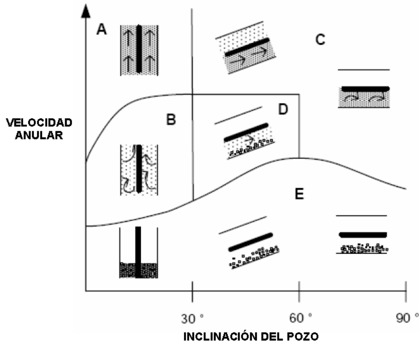
Fig. 3.15. Zonas de limpieza de un pozo de acuerdo a su inclinación y velocidad anular
