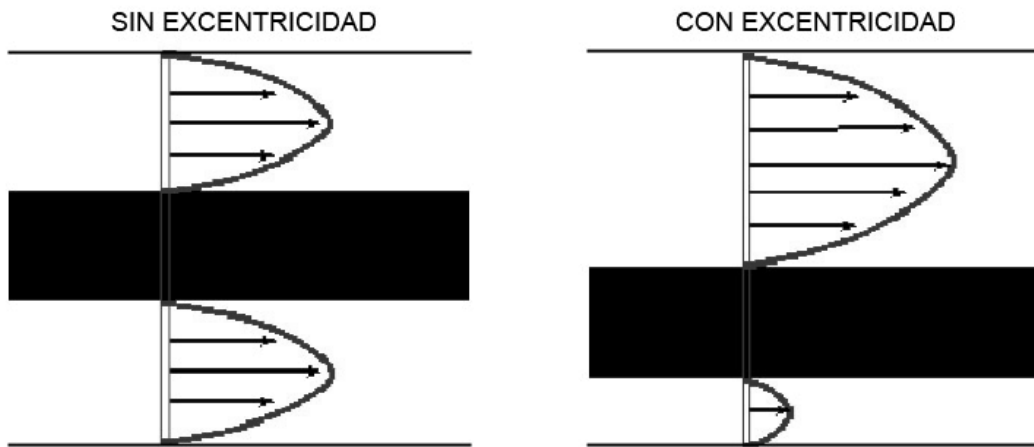
Fig. 3.17. Efecto de la excentricidad de la tubería sobre la velocidad del fluido
