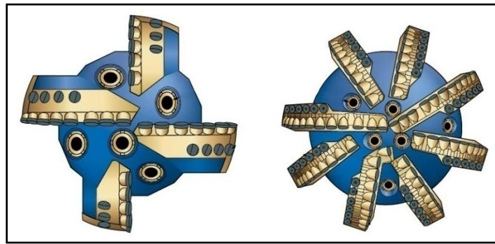
Fig. 2.5. Diferentes tipos de estructuras de corte
