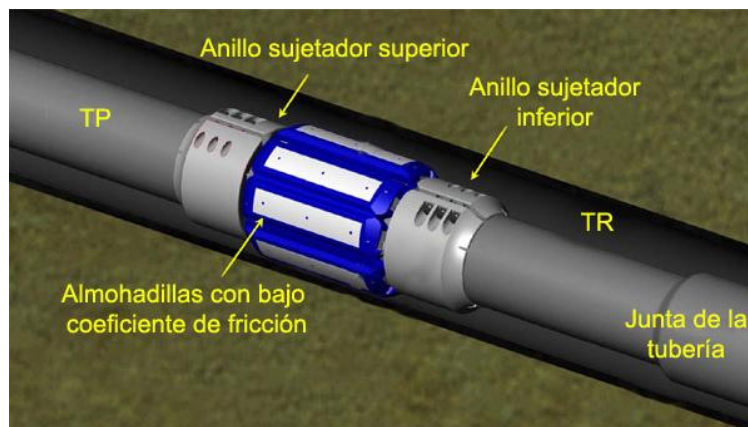
Fig. 4.5. Protector no-rotatorio de la marca Western Well Tool
