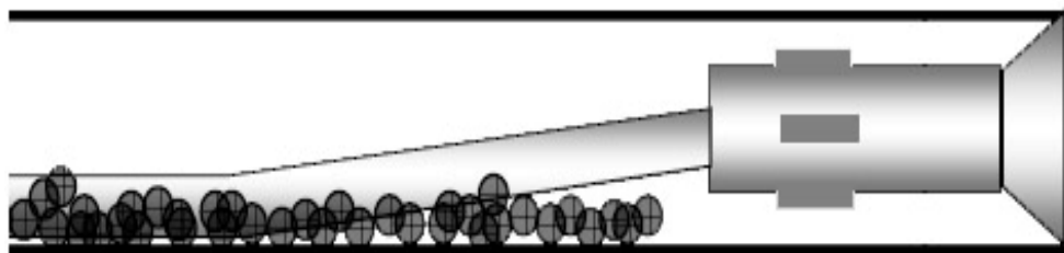
Fig. 3.4. Fenómeno de arado
