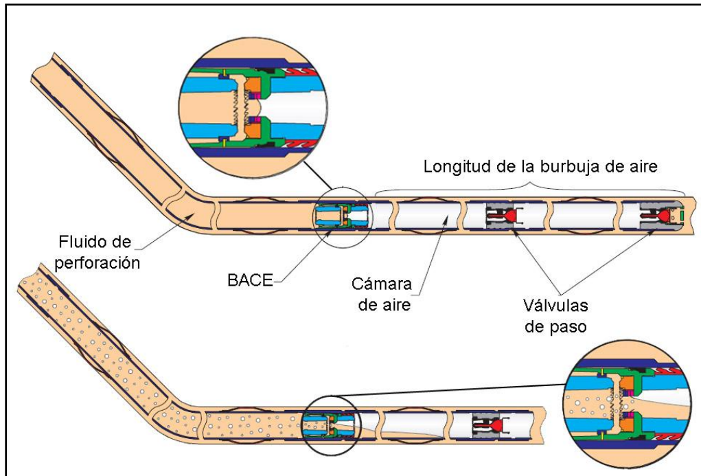
Fig. 2.13. Técnica de flotación de TR
