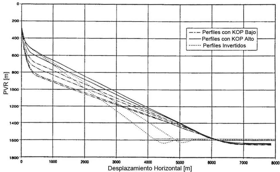
Fig. 4.3. Diferentes perfiles direccionales para un mismo pozo
