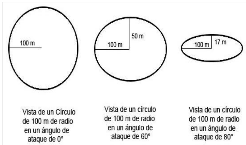
Fig. 1.10. Efecto del ángulo de ataque en forma y tamaño
