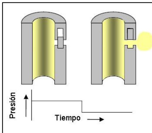
Fig. 2.11. Diagrama de pulso negativo
