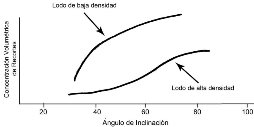
Fig. 3.8. Efecto de la densidad del lodo en la altura de la cama de recortes
