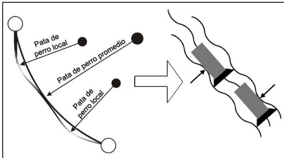
Fig. 4.2. Tortuosidad en un pozo direccional
