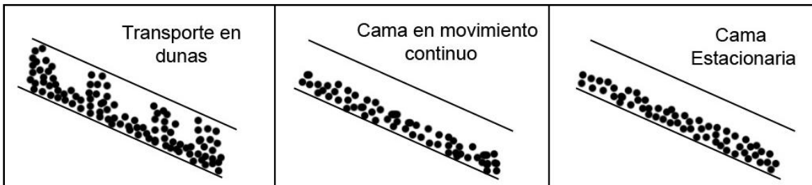
Fig. 3.7. Mecanismos de transporte por rodamiento
