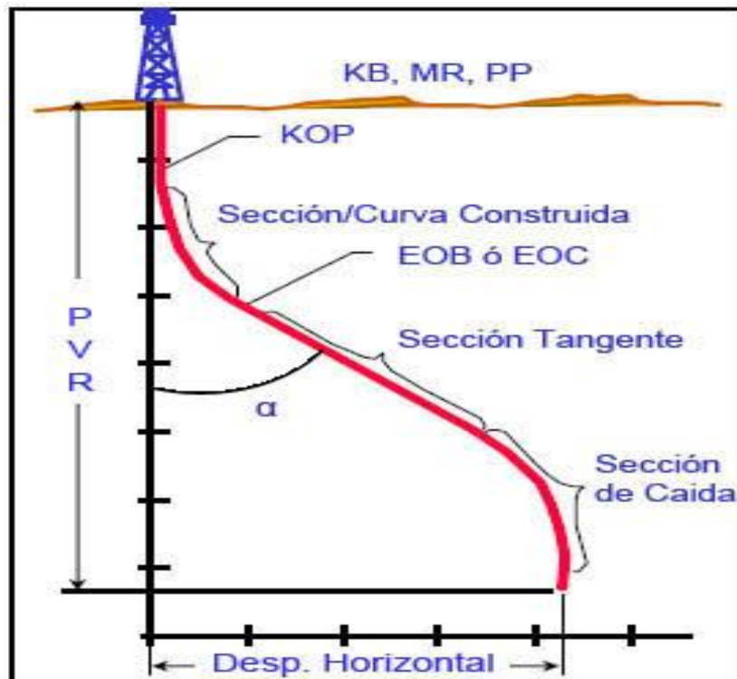
Fig.1.6. Nomenclatura usada en pozos direccionales
