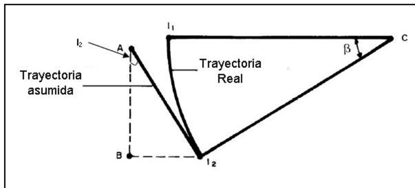
Fig. 5.7. Diferencia entre la trayectoria real vs la calculada por el método tangencial
