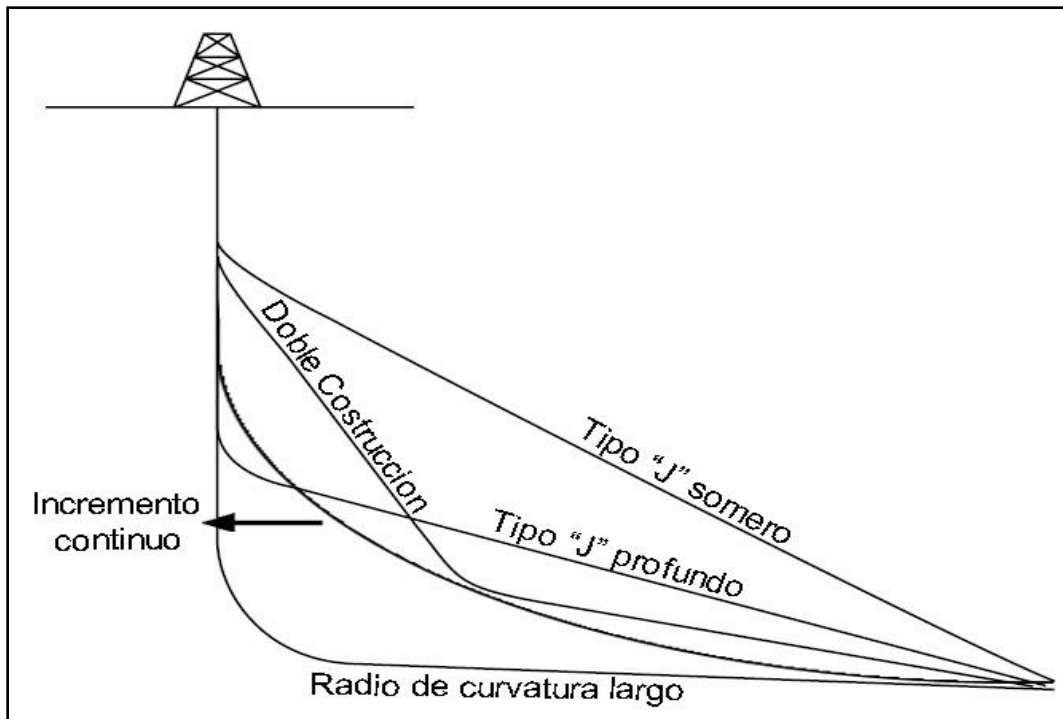
Fig. 5.1. Diferentes tipos de trayectorias para pozos de alcance extendido
