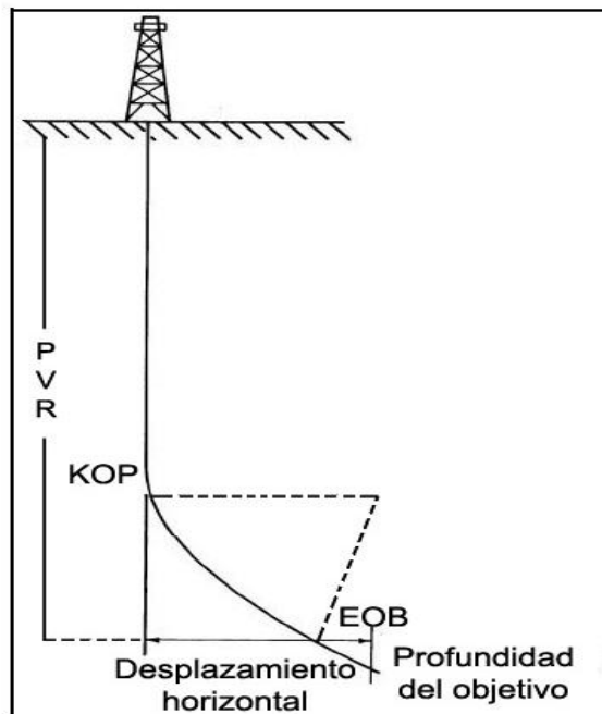
Fig. 1.4. Perfil básico de un pozo tipo III
