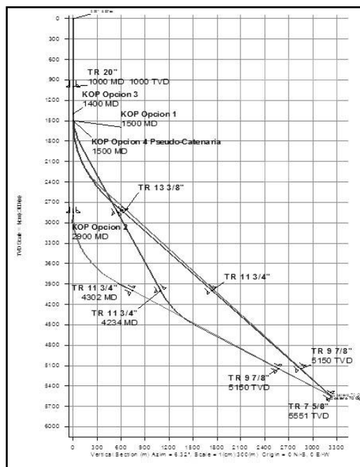
Fig. 6.14. Diferentes trayectorias estudiadas
