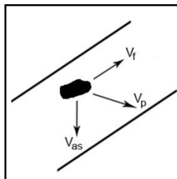
Fig. 3.1. Diagrama de cuerpo libre de una partícula en un pozo direccional
