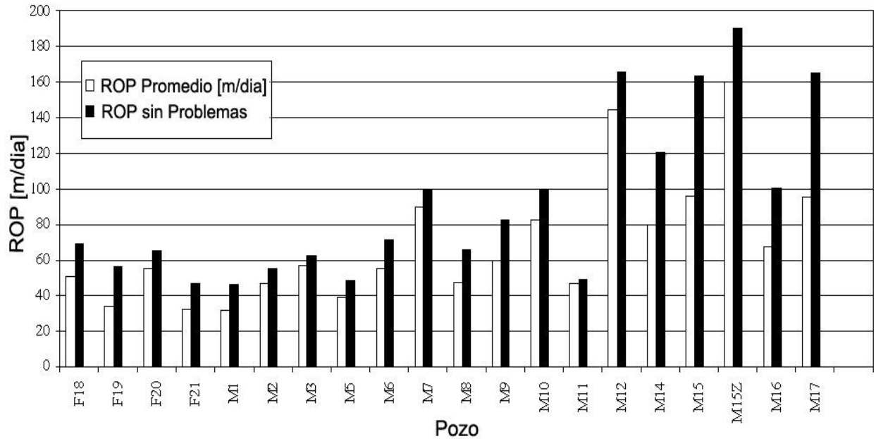
Fig. 6.6. Ritmo de penetración promedio por pozo
