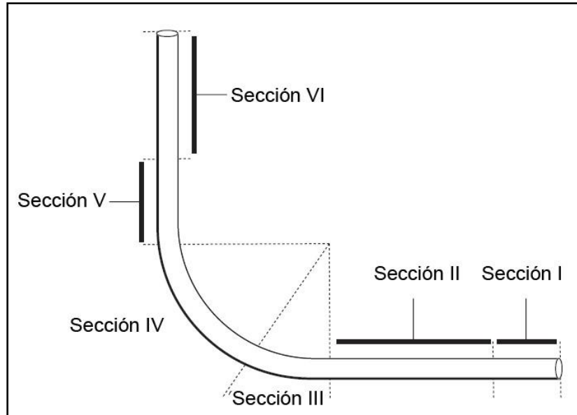
Fig. 4.4. Secciones de un pozo tomando en cuenta el torque y arrastre
