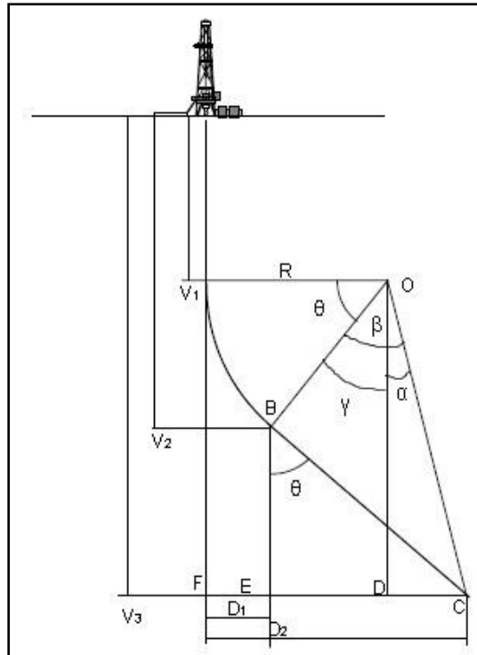
Fig. 5.2. Geometría de un pozo tipo "J"
