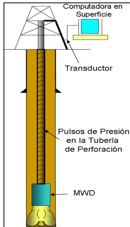
Fig. 2.9. Esquema de transmisión de datos
