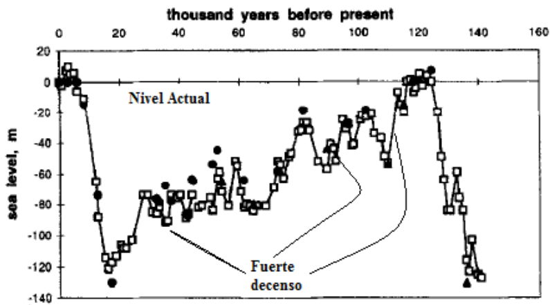
Figura 2.4: Nivel del mar durante los últimos 140 mil años según terrazas de coral de Huon (nueva Guinea) (extraído y modificado de Chappell J. et al., 1986).
