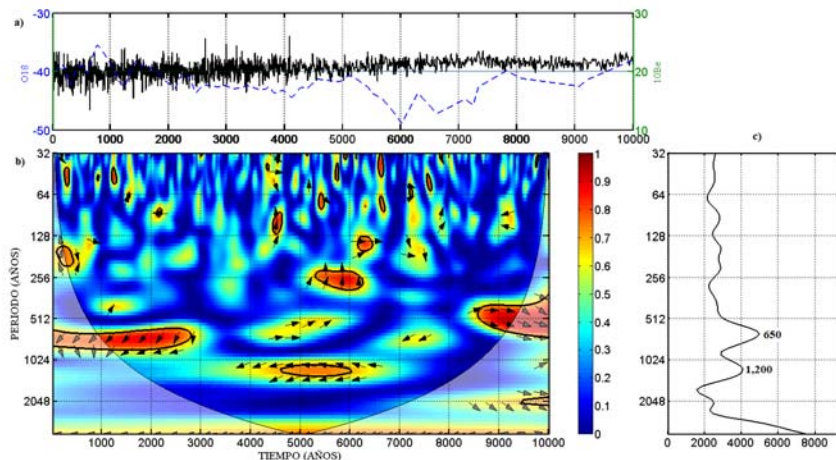
Figura 5.11: Espectro Wavelet de Coherencia entre el berilio-10 e isótopos de oxígeno-18 del polo Sur, a) serie de tiempo del berilio-10 e isótopos de oxígeno-18, b) espectro Wavelet de Coherencia, c) espectro Wavelet Global.
