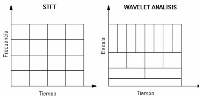
Figura 4.6: Plano tiempo-frecuencia de STFT y tiempo-escala de CWT
