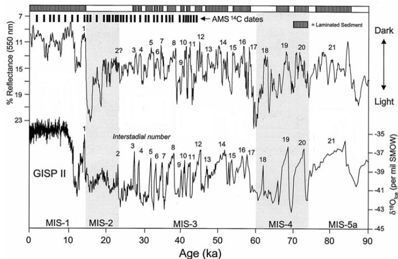
Figura 3.14: Inestabilidad climática de la última glaciación, la gráfica de arriba muestra los registros de los sedimentos de la cuenca tropical carriaco de Venezuela, y la gráfica de abajo muestra los registros obtenidos del sondeo en el pozo GISP2 (extraído de Larry C. Peterson, et al., 2000)
