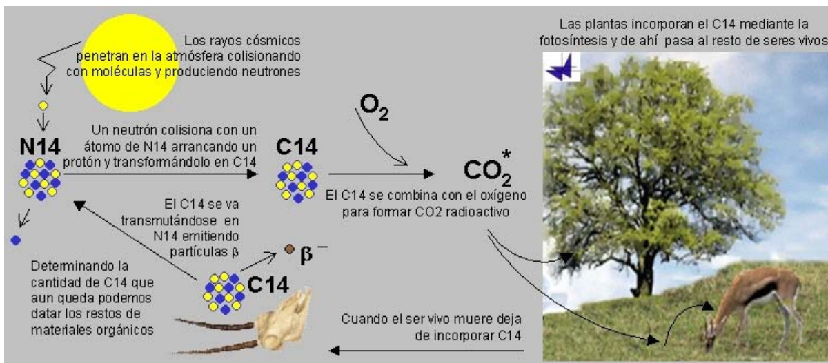
Figura 3.7: Proceso de generación-degradación del ^{14}C
