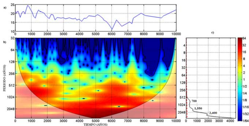
Figura 5.5: Espectro Wavelet del Berilio-10 del polo Sur, a) serie de tiempo del Berilio-10, b) espectro Wavelet Morlet, c) espectro Wavelet Global.
