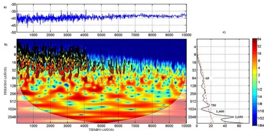
Figura 5.4: Espectro Wavelet de los isótopos de oxígeno-18 del polo Sur, a) serie de tiempo de los isótopos de oxígeno-18, b) espectro Wavelet Morlet, c) espectro Wavelet Global.
