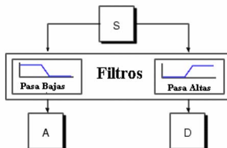
Figura 4.8: Proceso de filtración de una señal mediante análisis Wavelet
