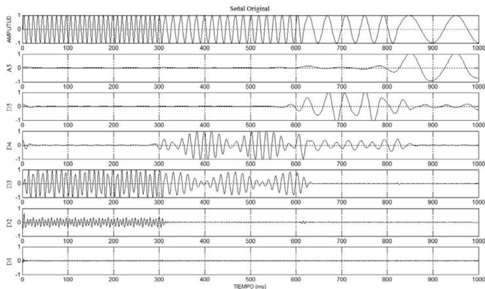
Figura 4.10: Descomposición de la señal no estacionaria, el nivel de descomposición utilizado fue de 5
