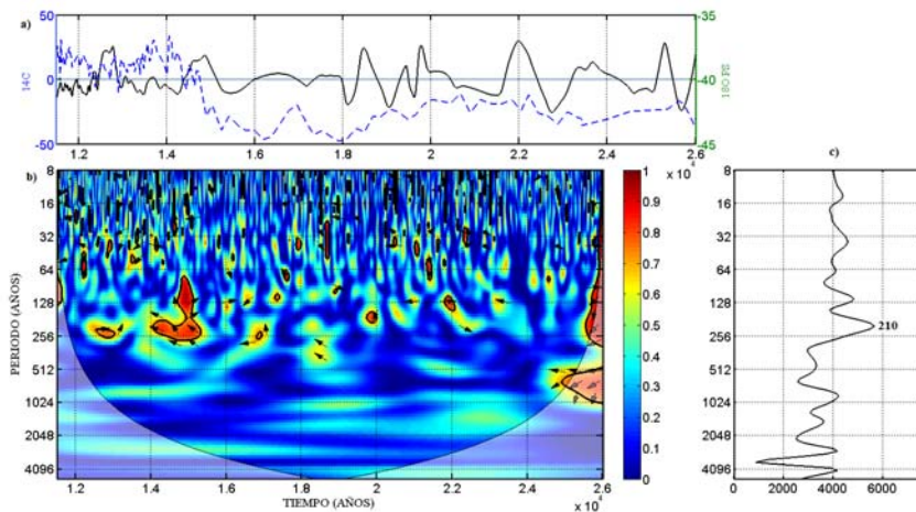
Figura 5.9: Espectro Wavelet de Coherencia entre el carbono-14 e isótopos de oxígeno-18 del polo Sur, a) serie de tiempo del carbono-14 e isótopos de oxígeno-18, b) espectro Wavelet de Coherencia, c) espectro Wavelet Global.
