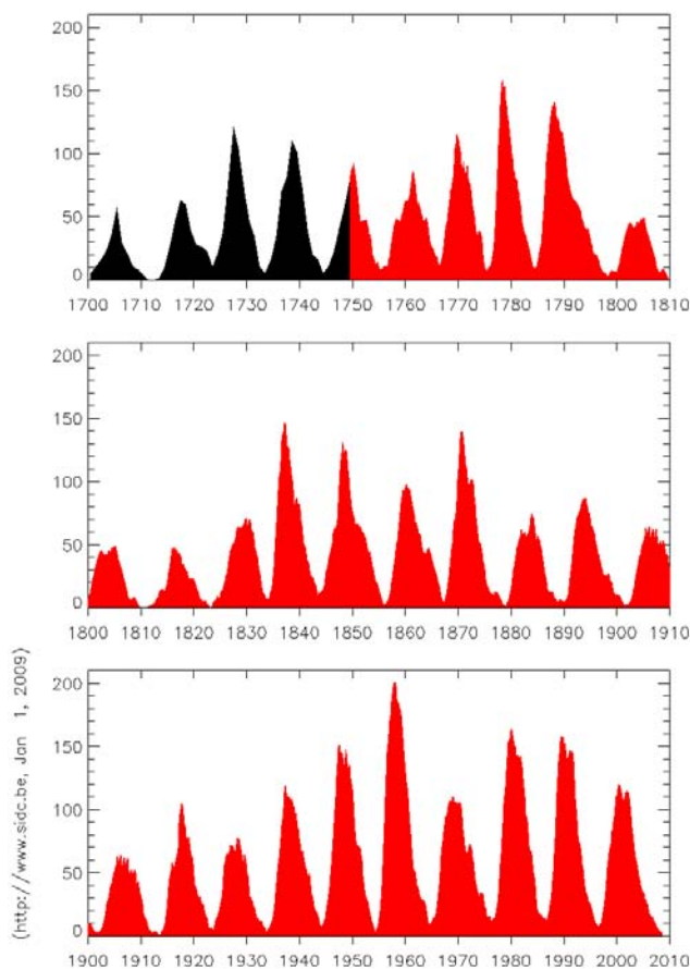
Figura 2.6: Numero de manchas Solares, en negro numero de manchas anuales y en rojo numero de manchas mensuales. (imagen extraída de SIDC Solar Influences Data Analysis Center)
