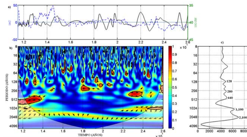
Figura 5.8: Espectro Wavelet de Coherencia entre el carbono-14 e isótopos de oxígeno-18 del polo Norte, a) serie de tiempo del carbono-14 e isótopos de oxígeno-18, b) espectro Wavelet de Coherencia, c) espectro Wavelet Global.
