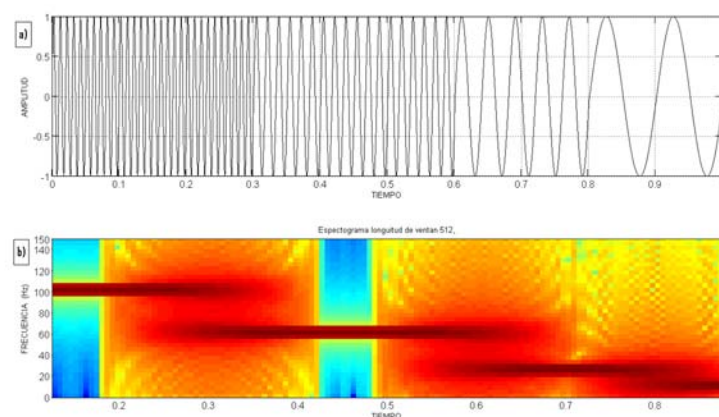
Figura 4.3: a) Señal no estacionaria, b) Espectrograma obtenido mediante la STFT con una ventana Hamming de longitud de 512
