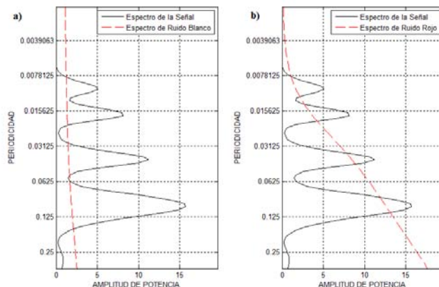
Figura 4.14: Espectro global de Wavelet que contienen al espectro a) de ruido blanco (línea punteada en rojo) y b) ruido rojo (línea punteada en rojo)
