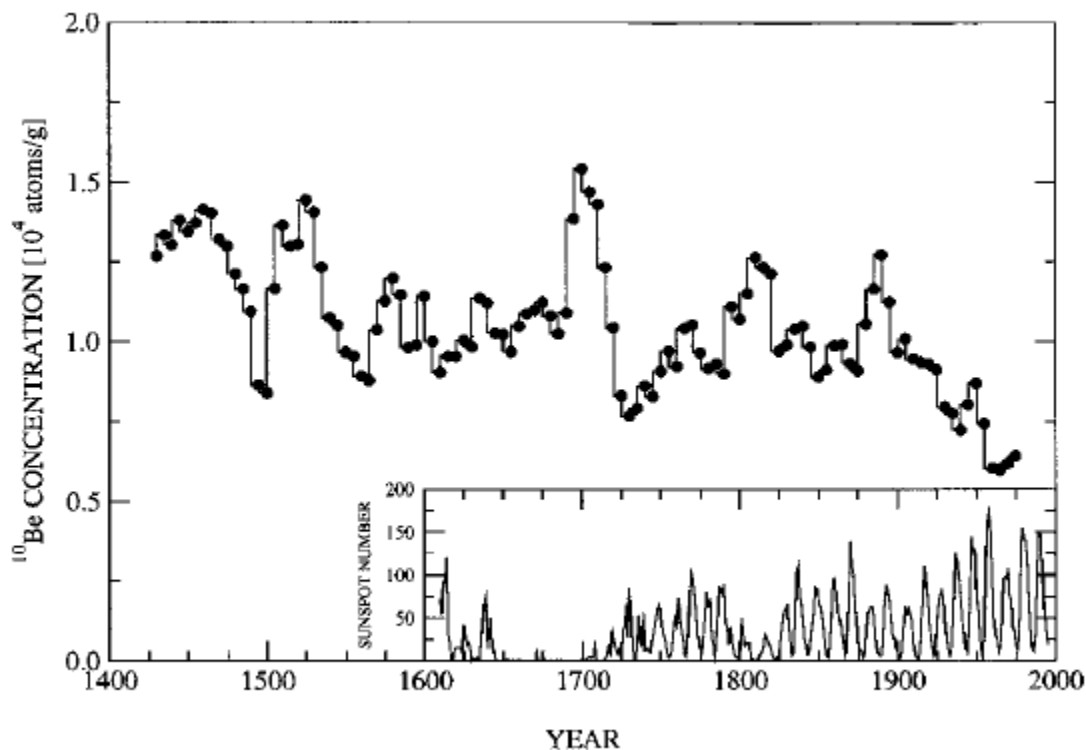
Figura 3.6: Relación entre los isótopos cosmogénicos de ^{10}\text{Be} y la actividad solar, en esta gráfica la actividad solar está representada por el número de manchas solares (extraído de McCracken K. G., et al., 2002)).
