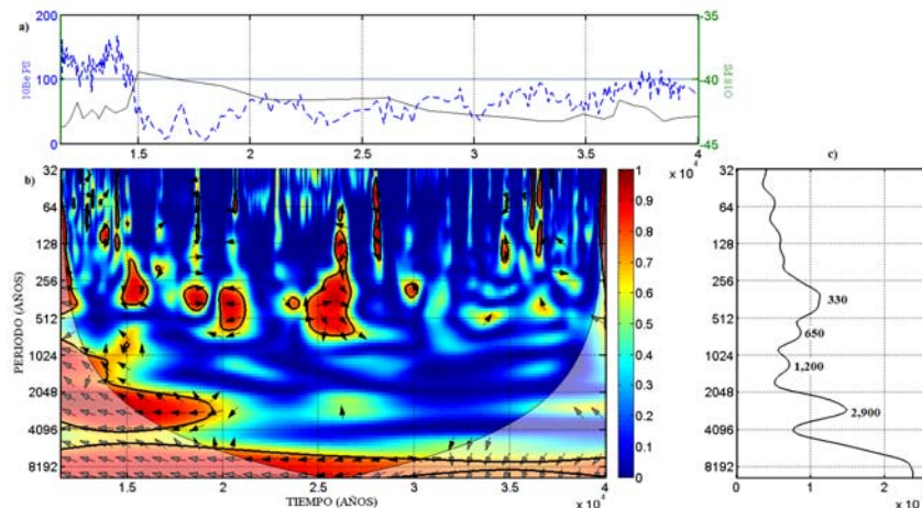
Figura 5.7: Espectro Wavelet de Coherencia entre el Berilio-10 e isótopos de oxígeno-18 del polo Sur, a) serie de tiempo del Berilio-10 e isótopos de oxígeno-18, b) espectro Wavelet de Coherencia, c) espectro Wavelet Global.
