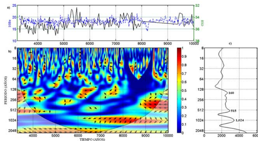
Figura 5.10: Espectro Wavelet de Coherencia entre el berilio-10 e isótopos de oxígeno-18 del polo Norte, a) serie de tiempo del berilio-10 e isótopos de oxígeno-18, b) espectro Wavelet de Coherencia, c) espectro Wavelet Global.
