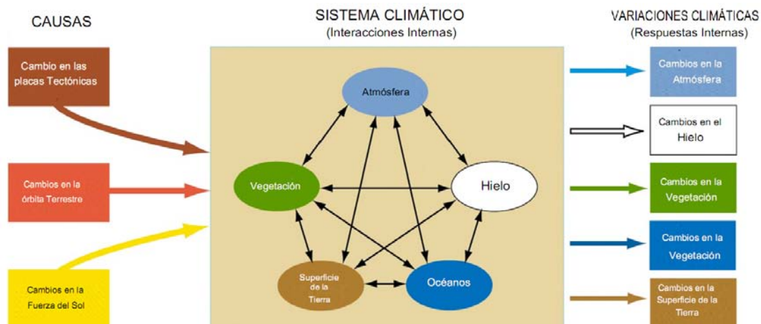
Figura 2.2: Interacciones entre los diferentes componentes existentes en el Sistema climático de la tierra (extraído de Ruddiman, 2002)
