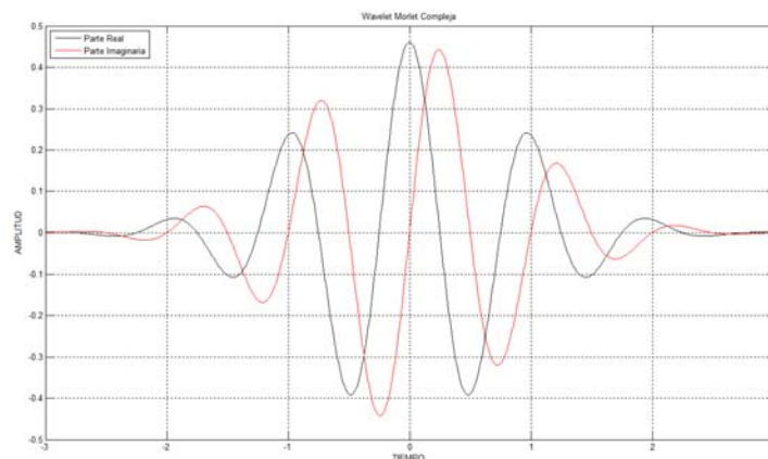
Figura 4.11: Gráfica de la Wavelet Morlet compleja
