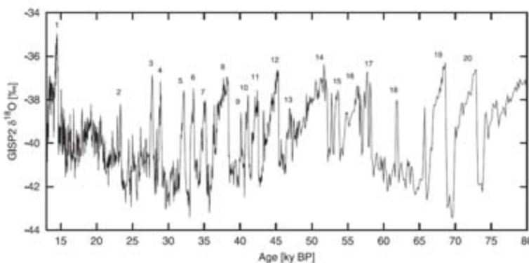
Figura 3.11: Relación isotópica de los \delta^{18}\text{O} en Groenlandia del pozo GISP2. La gráfica muestra las oscilaciones de escala milenaria y enumera en la parte superior los eventos Dansgaard-Oeschger (extraído de Dansgaard, 1993)
