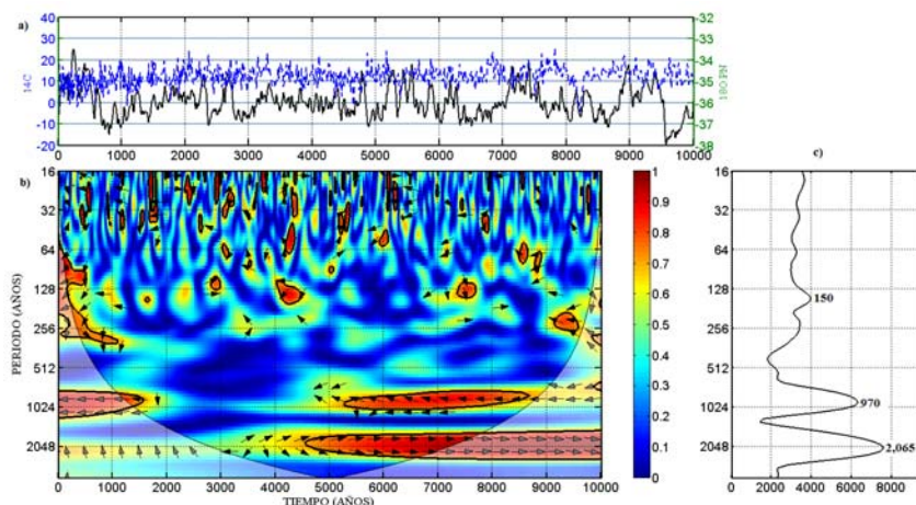
Figura 5.12: Espectro Wavelet de Coherencia entre el carbono-14 e isótopos de oxígeno-18 del polo Norte, a) serie de tiempo del carbono-14 e isótopos de oxígeno-18, b) espectro Wavelet de Coherencia, c) espectro Wavelet Global.
