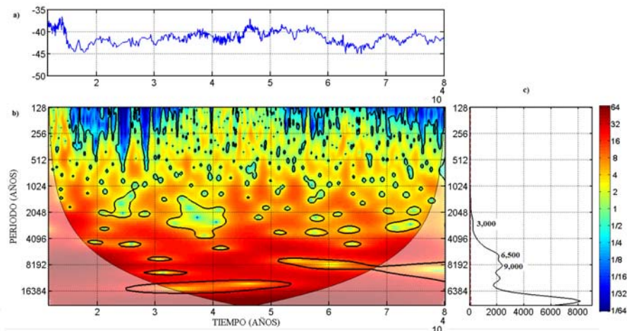
Figura 5.2: Espectro Wavelet de los isótopos de oxígeno-18 del polo Sur, a) serie de tiempo de los isótopos de oxígeno-18, b) espectro Wavelet Morlet, c) espectro Wavelet Global.
