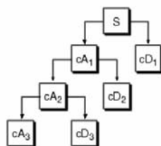
Figura 4.9: Proceso de descomposición múltiple de una señal
