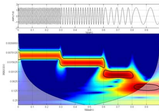
Figura 4.12: Espectro de potencias de Wavelet con frecuencias de 10,25,75,100 Hz
