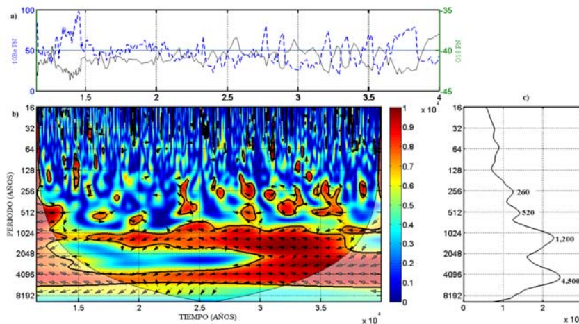
Figura 5.6: Espectro Wavelet de Coherencia entre el Berilio-10 e isótopos de oxígeno-18 del polo Norte, a) serie de tiempo del Berilio-10 e isótopos de oxígeno-18, b) espectro Wavelet de Coherencia, c) espectro Wavelet Global.
