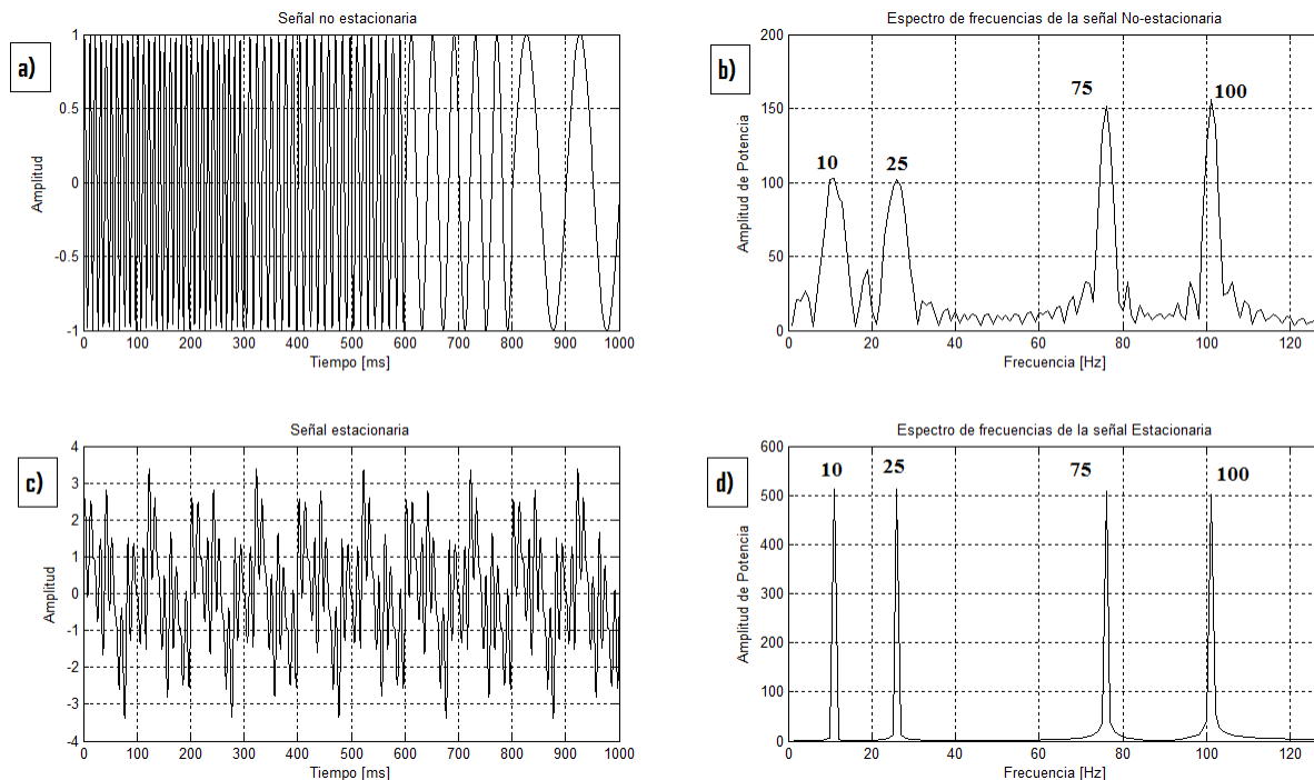
Figura 4.1: a) Señal con diferente contenido de frecuencia y el cual cambia en el tiempo, b) Espectro de la señal Señal con diferente contenido de frecuencia y el cual cambia en el tiempo, c) Señal con diferente contenido de frecuencia , pero la cual esta presente en todo su intervalo de tiempo, d) Espectro de la señal con contenido de frecuencia diferente , pero la cual esta presente en todo su intervalo de tiempo
