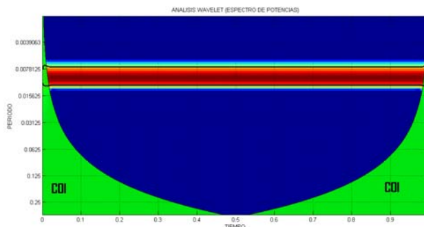
Figura 4.13: Espectro de potencias Wavelet donde se señala el COI en color verde
