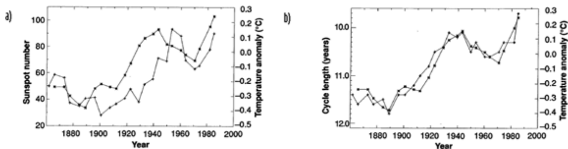
Figura 2.9: a) Anomalías de temperaturas del hemisferio norte (*) y valores medios del número de manchas solares (+). b) Anomalías de temperaturas del hemisferio norte (*) y variación en la duración del ciclo de manchas solares (+) (extraído de Friis, 1991).
