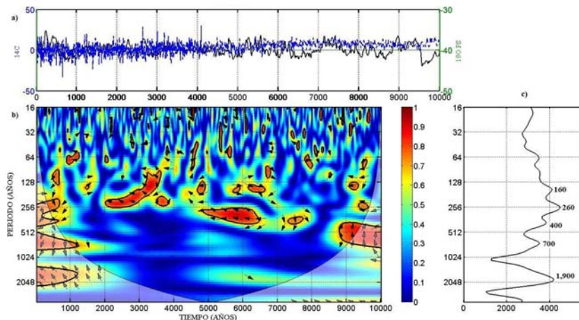
Figura 5.13: Espectro Wavelet de Coherencia entre el carbono-14 e isótopos de oxígeno-18 del polo Sur, a) serie de tiempo del carbono-14 e isótopos de oxígeno-18, b) espectro Wavelet de Coherencia, c) espectro Wavelet Global.
