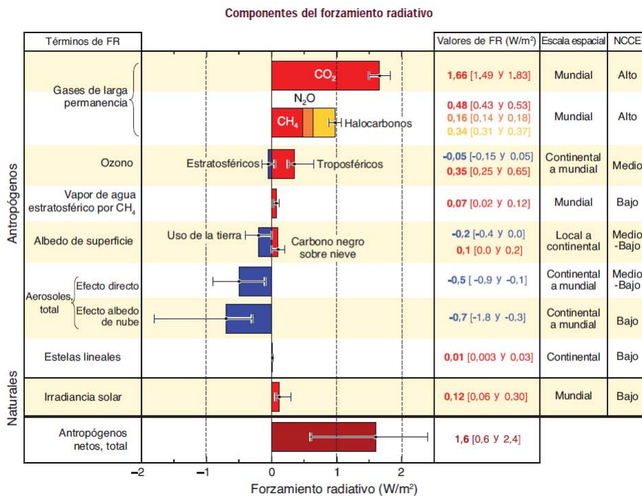
Figura 2.7: Gráfico del forzamiento radiativo y su respectivo nivel de conocimiento (extraído del reporte del IPCC, 2007)
