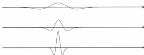
Figura 4.5: Imagen que muestra el concepto de escalamiento de una Wavelet (Extraída de Paul S, 2002)
