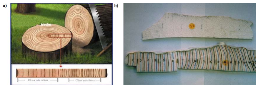
Figura 3.1: a) Imagen que muestra los anillos contenidos en un árbol. (Extraída de www.seed.slb.com/ ), b) Segmento de un núcleo de coral obtenido de Urvina Bay, Galápagos. Las líneas negras representan las bandas anuales, las líneas blancas, azules y rojas el año dividido en cuartos.
