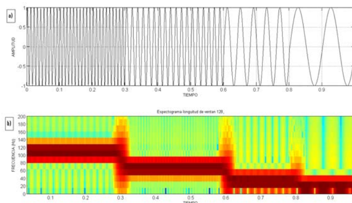
Figura 4.2: a) Señal no estacionaria, b) Espectrograma obtenido mediante la STFT con una ventana Hamming de longitud de 128
