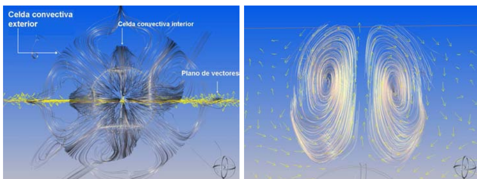
(a) Vista superior de una celda convectiva. (b) Vórtices de la celda convectiva interior.
