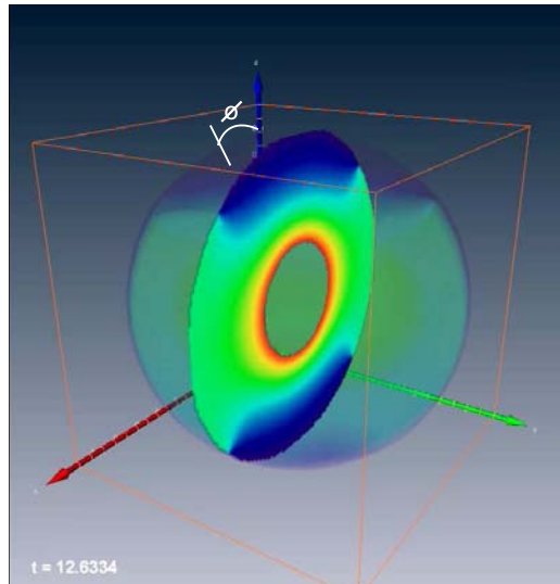
Figura 4.8: Distribución de temperaturas en el estado estacionario t > 12.6 (s).
