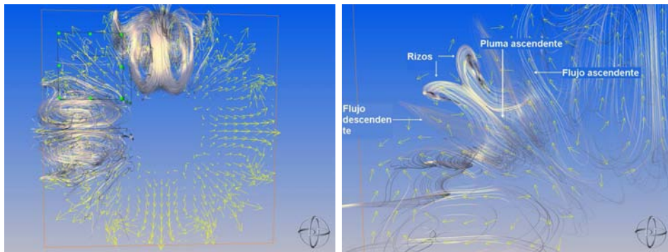
(a) Plano de flujo ascendente. (b) Región de flujo entre dos celdas convectivas.
