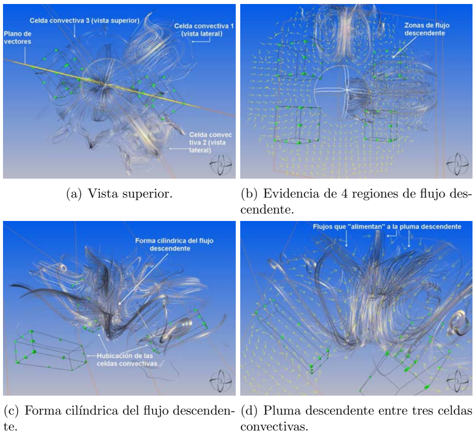
Figura 5.8: Región de flujo entre tres celdas convectivas.
