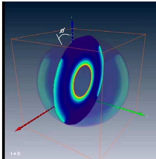
Figura 4.6: Distribución de temperaturas al inicio de los cálculos t = 0(s) .
