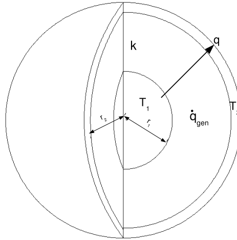
Figura 2.3: Esquema del proceso de conducción de calor con generación de energía térmica \dot{q}_{gen} por unidad de volumen.
