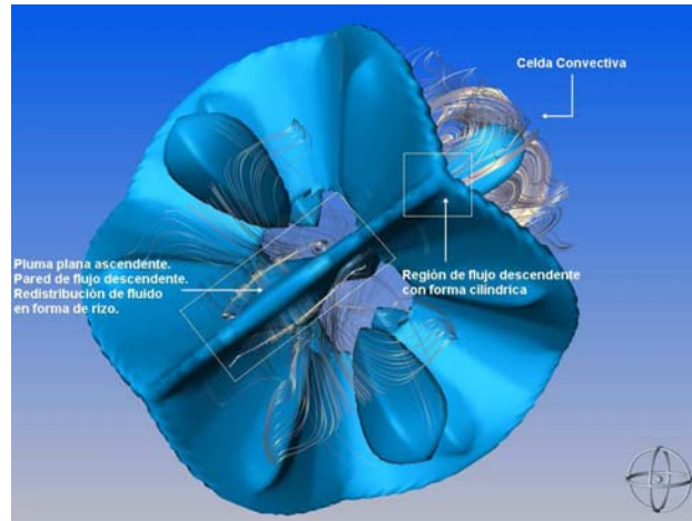
(a) Mapa general del flujo.
