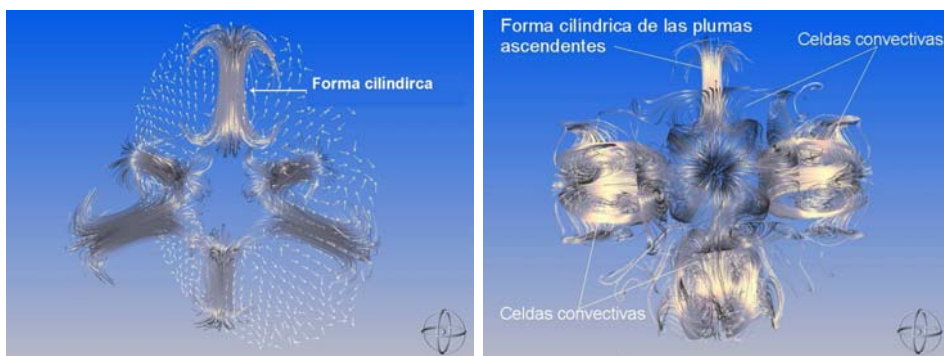
(a) Hubicación simétrica de las plumas ascendentes con forma cilíndrica (b) Pluma ascendente y celdas convectivas.
