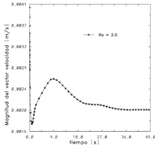
Figura 5.1: Magnitud del vector velocidad. A partir de t = 35(s) se alcanza el estado estacionario.
