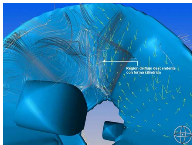
(c) Flujo cilíndrico descendente en la intersección de tres paredes de flujo.
