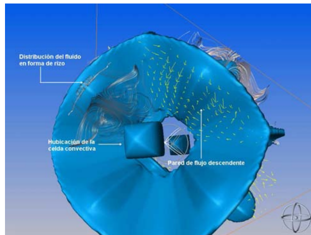
(b) Paredes de flujo descendente, con una pluma aplana-da de flujoascendente en el centro.
