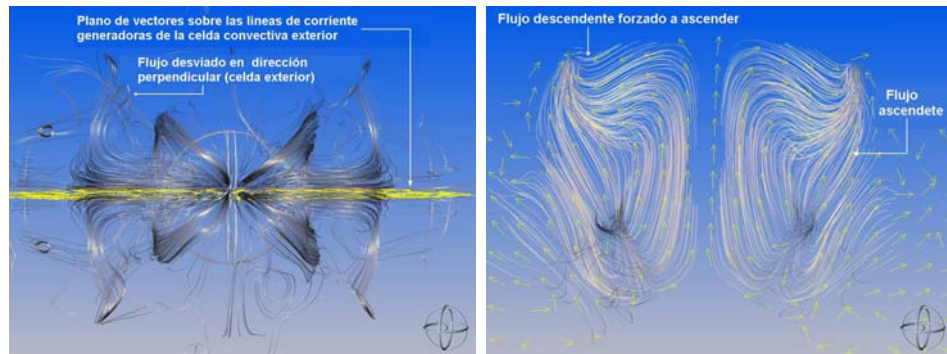
(a) Flujo desviado perpendicularmente de su dirección original de ascenso. (b) Plano de flujo totalmente ascendente.
