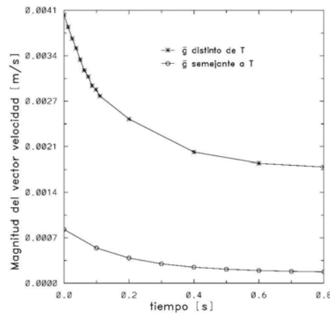
Figura 5.2: Magnitud de la velocidad con Ra = 3 .
