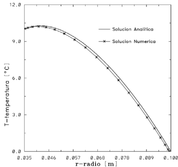
Figura 4.5: Solución analítica y solución numérica del problema de conducción de calor en esferas concéntricas con generación volumétrica de calor en estado permanente t > 0.1 \times 10^{-1} (s).
