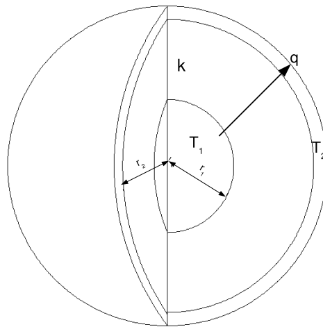
Figura 2.2: Modelo para el análisis de conducción en el sistema esférico por capas, con ánulo esférico sólido con conductividad térmica k y transferencia calor por conducción q .
