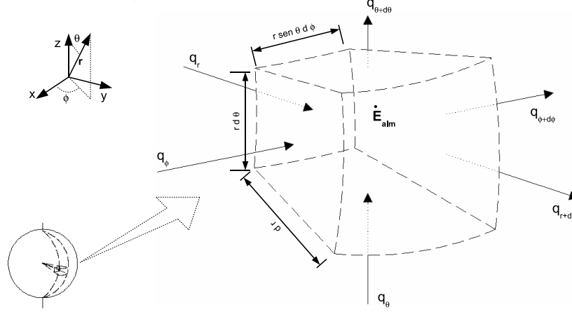
Figura A.1: Volumen de control diferencial, (dr, rd\theta, r\text{sen}(\theta)d\phi) , para el análisis de conducción en coordenadas esféricas (r, \theta, \phi)
