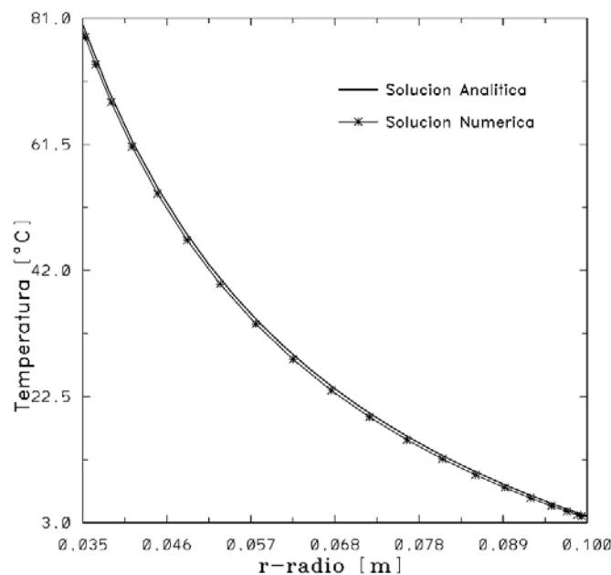
Figura 4.3: Solución analítica y solución numérica del problema de difusión de calor en esferas concéntricas; la temperatura de la esfera interna es de 80 °C y la externa de 4 °C.
