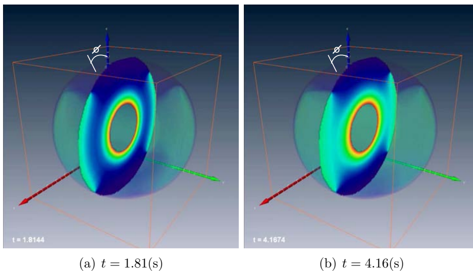
Figura 4.7: Distribución de temperaturas en el estado transitorio.
