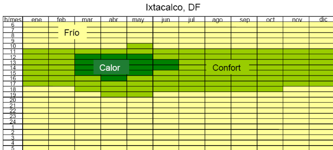
Figura 5.8.2. Diagrama de isorequerimientos para Iztacalco, DF (Fuente: Morillón, D. Atlas del bioclima de México, II UNAM)
