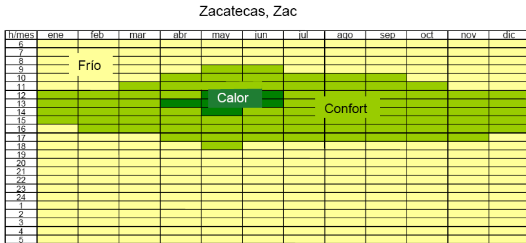
Figura 5.43. Diagrama de isorequerimientos para Zacatecas (Fuente: Morillón, D. Atlas del bioclima de México, II UNAM)
