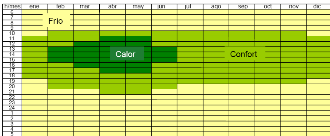
Figura 5.13. Diagrama de isorequerimientos para Cuernavaca (Fuente: Morillón, D. Atlas del bioclima de México, II UNAM)
