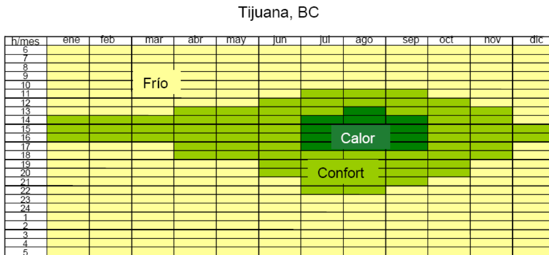
Figura 5.35. Diagrama de isorequerimientos para Tijuana (Fuente: Morillón, D. Atlas del bioclima de México, II UNAM)
