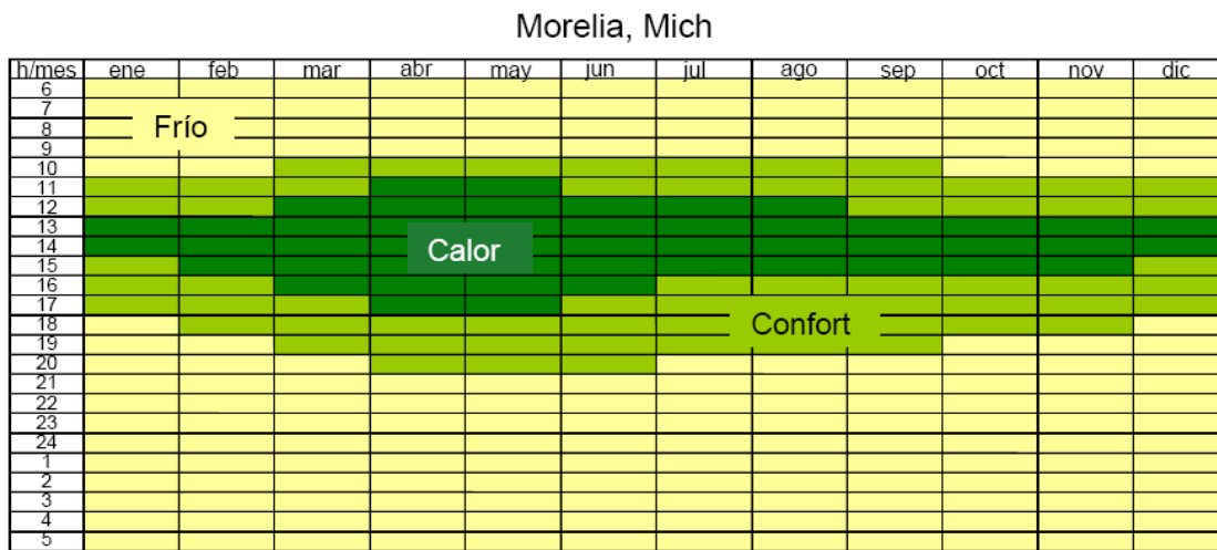
Figura 5.26. Diagrama de isorequerimientos para Morelia (Fuente: Morillón, D. Atlas del bioclima de México, II UNAM)
