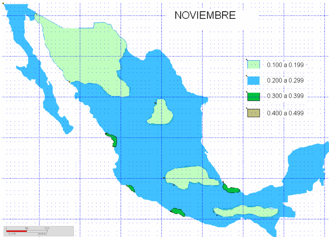
Figura 4.1.1.11. Factores de ahorro de aire acondicionado para noviembre
