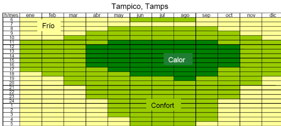
Figura 5.33. Diagrama de isorequerimientos para Tampico (Fuente: Morillón, D. Atlas del bioclima de México, II UNAM)
