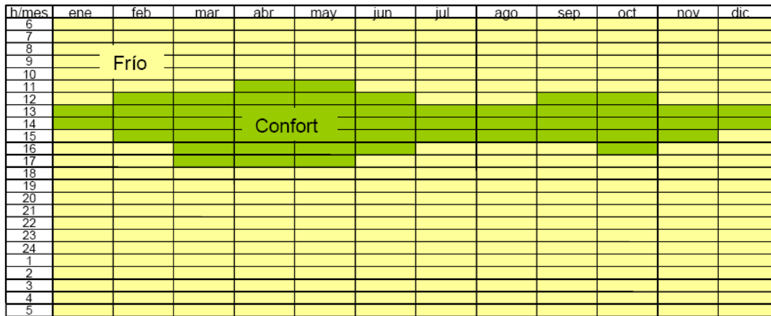
Figura 5.37. Diagrama de isorequerimientos para Toluca (Fuente: Morillón, D. Atlas del bioclima de México, II UNAM)
