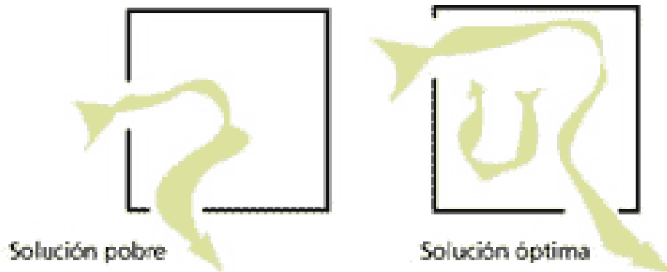
Figura 2.1.2.5. Aberturas ubicadas en paredes adyacentes
