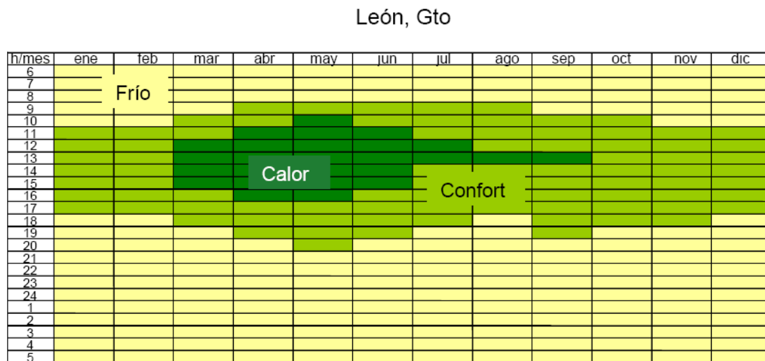
Figura 5.20. Diagrama de isorequerimientos para León (Fuente: Morillón, D. Atlas del bioclima de México, II UNAM)
