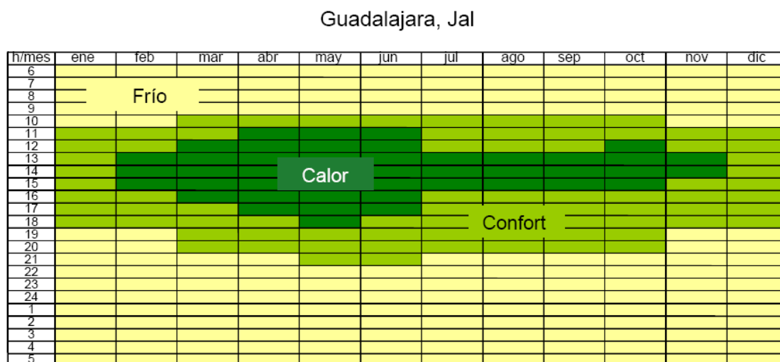
Figura 5.16. Diagrama de isorequerimientos para Guadalajara (Fuente: Morillón, D. Atlas del bioclima de México, II UNAM)
