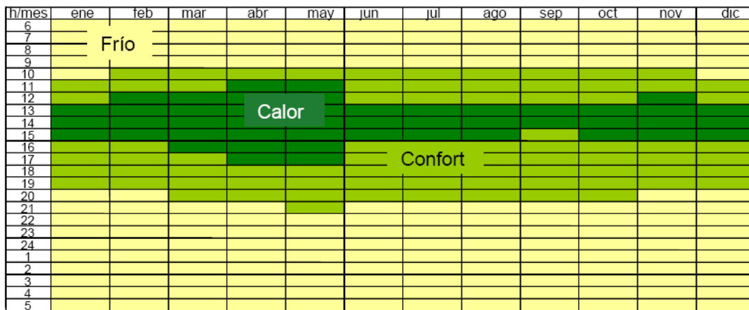
Figura 5.7. Diagrama de isorequerimientos para Chilpancingo (Fuente: Morillón, D. Atlas del bioclima de México, II UNAM)
