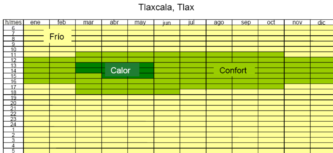
Figura 5.36. Diagrama de isorequerimientos para Tlaxcala (Fuente: Morillón, D. Atlas del bioclima de México, II UNAM)
