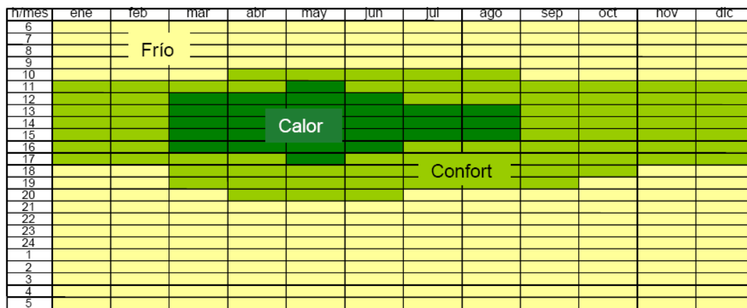
Figura 5.30. Diagrama de isorequerimientos para Querétaro (Fuente: Morillón, D. Atlas del bioclima de México, II UNAM)
