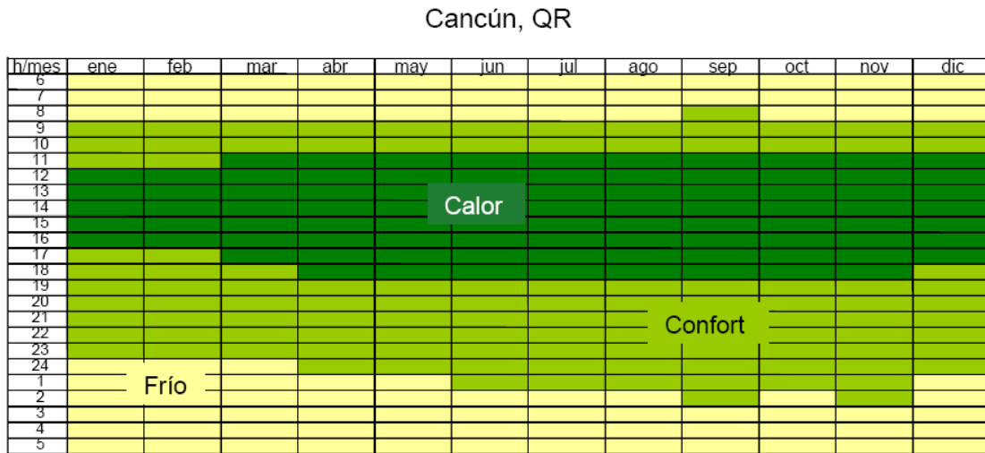
Figura 5.4. Diagrama de isorequerimientos para Cancún (Fuente: Morillón, D. Atlas del bioclima de México, II UNAM)
