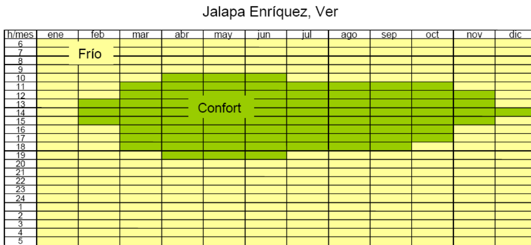
Figura 5.42. Diagrama de isorequerimientos para Xalapa (Fuente: Morillón, D. Atlas del bioclima de México, II UNAM)
