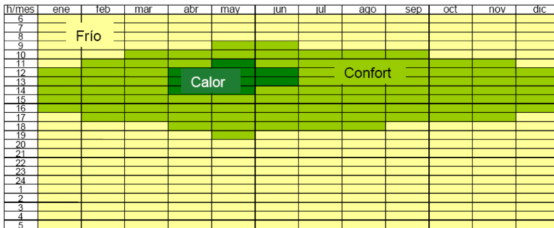
Figura 5.17. Diagrama de isorequerimientos para Guanajuato (Fuente: Morillón, D. Atlas del bioclima de México, II UNAM)
