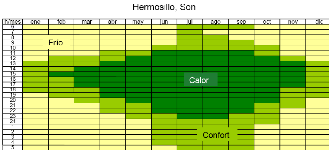
Figura 5.18. Diagrama de isorequerimientos para Hermosillo (Fuente: Morillón, D. Atlas del bioclima de México, II UNAM)
