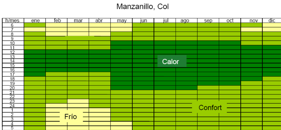
Figura 5.21. Diagrama de isorequerimientos para Manzanillo (Fuente: Morillón, D. Atlas del bioclima de México, II UNAM)
