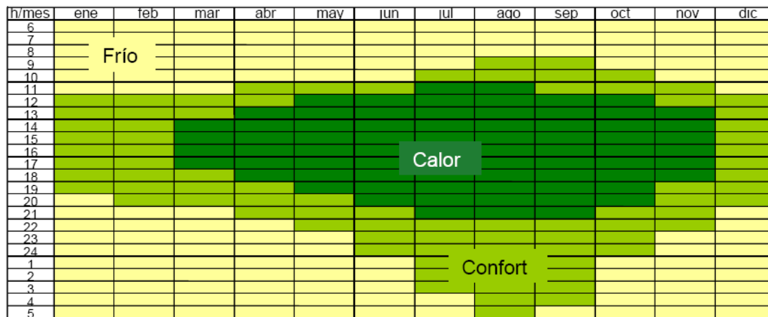
Figura 5.19. Diagrama de isorequerimientos para La Paz (Fuente: Morillón, D. Atlas del bioclima de México, II UNAM)
