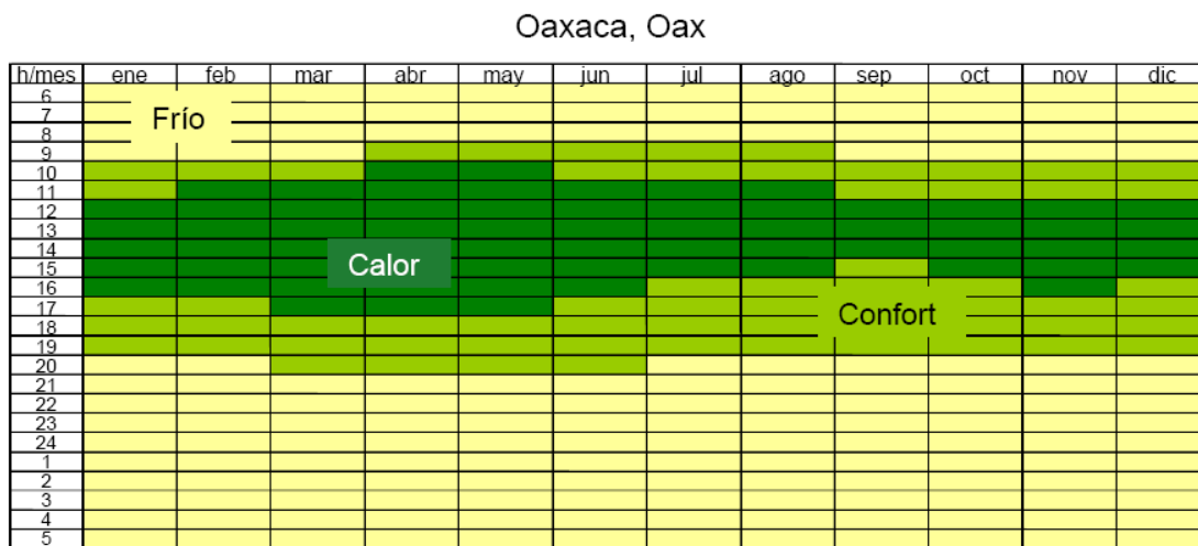
Figura 5.27. Diagrama de isorequerimientos para Oaxaca (Fuente: Morillón, D. Atlas del bioclima de México, II UNAM)
