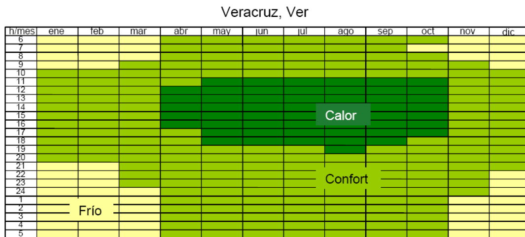
Figura 5.40. Diagrama de isorequerimientos para Veracruz (Fuente: Morillón, D. Atlas del bioclima de México, II UNAM)
