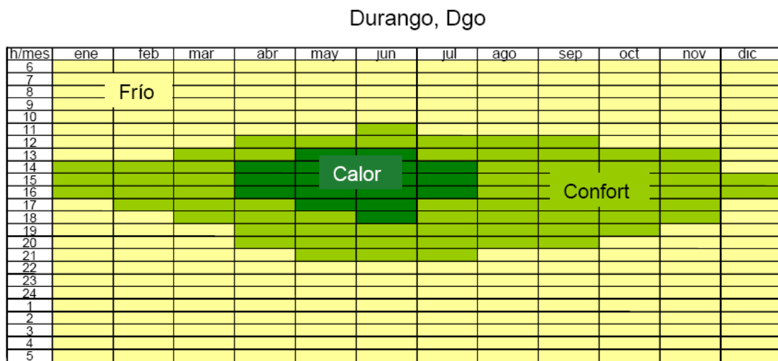
Figura 5.15. Diagrama de isorequerimientos para Durango (Fuente: Morillón, D. Atlas del bioclima de México, II UNAM)
