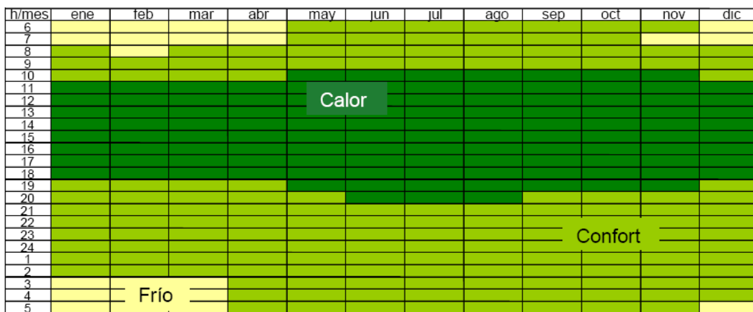
Figura 5.1. Diagrama de isorequerimientos para Acapulco (Fuente: Morillón, D. Atlas del bioclima de México, II UNAM)
