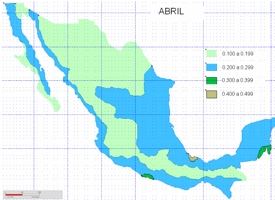
Figura 4.1.1.4. Factores de ahorro de aire acondicionado para abril
