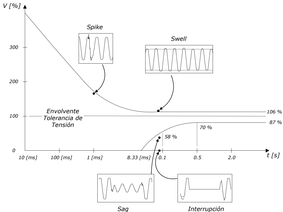
Curva CBEMA
