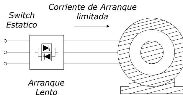
Arrancador a tensión reducida
