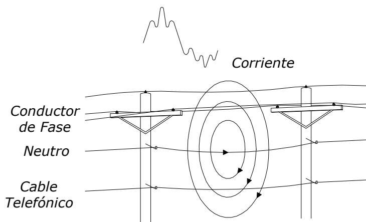
Tensiones inducidas en los circuitos de telefonía
