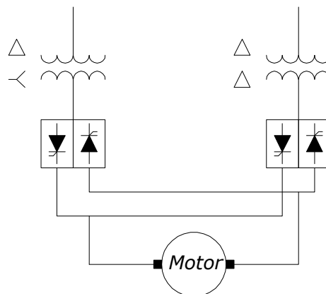
Convertidor de 12 pulsos
