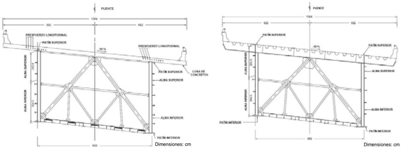
a) Sección transversal con piso de concreto
