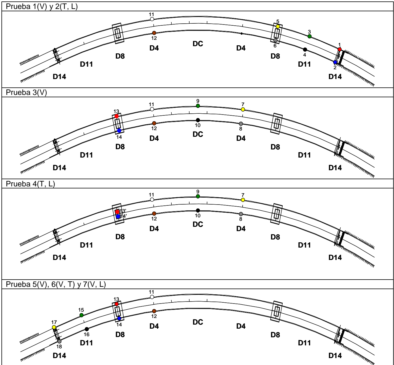
Figura 27 Programa de pruebas, vibración ambiental: primera etapa, agosto del 2006
