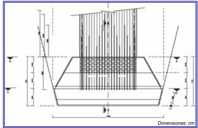
VISTA PLANTA
