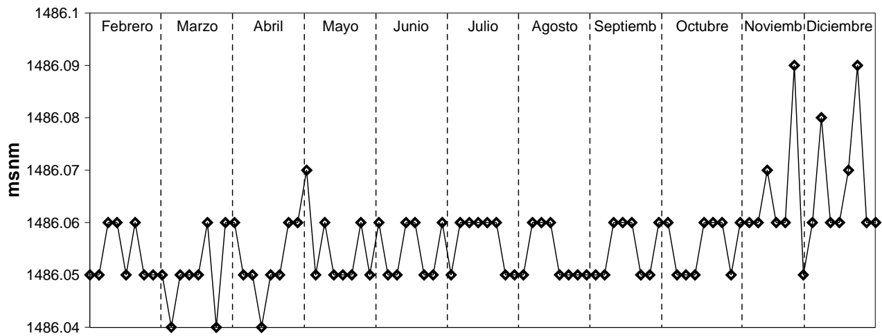
Figura G7 Registro topográfico en elevación correspondientes al punto D7-D8E de la superestructura del puente San Cristóbal (año 2007)
