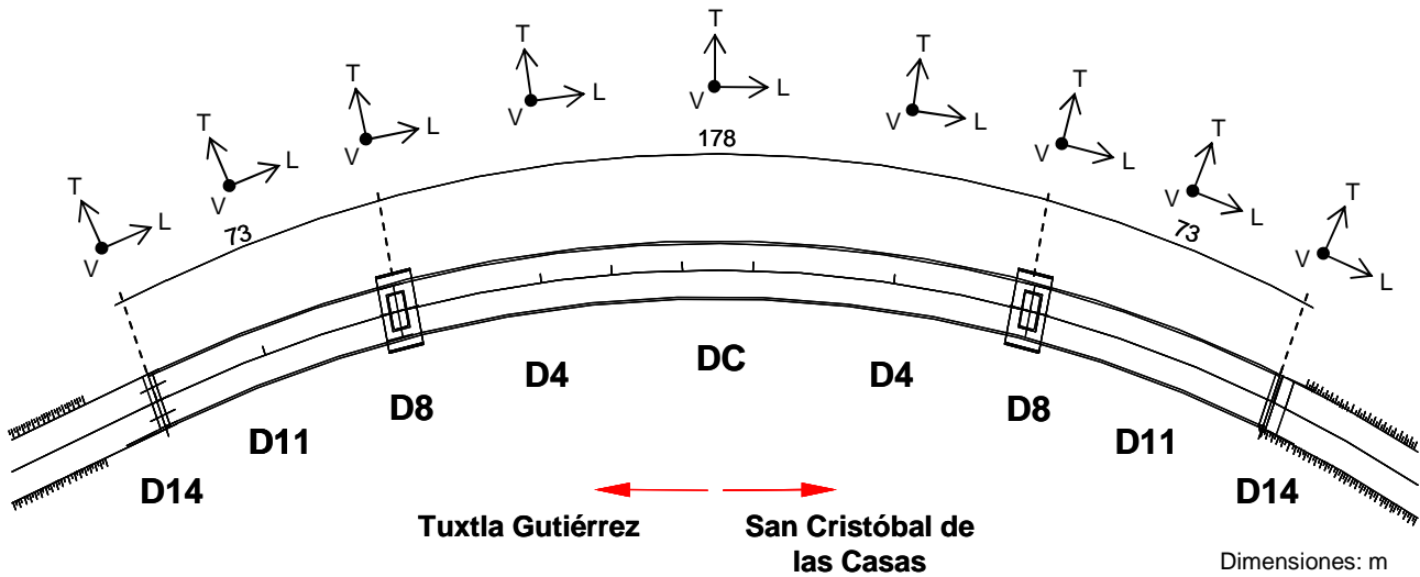
Figura 11 Ubicación de las dovelas instrumentadas del puente San Cristóbal (vista en planta)
