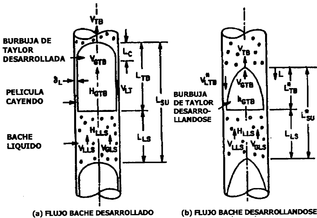
Fig. 2 Diagrama Flujo Bache
