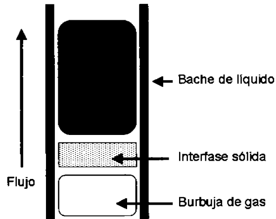
Figura 3.1. Operación ideal de una burbuja de gas en un sistema de bombeo neumático.
