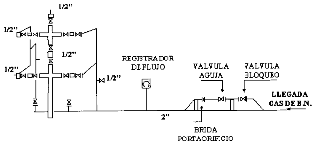
Diagrama típico para la inyección de gas de B.N. en pozos
