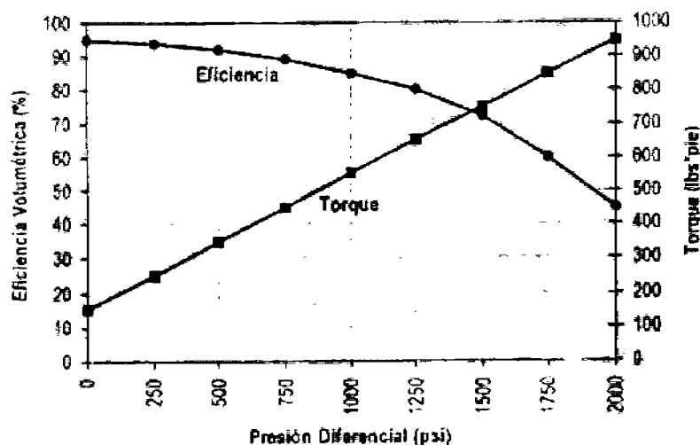
Figura 1.3. Curva típica de comportamiento de una bomba BCP obtenida del banco de pruebas 2
