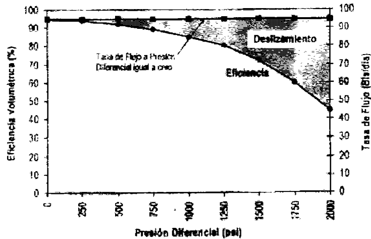
Figura 1.4. Efecto de deslizamiento sobre la eficiencia volumétrica de la bomba 2
