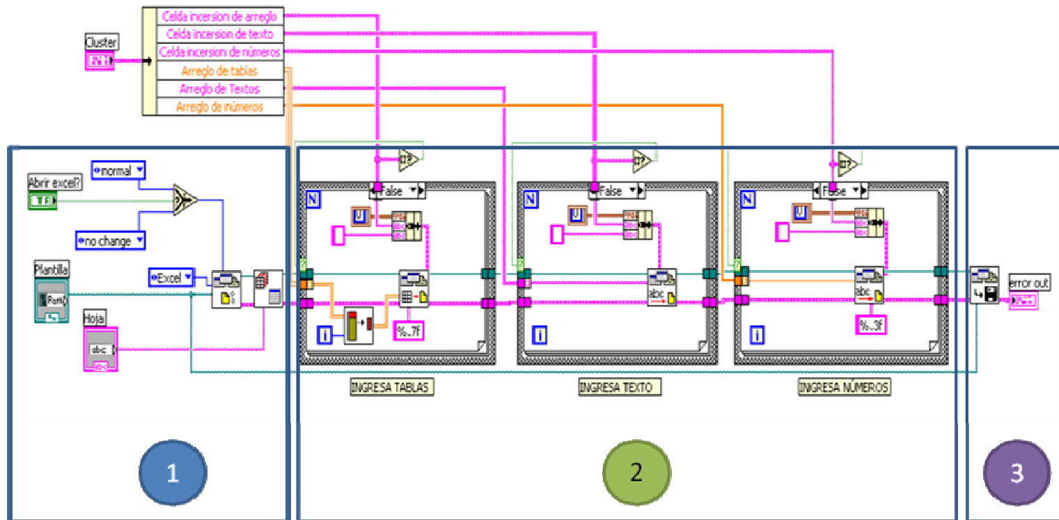
Figura 2.32.Código del VI Excel.
