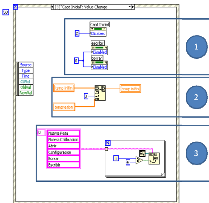
Figura 2.20. Código de inicia calibración.
