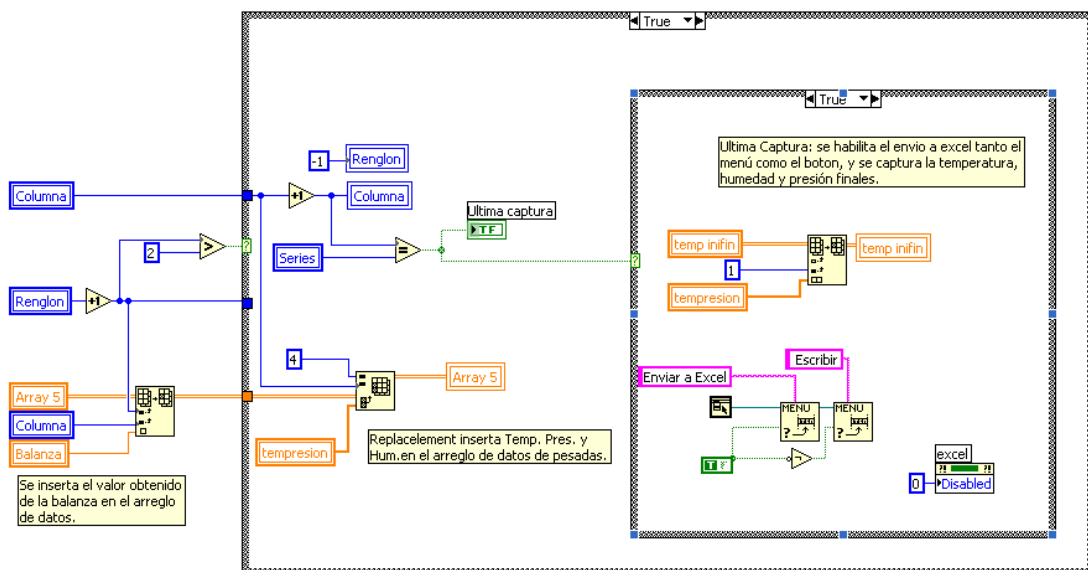
Figura 1.6. Diagrama de bloques.
