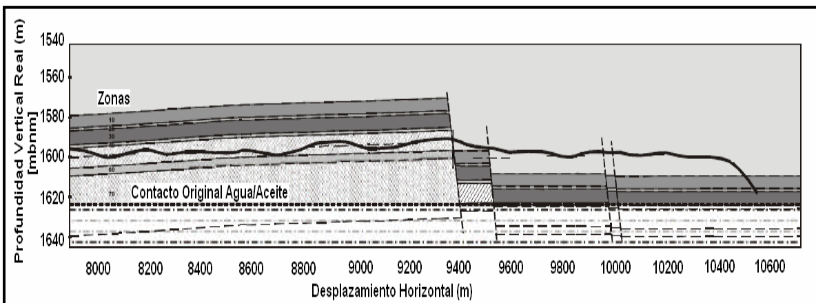
Figura 3.5. Sección Final del Pozo M-16Z en el agujero de 8 1/2”.
