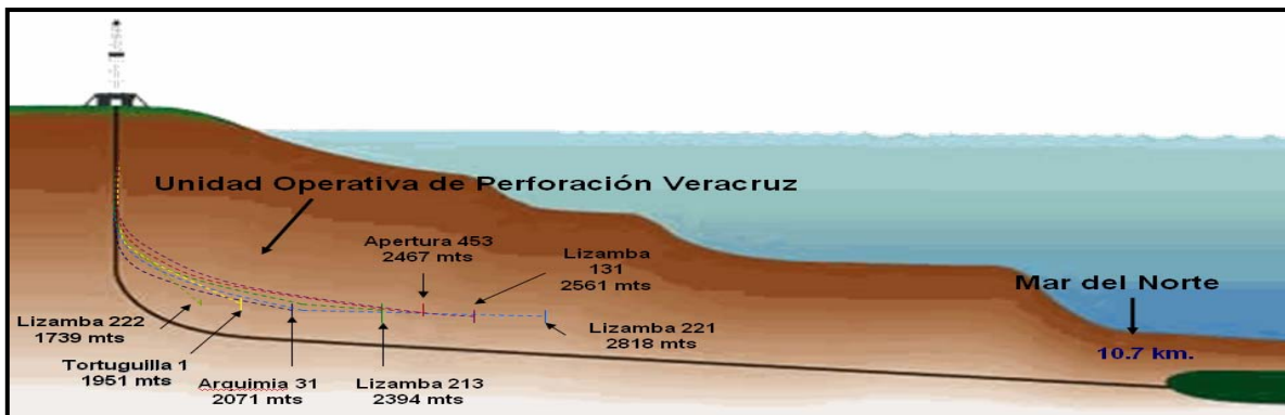
Figura 2.2. Representación esquemática de los alcances de pozos en Veracruz.
