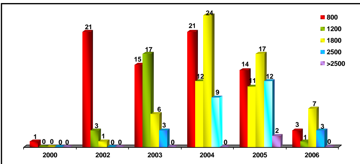
Figura 1.8. Desplazamiento de los pozos en el Activo Integral Veracruz.
