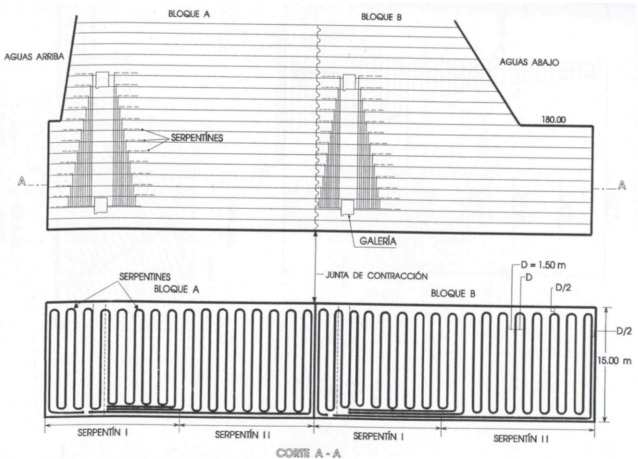
Figura 5.1 Ejemplo de las características de los serpentines y su disposición típica en la Presa Huites
