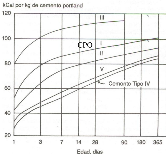
Fig. 4.2 Curvas típicas de calor de hidratación para diversos tipos de cemento
