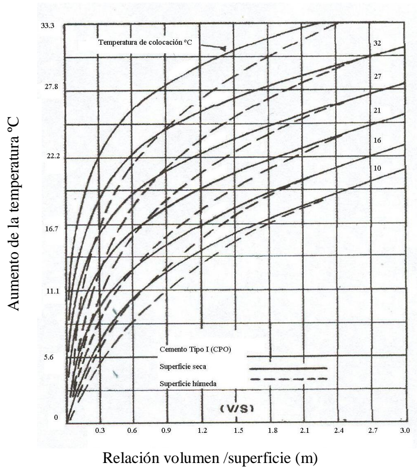
Fig. 4.3 Aumento de la temperatura del concreto para diversas temperaturas de colocación 223 kg/m 3 de cemento Difusividad 0.0046 m/hora Temperatura de colocación igual a la del aire ACI 207.2R 95
