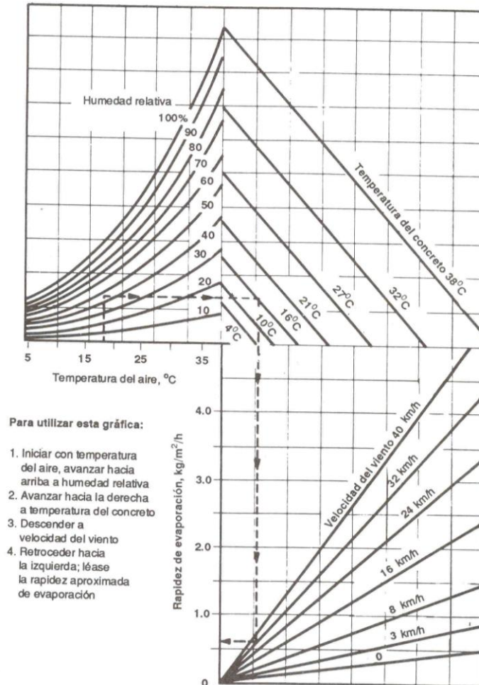
Fig. 4.1 Efecto de la temperatura del concreto y las condiciones ambientales en la rapidez de evaporación de la humedad superficial del concreto
