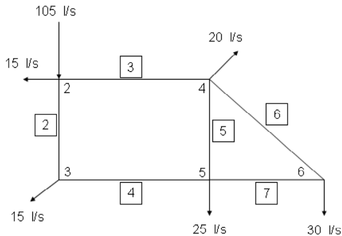
Figura 1-2: Red de tuberías. Disposición de tubos y nudos. Gastos de entrada y salida.
