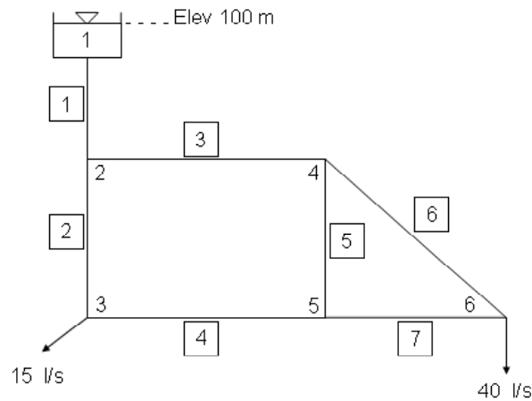
Figura 1-5: Red de tuberías. Disposición de tubos y nudos. Gastos de salida.
