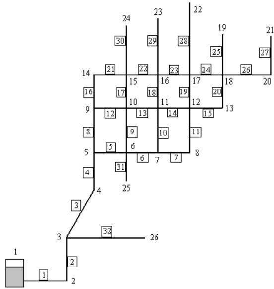
Figura 4-3: Red de tuberías para rehabilitación en ejemplo segundo.
