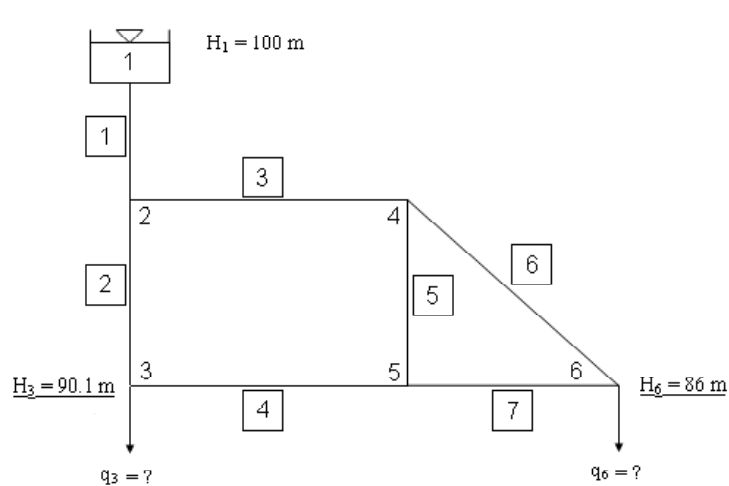
Figura 1-3: Red de tuberías. Disposición de tubos y nudos. Cargas piezométricas conocidas.
