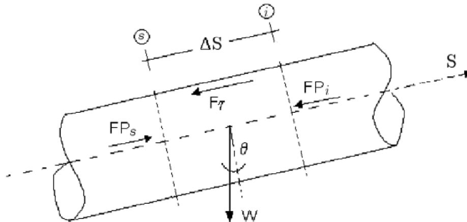
Figura 1-1: Flujo desarrollado entre dos secciones de una vena líquida.
