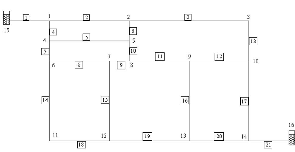
Figura 4-1: Red de tuberías para rehabilitación en ejemplo primero.
