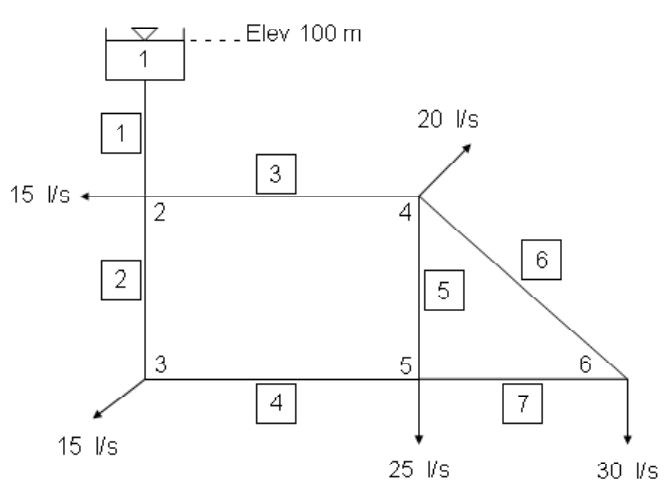
Figura 1-4: Red de tuberías. Disposición de tubos y nudos. Gastos de salida.
