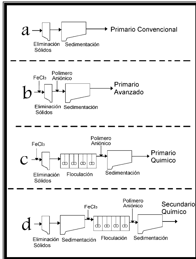
Figura 2.1. CONFIGURACIONES BÁSICAS DEL TRATAMIENTO PRIMARIO (Fuente: Shao et al., 1996)
