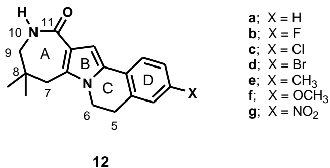
Figura 6. Estructura de las diazanaftoazulenonas 12a-g .
