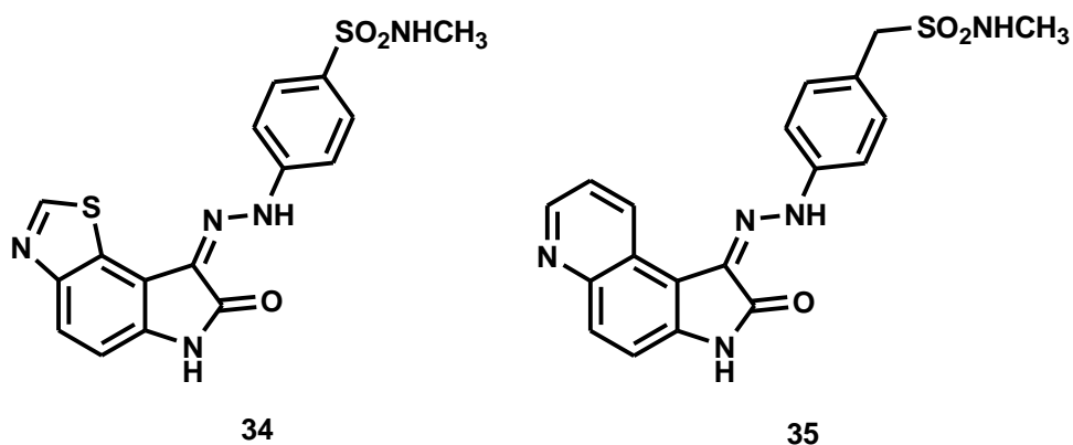
Figura 16. Oxindoles GW9499 34 y GW5181 35 .
