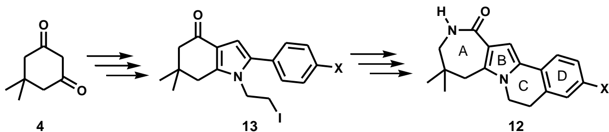
Esquema 2. Secuencia de síntesis para obtener las diazanaftoazulenonas 12a-g .
