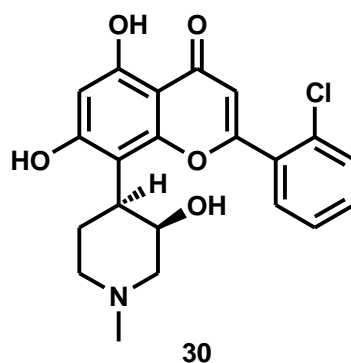
Figura 14. Inhibidor de las CDKs más avanzado, Flavopiridol 30 .
