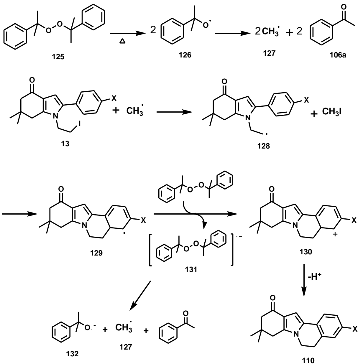
Esquema 34. Propuesta del mecanismo de reacción de la ciclación radical oxidativa.
