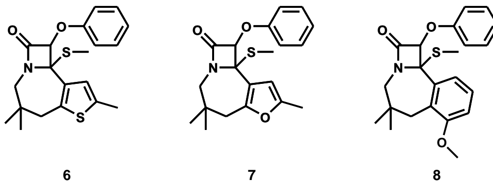
Figura 4. Modificaciones bioisostéricas de la molécula líder 5 .
