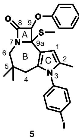
Figura 3. Estructura de la azetopirroloazepinona 5 .
