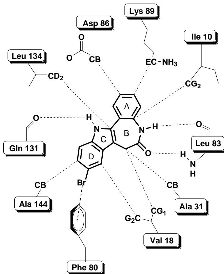
Figura 2. Posibles interacciones entre kenpaullona y CDK2.
