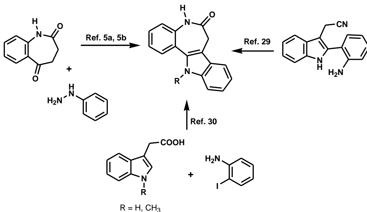
Esquema 3. Resumen de algunos métodos de síntesis de paullonas.
