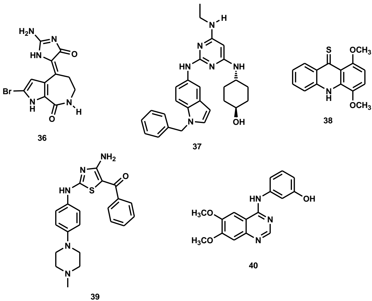
Figura 17. Inhibidores de CDK2 y CDK4.
