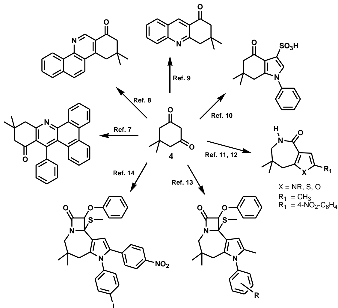
Esquema 1. Compuestos heterocíclicos sintetizados a partir de dimedona 4 .
