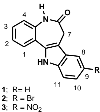
Figura 1. Estructura de la paullona 1 , la kenpaullona 2 y la alsterpaullona 3 .
