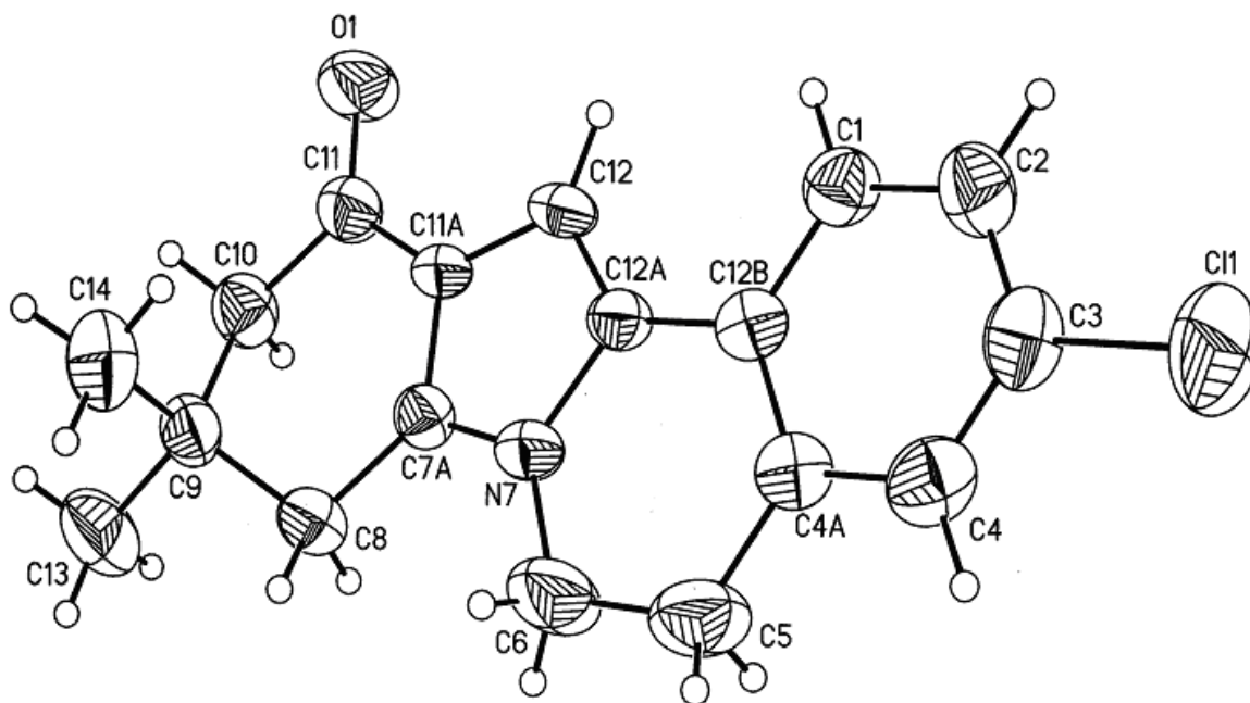
Figura 19. Representación ORTEP del compuesto 110c .
