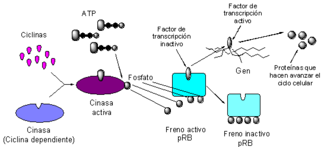
Figura 12. Mecanismo de acción de las CDKs
