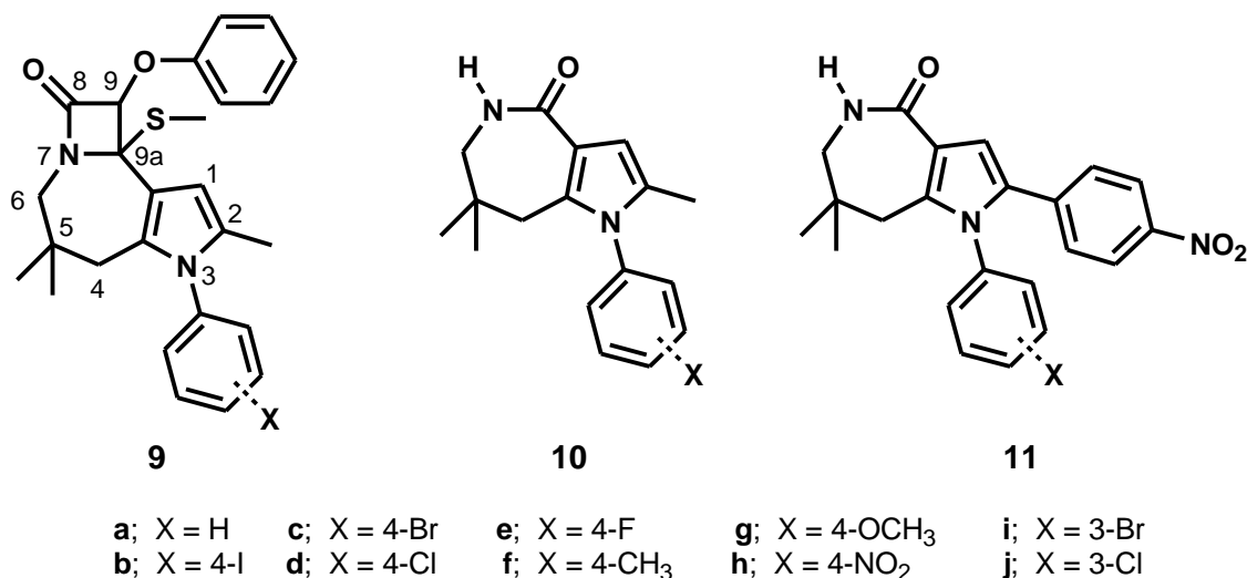
Figura 5. Series de compuestos que se generaron por las modificaciones estructurales de 5.
