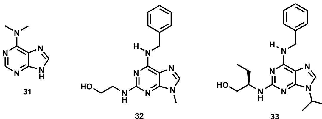
Figura 15. Purinas que actúan como inhibidores de CDKs.
