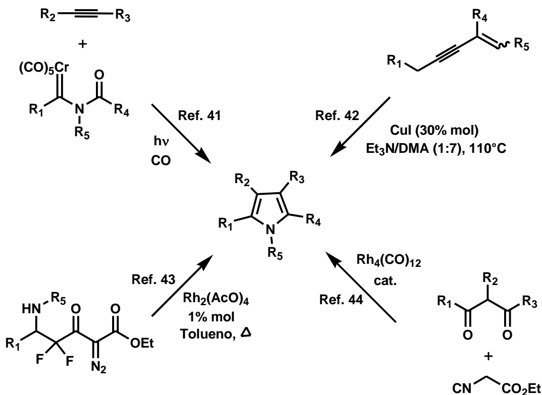
Esquema 17. Otro métodos de obtención de pirroles.
