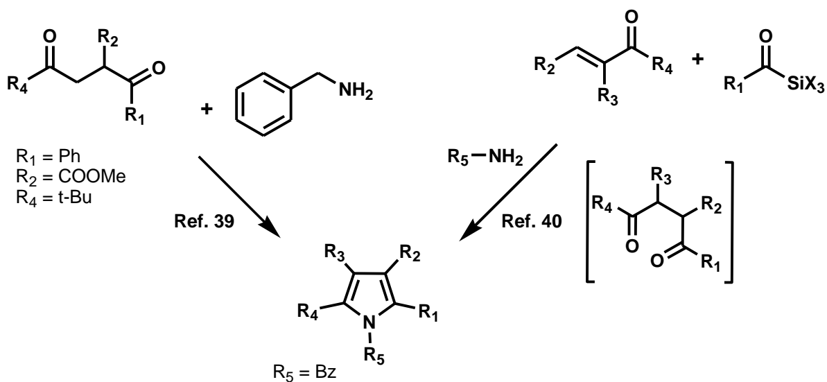
Esquema 14. Algunos métodos de síntesis de Paal-Knorr.
