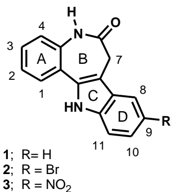
Figura 18. Estructura de las paullonas.
