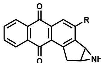
18 R = OCH 2 CH 2 N(CH 2 CH 2 Cl) 2
