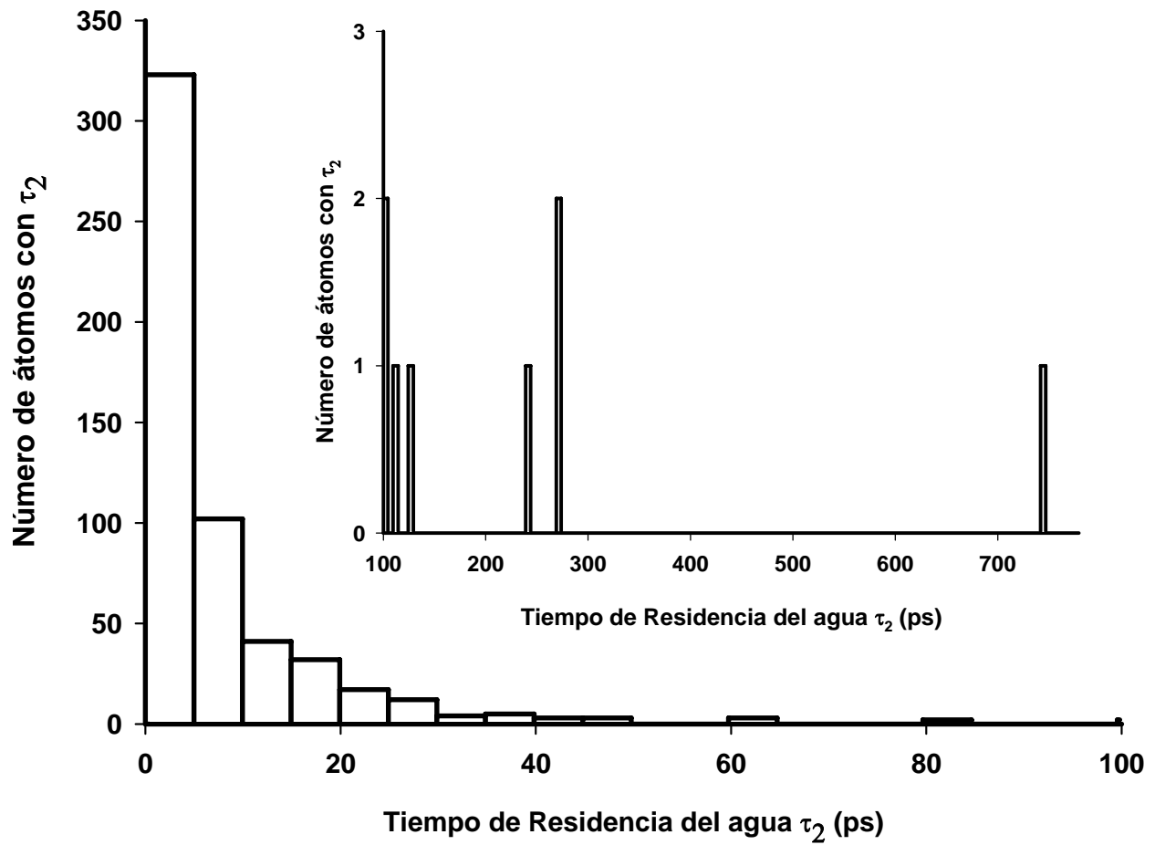
Figura 4.4. Distribución de los tiempos residencia de las moléculas de agua dentro de la primera esfera de solvatación de la proteína tendamistat, sin considerar los átomos de hidrógeno y teniendo en cuenta \tau_2 de decaimiento.
