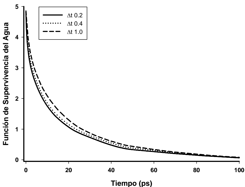
Figura 3.5. Función de supervivencia vs tiempo de residencia del agua en la esfera de solvatación del átomo de N de la cadena principal del aminoácido Gly1 de la FKBP12, a diferentes \Delta t . Línea continua \Delta t = 0.2 ps, línea punteada \Delta t = 0.4 ps y línea discontinua \Delta t = 1.0 ps.
