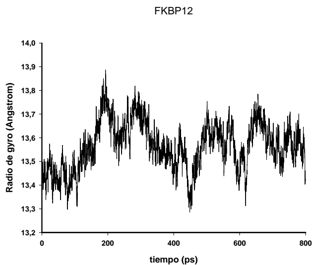
Figura 3.4. Radio de giro vs tiempo. En las cinco gráficas se representan los 800 ps que se eligieron de cada una de las proteínas, y los cuales se utilizan más adelante en el análisis de la simulación de dinámica molecular.
