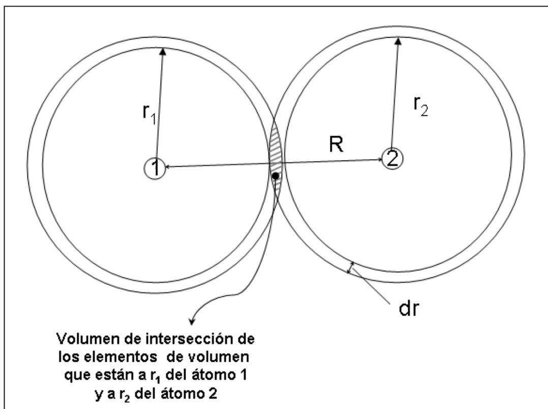
Figura 2.2. Representación de la intersección de las esferas de solvatación de dos átomos de una proteína o de proteínas diferentes. La zona delimitada mediante líneas indica el volumen de intersección. R es la distancia entre los dos átomos, r_1 y r_2 el radio de cada esfera y dr es la diferencia entre las dos esferas de un mismo átomo.
