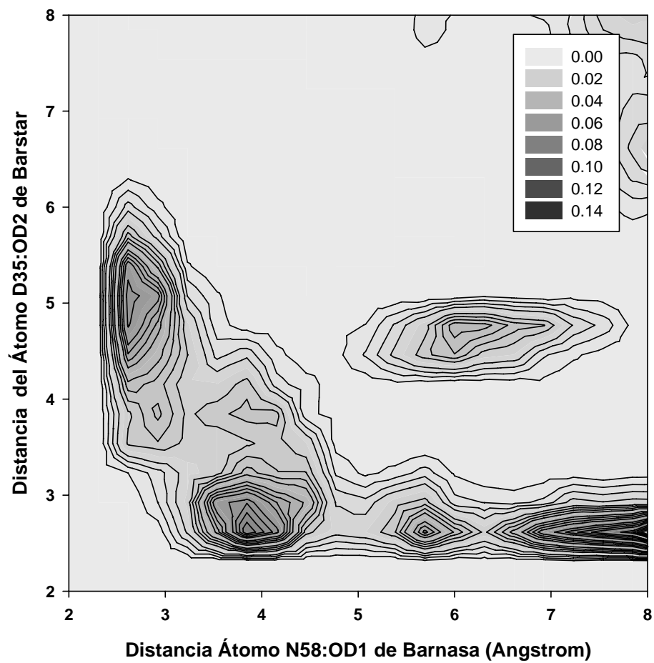
Figura 4.25. Evaluación de la función radial de dos centros para átomos de la interfase entre barnasa y barstar, con la finalidad de identificar moléculas de agua que medien dichas interacciones.
