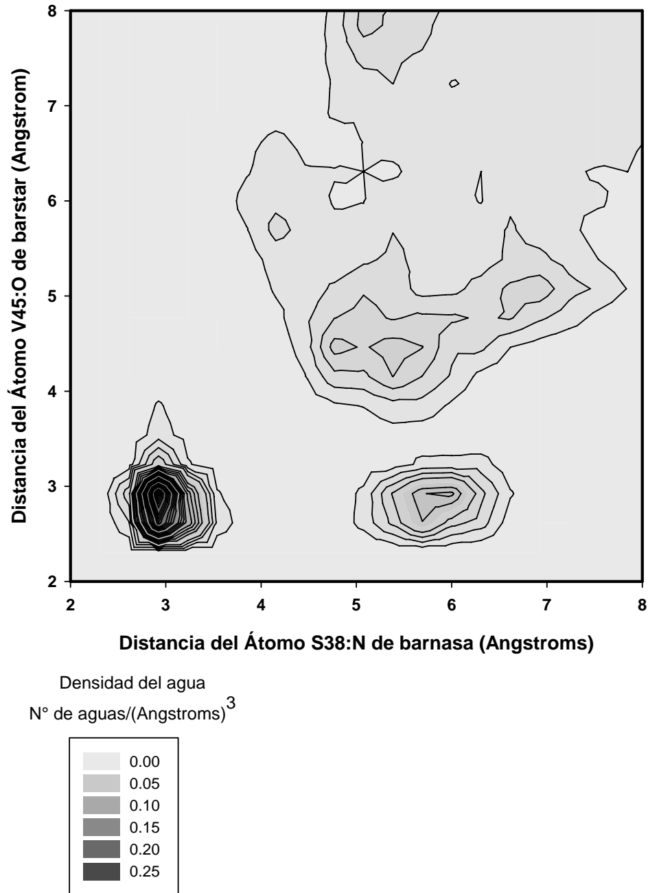
Figura 2.4. Evaluación de la función radial de dos centros para el nitrógeno de la serina 38 de la cadena principal de la proteína barnasa y el oxígeno del grupo carbonilo de la valina 45 de la proteína barstar. La zona de alta densidad (zona oscura) es un indicador de que ambos átomos coordinan simultáneamente a una misma molécula de agua, pues la distancia de la molécula de agua con respecto a cada uno de los átomos, corresponde a una distancia típica de un puente de hidrógeno.
