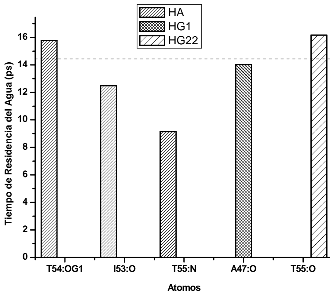
Figura 4.20. Diagrama de barras en el que se muestran los átomos que pueden formar puentes de hidrógeno con los HA, HG1 y HG22 de la Thr54 de la proteína tendamistat a una distancia inferior a los 5 Å, considerando \tau_2 de decaimiento. La línea punteada indica el tiempo promedio de permanencia de las moléculas de agua dentro de la primera esfera de solvatación, considerando P_\alpha(t=0) > 0.15 .
