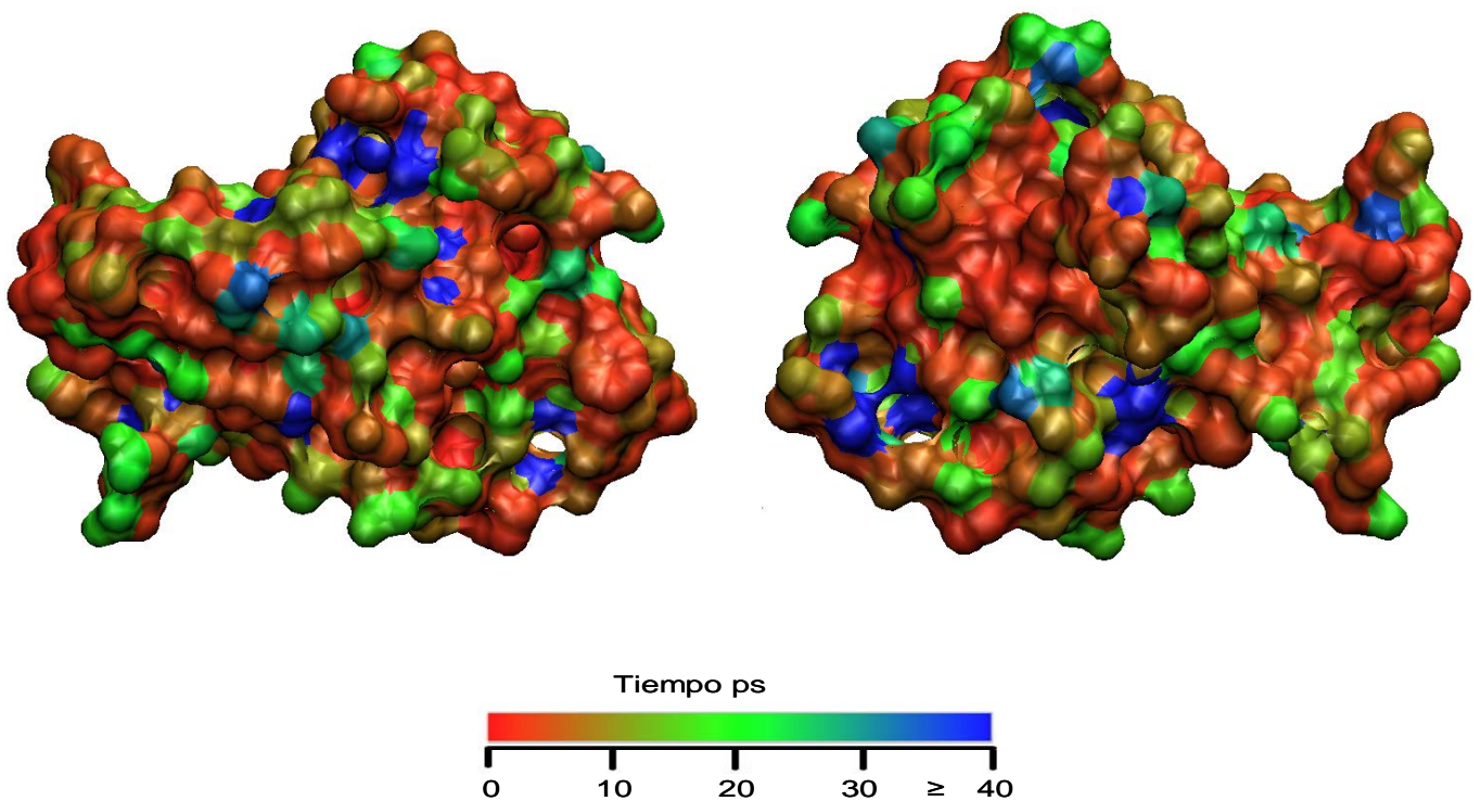
Figura 4.6. Distribución de las moléculas de agua en la proteína FKBP12, de acuerdo al tiempo de residencia de éstas en la proteína, mediante la evaluación de la función de supervivencia, teniendo en cuenta \tau_2 de decaimiento. La escala de colores es un indicador del tiempo de residencia de las moléculas de agua en la primera esfera de solvatación. Esta escala va desde el rojo que corresponde a las moléculas de agua que se intercambian rápidamente con el seno de la solución, al azul que indica altos tiempos de residencia de las moléculas de agua.
