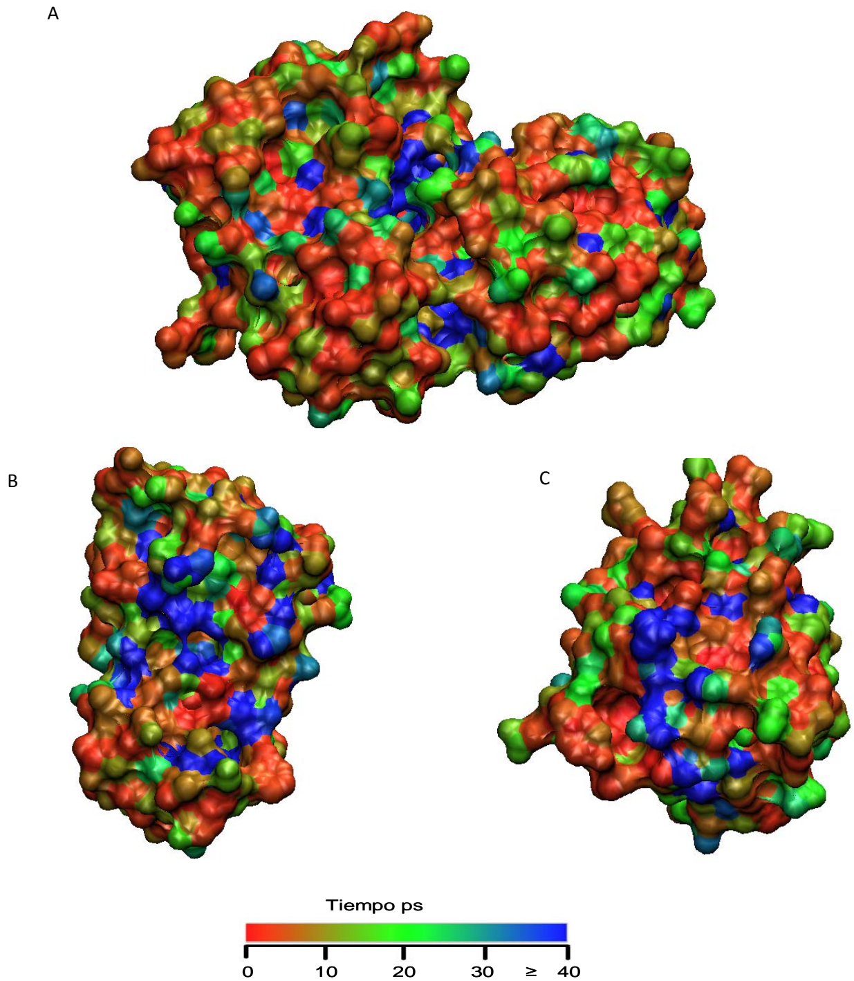
Figura 4.8. Distribución de las moléculas de agua en el complejo, de acuerdo al tiempo de residencia de éstas en la proteína, mediante la evaluación de la función de supervivencia, teniendo en cuenta \tau_2 de decaimiento. La escala de colores es un indicador del tiempo de residencia de las moléculas de agua en la primera esfera de solvatación. Esta escala va desde el rojo que corresponde a las moléculas de agua que se intercambian rápidamente con el seno de la solución, al azul que indica altos tiempos de residencia de las moléculas de agua. En A se observa el complejo, en B se muestra el lado de la proteína barnasa que interactúa con la proteína barstar, en C se muestra el lado de la proteína barstar que interactúa con barnasa.
