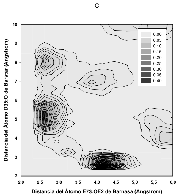
Figura 4.22. Evaluación de la función radial de dos centros para átomos de la interfase entre barnasa y barstar, con la finalidad de identificar moléculas de agua que medien dichas interacciones.
