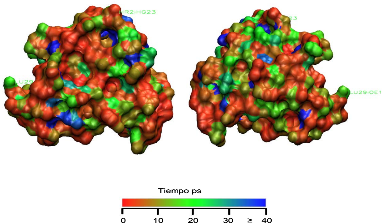
Figura 4.7. Distribución de las moléculas de agua en la proteína tendamistat, de acuerdo al tiempo de residencia de éstas en la proteína, mediante la evaluación de la función de supervivencia, teniendo en cuenta \tau_2 de decaimiento. La escala de colores es un indicador del tiempo de residencia de las moléculas de agua en la primera esfera de solvatación. Esta escala va desde el rojo que corresponde a las moléculas de agua que se intercambian rápidamente con el seno de la solución, al azul que indica altos tiempos de residencia de las moléculas de agua.
