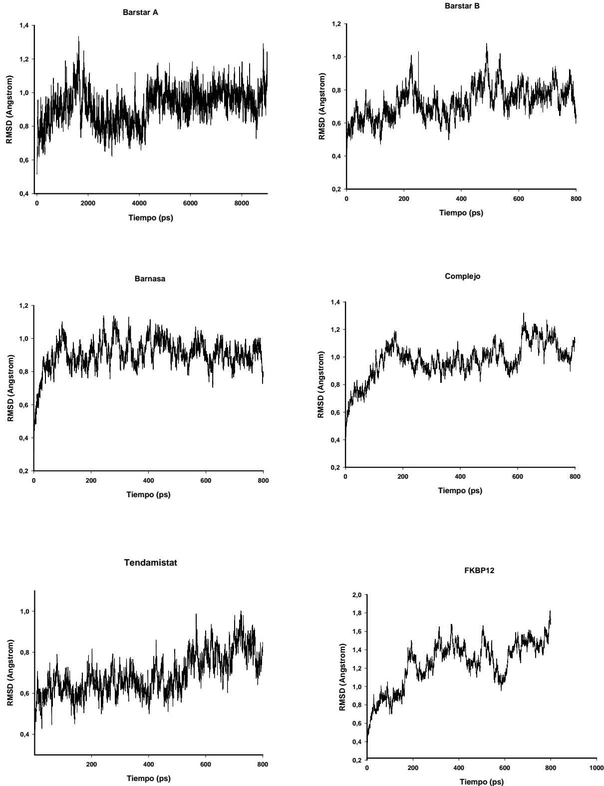
Figura 3.3. Gráficas de RMSD vs tiempo. La primera gráfica de barstar (barstar A) es una representación de los últimos 9000 ps de su trayectoria de 15000 ps. La segunda gráfica de barstar (barstar B) corresponde a la elección de los 800 ps más estables, considerando la gráfica de los 9000 ps (barstar A). En las restantes gráficas se representan los 800 ps más estables de cada una de las proteínas, los cuales se eligieron para el posterior análisis. Para construir cada una de estas gráficas, se consideró la primera configuración después del equilibrio de la dinámica molecular, como la de referencia.
