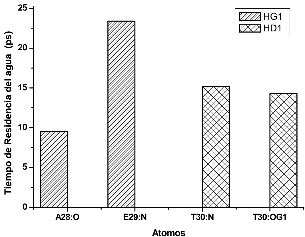
Figura 4.18. Diagrama de barras en el que se muestran los átomos que pueden formar puentes de hidrógeno con los HG1 y HD1 de la Pro50 de la proteína tendamistat a una distancia inferior a los 5 Å, considerando \tau_2 de decaimiento. La línea punteada indica el tiempo promedio de permanencia de las moléculas de agua dentro de la primera esfera de solvatación, considerando P_\alpha(t=0) > 0.15 .
