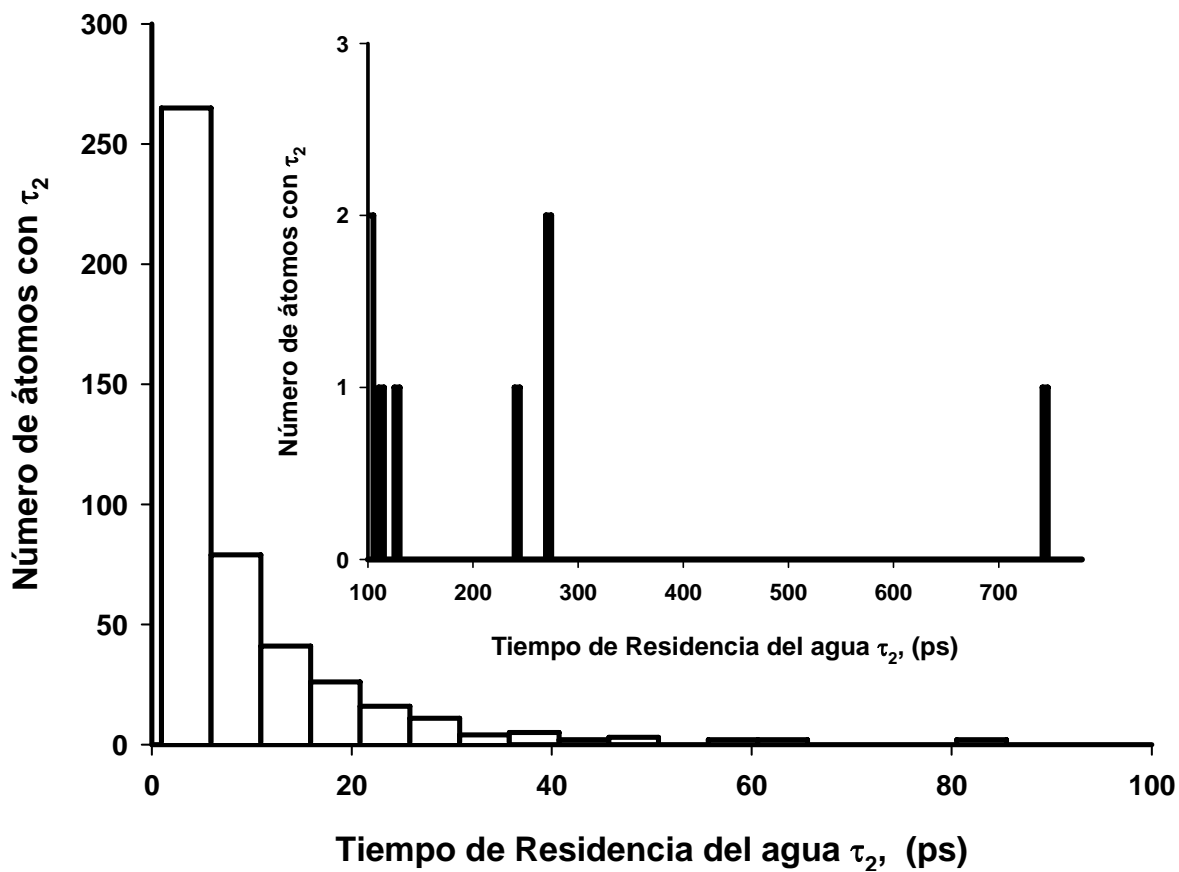
Figura 4.5. Distribución de los tiempos residencia de las moléculas de agua de la proteína tendamistat dentro de la primera esfera de solvatación, considerando los valores de P_\alpha(t=0) > 0.15 y teniendo en cuenta \tau_2 de decaimiento.
