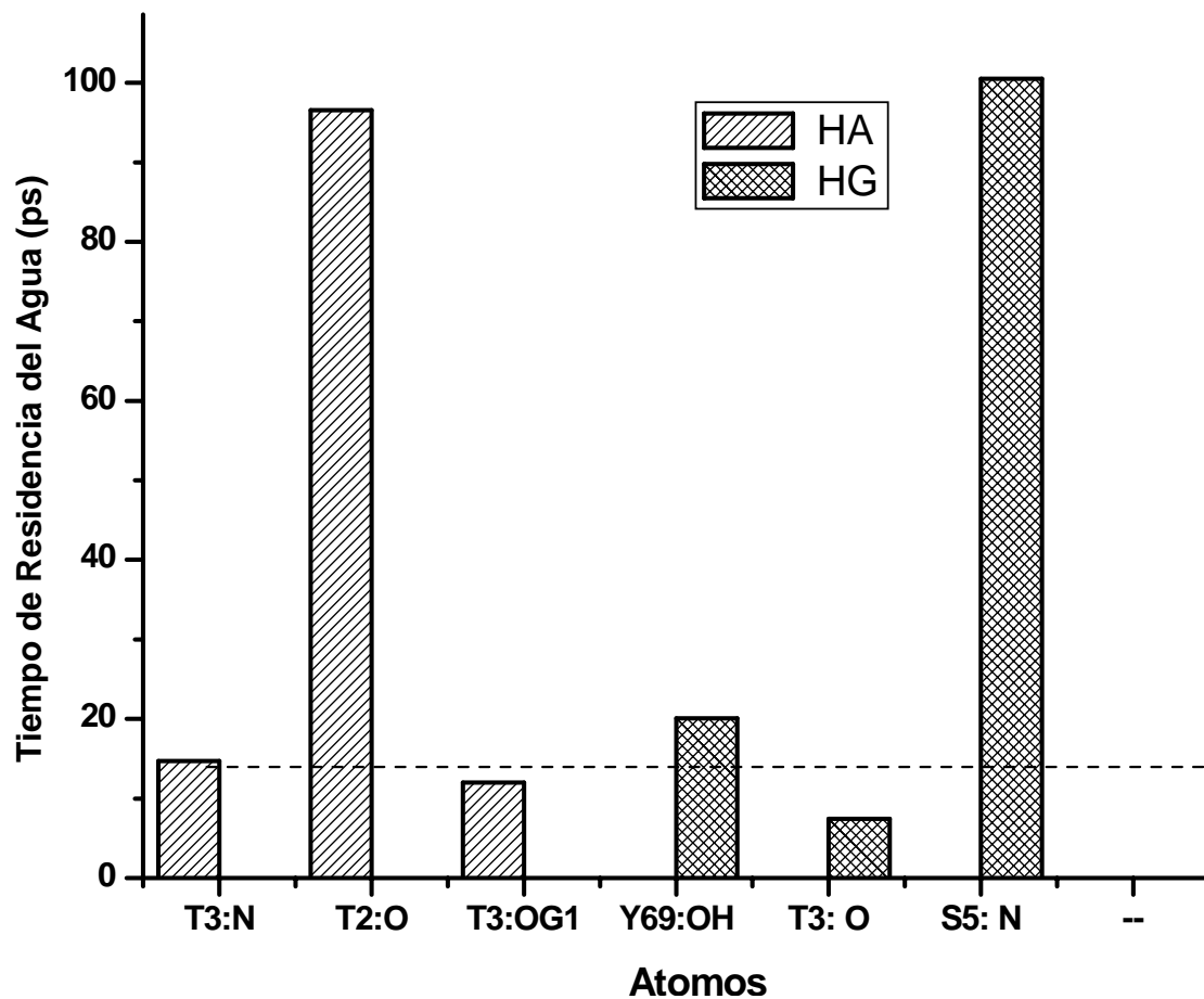
Figura 4.19. Diagrama de barras en el que se muestran los átomos que pueden formar puentes de hidrógeno con los HA y HG de la Thr3 de la proteína tendamistat a una distancia inferior a los 5 Å, considerando \tau_2 de decaimiento. La línea punteada indica el tiempo promedio de permanencia de las moléculas de agua dentro de la primera esfera de solvatación, considerando P_\alpha(t=0) > 0.15 .
