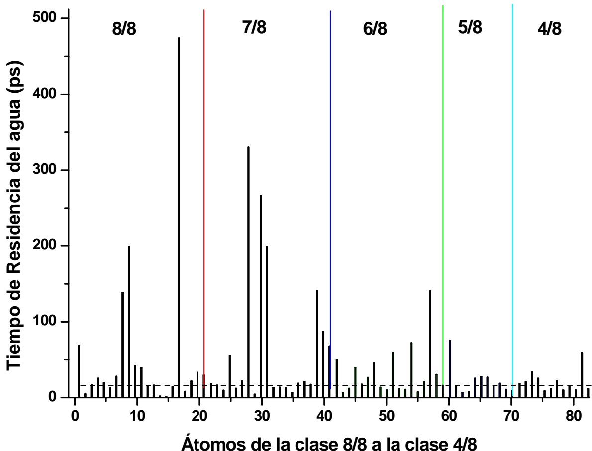
Figura 4.12. Gráfica del tiempo de residencia del agua. Comparación de los sitios de hidratación de la simulación de DM de la FKBP12, considerando \tau_2 de decaimiento vs los átomos correspondientes a las clases de los sitios de hidratación reportados por Karplus 16 . La línea punteada representa el tiempo promedio de permanencia de las moléculas de agua en la esfera de solvatación, cuando P_\alpha(t=0) > 0.15 .
