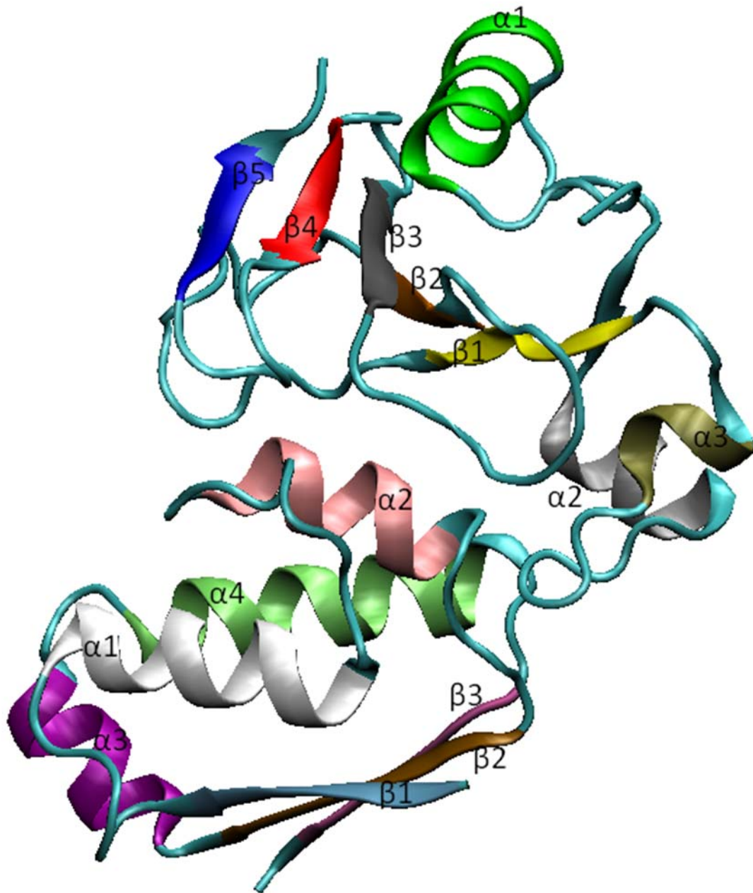
Figura 2.7. Diagrama del complejo barnasa-barstar plegado, utilizando el programa VMD. Barnasa está formada por 3 hélices \alpha ( \alpha 1 de color verde, \alpha 2 de color plata y \alpha 3 de color beigs) y 5 hojas \beta antiparalelas ( \beta 1 de color amarillo, \beta 2 de color naranja, \beta 3 de color gris, \beta 4 de color rojo y \beta 5 de color azul) y barstar la integran 4 hélices \alpha ( \alpha 1 de color blanco, \alpha 2 de color rosado, \alpha 3 de color morado y \alpha 4 de color verde claro) y 3 hojas \beta paralelas ( \beta 1 de color azul claro, \beta 2 de color café y \beta 3 de color morado claro).
