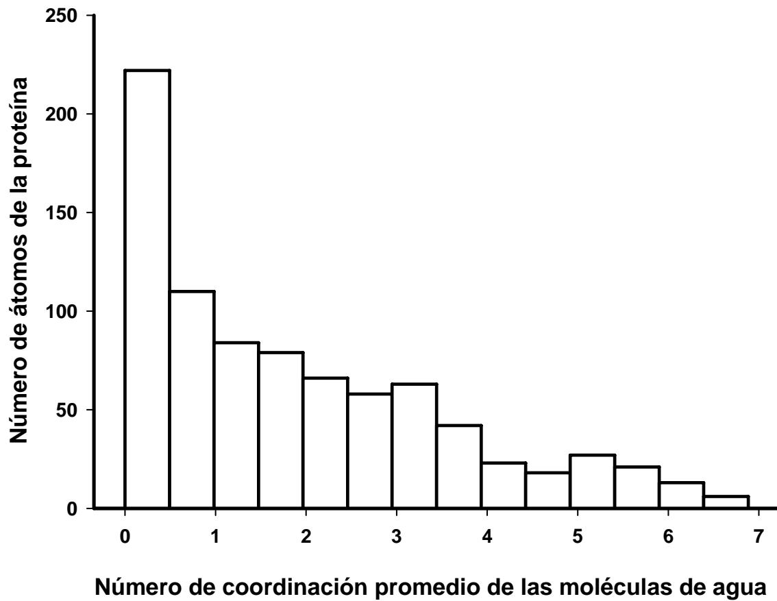
Figura 4.10. Distribución del número de moléculas de agua en la primera esfera de solvatación de los átomos de la proteína FKBP12, sin considerar los átomos de hidrógeno; los datos se obtuvieron del valor de P_{\alpha}(t=0) (promedio del número de aguas coordinadas a un átomo).
