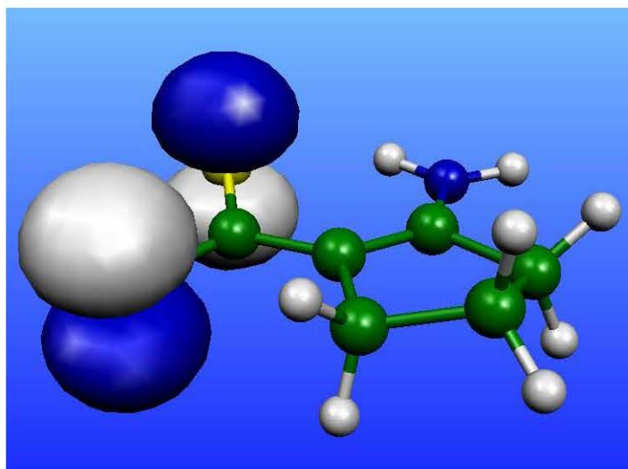
Figura 3.2.2 HOMO del anión AACD (calculado al nivel RHF/HW)
