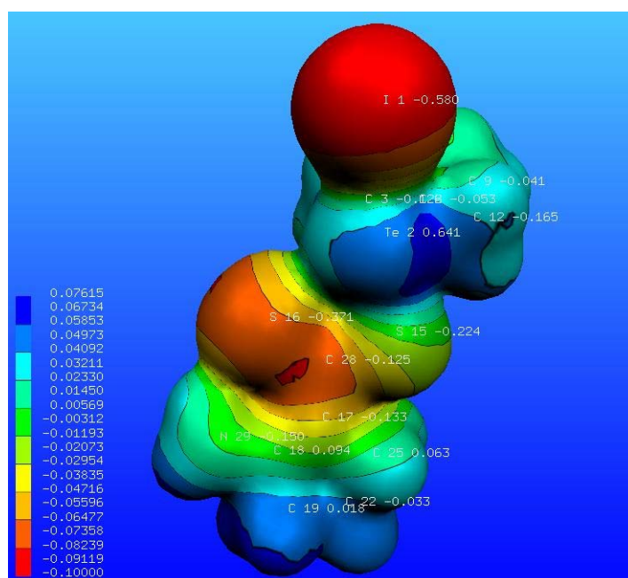
Figura 3.3.2 Cargas de Mulliken y potencial electrostático sobre la superficie de densidad electrónica ( 0.01 \text{ e}\text{\AA}^{-3} ) del compuesto Te1. Calculado a nivel RHF/TZ-SDD DZ
