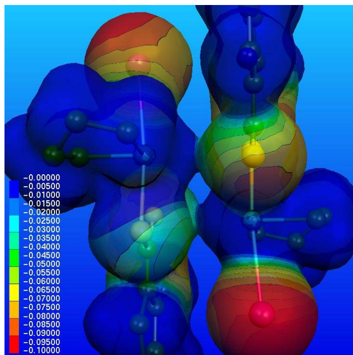
Figura 3.3.3 Potencial electrostático sobre la superficie de densidad electrónica (0.01) de la estructura dimérica del compuesto Te1. Calculado a nivel RHF/TZ-SDD DZ (Los átomos de H han sido omitidos por claridad)
