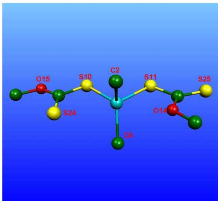
Figura 3.5.2. Esquema de numeración general para los compuestos (1), (2) y (3).
