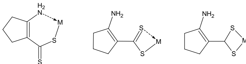
Esquema 1.2 Patrones de coordinación bidentada del AACD
