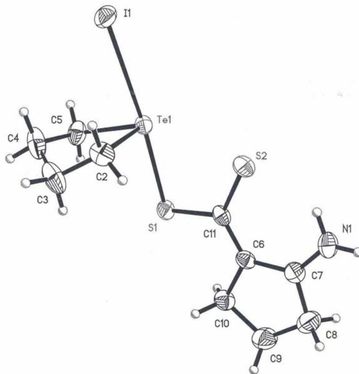
Figura 2.5.2 Gráfica ORTEP para el compuesto 1-yodo-1-(2-amino-1-ciclopentenditiocarboxilato) Telurolano (Te1)
