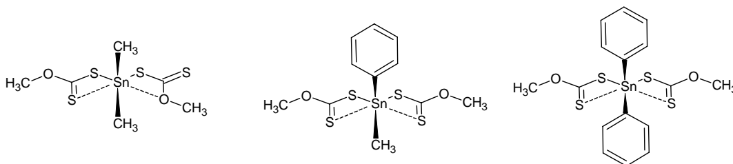
Figura 3.5.1 Xantatos de diorganilestano (IV). Compuestos (1), (2) y (3), respectivamente
