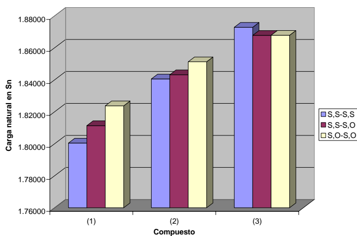
Figura 3.5.3. Cargas naturales para Sn en (1), (2) y (3). Calculados a nivel RHF/TZ-SDD DZ
