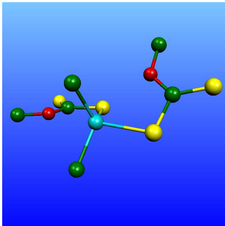
Figura 3.5.7. Estructura final del compuesto (1) calculada a nivel RHF/SDD DZ (Los átomos de H han sido omitidos para mayor claridad)
