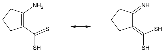
Esquema 1.1 Equilibrio tautomérico del AACD
