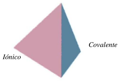
Figura 1.1 Espectro continuo del enlace químico según el tetraedro de Laing
