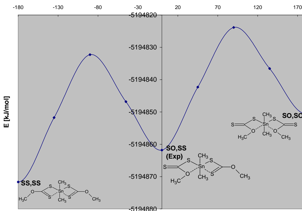
Figura 3.5.6 Perfil energético para la rotación de ambos ligantes en (1) partiendo de la coordinación experimental. Calculado a nivel RHF/TZ-SDD DZ
