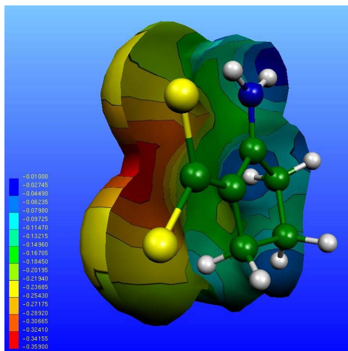
Figura 3.2.1 Potencial electrostático del anión AACD graficado sobre la superficie de densidad electrónica (calculada al nivel RHF/HW y graficada a 0.01e\text{\AA}^{-3} )
