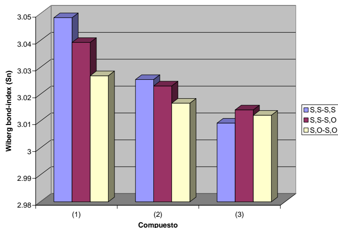
Figura 3.5.4. Índice de enlace de Wiberg total para Sn. Calculados a nivel RHF/TZ-SDD DZ
