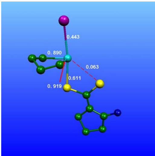
Figura 3.3.1 Índices de enlace de Wiberg para los poliedros de coordinación.
