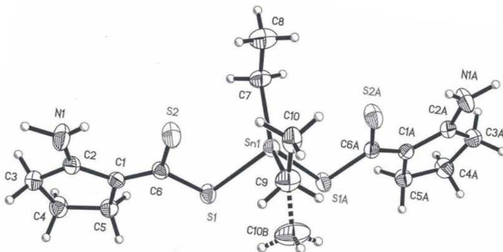
Figura 2.5.1 Gráfica ORTEP para el compuesto bis(2-amino-1-ciclopentenditiocarboxilato) de dietilestaño (IV) (Sn1)
