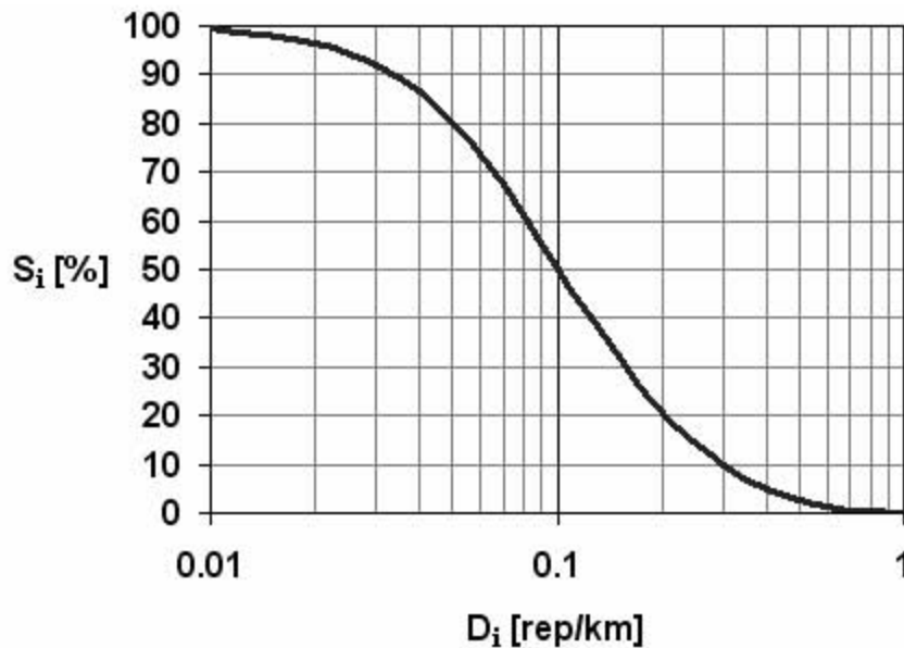
Figura 6-5. Función de serviciabilidad estándar propuesta por NIBS (1996)
