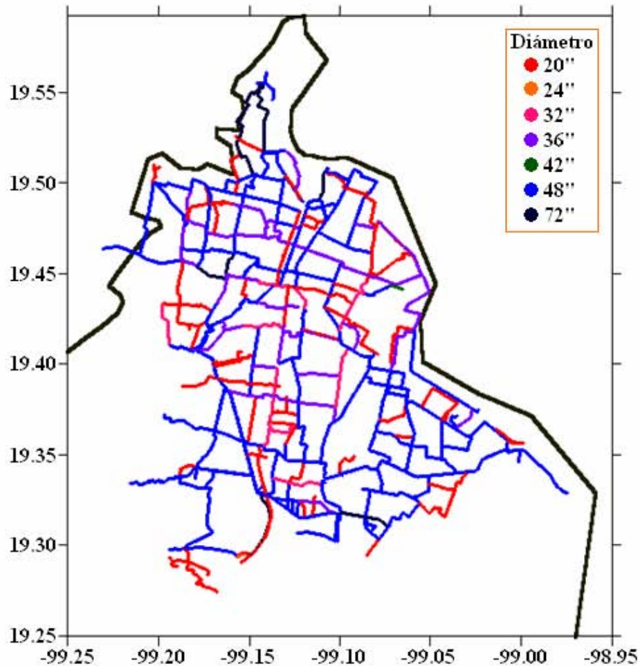
Figura 5-1. Red primaria de distribución de agua potable del Distrito Federal
