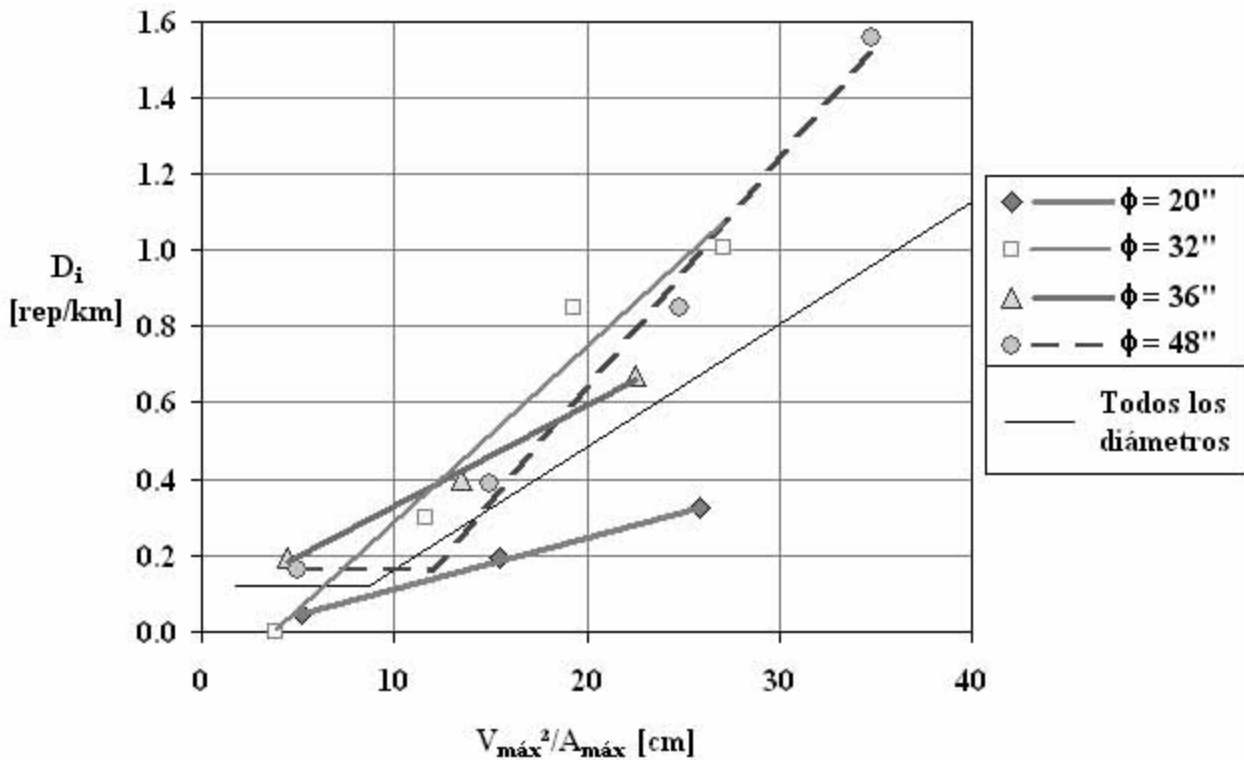
Figura 5-10. Funciones de daño para cuatro diámetros
