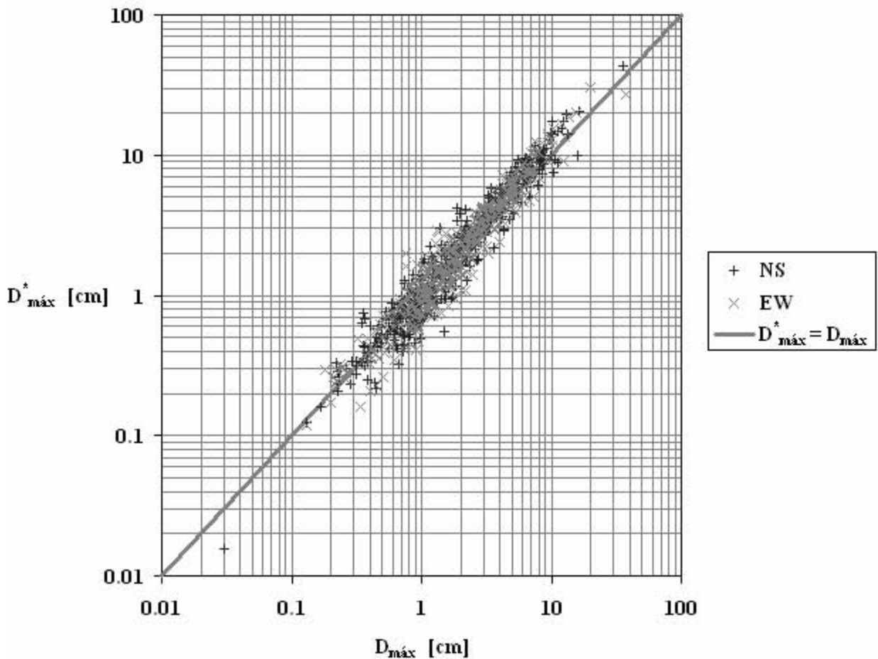
Figura 4-5. D_{m\acute{a}x}^* vs. D_{m\acute{a}x} para los registros de la Tabla 4-1
