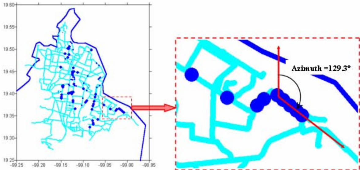
Figura 5-8. Detalle de un grupo de reparaciones consecutivas en un tramo de la RPDAP
