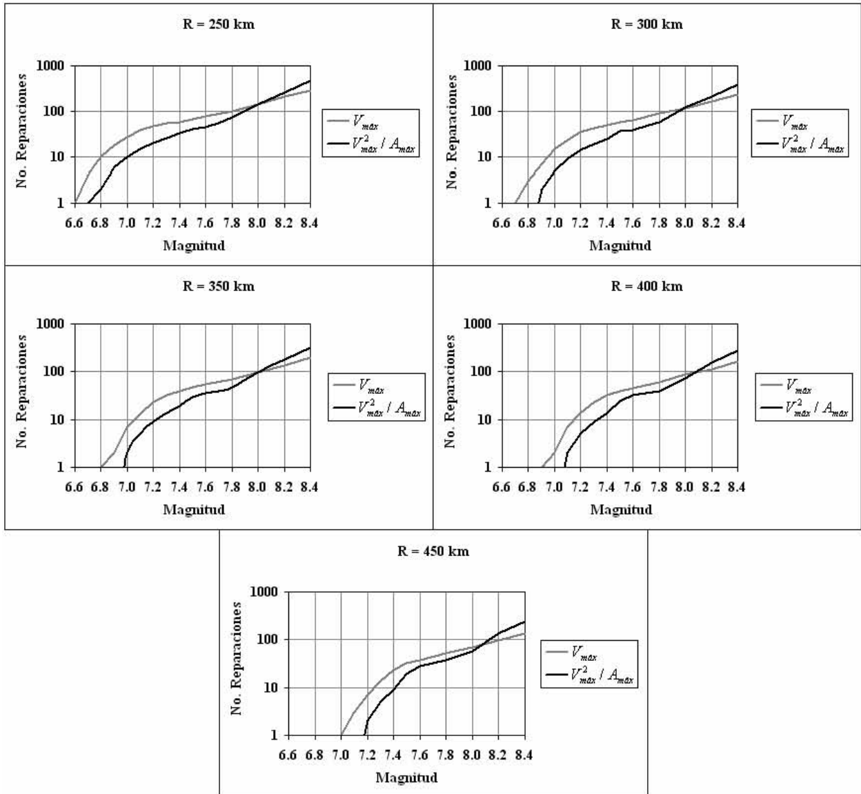
Figura 6-3. Comparación de resultados entre el modelo de Pineda y Ordaz (2003) y el propuesto (usando el parámetro)
