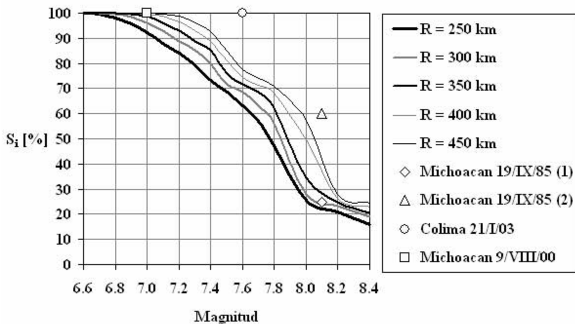
Figura 6-6. Índice medio de serviciabilidad empleando la función de serviciabilidad de NIBS y tres valores de S_i asociados a sismos pasados
