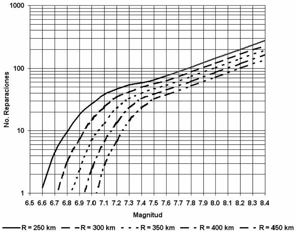
Figura 6-1. Curvas de daño usando V_{máx} (Pineda y Ordaz, 2003)
