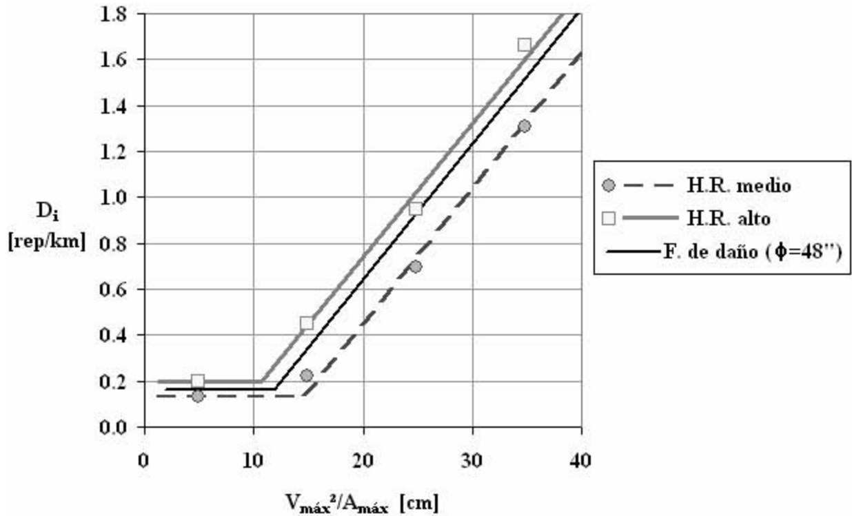
Figura 5-11 Funciones de daño sísmico para dos niveles de hundimiento relativo (H.R.)
