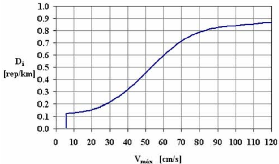
Figura 5-2. Función de daño propuesta por Pineda y Ordaz (2003)
