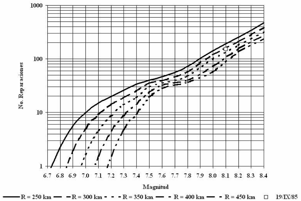
Figura 6-2. Curvas de daño usando el parámetro V_{máx}^2 / A_{máx}
