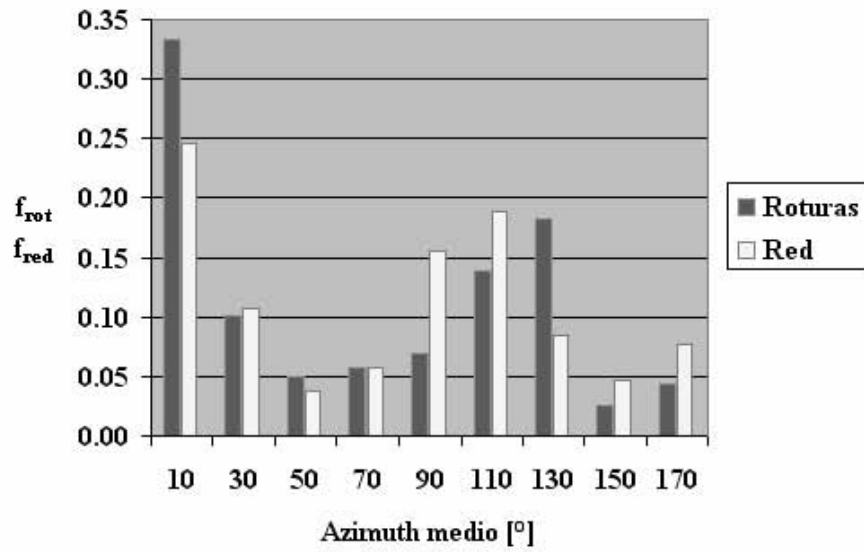
Figura 5-6. Frecuencias relativas para las reparaciones y la red asociadas a diferentes orientaciones de las tuberías
