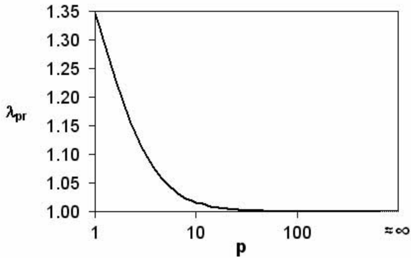
Figura 4-3. Variación de \lambda_{pr} con el ancho de banda (definido por p )
