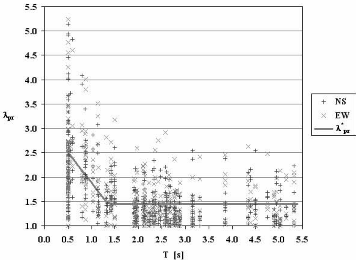
Figura 4-4. \lambda_{pr} vs. T para los registros de la tabla 1 y gráfica de \lambda_{pr}^* (ec. 4-20)
