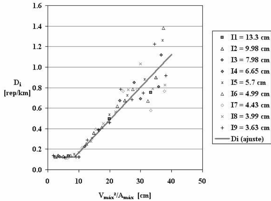
Figura 5-4. Función de daño en términos del parámetro V_{\max}^2 / A_{\max}
