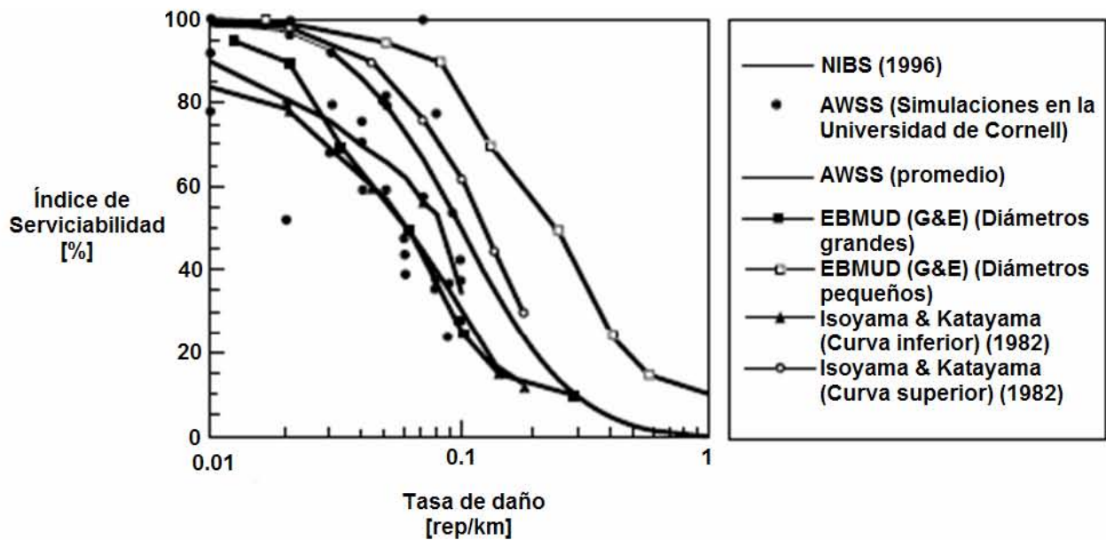
Figura 6-4. Curvas de fragilidad para evaluación sísmica de sistemas de distribución de agua (O’rourke y Liu, 1996)
