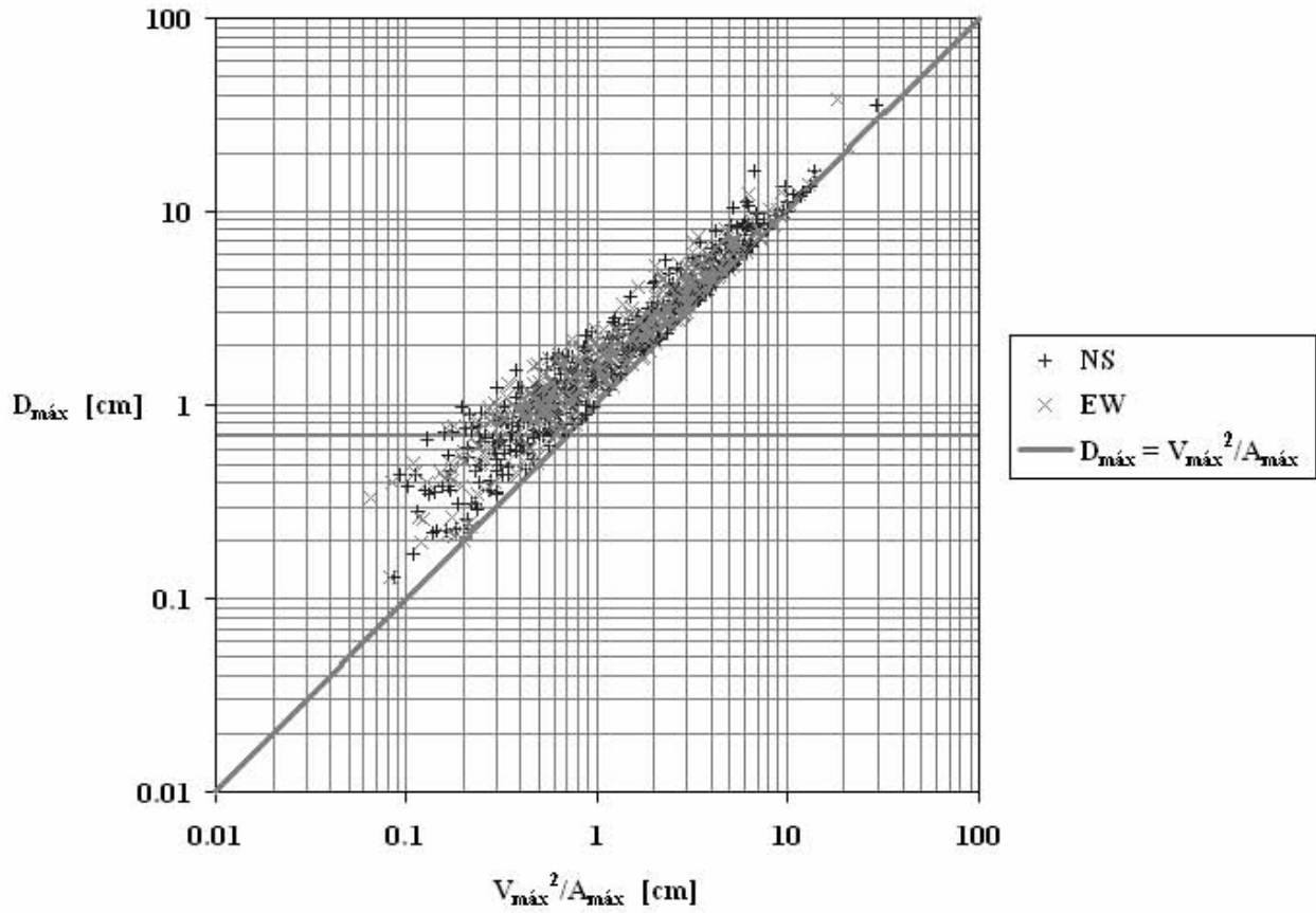
Figura 4-1. Gráfica de D_{máx} vs. V_{máx}^2 / A_{máx} para los registros de la Tabla 4-1
