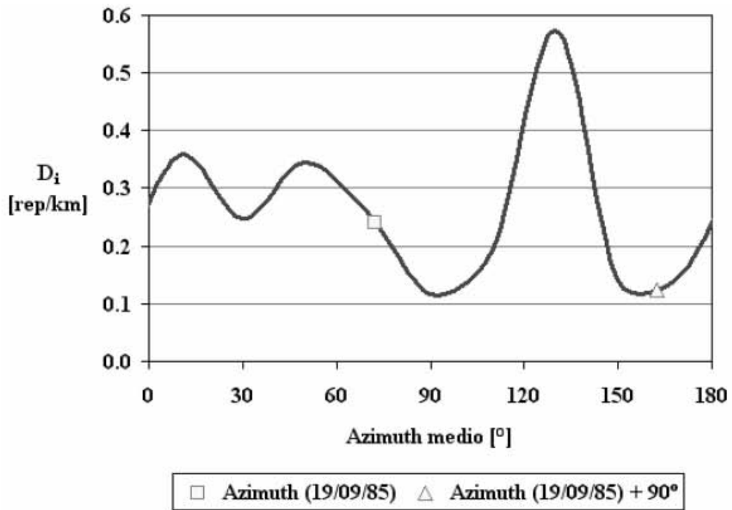
Figura 5-7. Tasa de daño en función del azimuth medio
