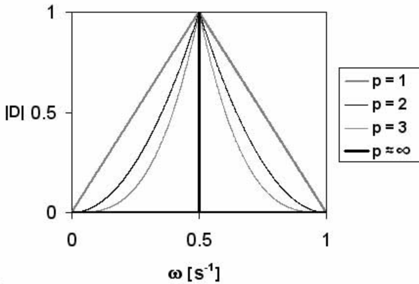
Figura 4-2. Gráfica de |D(\omega)| (ejemplo de aplicación)
