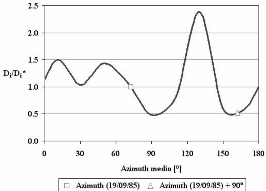
Figura 5-9. Tasa de daño normalizada con respecto al valor de D_i^*
