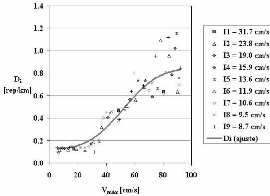
Figura 5-5. Función de daño propuesta por Pineda y Ordaz (2003) y puntos de daño empleados
