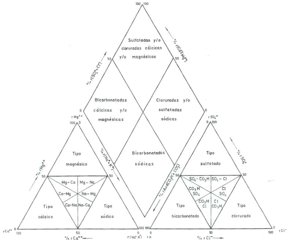
Figura 4.9 Tipos de aguas deducidas de un diagrama triangular de Piper.
