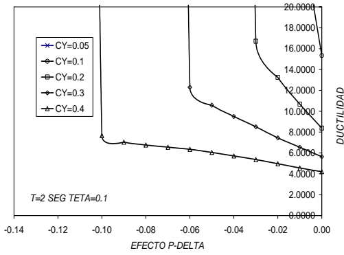
c) \theta=0.10
