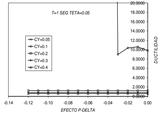
b) \theta=0.05
