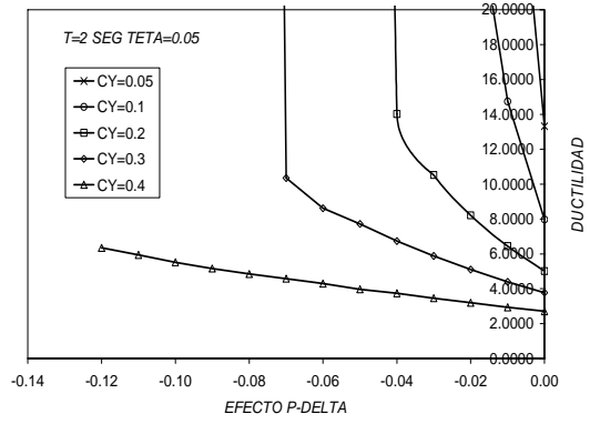
b) \theta=0.05
