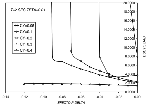
a) \theta=0.01
