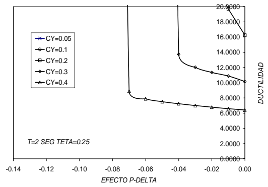
d) \theta=0.25
