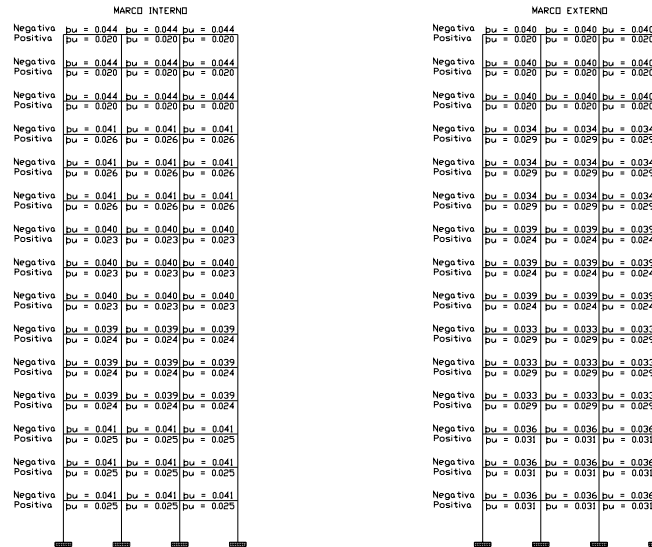
Figura 5.4 Capacidades Rotacionales en Marcos Interno y Externo del Edificio B.
