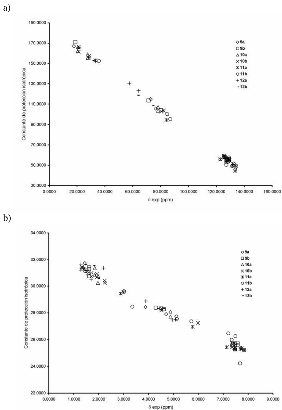
Figura 61. a) Correlación entre \sigma_{\text{is}} calculada y \delta_{\text{exp}} de ^{13}\text{C} para los pares diastereoméricos 9-12 .
