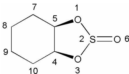
Figura 39. Sulfito cíclico 10
