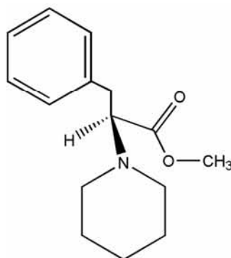
Figura 24. Compuesto 3
