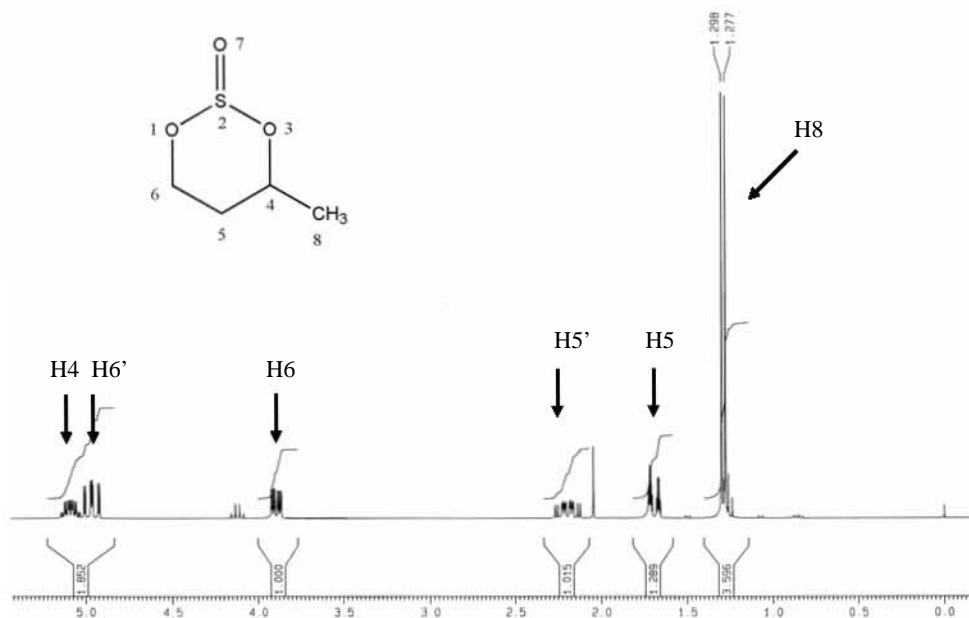
Espectro 25. RMN de ^1\text{H} de 12a
