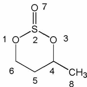
Figura 52. Sulfito cíclico 12
