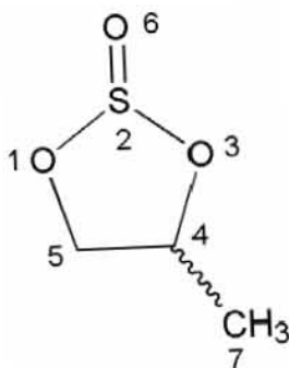
Figura 38. Sulfito cíclico 9
