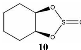
10 Hexahidro-benzo-[d]-1,3,2-dioxatiolano-2-óxido
