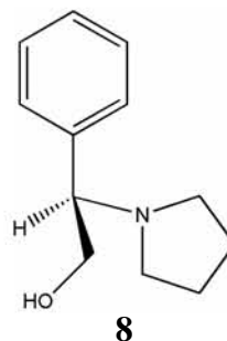
8 (2 R )-2-fenil-2-pirrolidin-1-il-etanol
