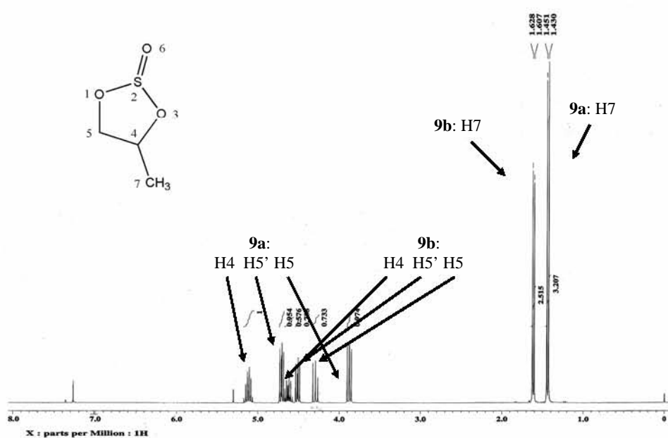
Espectro 18. RMN de 1 H de 9a-9b (Producto de reacción en condiciones de reflujo de benceno)
