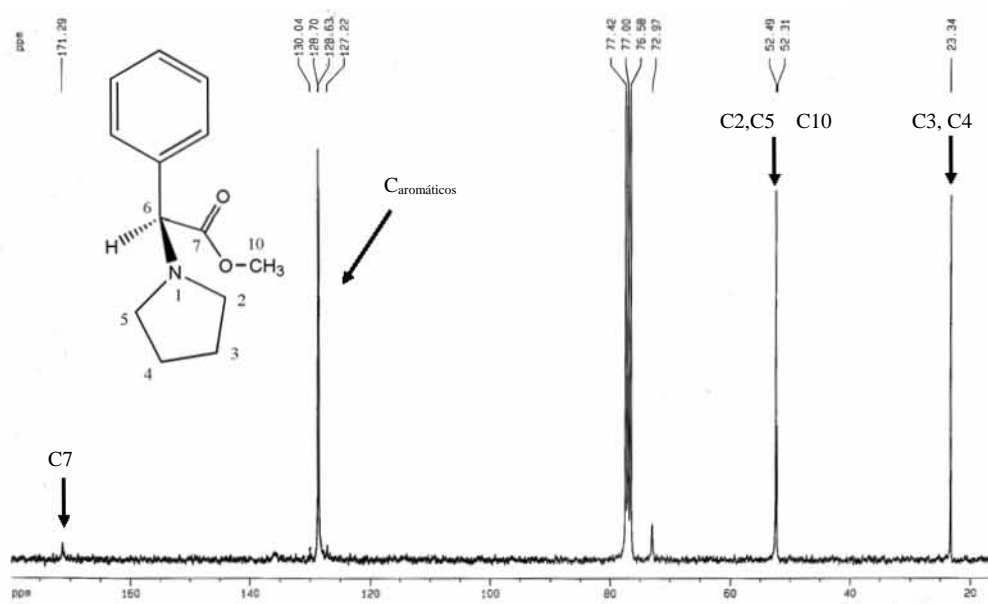
Espectro 12. RMN de ^{13}\text{C} de 6
