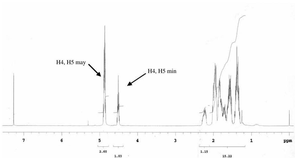
Figura 45. Espectro de RMN de ^1\text{H} (300 MHz) de la mezcla de diasterómeros 10a y 10b . Disolvente: \text{CDCl}_3 . Temperatura ambiente
