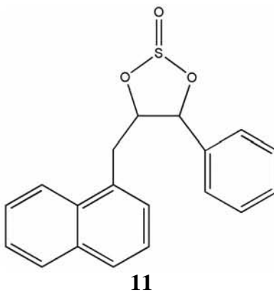
11 4-naftalen-1-il-metil-5-fenil-1,3,2-dioxatiolano-2-óxido
