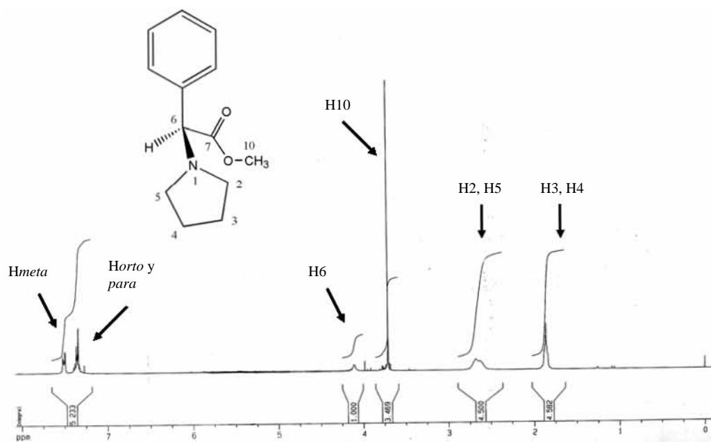
Espectro 11. RMN de ^1\text{H} de 6
