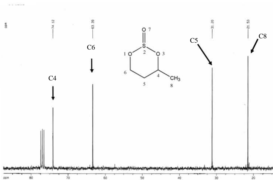
Espectro 28. RMN de 13 C de 12b
