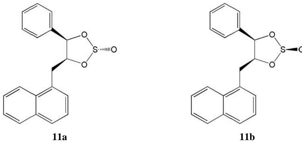
Figura 51. Estructuras de los diastéromeros 11a y 11b
