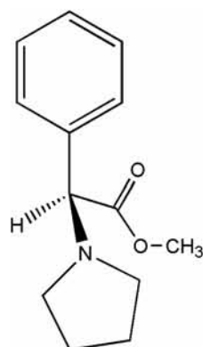
Figura 28. Compuesto 6
