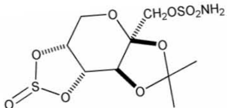
Figura 13. Sulfito cíclico 33 con actividad anticonvulsiva
