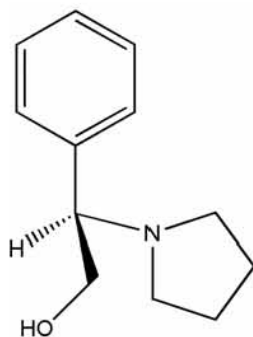
Figura 30. Compuesto 8
