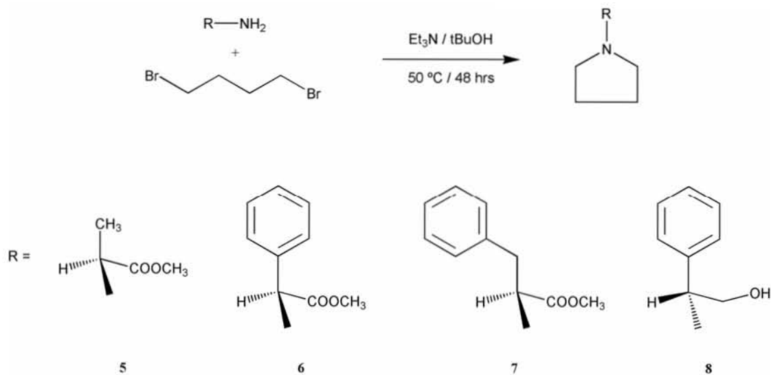
Figura 65. Esquema general de síntesis de los compuestos 5-8
