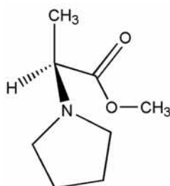
Figura 27. Compuesto 5
