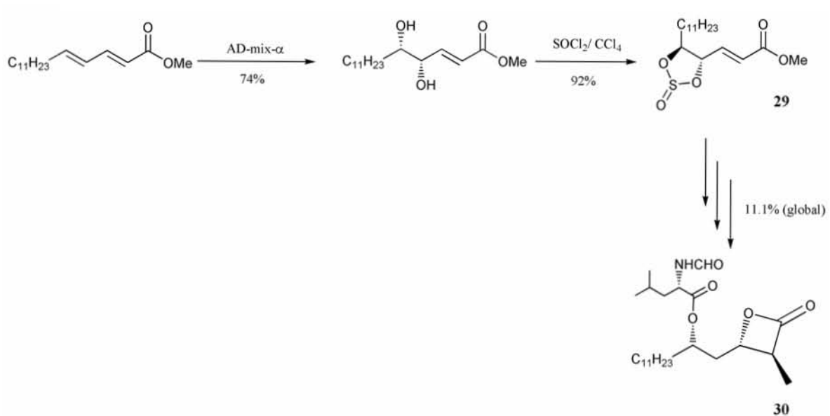
Figura 11. Empleo del sulfito 29 en la síntesis de 30
