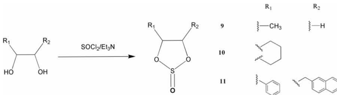
Figura 66. Síntesis de los derivados 9-11
