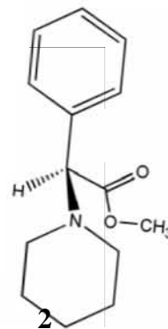
(2 S )-2-fenil-2-piperidin-1-il-acetato de metilo
