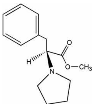
Figura 29. Compuesto 7
