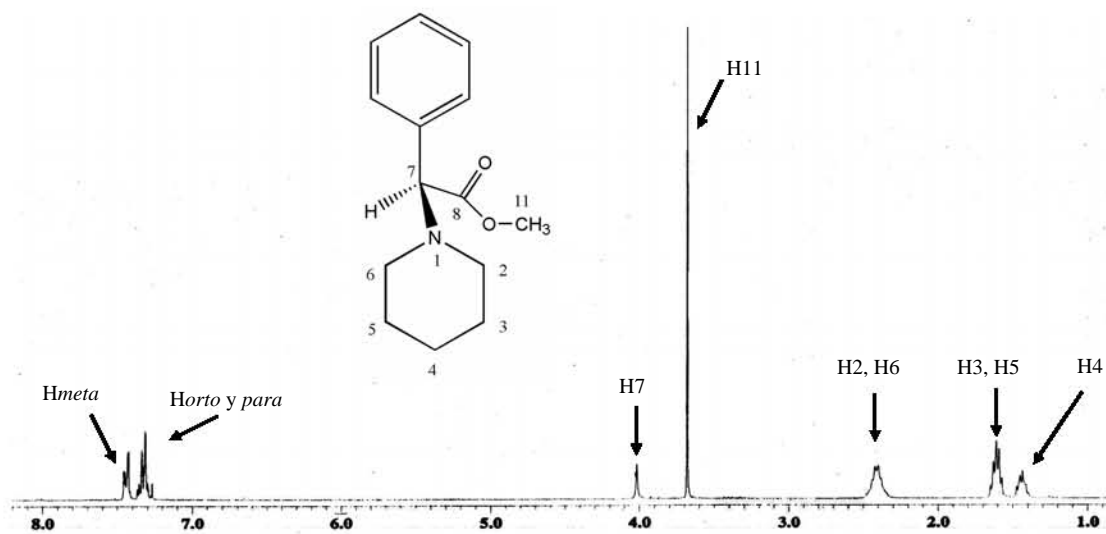
Espectro 3. RMN de ^1\text{H} de 2
