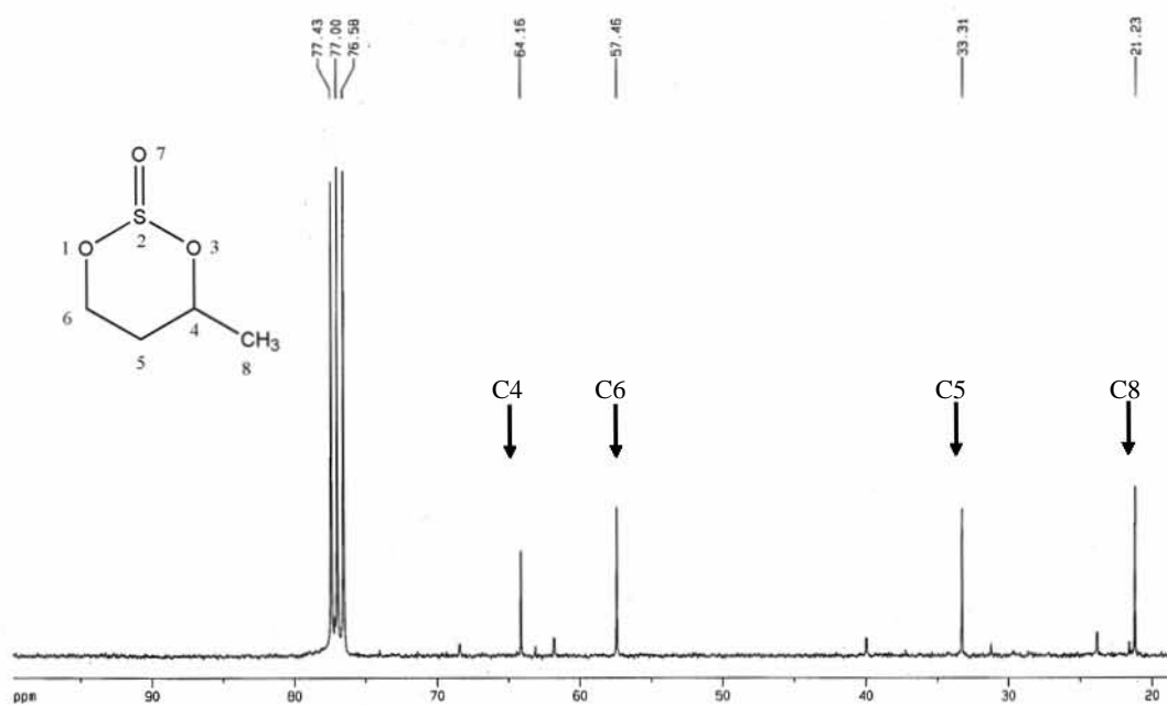
Espectro 26. RMN de ^{13}\text{C} de 12a
