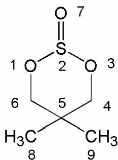
Figura 53. Sulfito cíclico 13
