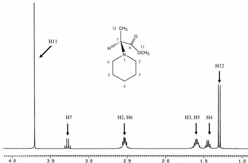
Espectro 1. RMN de ^1\text{H} de 1
