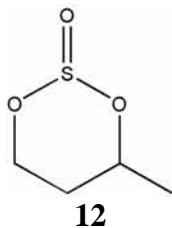
12 4-metil-1,3,2-dioxatiano-2-óxido
