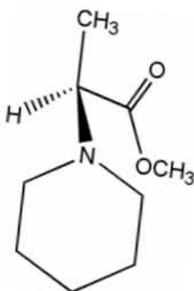
Figura 22. Compuesto 1
