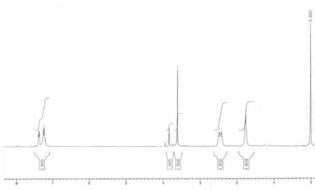
Figura 35. Espectros de RMN de 1 H de (300 MHz) de 6 a temperatura ambiente
