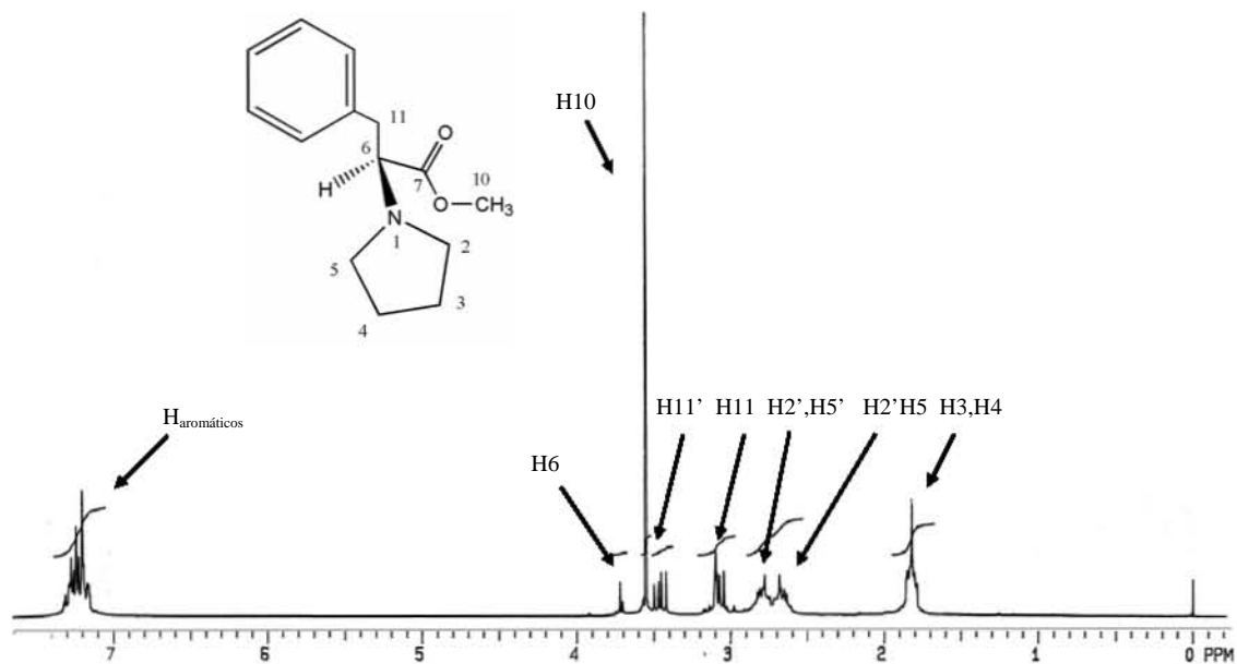
Espectro 13. RMN de ^1\text{H} de 7
