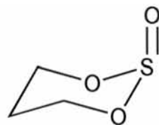
Figura 19. Sulfito cíclico 38
