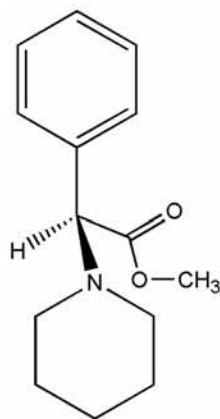
Figura 23. Compuesto 2
