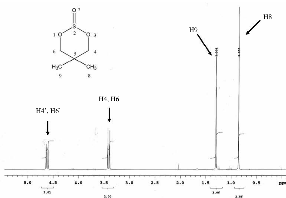
Espectro 29. RMN de ^1\text{H} de 13
