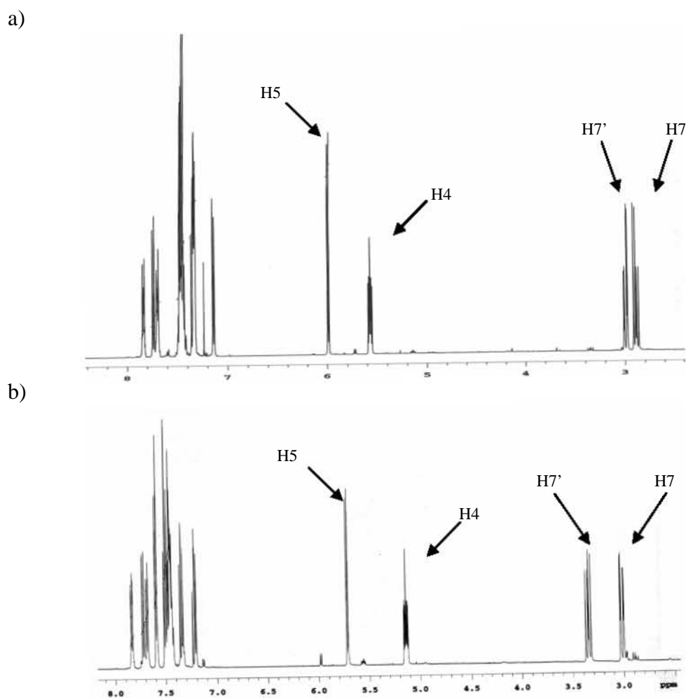
Figura 50. Espectros de RMN de ^1\text{H} (500 MHz) de los diastereómeros a) 11a y b) 11b .
