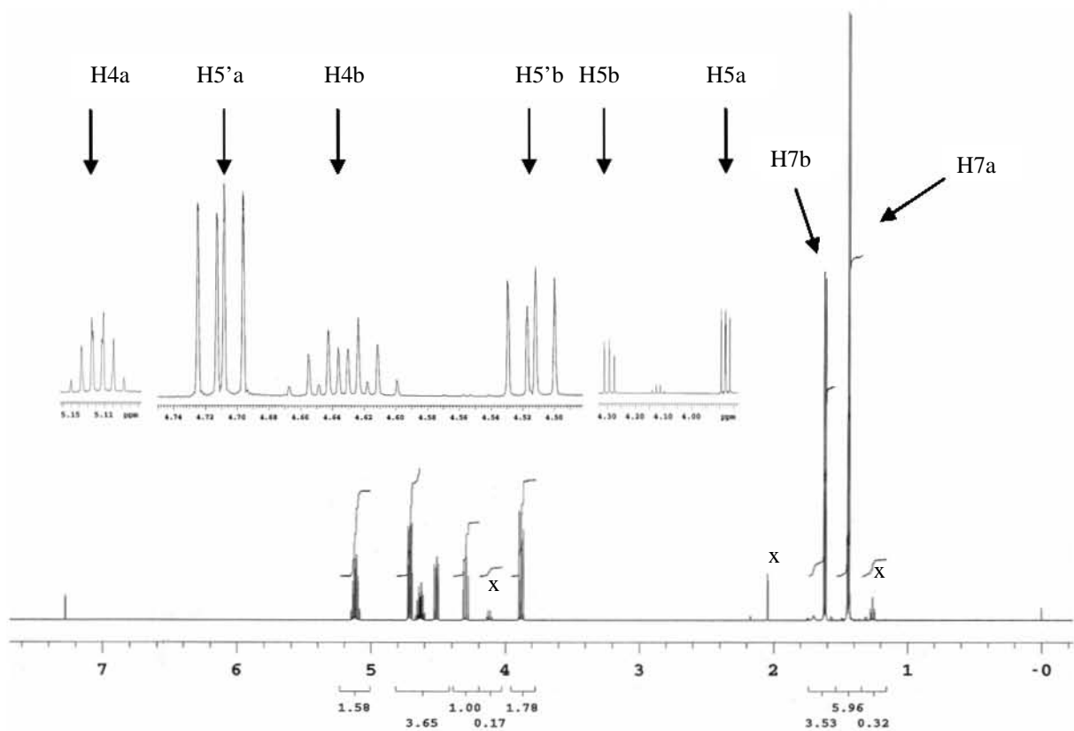
Figura 42. Espectro de RMN de 1 H (300 MHz) de la mezcla de 9a y 9b .
