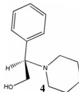
(2 R )-2-fenil-2-piperidin-1-il-etanol
