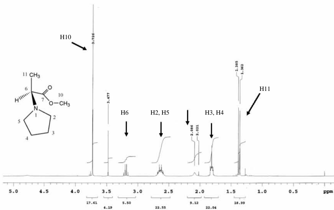
Espectro 9. RMN de 1 H de 5
