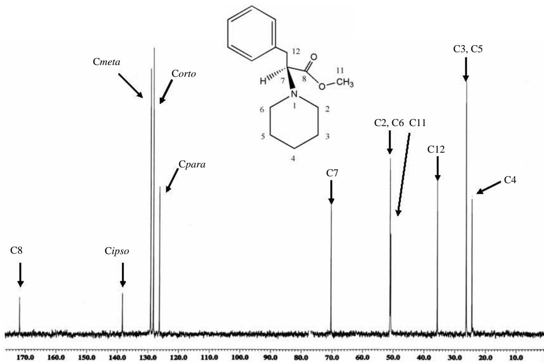
Espectro 6. RMN de ^{13}\text{C} de 3
