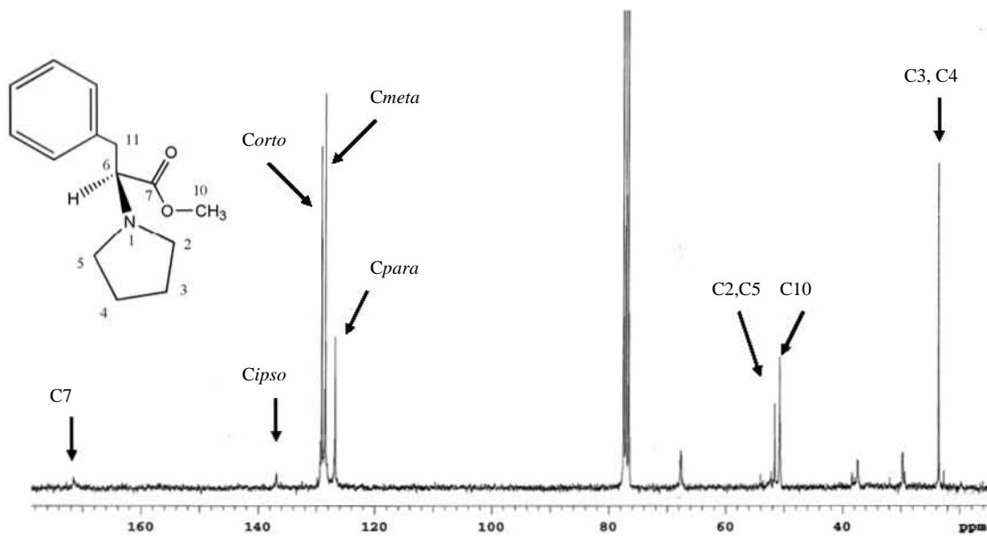
Espectro 14. RMN de ^{13}\text{C} de 7
