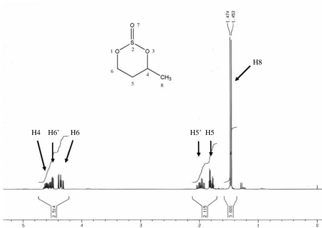
Espectro 27. RMN de 1 H de 12b
