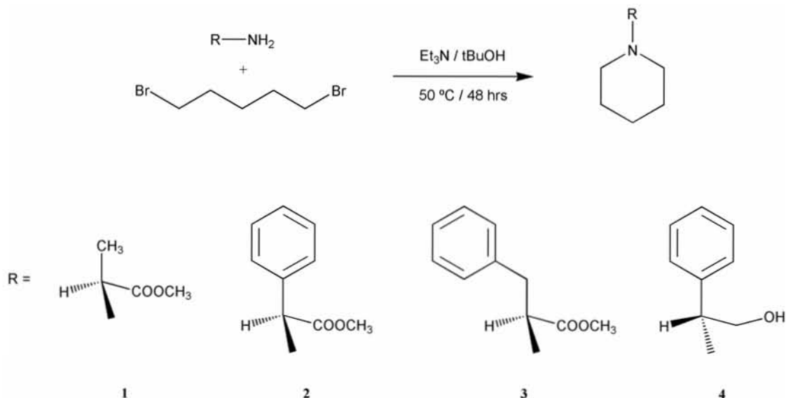
Figura 64. Metodología general para la síntesis de los derivados de piperidina 1-4
