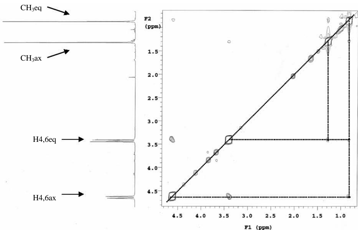
Figura 59. Espectro NOESY (300 MHz) de 13 ( \text{CDCl}_3 , temperatura ambiente)
