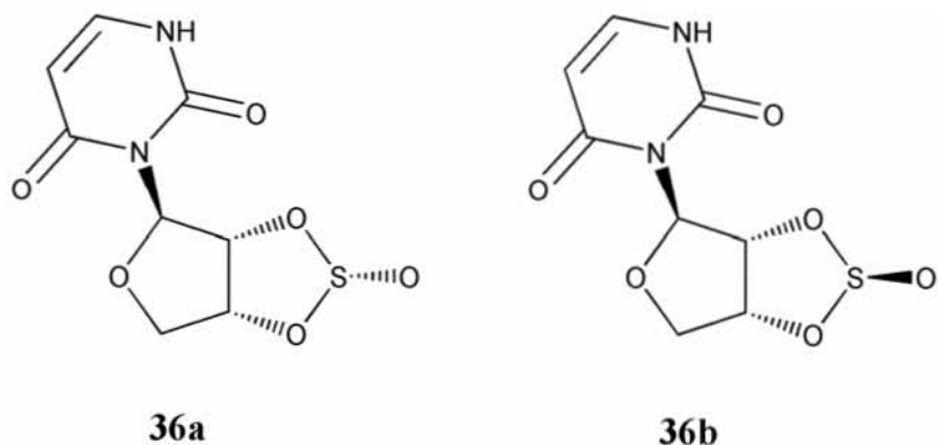
Figura 17. Sulfitos epímeros 36a y 36b
