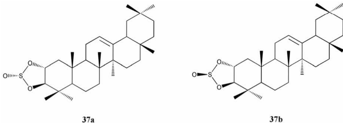
Figura 18. Sulfitos cíclicos 37a y 37b
