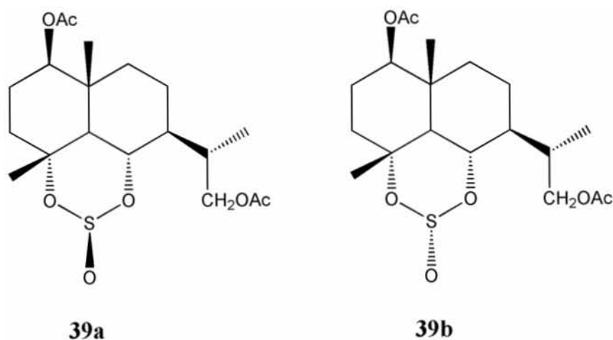
Figura 21. Sulfitos cíclicos 39a y 39b
