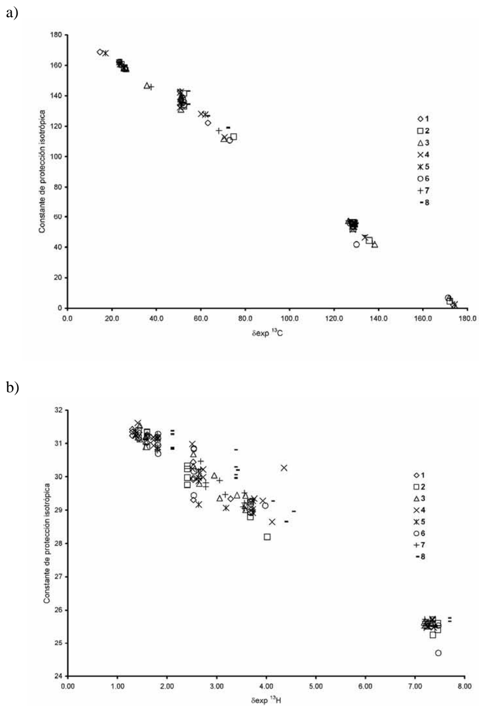
Figura 36. a) Gráfica de correlación entre \sigma_{\text{is}} calculada para cI y \delta_{\text{exp}} de ^{13}\text{C} para los compuestos 1-8 . b) Gráfica de correlación entre \sigma_{\text{is}} calculada para cI y \delta_{\text{exp}} de ^1\text{H} para los compuestos 1-8
