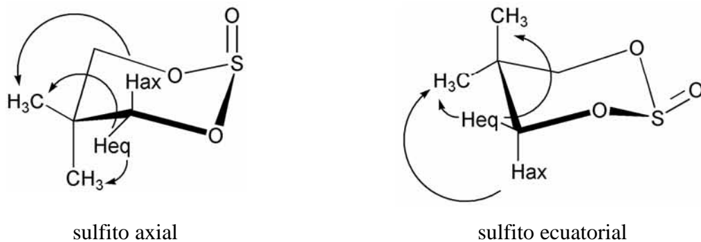
Figura 60. Posibles interacciones NOE en las dos conformaciones de 13
