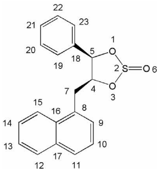
Figura 40. Sulfito cíclico 11
