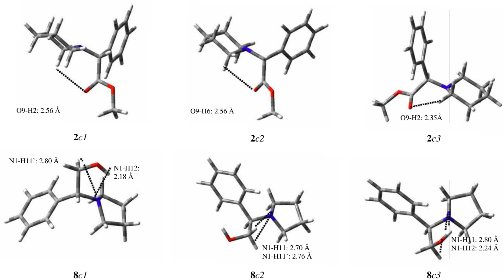
Figura 37. Variación de las distancias entre N1 y los hidrógenos del sustituyente y entre el oxígeno del carboxilo con los hidrógenos del heterociclo en los tres conformeros estudiados para 3 y 8
