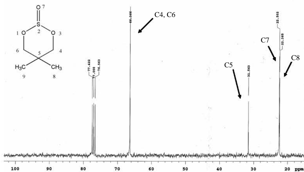
Espectro 30. RMN de ^{13}\text{C} de 13
