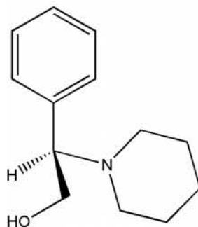
Figura 25. Compuesto 4
