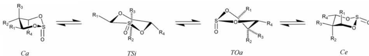
Figura 20. Posibilidades conformacionales del sistema de 1,3,2-dioxatiano-2-óxido
