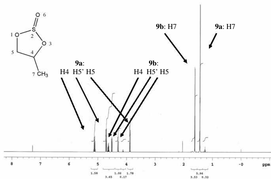
Espectro 17. RMN de 1 H de 9a-9b (Producto de reacción en éter etílico a 0 °C)
