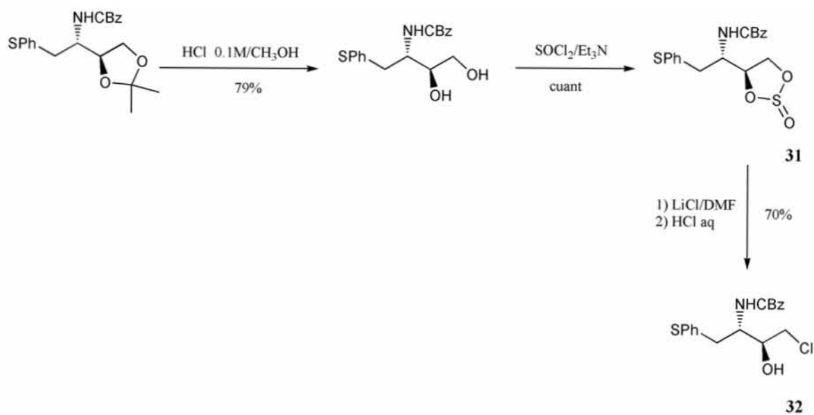
Figura 12. Apertura del sulfito cíclico 31 para la síntesis enantioselectiva de 32
