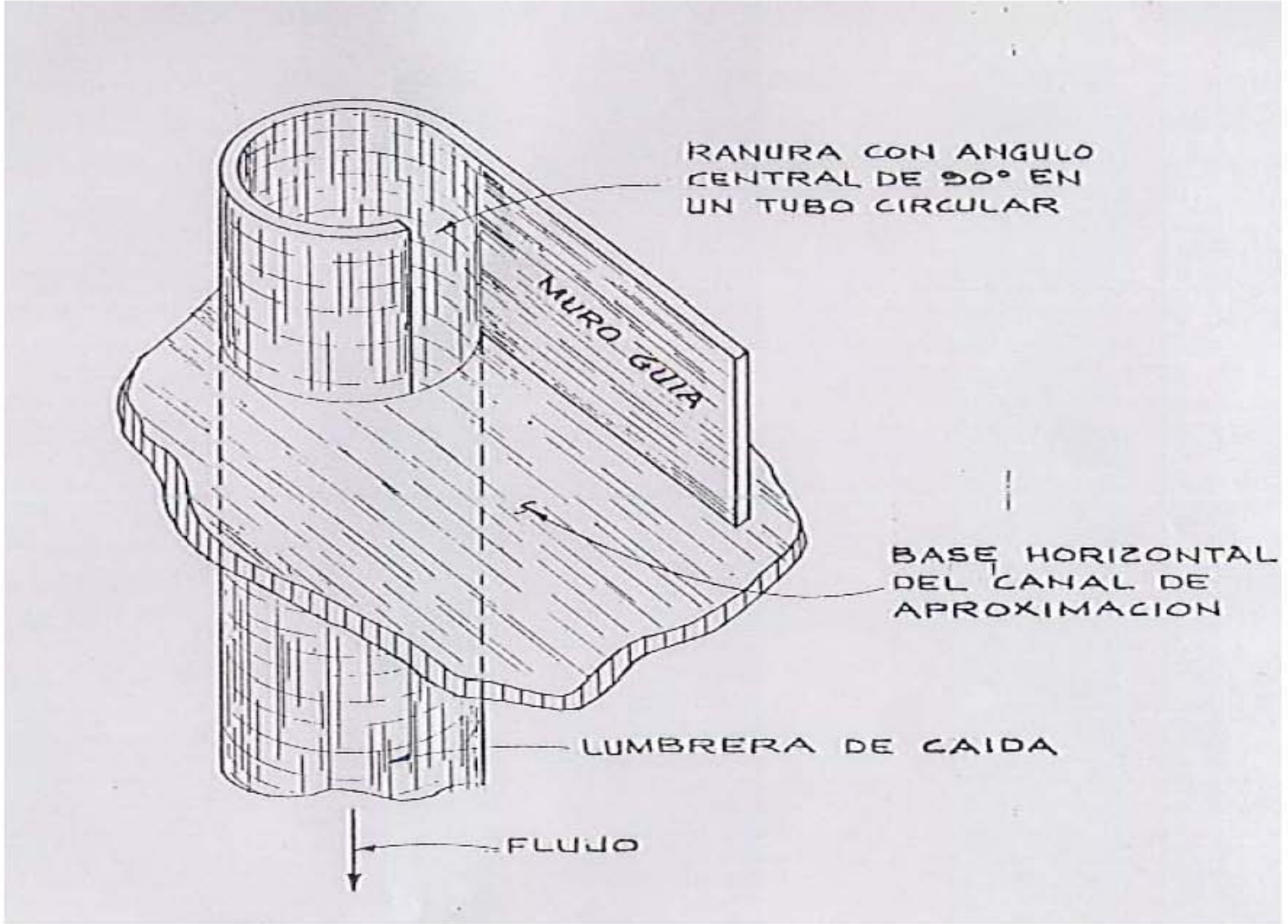
FIGURA 2.1 LUMBRERA DE RANURA VERTICAL DE QUICK
