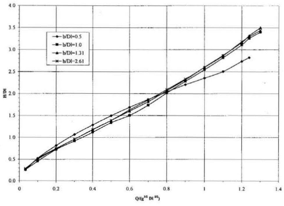
FIGURA 2.13 CURVAS DIMENSIONALES
