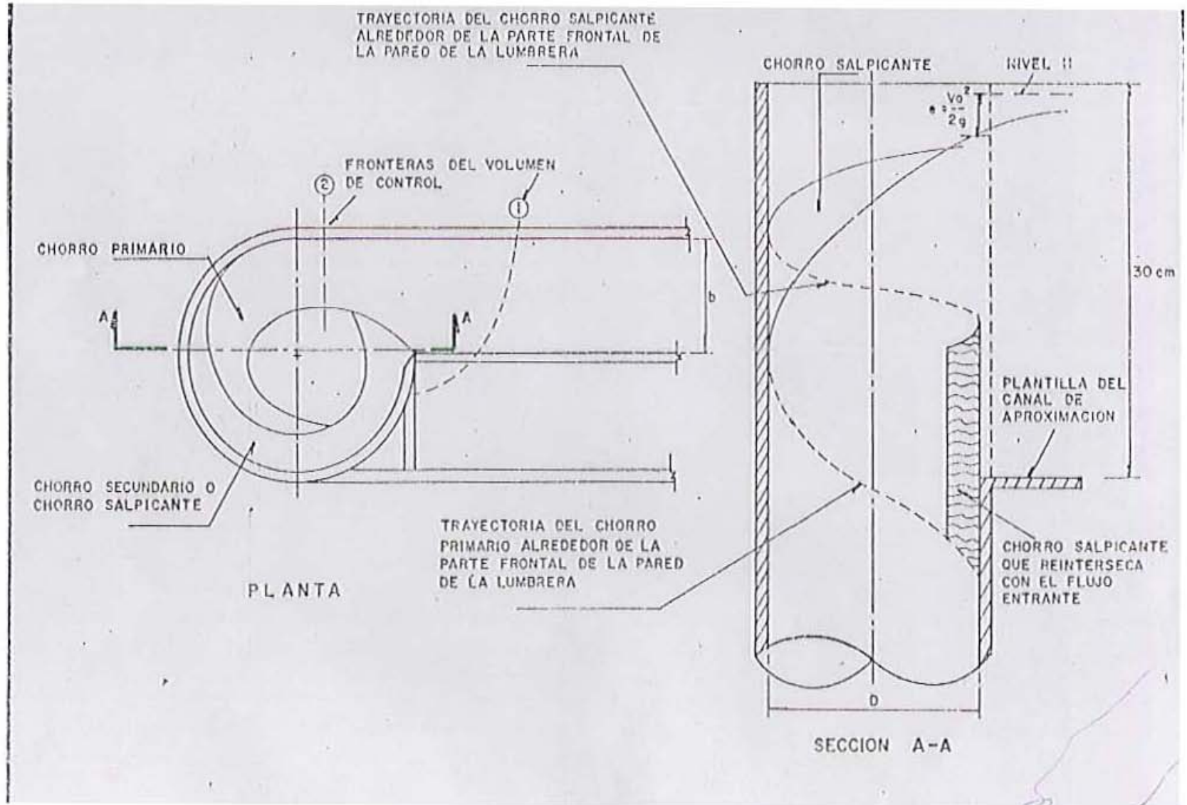
FIGURA 2.3 VARIABLES PARA EL FLUJO DE VORTICE
