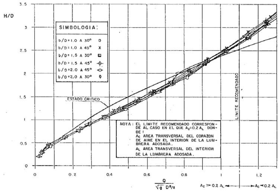
FIGURA 2.12 CURVAS DIMENSIONALES
