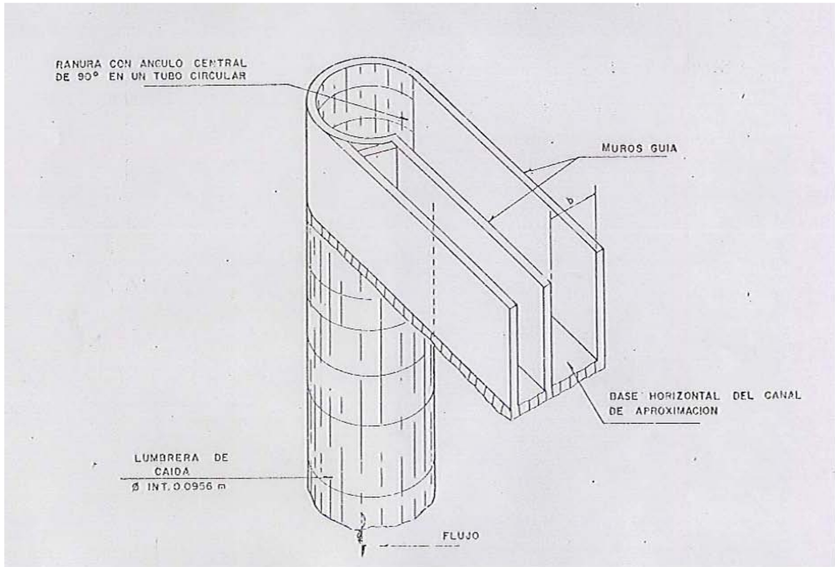
FIGURA 2.2 FIGURA CON MODIFICACION POR LA DGOH
