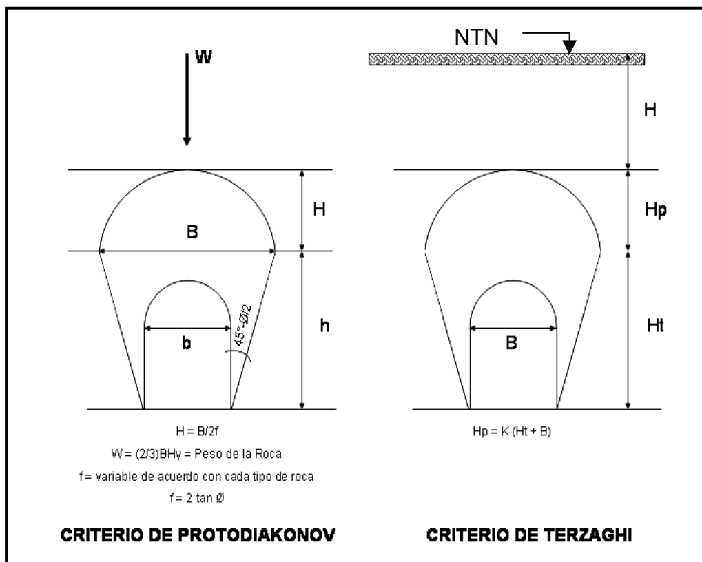
FIGURA IV.10 CRITERIO DE PROTODIAKONOV Y TERZAGHI PARA DETERMINAR LA CRAGA SOBRE LA ROCA
