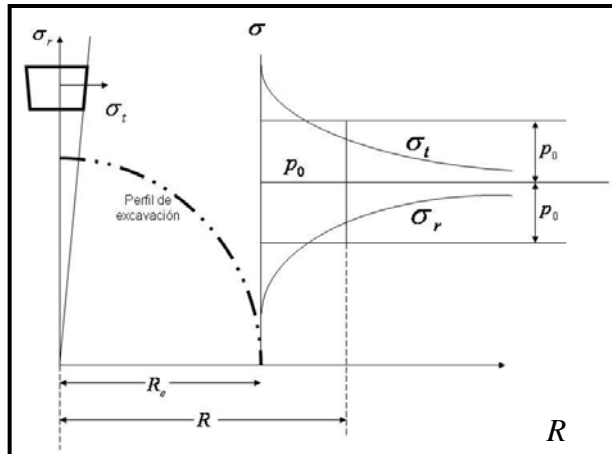
FIGURA IV.16 DIAGRAMA DE ESFUERZOS TANGENCIALES Y RADIALES
