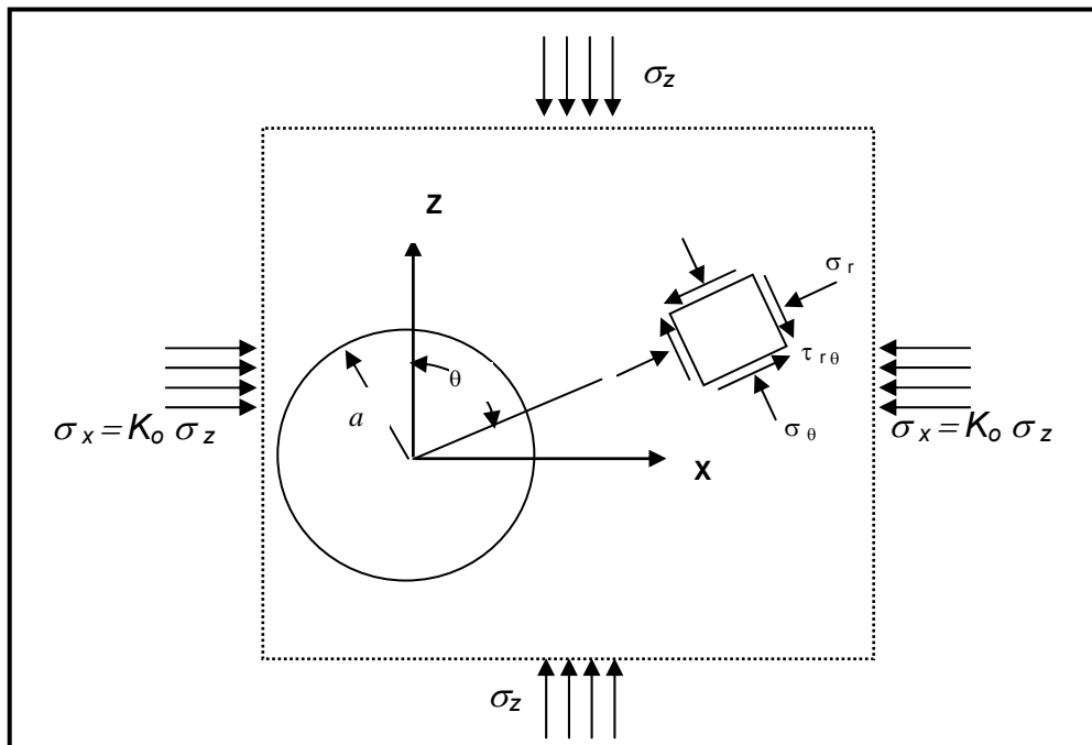
FIGURA III.3 ESTADO DE ESFUERZOS ALREDEDOR DE UNA EXCAVACIÓN
