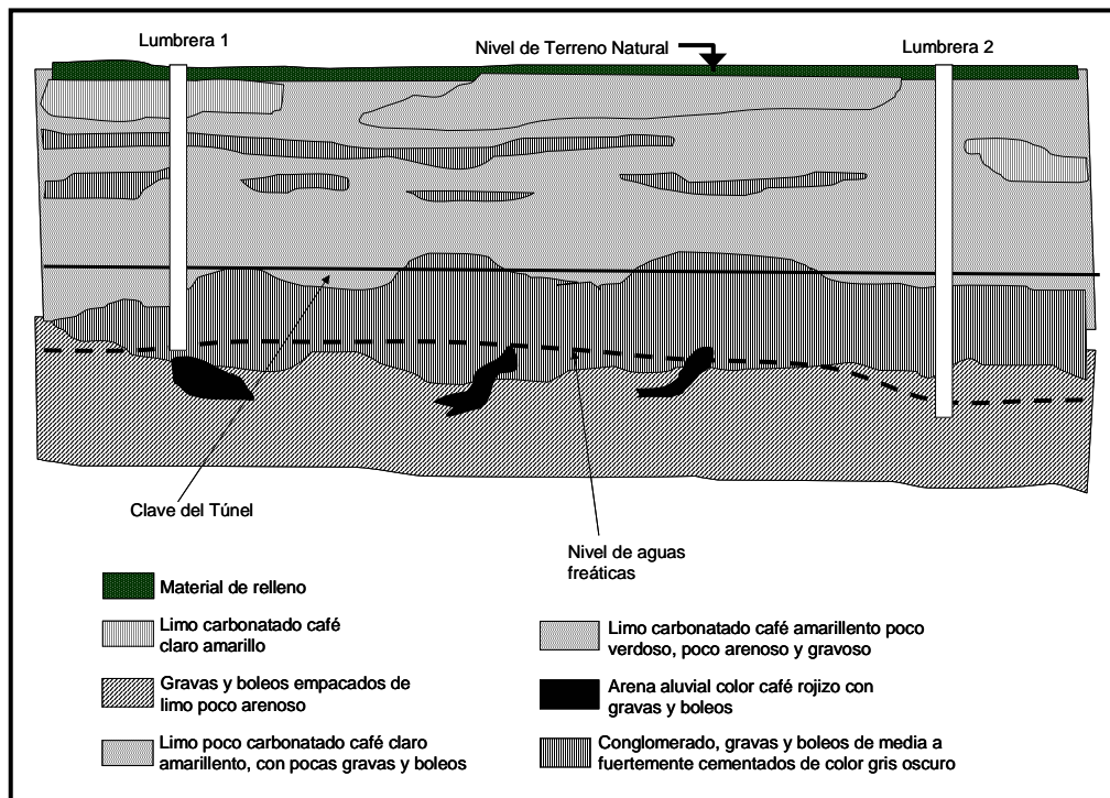
FIGURA V.2 PERFIL ESTRATIGRÁFICO
