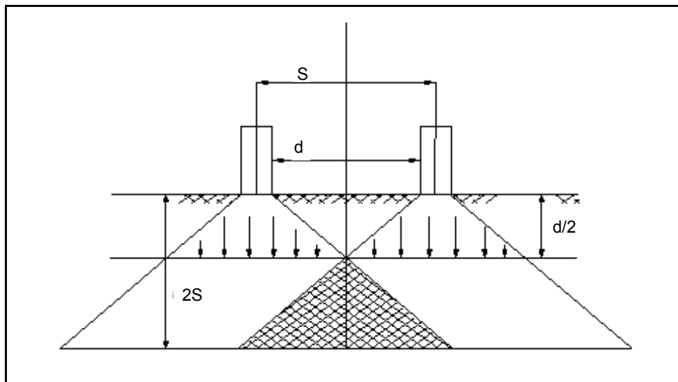
FIGURA I.5 “ESFUERZOS RESULTANTES EN LA ESTRUCTURA DEL PAVIMENTO EN RELACIÓN DE LA PROFUNDIDAD
