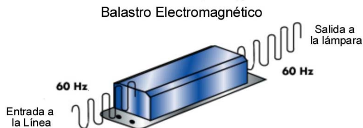
Figura 2.34A Frecuencia de Operación de un Balastro ELMG Fuente: Electronic Ballasts (28)
