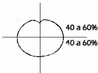
Figura 2.59 Flujo Luminoso Difuso-Directo Fuente: FIDE (48)
