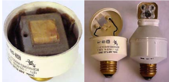
Figura 2.28 Vista del Núcleo del Balastro (Izq.) y Balastro Electromagnético (Der.) Fuente: Fotografías de Diversas Marcas
