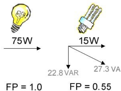
Figura 4.12 Comparación del FP, incandescente vs LFC. Fuente: PAESE
