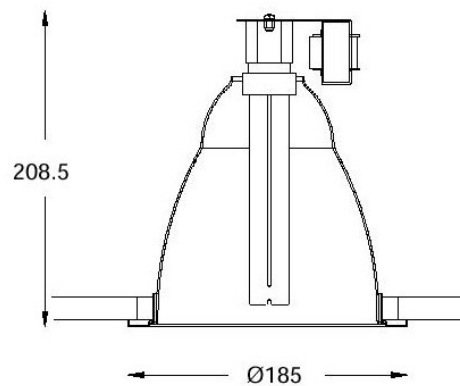
Figura 2.62 Luminario Tipo Downlight Lámpara-Vertical Fuente: Philips
