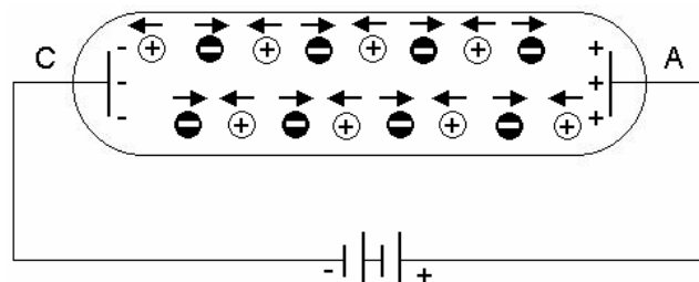
Figura 2.4 Representación Esquemática de una Descarga Gaseosa en DC Fuente: Principios Sobre Generación de Luz, Philips (7)
