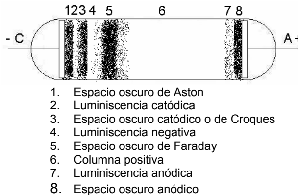
Figura 2.5 Zonas Brillantes y Oscuras de una Descarga Luminiscente en DC Fuente: Principios Sobre Generación de Luz, Philips (7)
