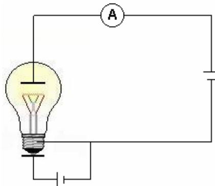
Figura 2.3 Efecto Termoiónico Fuente: Historia de la Tecnología del Semiconductor (6)
